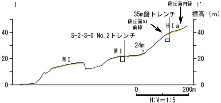
地形断面図
