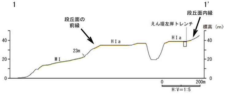
地形断面図
