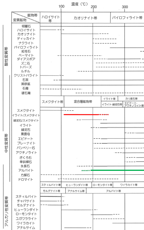
各変質帯に特徴的な鉱物とそれらの概略の生成温度 (井上(2003)に一部加筆)
