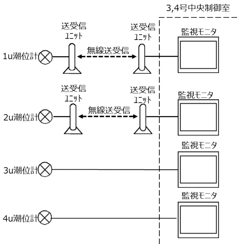
第 10.6.1.1.8 図 潮位計概念図
