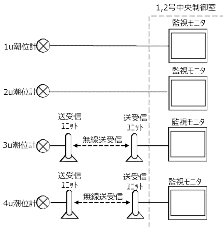
第10.6.1.1.8図 潮位計概念図
