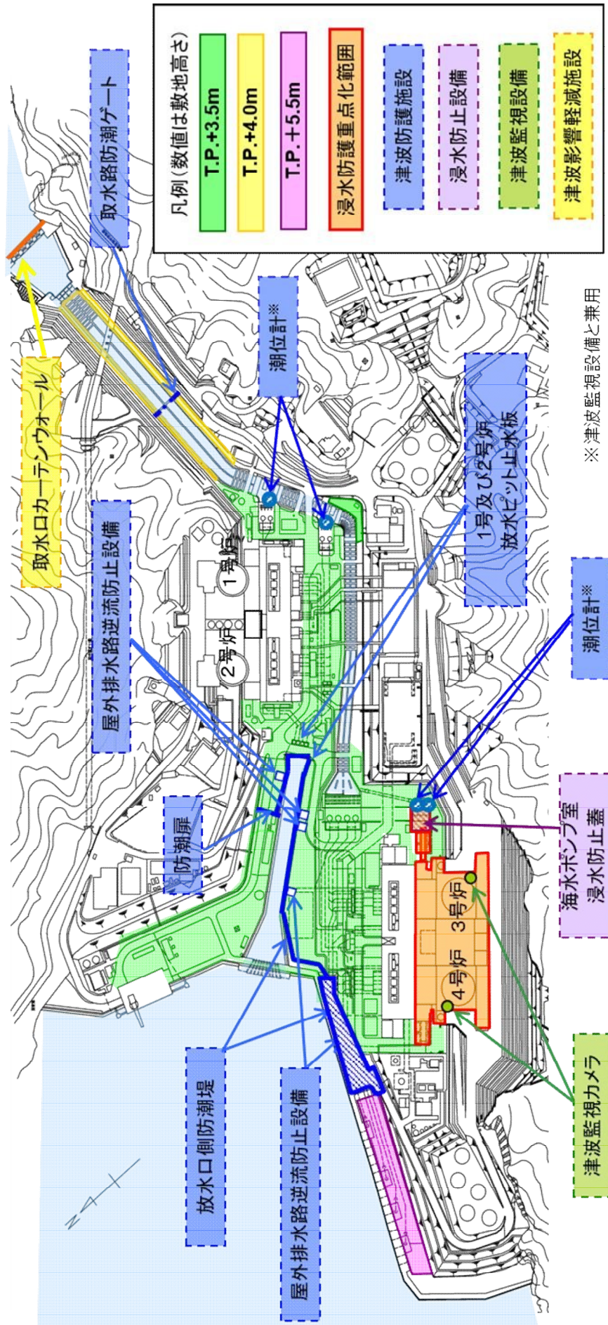
第 1.5.4 図 敷地の特性に応じた津波防護の概要
