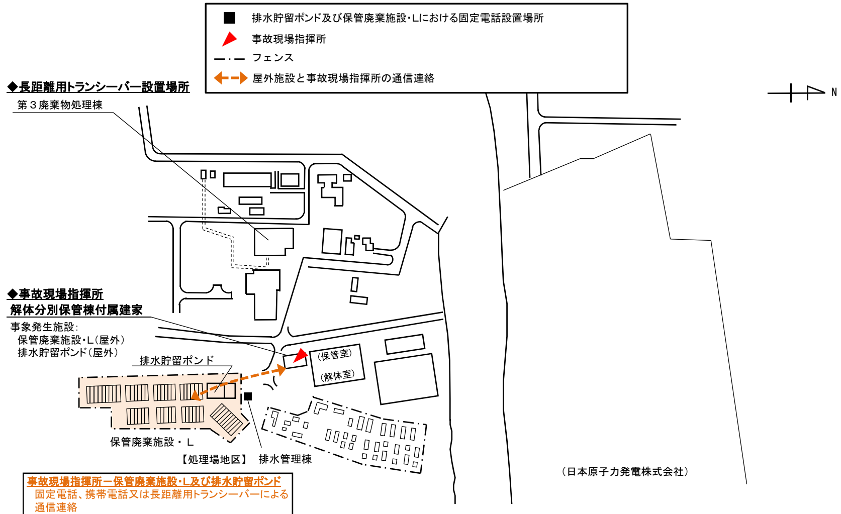
図-2.1 保管廃棄施設・L及び排水貯留ポンドの通信連絡設備の配置図
