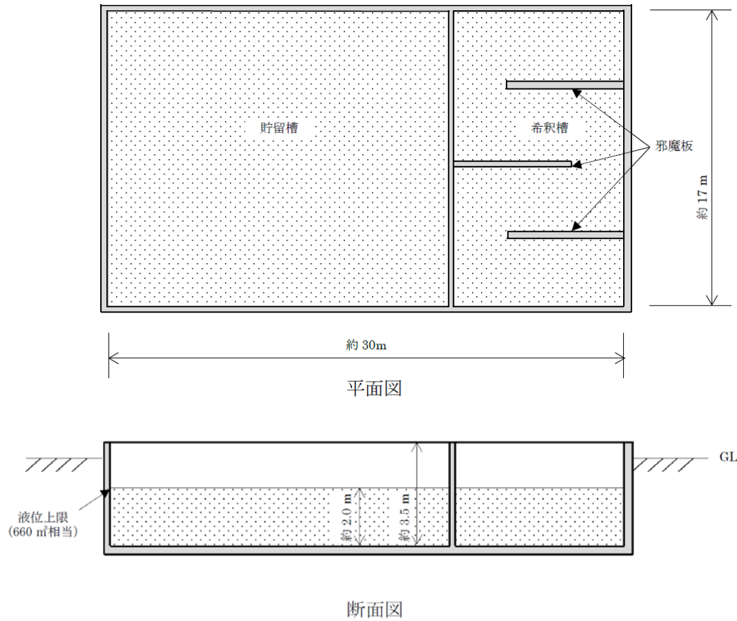
排水貯留ポンド概略図
