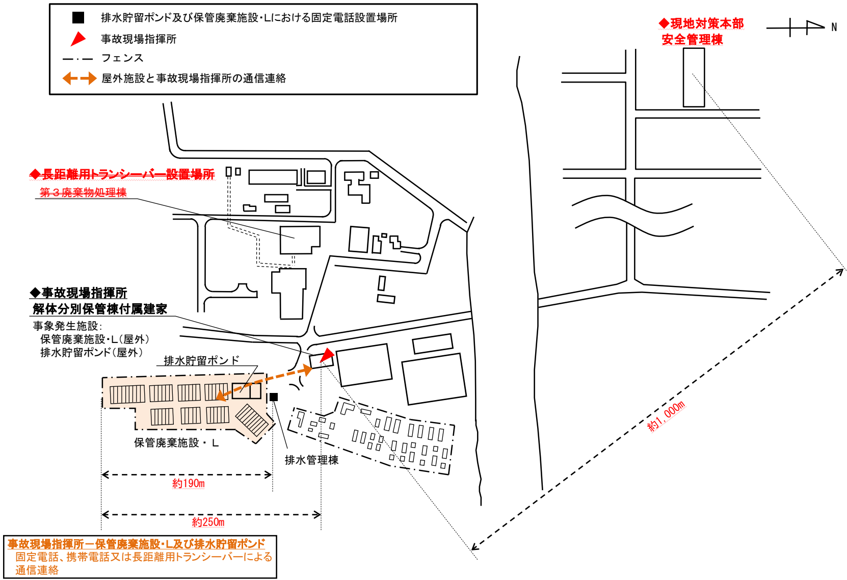
図-2.1 保管廃棄施設・L及び排水貯留 Pondの通信連絡設備の配置図
