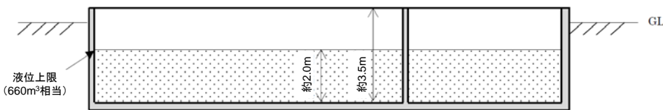
断面図
