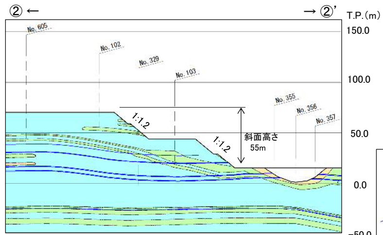
2号炉西側切取斜面(②-②' 断面, 岩級・シーム) 0 50m ※斜面頂部を対策工により切取済み
