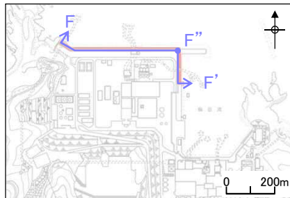
評価対象施設配置図
