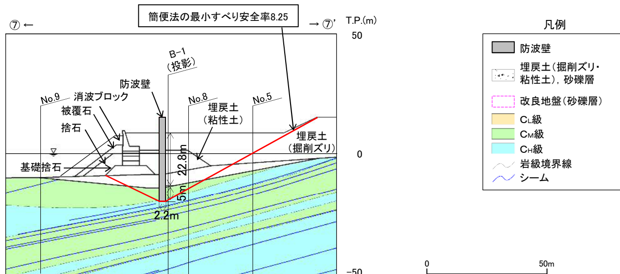
防波壁(多重鋼管杭式擁壁) ⑦-⑦'断面横断面図(岩級・シーム)
