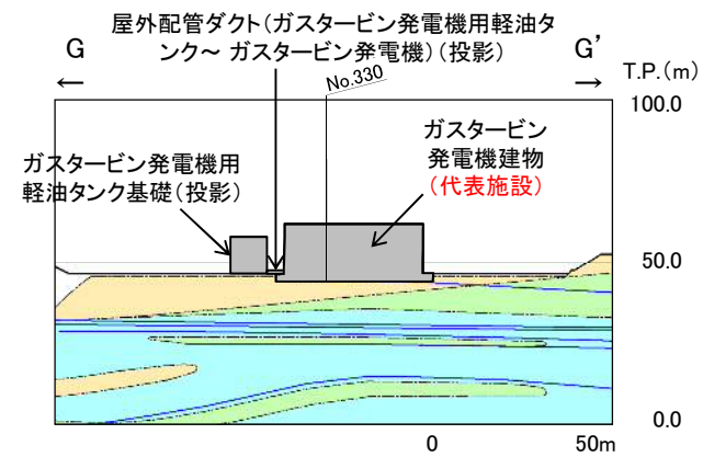
地質断面図(G-G'断面, 岩級・シーム)
