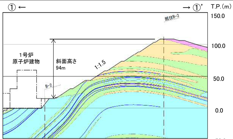
2号炉南側切取斜面(①-①' 断面, 岩級・シーム) 0 50m
