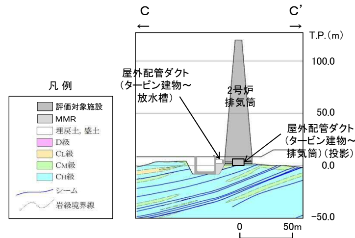
地質断面図(C-C'断面, 岩級・シーム)
