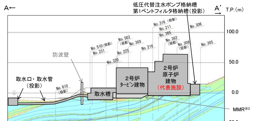
地質断面図(A-A'断面, 岩級・シーム)
