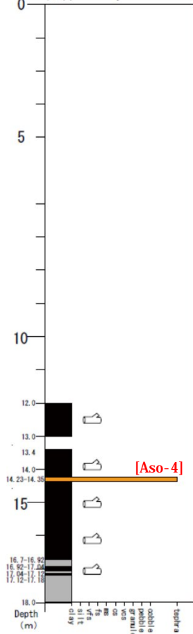
孔名: S-1B(EL=335.007m)
