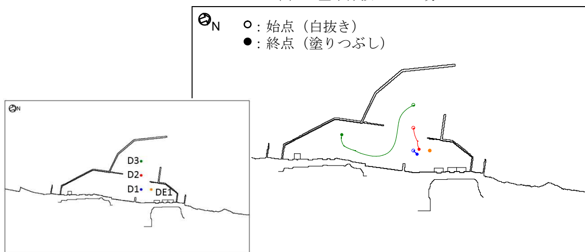
(2) 基準津波 2 : 240 分
