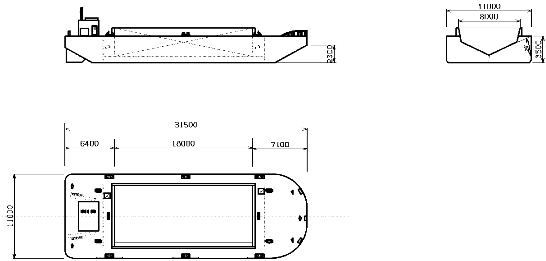
第1図 土運船の外形図
