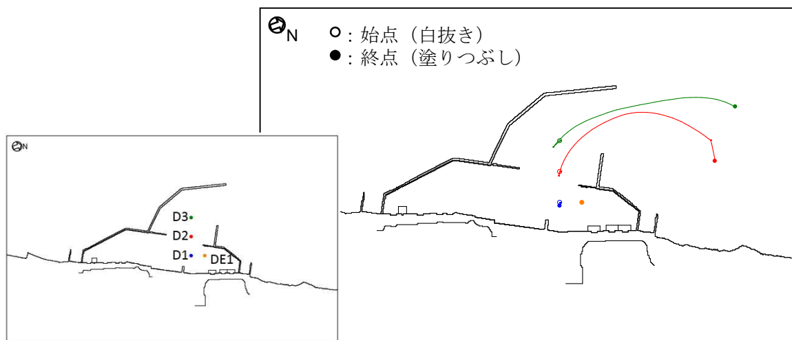
(3) 基準津波 3 : 240 分
