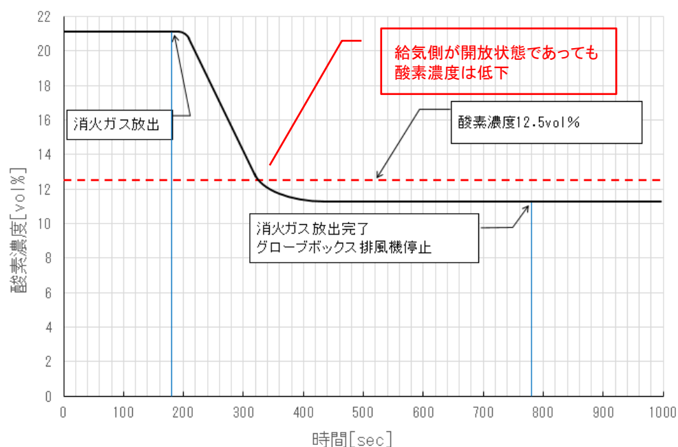
第2図 消火ガス放出時のGB内の酸素濃度の変化
