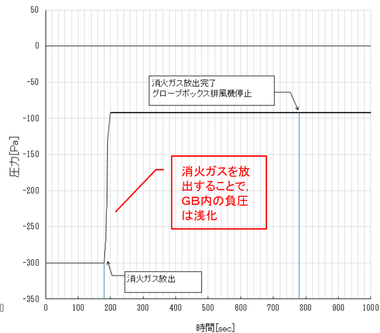
第3図 消火ガス放出時のGB内の負圧の変化
