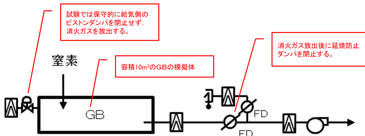
第1図 グローブボックス負圧確認試験装置の系統図
