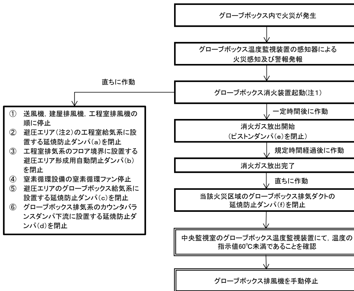
図1 【グローブボックス内火災が発生した際の感知から影響軽減までの流れ(フロー)】
