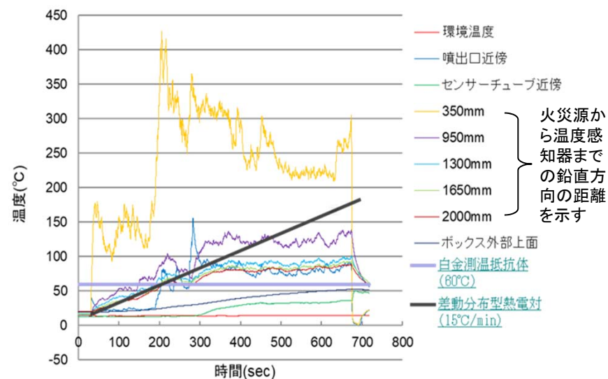
第2図 潤滑油火災を模擬した試験における温度変化
