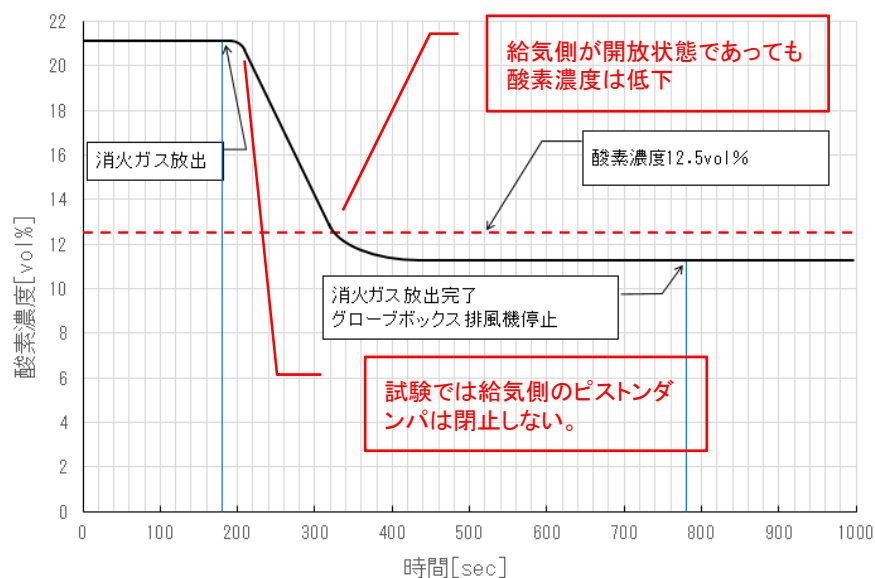
第1図 グローブボックス内に消火ガスを放出した際の酸素濃度変化
