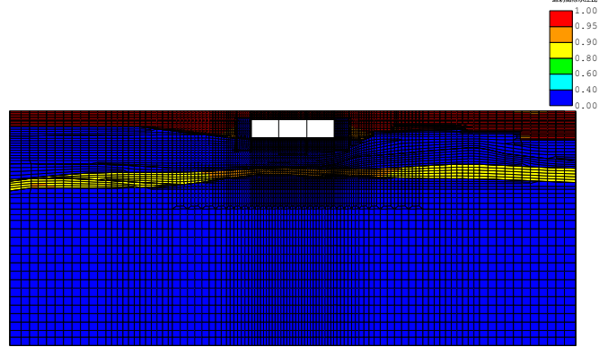
(FLIP応答コンター図) case3-Sa3-- 残留透射間隙水圧比分布図 TIME= 35.000s
