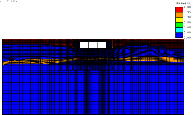
(FLIP応答コンター図) case3-Sa3-- 残留過剰間隙水圧比分布図 TIME= 61.000s
