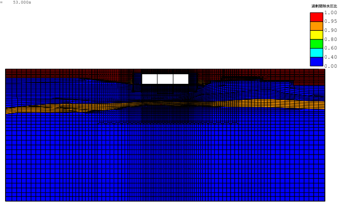
(FLIP応答コンター図) case3-Sa3-- 残留過剰間隙水圧比分布図 TIME= 53.000s
