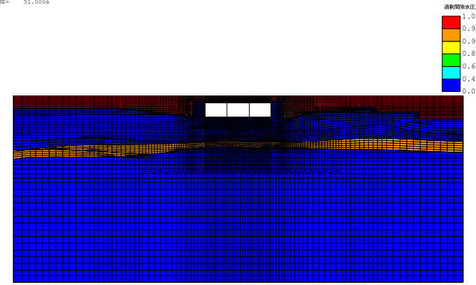
(FLIP応答コンター図) case3-Sa3-- 残留過剰間隙水圧比分布図 TIME= 51.000s
