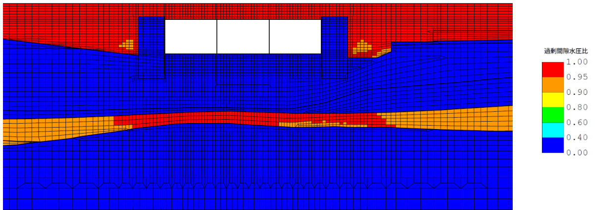
(b) 最大過剰間隙水圧比分布
