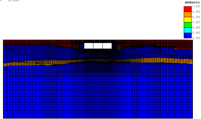
(FLIP応答コンター図) case3-Sa3-- 残留透射間隙水圧比分布図 TIME= 38.000s
