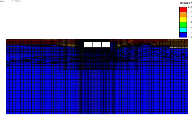
(FLIP応答コンター図) case3-Sa3-- 残留過剰間隙水圧比分布図 TIME= 12.000s
