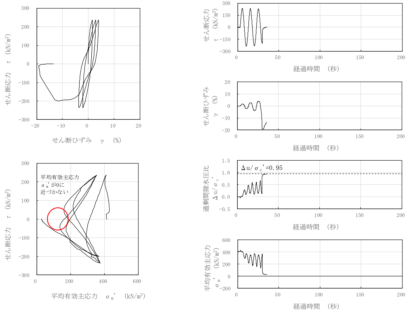
図 3-116 液状化試験結果 (A2s 層, FS02-2-9, GL. -22.85~23.00m, 有効拘束圧 412 \text{kN/m}^2 , せん断応力比=0.575)
