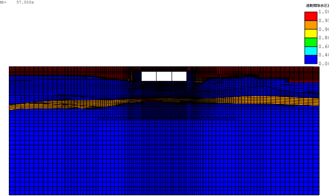
(FLIP応答コンター図) case3-Sa3-- 残留過剰間隙水圧比分布図 TIME= 57.000s
