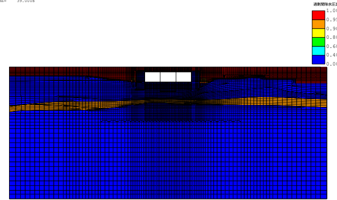
(FLIP応答コンター図) case3-Sa3-- 残留透射間隙水圧比分布図 TIME= 39.000s
