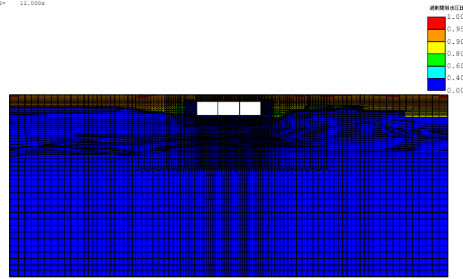
(FLIP応答コンター図) case3-Sa3-- 残留過剰間隙水圧比分布図 TIME= 11.000s
