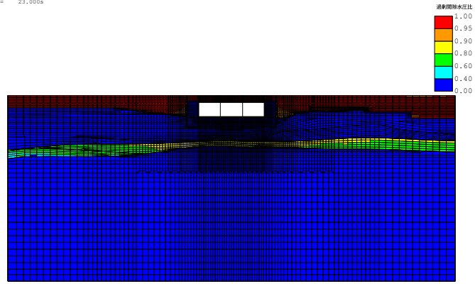
《FLIP応答コンター図》 case3-Sa3-- 残留過剰間隙水圧比分布図 TIME= 23.000s
