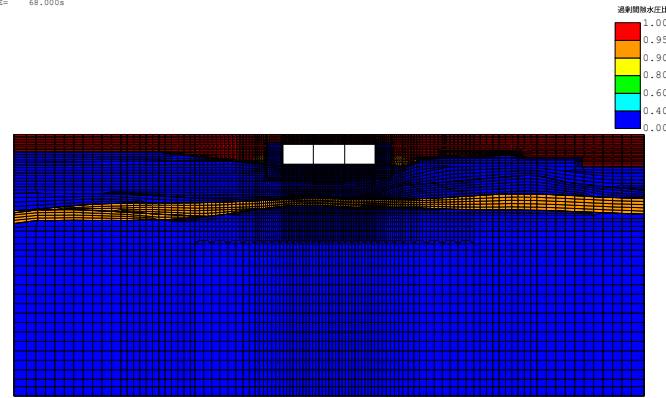
(FLIP応答コンター図) case3-Sa3-- 残留透射間隙水圧比分布図 TIME= 68.000s
