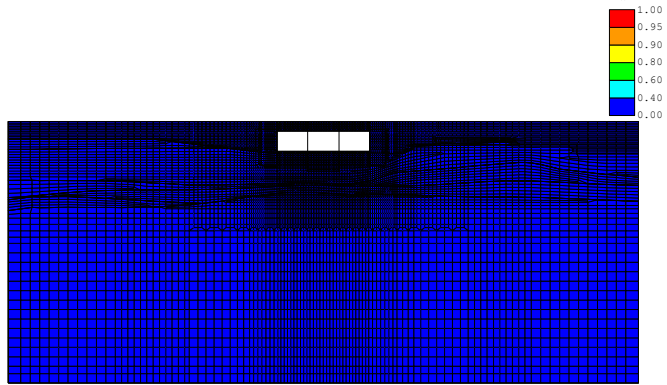
(FLIP応答コンター図) case3-Sa3-- 残留透射間隙水圧比分布図 TIME= 4.000s
