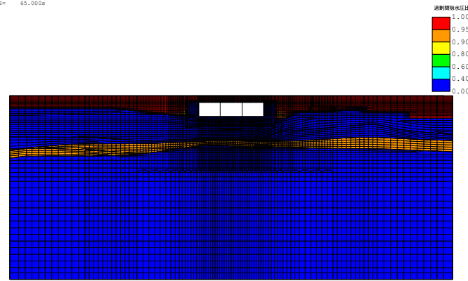
(FLIP応答コンター図) case3-Sa3-- 残留透射間隙水圧比分布図 TIME= 65.000s
