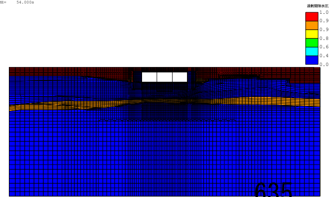
(FLIP応答コンター図) case3-Sa3-- 残留過剰間隙水圧比分布図 TIME= 54.000s
