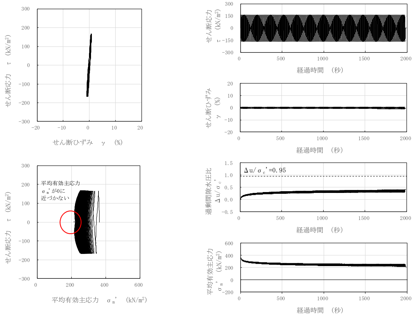
図 3-104 液状化試験結果 (A2s 層, FS-3-1-3, GL. -27.03~27.18m, 有効拘束圧 363\text{kN/m}^2 , せん断応力比=0.458)
