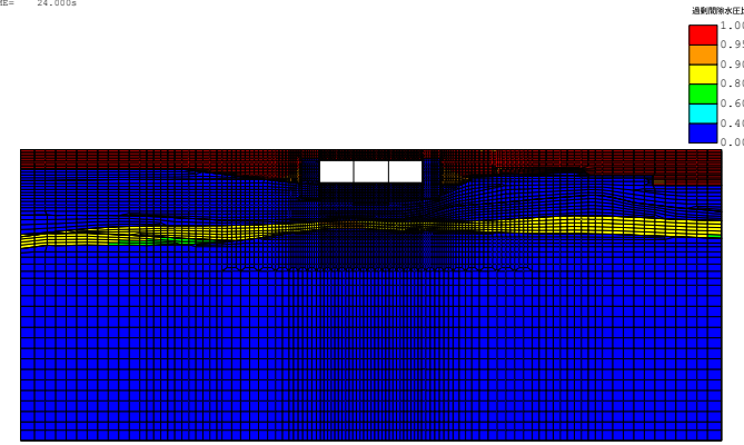
《FLIP応答コンター図》 case3-Sa3-- 残留過剰間隙水圧比分布図 TIME= 24.000s
