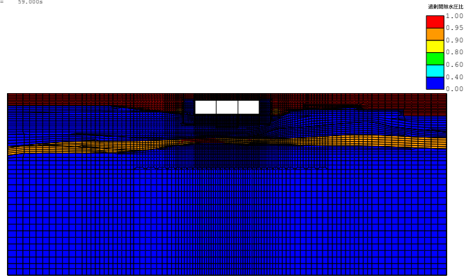
(FLIP応答コンター図) case3-Sa3-- 残留過剰間隙水圧比分布図 TIME= 59.000s
