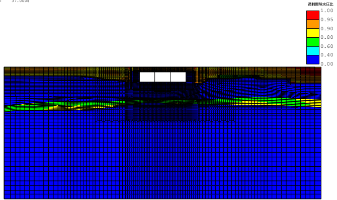
(FLIP応答コンター図) case3-Sa3-- 残留透射間隙水圧比分布図 TIME= 37.000s
