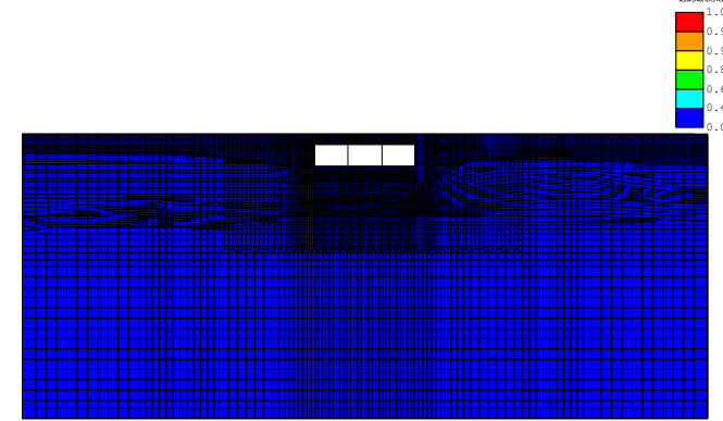
(FLIP応答コンター図) case3-Sa3-- 残留透射間隙水圧比分布図 TIME= 3.000s
