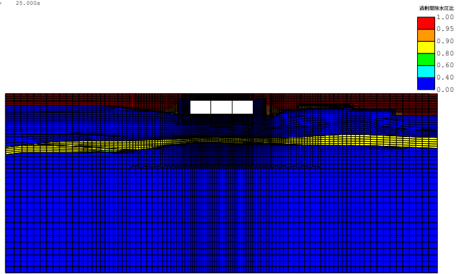
《FLIP応答コンター図》 case3-Sa3-- 残留過剰間隙水圧比分布図 TIME= 25.000s
