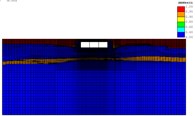
(FLIP応答コンター図) case3-Sa3-- 残留過剰間隙水圧比分布図 TIME= 58.000s
