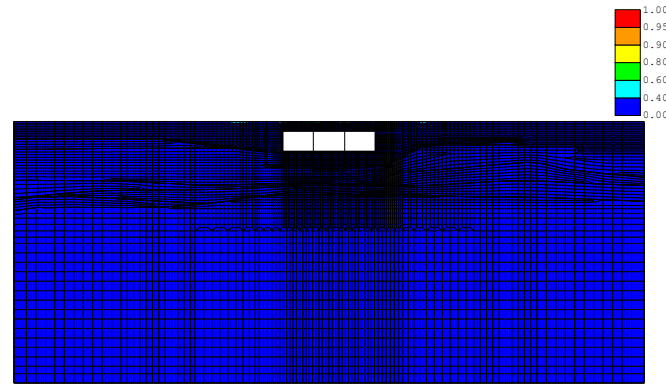
(FLIP応答コンター図) case3-Sa3-- 残留透射間隙水圧比分布図 TIME= 5.000s
