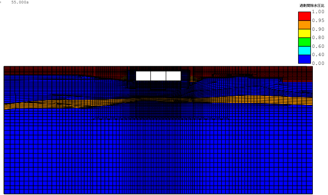
(FLIP応答コンター図) case3-Sa3-- 残留過剰間隙水圧比分布図 TIME= 55.000s
