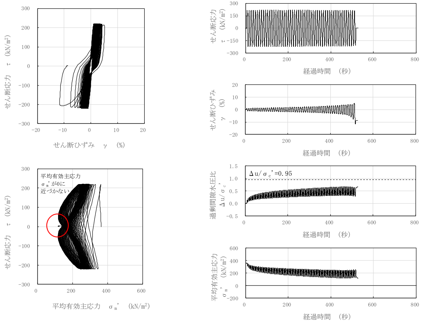
図 3-100 液状化試験結果 (A2s 層, FS-4-1-3, GL. -27.12~27.29m, 有効拘束圧 363\text{kN/m}^2 , せん断応力比=0.605)
