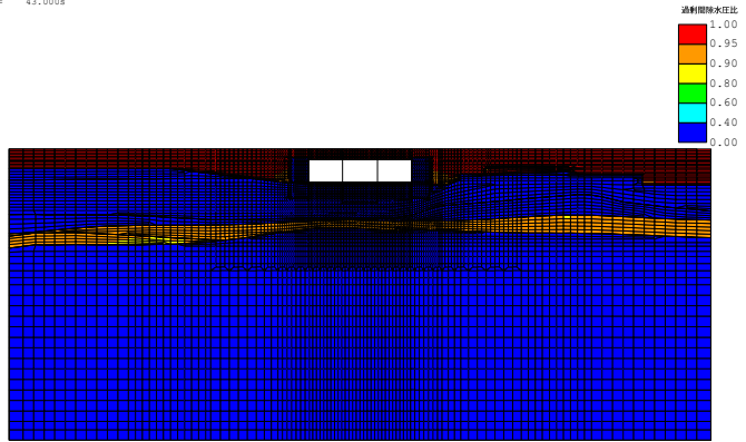
(FLIP応答コンター図) case3-Sa3-- 残留透射間隙水圧比分布図 TIME= 43.000s
