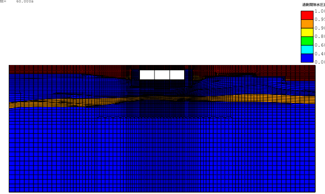
(FLIP応答コンター図) case3-Sa3-- 残留過剰間隙水圧比分布図 TIME= 60.000s
