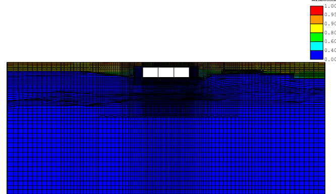
(FLIP応答コンター図) case3-Sa3-- 残留透射間隙水圧比分布図 TIME= 8.000s
