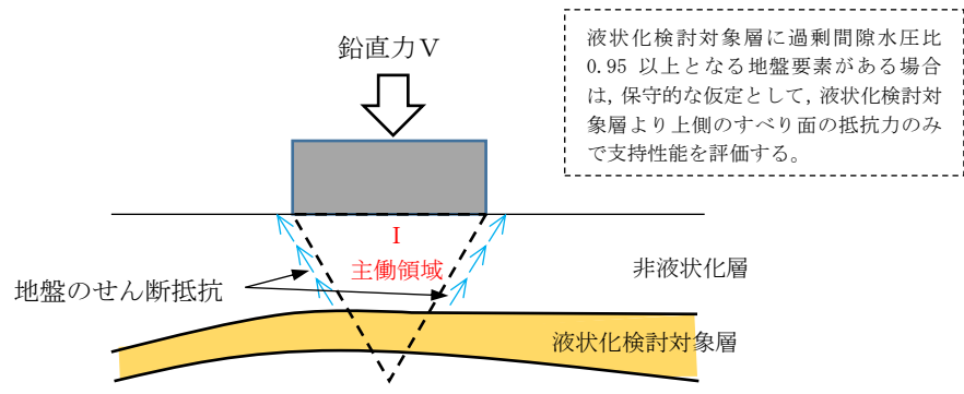
(a) 液化化検討対象層を考慮した支持性能評価の概念図
