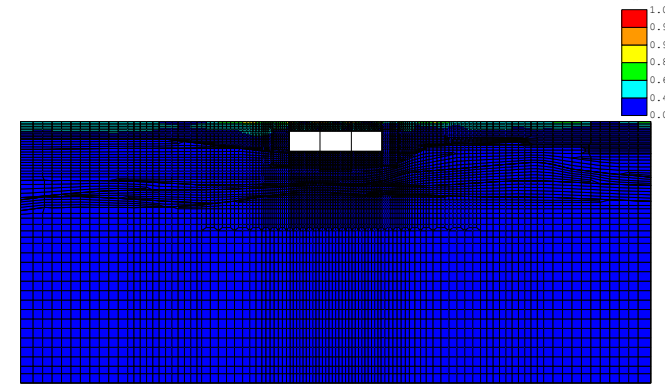
(FLIP応答コンター図) case3-Sa3-- 残留透射間隙水圧比分布図 TIME= 6.000s
