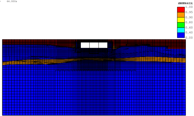
(FLIP応答コンター図) case3-Sa3-- 残留透射間隙水圧比分布図 TIME= 64.000s
