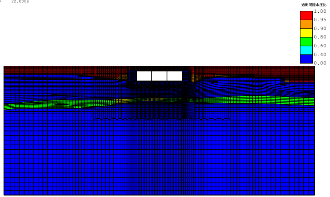
《FLIP応答コンター図》 case3-Sa3-- 残留過剰間隙水圧比分布図 TIME= 22.000s
