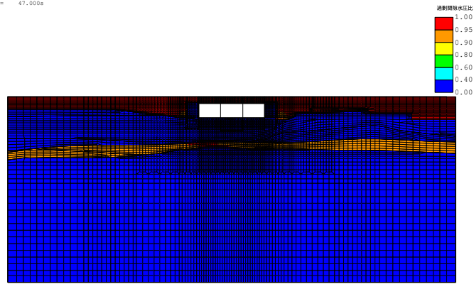
(FLIP応答コンター図) case3-Sa3-- 残留過剰間隙水圧比分布図 TIME= 47.000s
