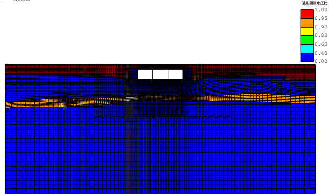
(FLIP応答コンター図) case3-Sa3-- 残留透射間隙水圧比分布図 TIME= 41.000s
