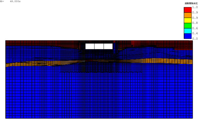
(FLIP応答コンター図) case3-Sa3-- 残留過剰間隙水圧比分布図 TIME= 48.000s
