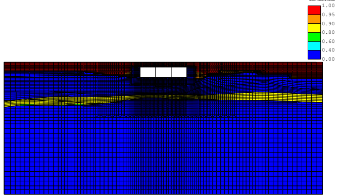
(FLIP応答コンター図) case3-Sa3-- 残留透射間隙水圧比分布図 TIME= 28.000s
