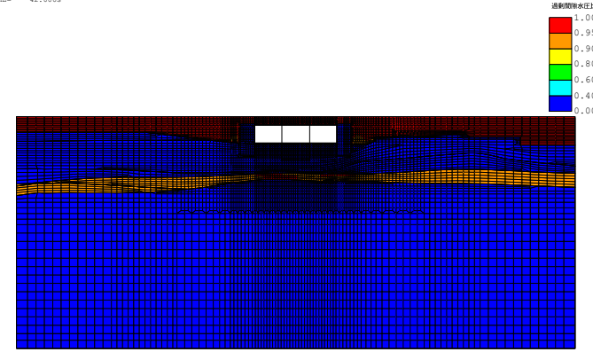
(FLIP応答コンター図) case3-Sa3-- 残留透射間隙水圧比分布図 TIME= 42.000s
