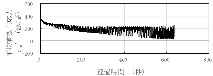
図 3-95 液状化試験結果 (A2s 層, FS-2-2-2, GL. -27.85~28.00m, 有効拘束圧 363kN/m 2 , せん断応力比=0.507)
