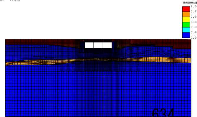
(FLIP応答コンター図) case3-Sa3-- 残留透射間隙水圧比分布図 TIME= 45.000s
