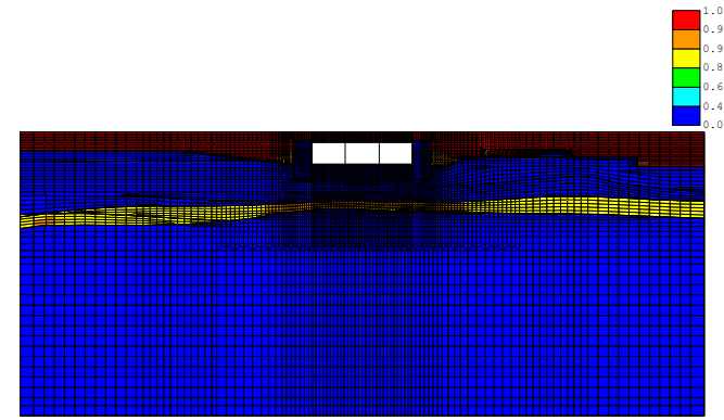
(FLIP応答コンター図) case3-Sa3-- 残留透射間隙水圧比分布図 TIME= 33.000s
