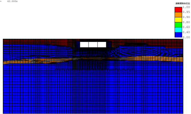
(FLIP応答コンター図) case3-Sa3-- 残留過剰間隙水圧比分布図 TIME= 62.000s
