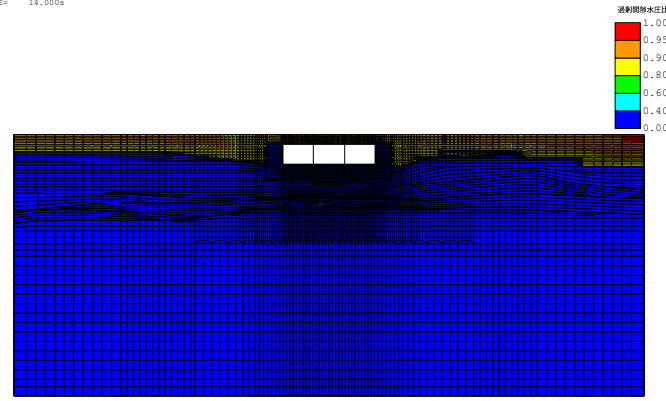
(FLIP応答コンター図) case3-Sa3-- 残留過剰間隙水圧比分布図 TIME= 14.000s
