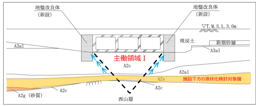
(b) 6号機取水路 (漸縮部) の例
