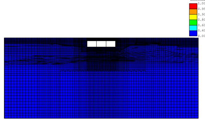
(FLIP応答コンター図) case3-Sa3-- 残留透射間隙水圧比分布図 TIME= 2.000s
