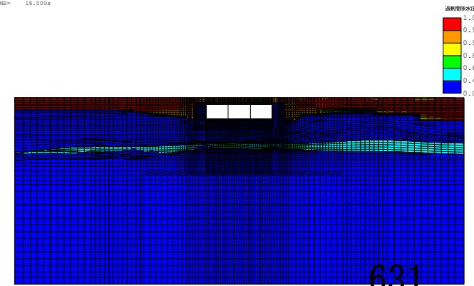
(FLIP応答コンター図) case3-Sa3-- 残留過剰間隙水圧比分布図 TIME= 18.000s
