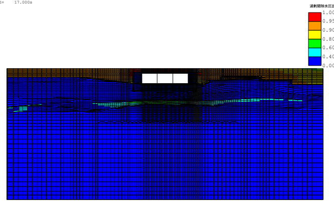
(FLIP応答コンター図) case3-Sa3-- 残留過剰間隙水圧比分布図 TIME= 17.000s
