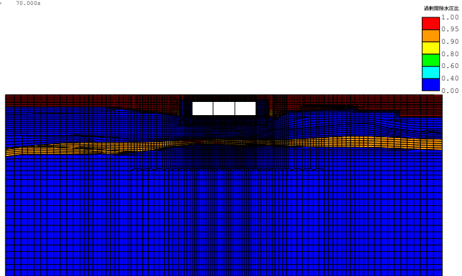
(FLIP応答コンター図) case3-Sa3-- 残留透射間隙水圧比分布図 TIME= 70.000s
