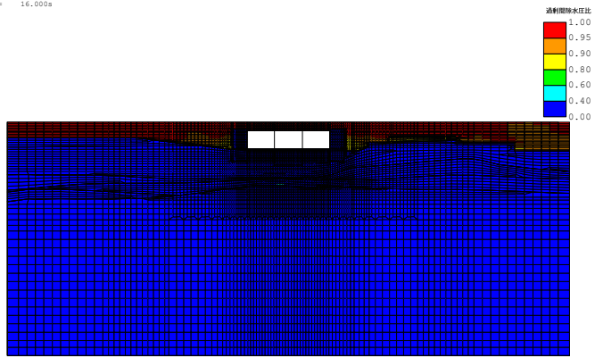
(FLIP応答コンター図) case3-Sa3-- 残留過剰間隙水圧比分布図 TIME= 16.000s
