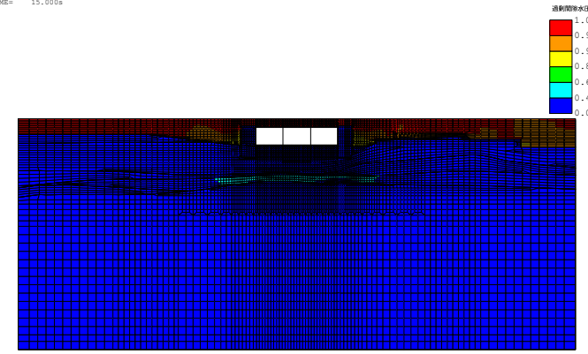
(FLIP応答コンター図) case3-Sa3-- 残留過剰間隙水圧比分布図 TIME= 15.000s
