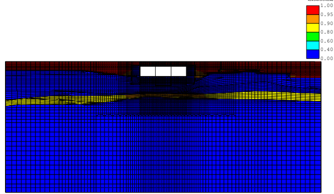
(FLIP応答コンター図) case3-Sa3-- 残留透射間隙水圧比分布図 TIME= 29.000s
