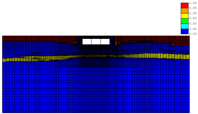
(FLIP応答コンター図) case3-Sa3-- 残留透射間隙水圧比分布図 TIME= 31.000s
