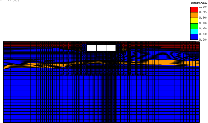
(FLIP応答コンター図) case3-Sa3-- 残留透射間隙水圧比分布図 TIME= 44.000s
