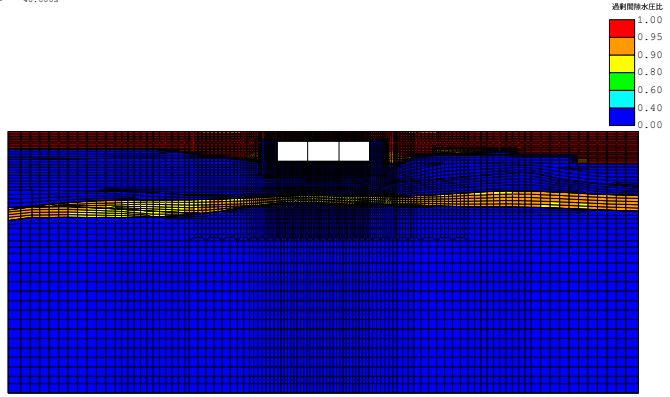
(FLIP応答コンター図) case3-Sa3-- 残留透射間隙水圧比分布図 TIME= 40.000s
