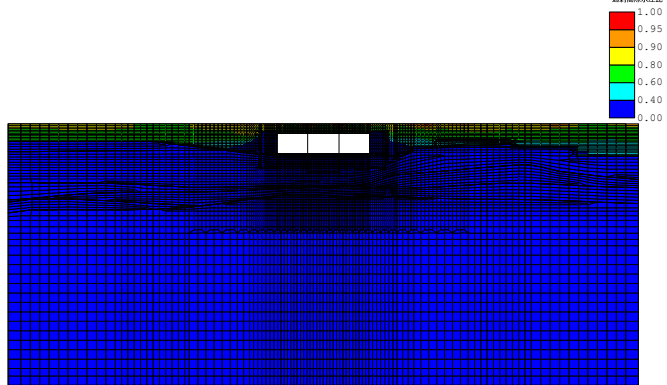
(FLIP応答コンター図) case3-Sa3-- 残留透射間隙水圧比分布図 TIME= 7.000s
