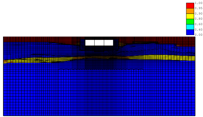
(FLIP応答コンター図) case3-Sa3-- 残留透射間隙水圧比分布図 TIME= 32.000s
