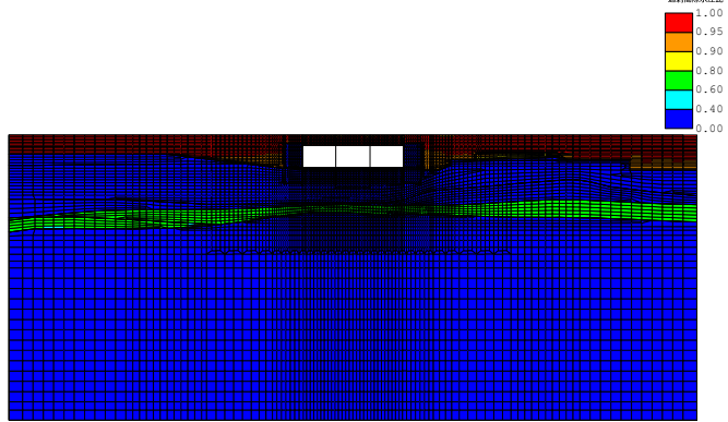
(FLIP応答コンター図) case3-Sa3-- 残留透射間隙水圧比分布図 TIME= 34.000s
