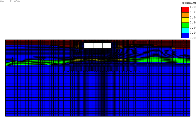
《FLIP応答コンター図》 case3-Sa3-- 残留過剰間隙水圧比分布図 TIME= 21.000s
