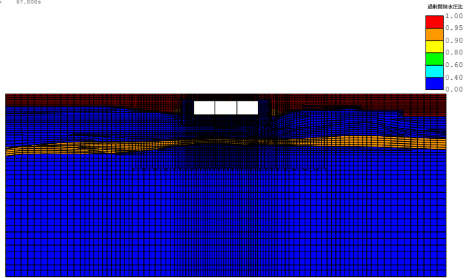
(FLIP応答コンター図) case3-Sa3-- 残留透射間隙水圧比分布図 TIME= 67.000s
