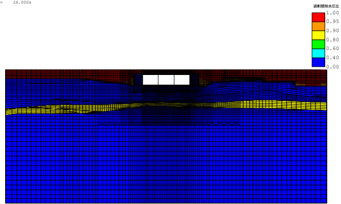
《FLIP応答コンター図》 case3-Sa3-- 残留過剰間隙水圧比分布図 TIME= 26.000s
