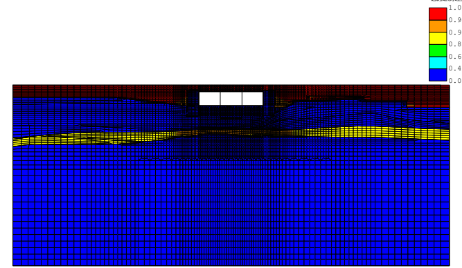
(FLIP応答コンター図) case3-Sa3-- 残留透射間隙水圧比分布図 TIME= 30.000s
