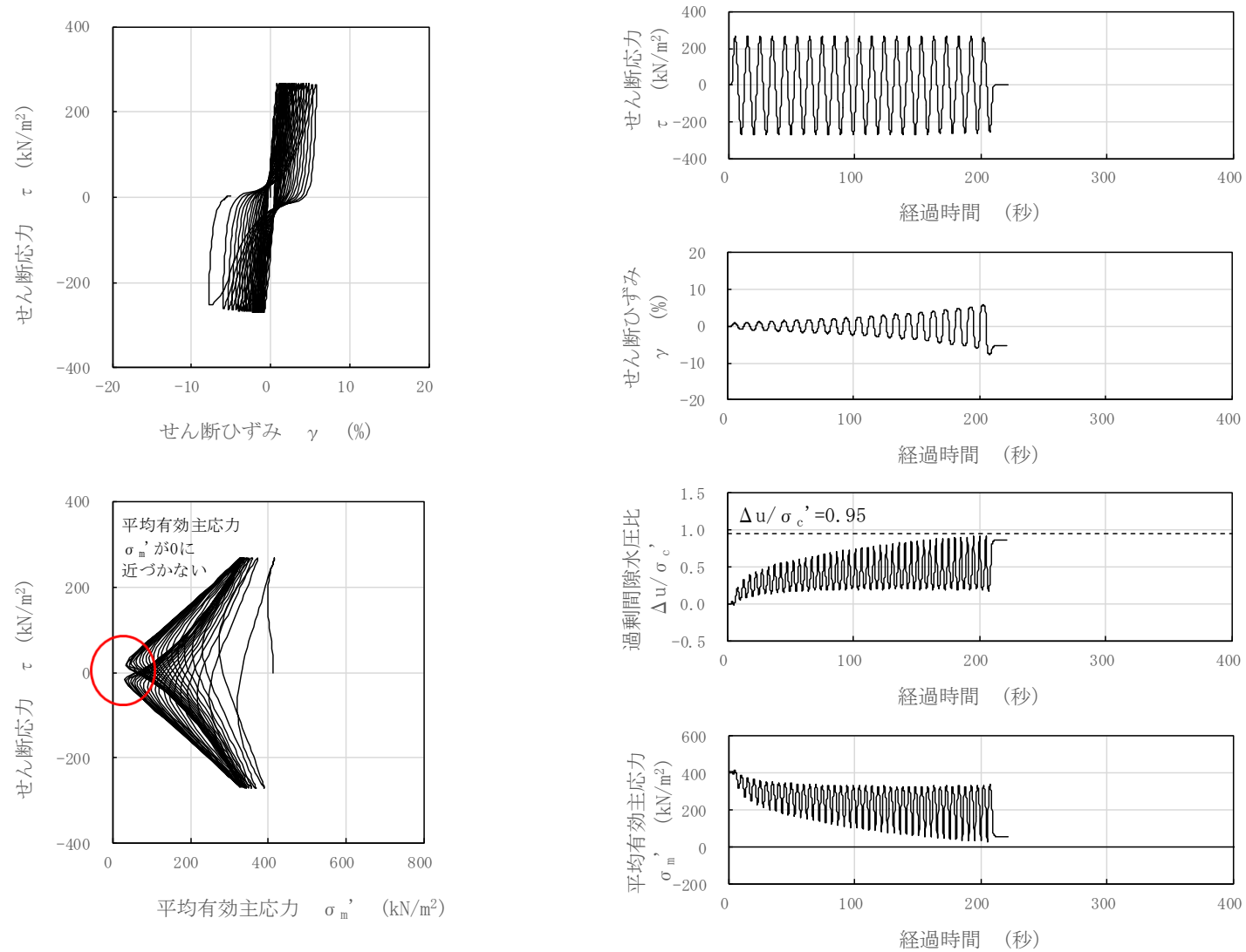
図 3-114 液状化試験結果 (A2s 層, FS-4-8-5, GL. -33.40~33.55m, 有効拘束圧 412kN/m 2 , せん断応力比=0.651)
