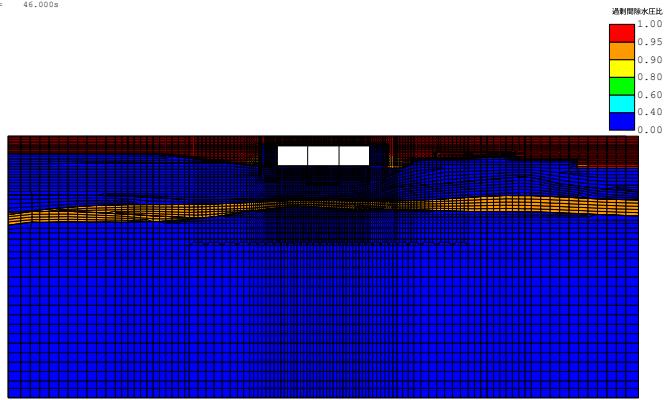
(FLIP応答コンター図) case3-Sa3-- 残留過剰間隙水圧比分布図 TIME= 46.000s
