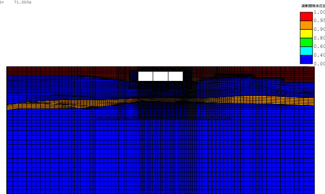
(FLIP応答コンター図) case3-Sa3-- 残留透射間隙水圧比分布図 TIME= 71.000s
