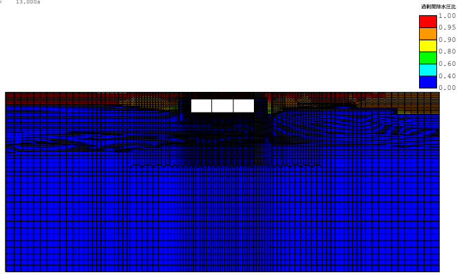
(FLIP応答コンター図) case3-Sa3-- 残留過剰間隙水圧比分布図 TIME= 13.000s
