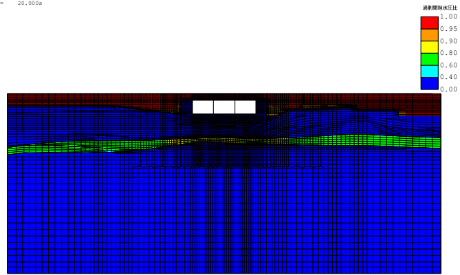
《FLIP応答コンター図》 case3-Sa3-- 残留過剰間隙水圧比分布図 TIME= 20.000s
