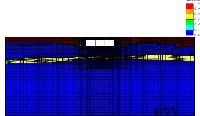
(FLIP応答コンター図) case3-Sa3-- 残留透射間隙水圧比分布図 TIME= 36.000s
