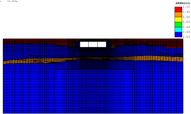
(FLIP応答コンター図) case3-Sa3-- 残留過剰間隙水圧比分布図 TIME= 56.000s
