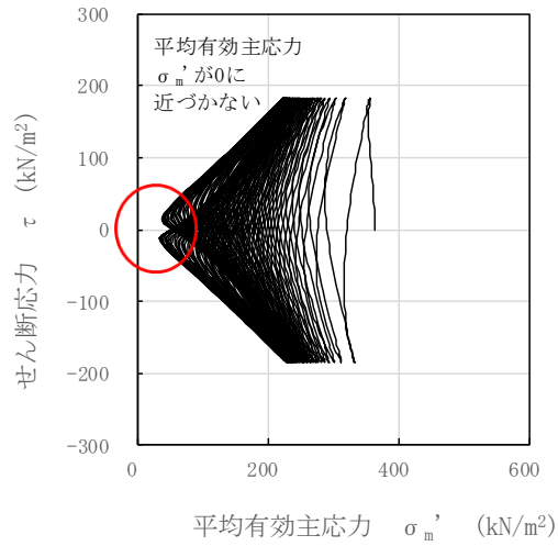
図 3-95 液状化試験結果 (A2s 層, FS-2-2-2, GL. -27.85~28.00m, 有効拘束圧 363kN/m 2 , せん断応力比=0.507)
