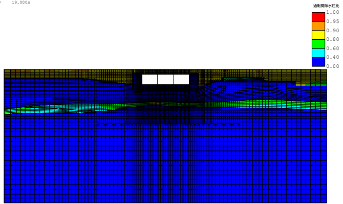
《FLIP応答コンター図》 case3-Sa3-- 残留過剰間隙水圧比分布図 TIME= 19.000s
