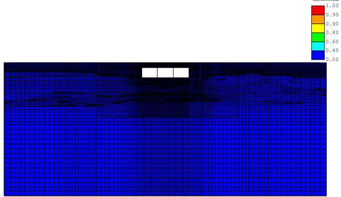
(FLIP応答コンター図) case3-Sa3-- 残留透射間隙水圧比分布図 TIME= 1.000s
