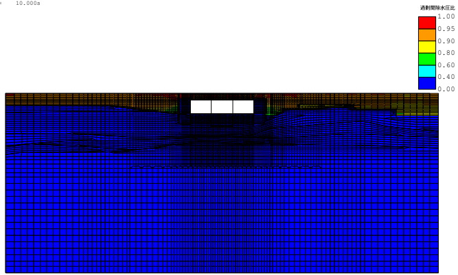
(FLIP応答コンター図) case3-Sa3-- 残留過剰間隙水圧比分布図 TIME= 10.000s
