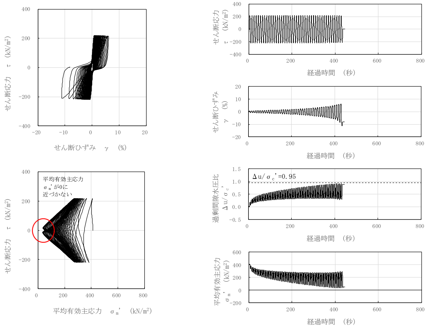
図 3-112 液状化試験結果 (A2s 層, FS-4-8-3, GL. -33.10~33.25m, 有効拘束圧 412kN/m 2 , せん断応力比=0.530)
