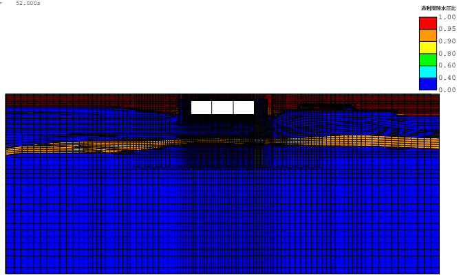
(FLIP応答コンター図) case3-Sa3-- 残留過剰間隙水圧比分布図 TIME= 52.000s
