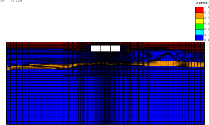
(FLIP応答コンター図) case3-Sa3-- 残留透射間隙水圧比分布図 TIME= 69.000s
