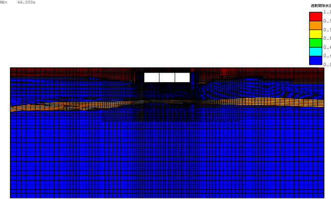
(FLIP応答コンター図) case3-Sa3-- 残留透射間隙水圧比分布図 TIME= 66.000s
