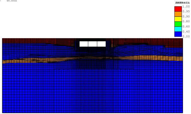
(FLIP応答コンター図) case3-Sa3-- 残留過剰間隙水圧比分布図 TIME= 49.000s
