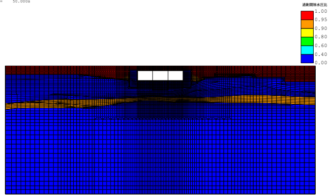
(FLIP応答コンター図) case3-Sa3-- 残留過剰間隙水圧比分布図 TIME= 50.000s
