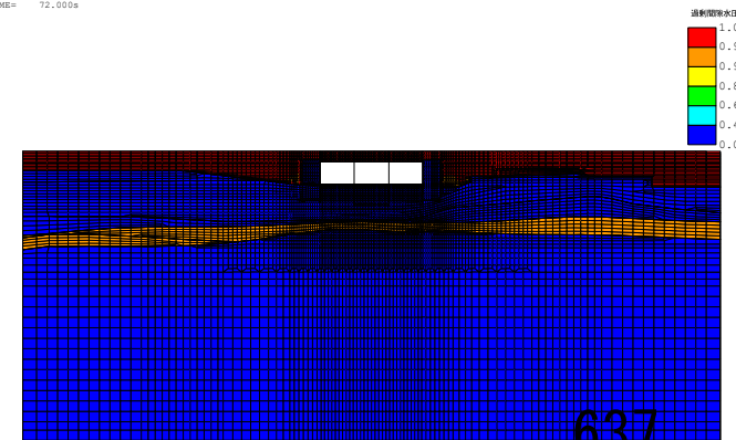
(FLIP応答コンター図) case3-Sa3-- 残留透射間隙水圧比分布図 TIME= 72.000s
