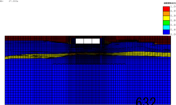
《FLIP応答コンター図》 case3-Sa3-- 残留過剰間隙水圧比分布図 TIME= 27.000s
