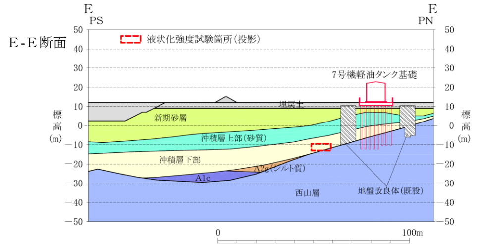
図 4-18 沖積層下部の液状化強度試験の試料採取位置
