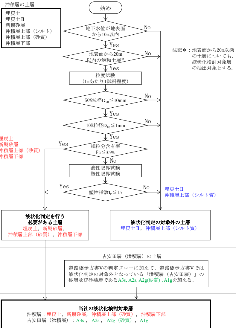
図4-11 液状化検討対象層の抽出フロー
