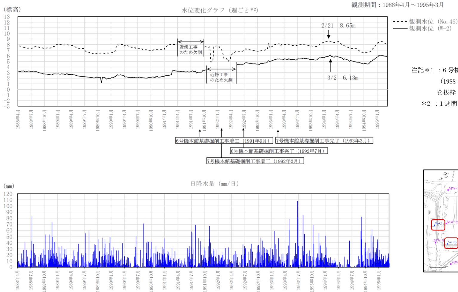
図 1-10 建設時の地下水位観測記録と降水量データ
