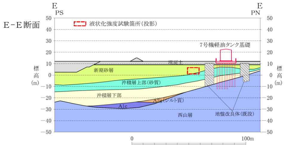
図 4-16 新期砂層の液状化強度試験の試料採取位置
