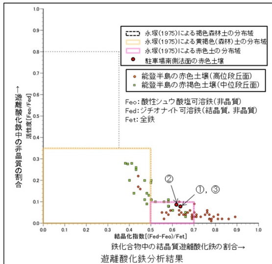
遊離酸化鉄分析結果
