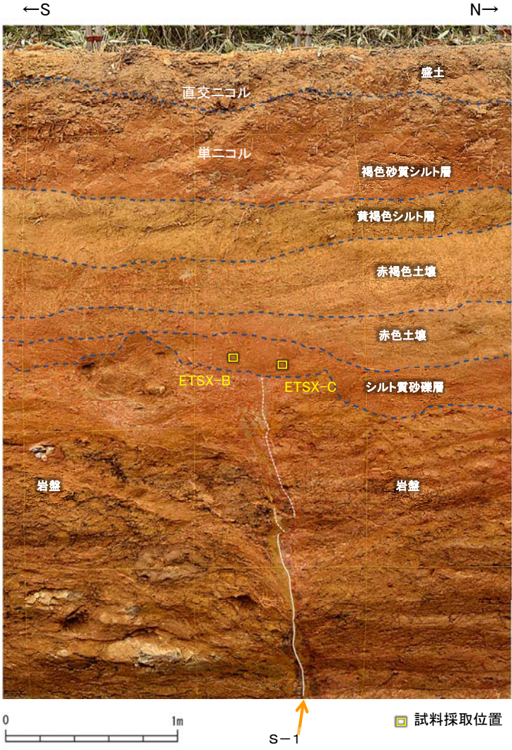
えん堤左岸トレンチ 西壁面写真
