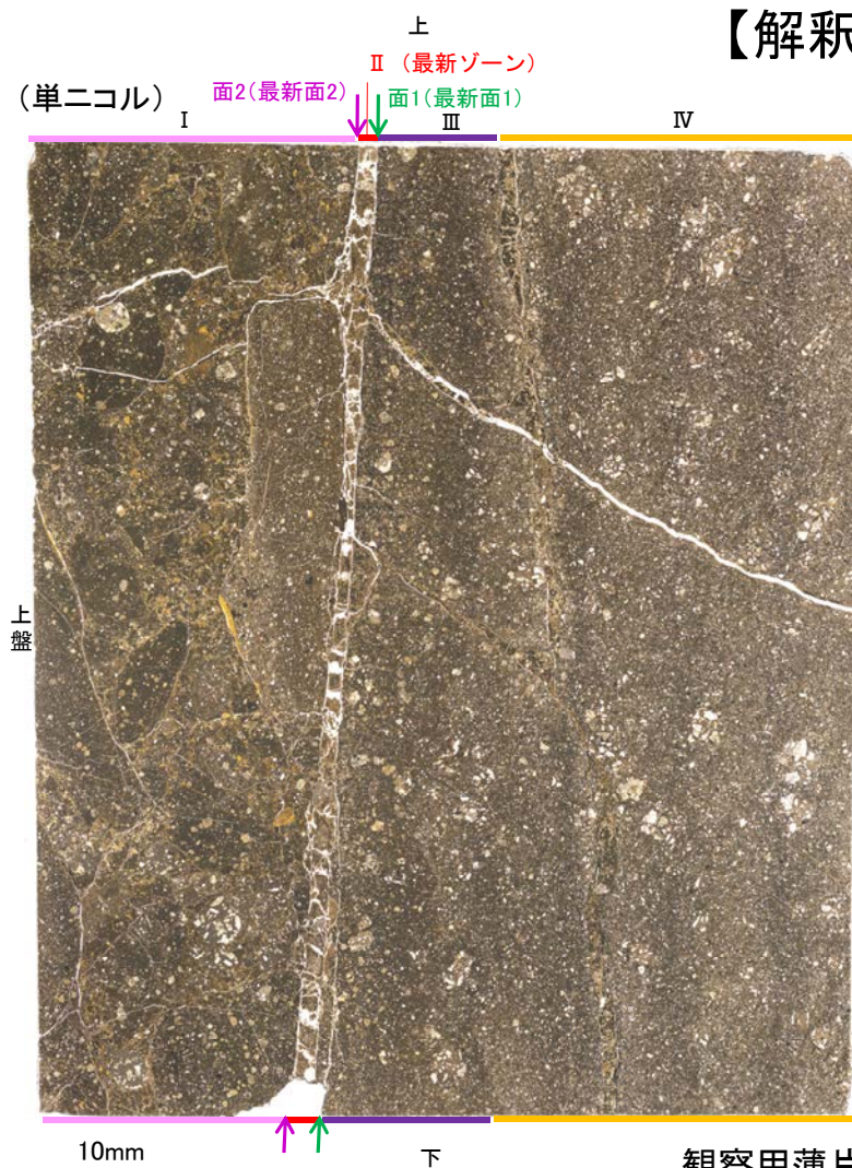
観察用薄片写真(K-6.2-2_100R)
