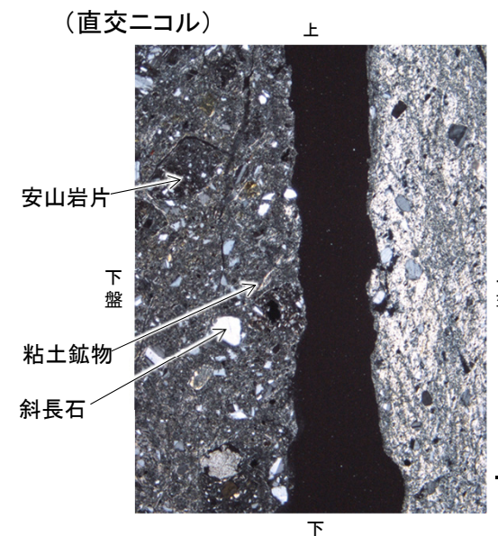
固結した角礫状破碎部の構成物
