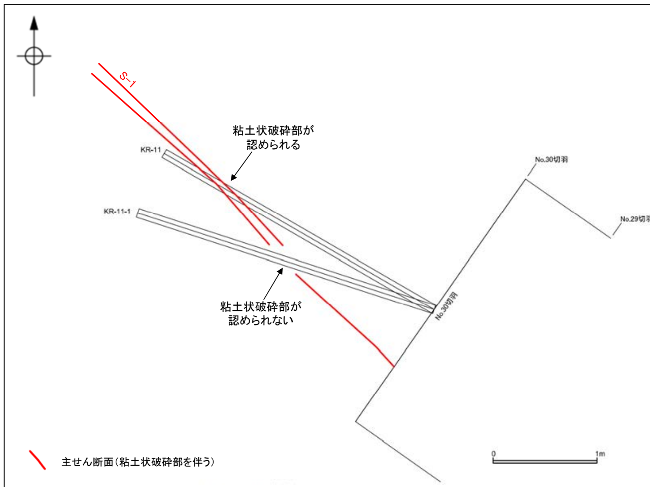
水平断面図 (EL-16.25m)
