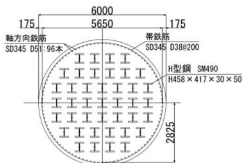
構造 I
