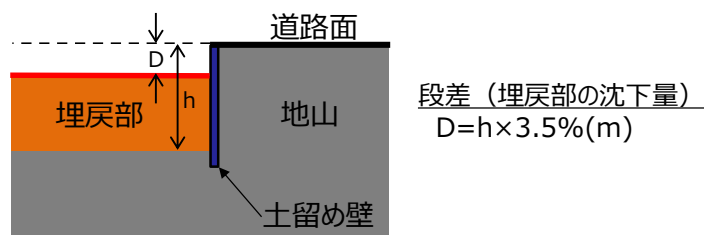
第4-16図 地山を垂直に掘削した箇所における段差発生状況
