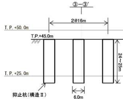
④-④' 断面図
