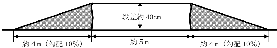
第5図 段差解消断面図（概要）
