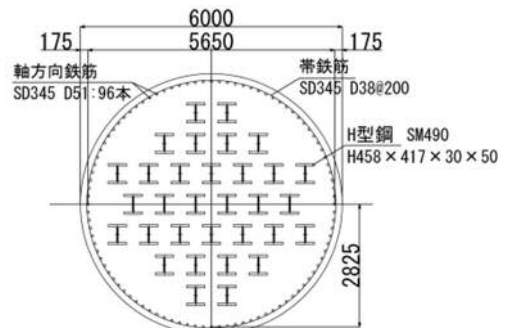
構造 II
