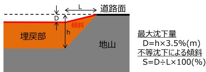
第4-17図 地山に勾配を設けて掘削した箇所の傾斜発生状況
