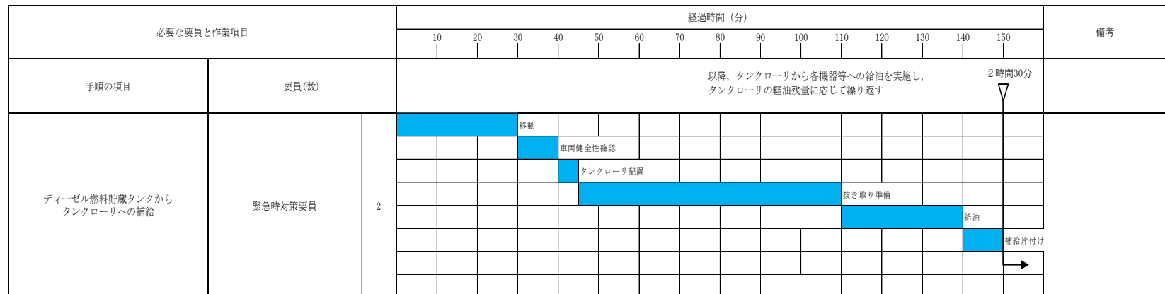
図7 ディーゼル燃料貯蔵タンクを使用した燃料抜き取り手順 タイムチャート
