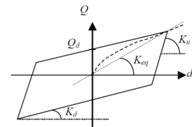
免震装置の特性を表す水平ばね (例：鉛プラグ入り積層ゴム)
