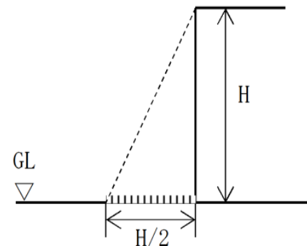
図1 外装材の落下による影響評価
