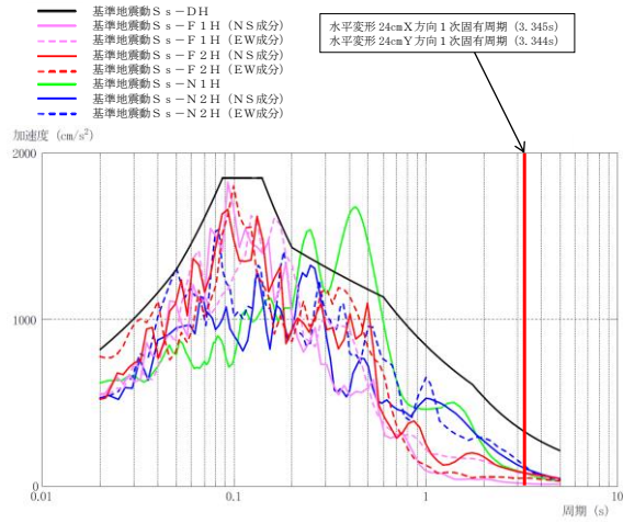
基準地震動 S s の加速度応答スペクトル (水平方向, h = 0.05)
