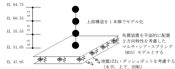
解析モデル
