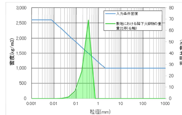
美浜発電所
