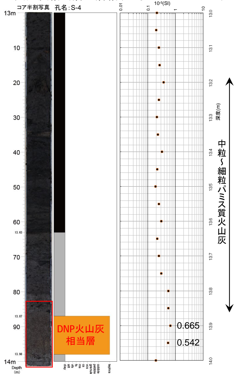
DNP火山灰相当層の層相(S4孔13.87-13.98m)
