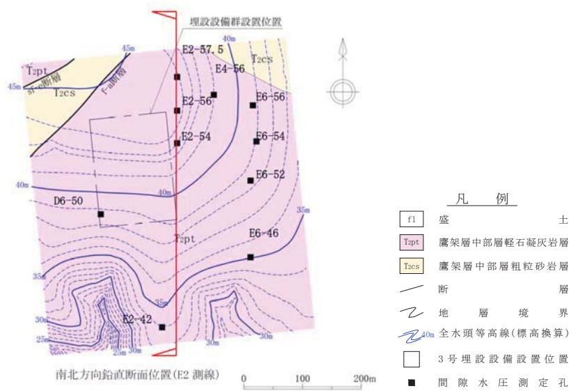
標高+22m 水平断面
