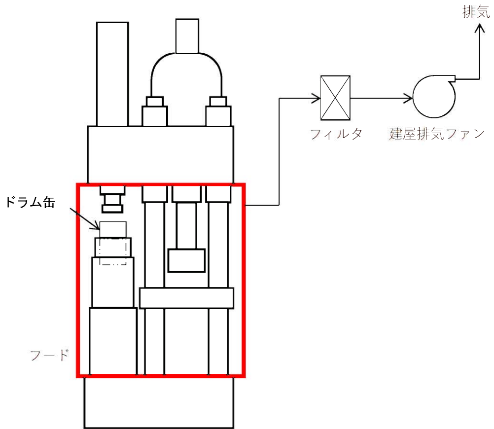
第 27-7 図 ベイラの散逸防止対策図
