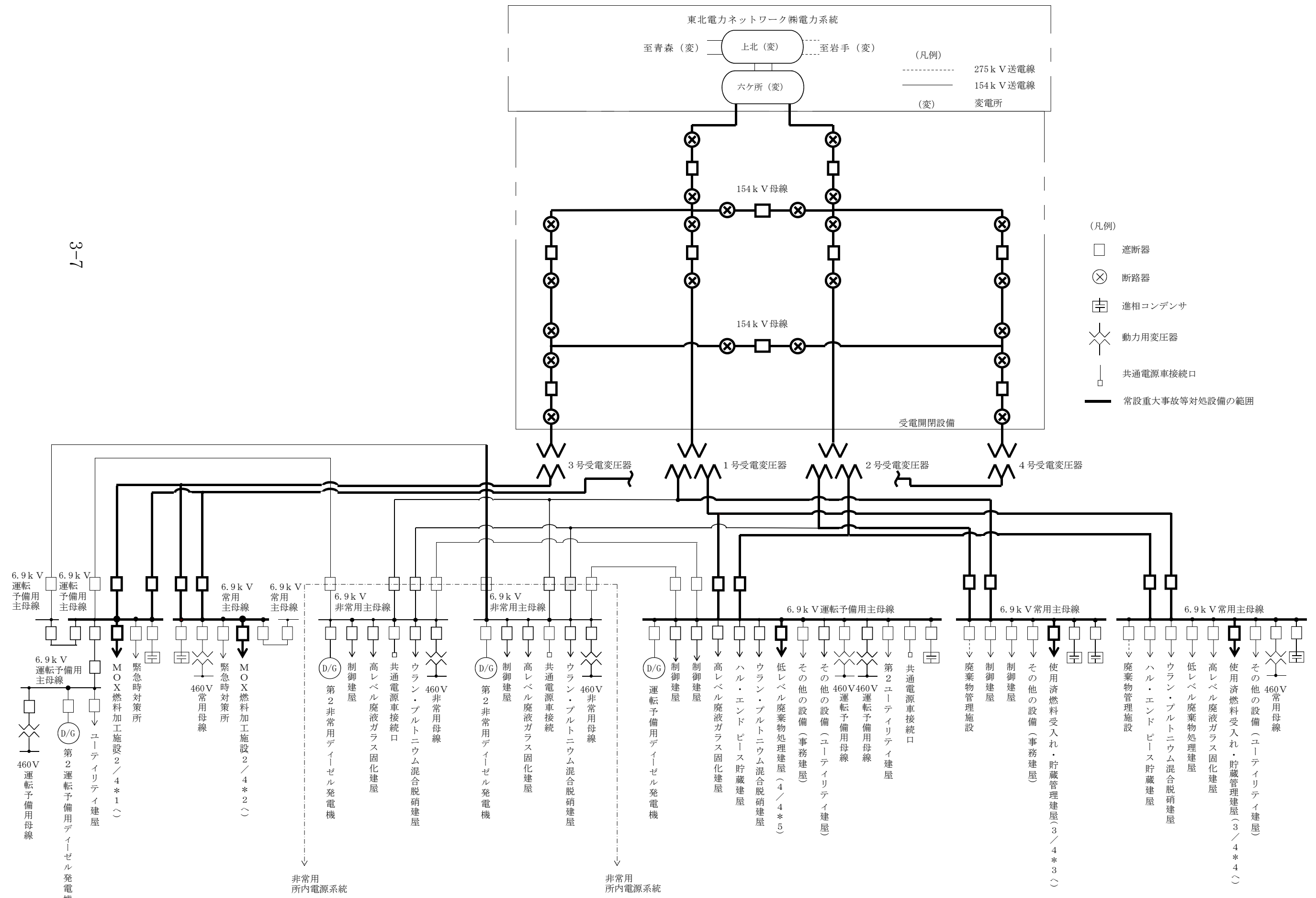
第32. 3図 燃料加工建屋の電源遮断時における重大事故等に対処するための設備の系統図 (1 / 4)
