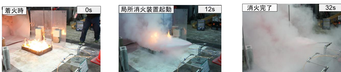
図 9. 火災源を ABC 粉末で覆えた場合の試験経過
