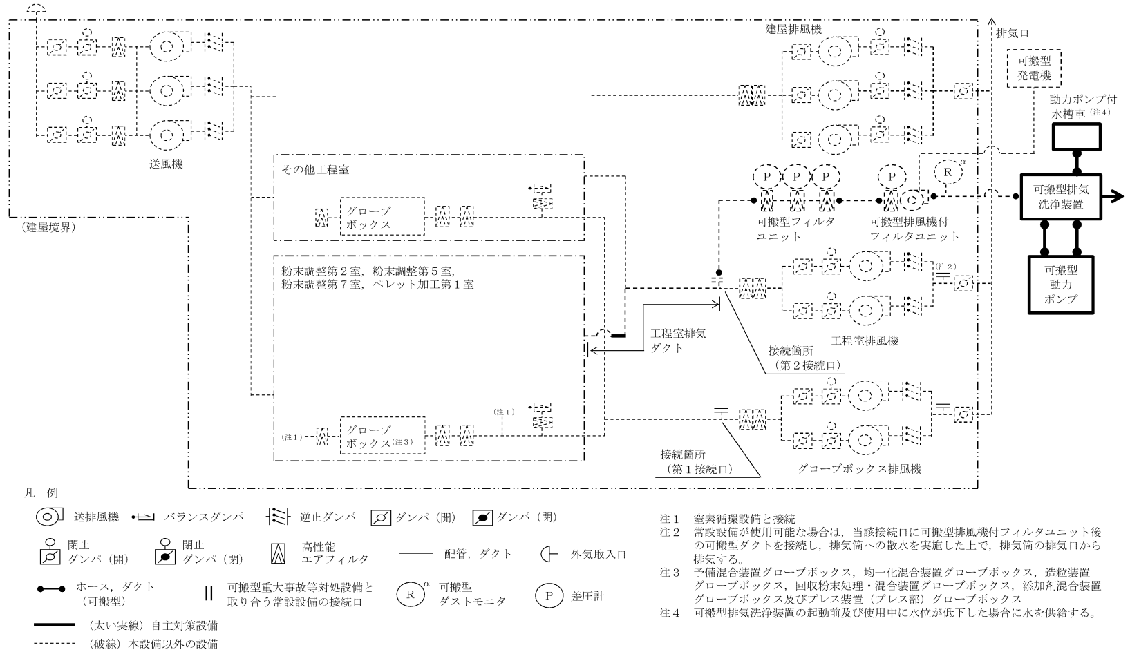
第29-5-4 図 閉じ込める機能の回復時における排気への散水の概略 (第2 接続口)
