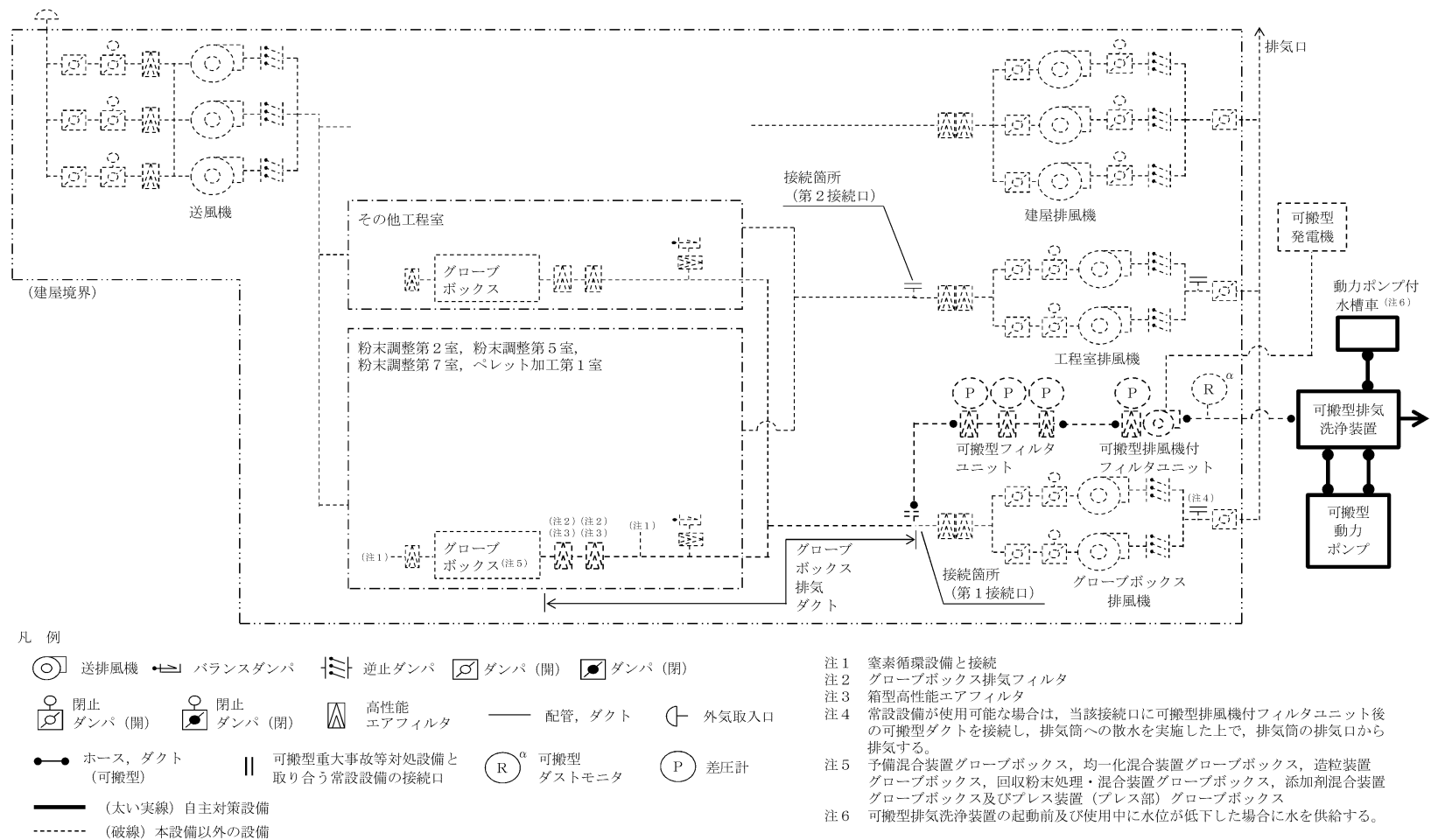
第29-5-3図 閉じ込める機能の回復時における排気への散水の概略（第1接続口）
