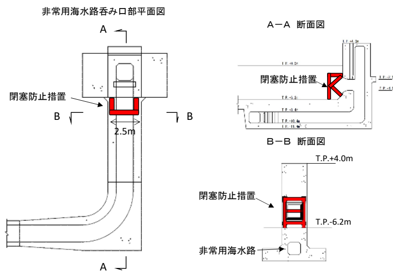
図-2-5-41 漂流物による閉塞防止措置
