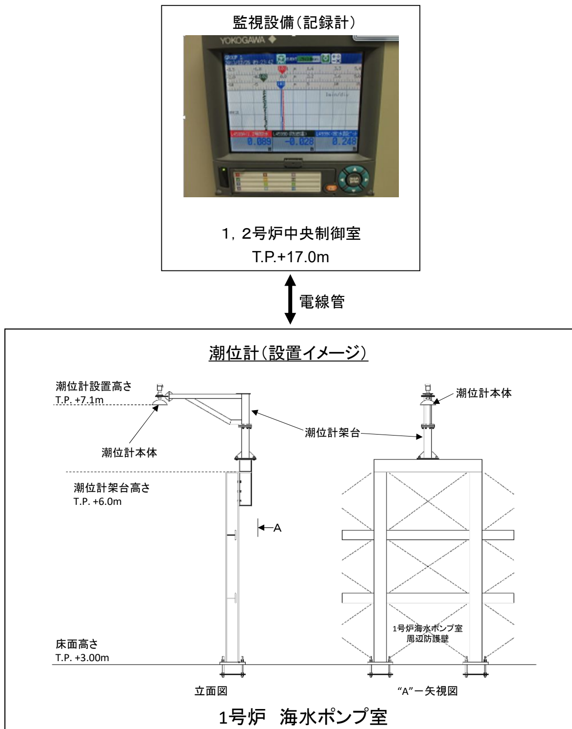
図 3-3-5 潮位計設備構成イメージ
