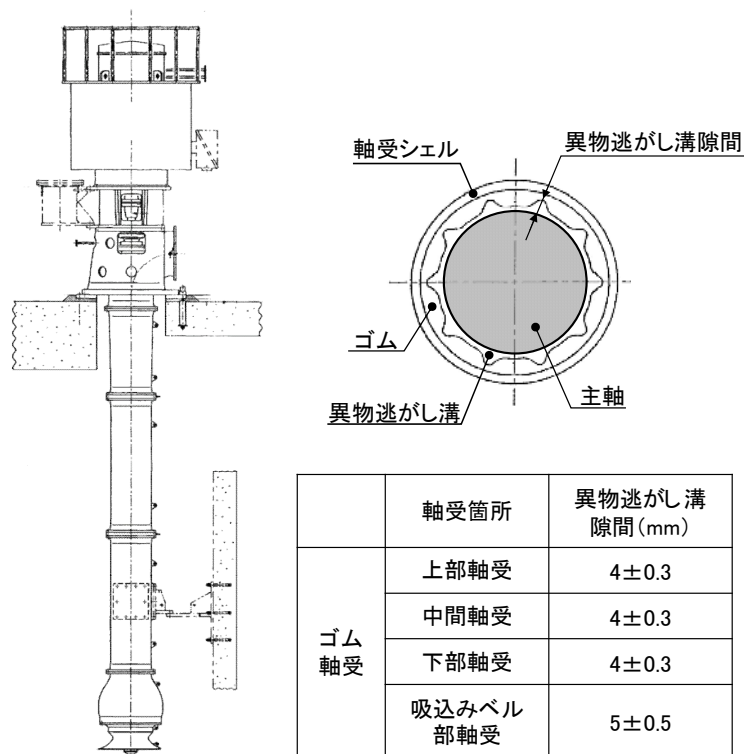
図-2-5-3 海水ポンプ軸受構造図
