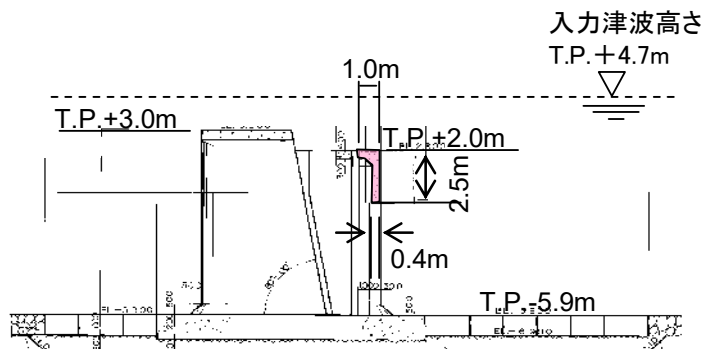
図-3-4-2 取水口カーテンウォール正面図
