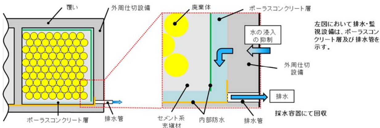
第1図 漏出防止機能のイメージ図
