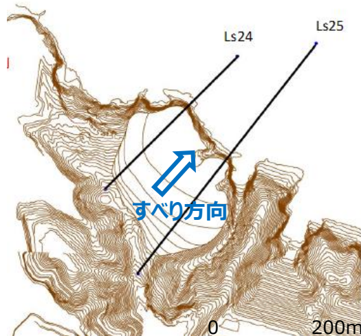
地すべり断面位置図
