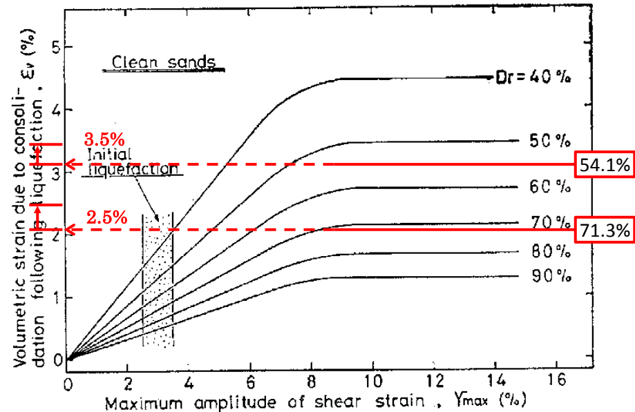
Ishihara et al. (1992) の地盤の最大せん断ひずみと体積ひずみの関係から設定した沈下率
