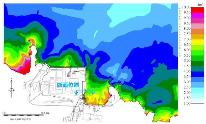
基準津波 1（防波堤無し）の最大水位上昇量分布
