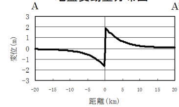
地盤変動量断面図
