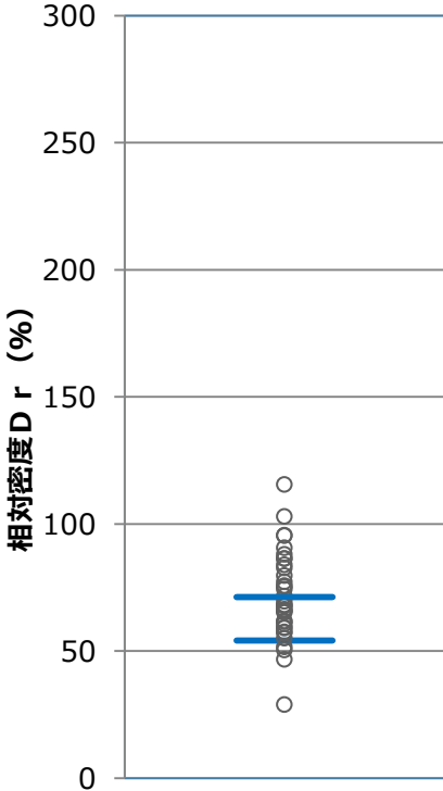
埋戻土（掘削ズリ）の相対密度
