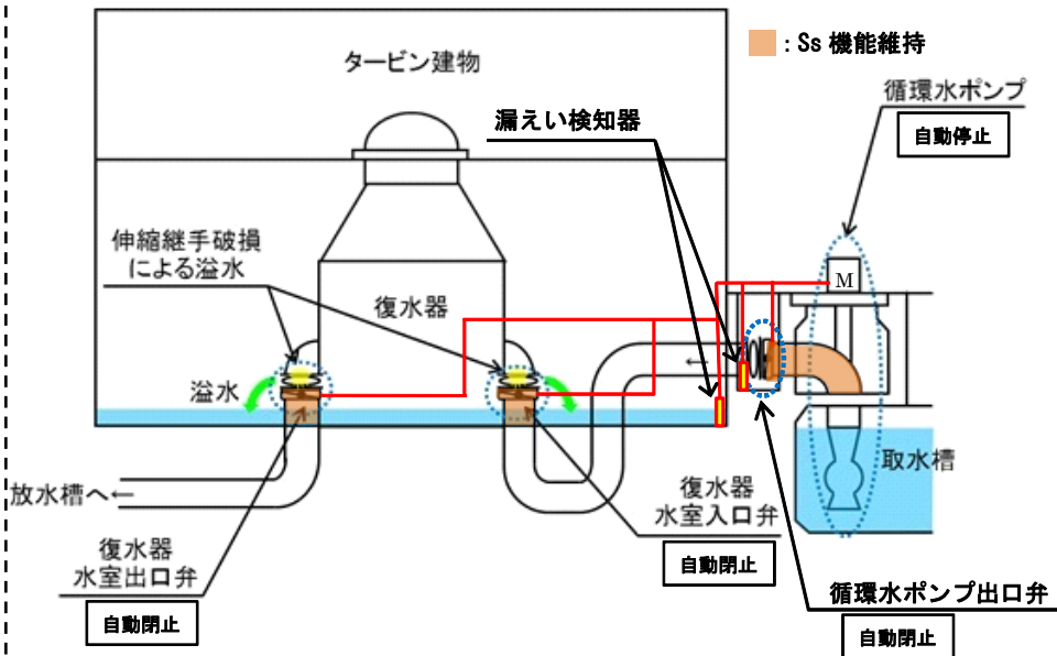
図 循環水ポンプ停止及び循環水系弁閉止インターロック設置概要図
