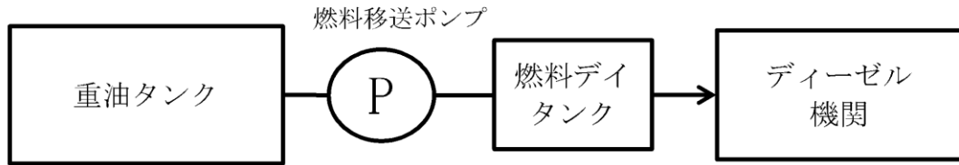
燃料油供給系統A
