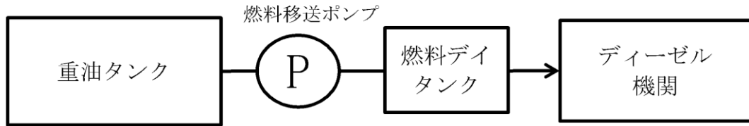
燃料油供給系統B
