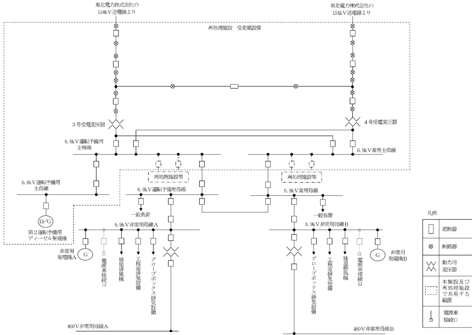
第3-4図 電力供給単線結線図
