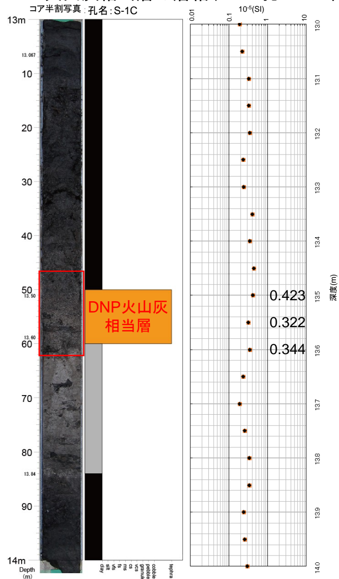
DNP火山灰相当層の層相(S-1C孔13.5m付近)
