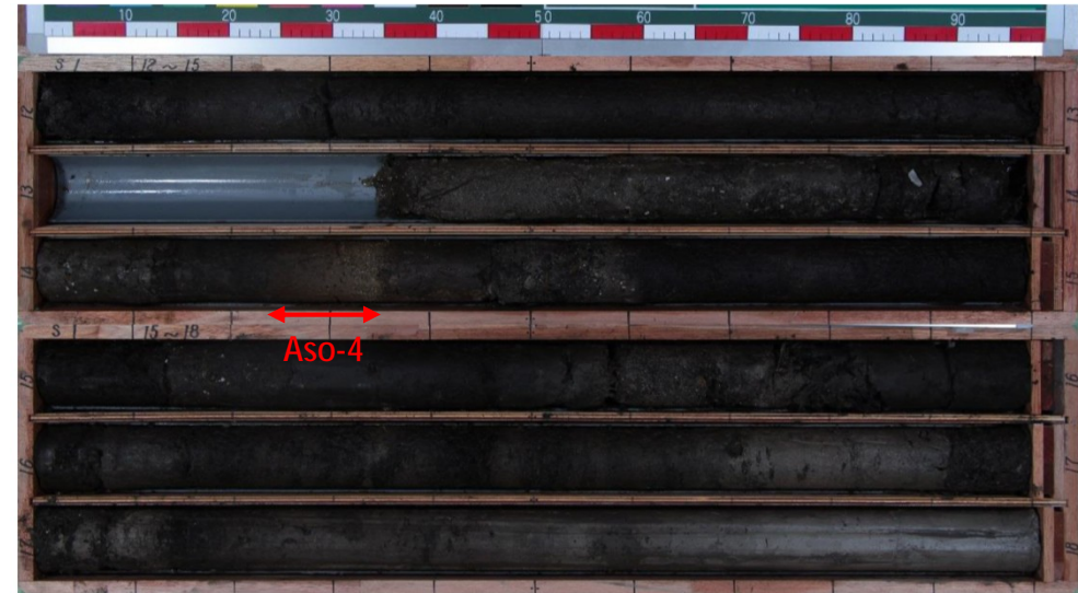
S1B地点の柱状図とコア写真
