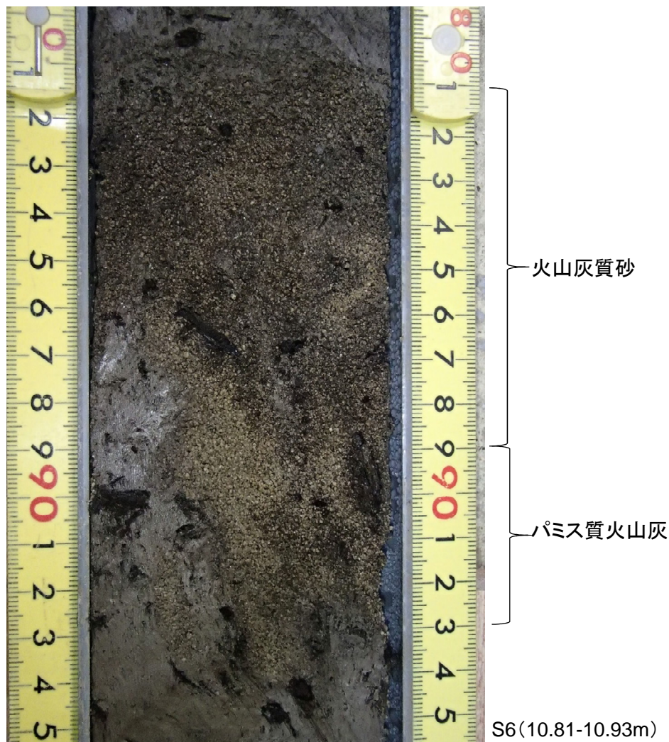
コア半割拡大写真(10.8m付近)
