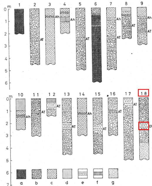
第5図 柱状図
