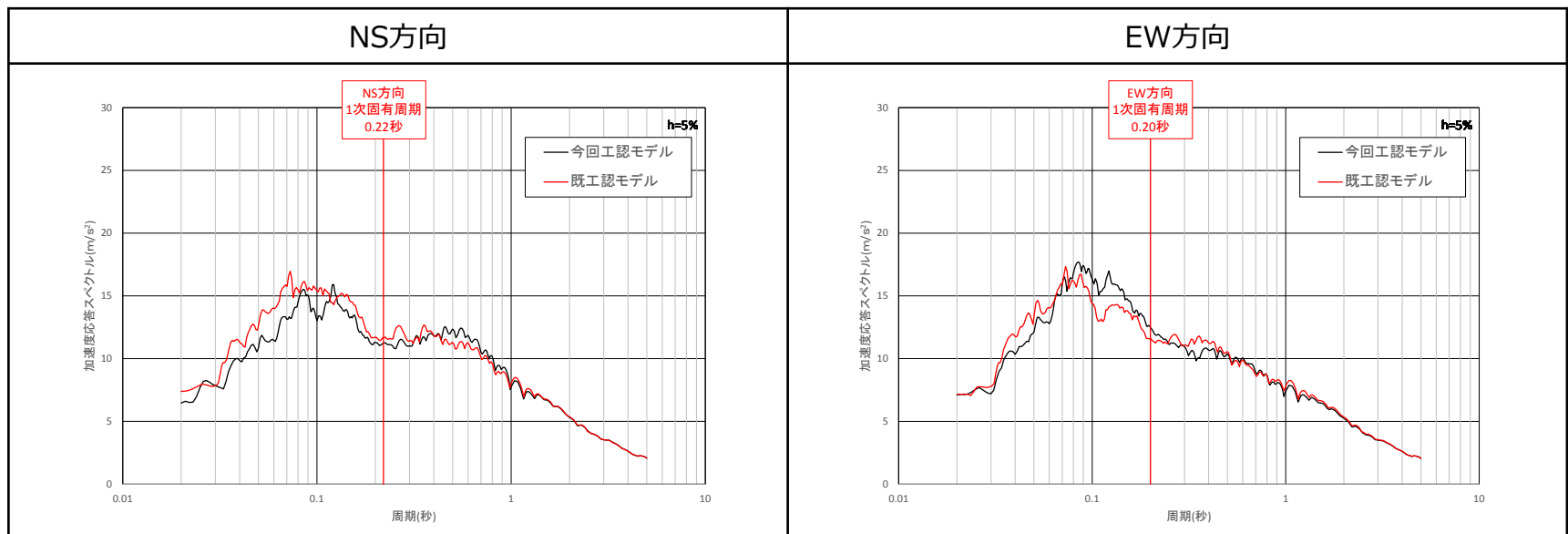
既工認モデルと今回工認モデルによる入力地震動の加速度応答スペクトルの比較
