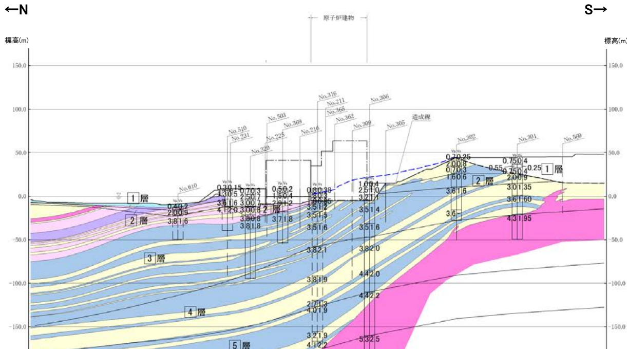
【参考2】2号地盤の岩相区分との比較(南北断面)
