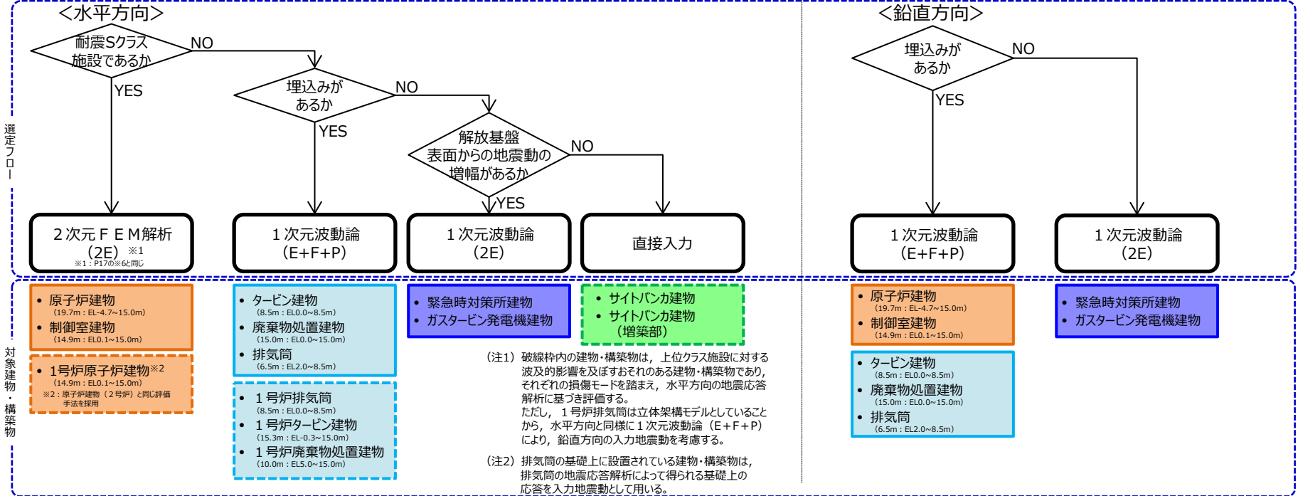
入力地震動の評価手法の選定フロー
