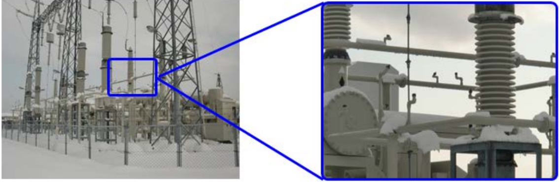
第 4-4-3 図 受電開閉設備全景
