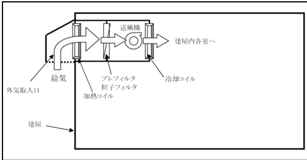
第 4-4-1 図 建屋給気ユニットにおける防食対策概要図 (フィルタによる塩分除去)
