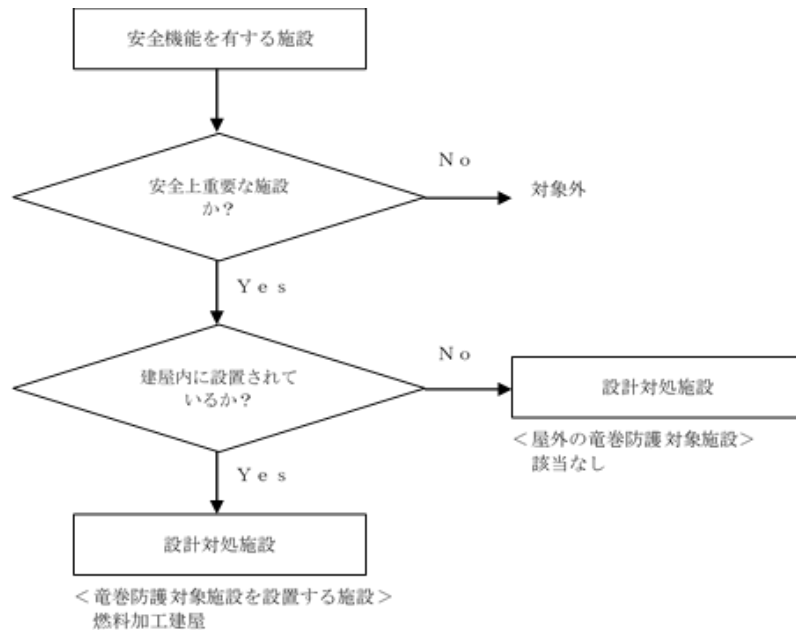
図3 飛来物に対する設計対処施設の選定フロー
