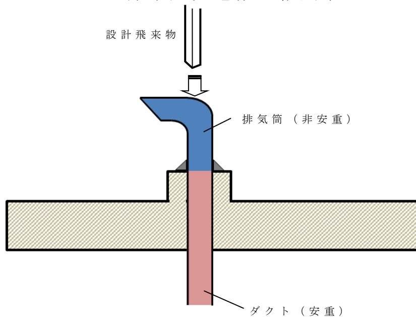
b . 非常用発電機の排気系
