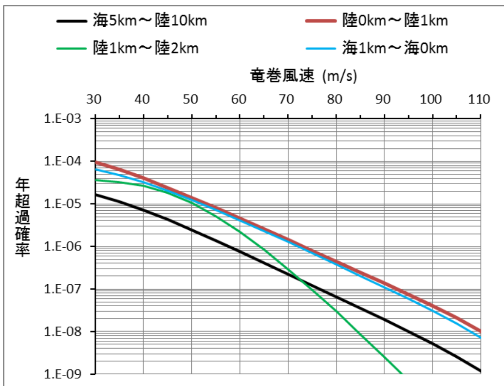
添3-16 図 竜巻最大風速のハザード曲線 (1 km 範囲) (参考)
