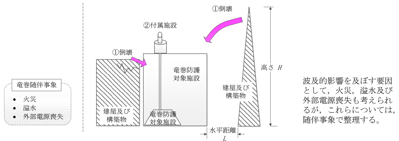
図7 竜巻防護対象施設に波及的影響を及ぼし得る施設のイメージ
