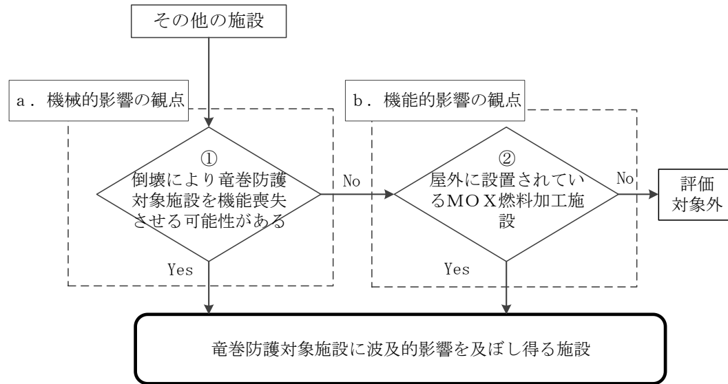
図6 評価対象抽出フロー
