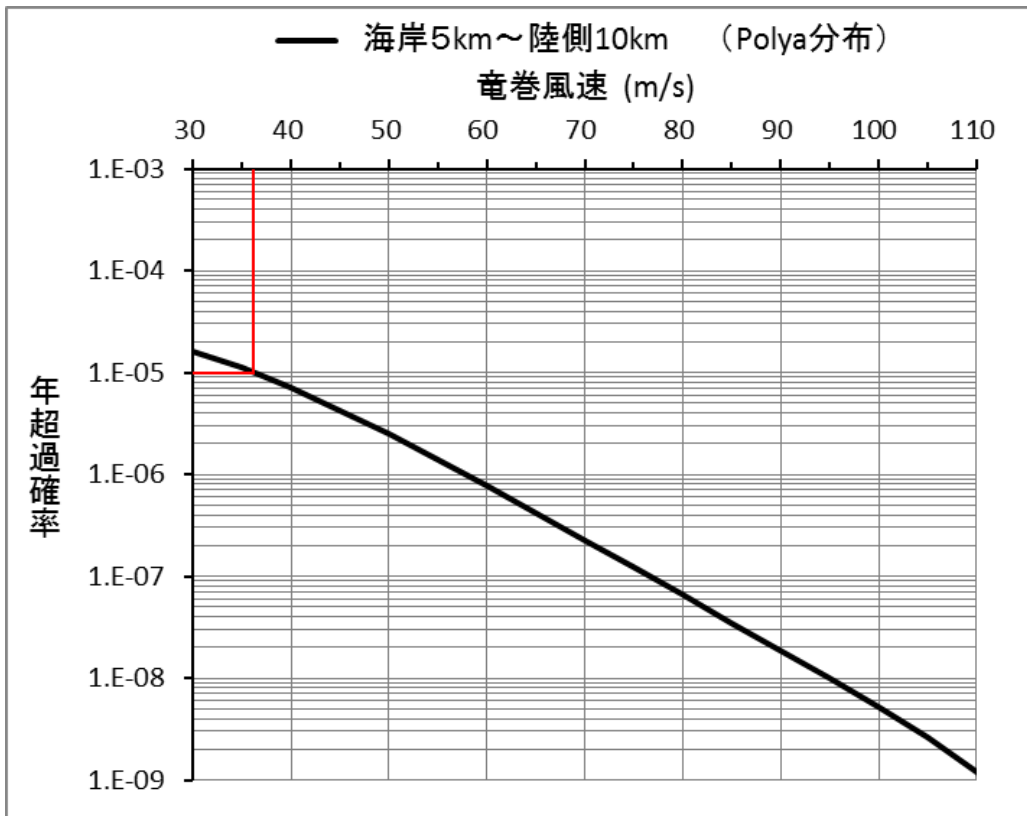
添3-15 図 竜巻最大風速のハザード曲線 (竜巻地域検討)
