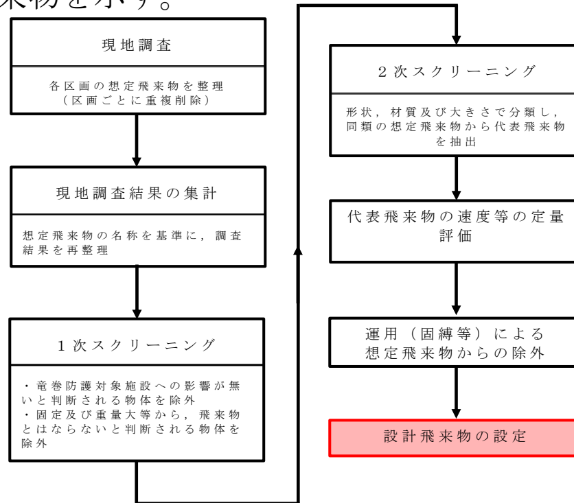
図11 設計飛来物の設定フロー
