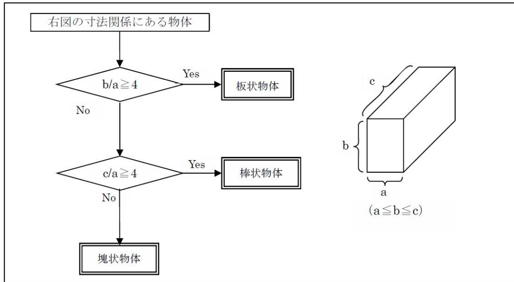
第 5 - 6 - 1 図 塊状，板状，棒状の判定フロー
