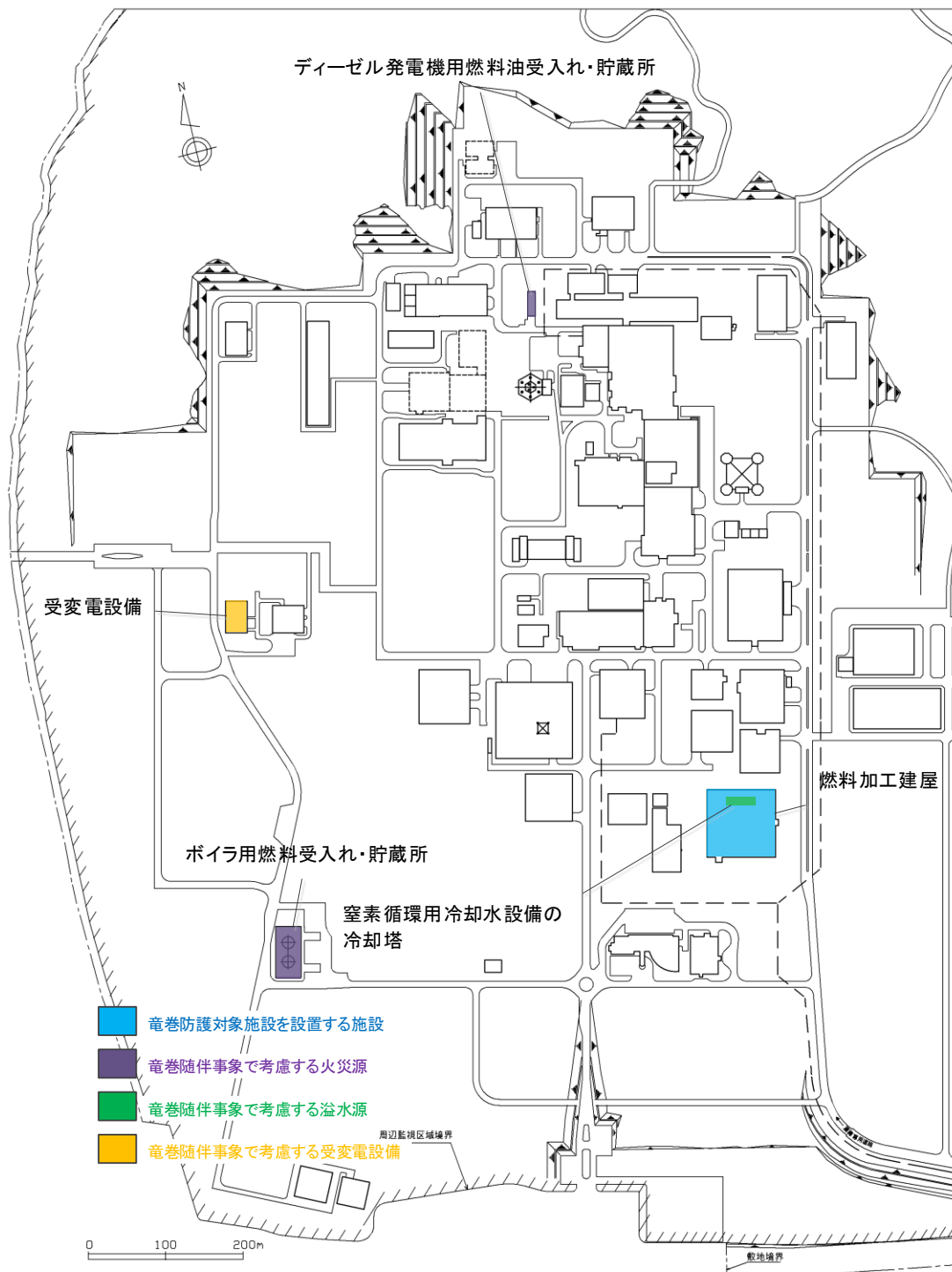
第 7 - 1 - 4 図 MOX 燃料加工施設の設計対処施設のうち 竜巻防護対象施設を設置する施設及び竜巻随 伴事象の検討対象施設の配置図
