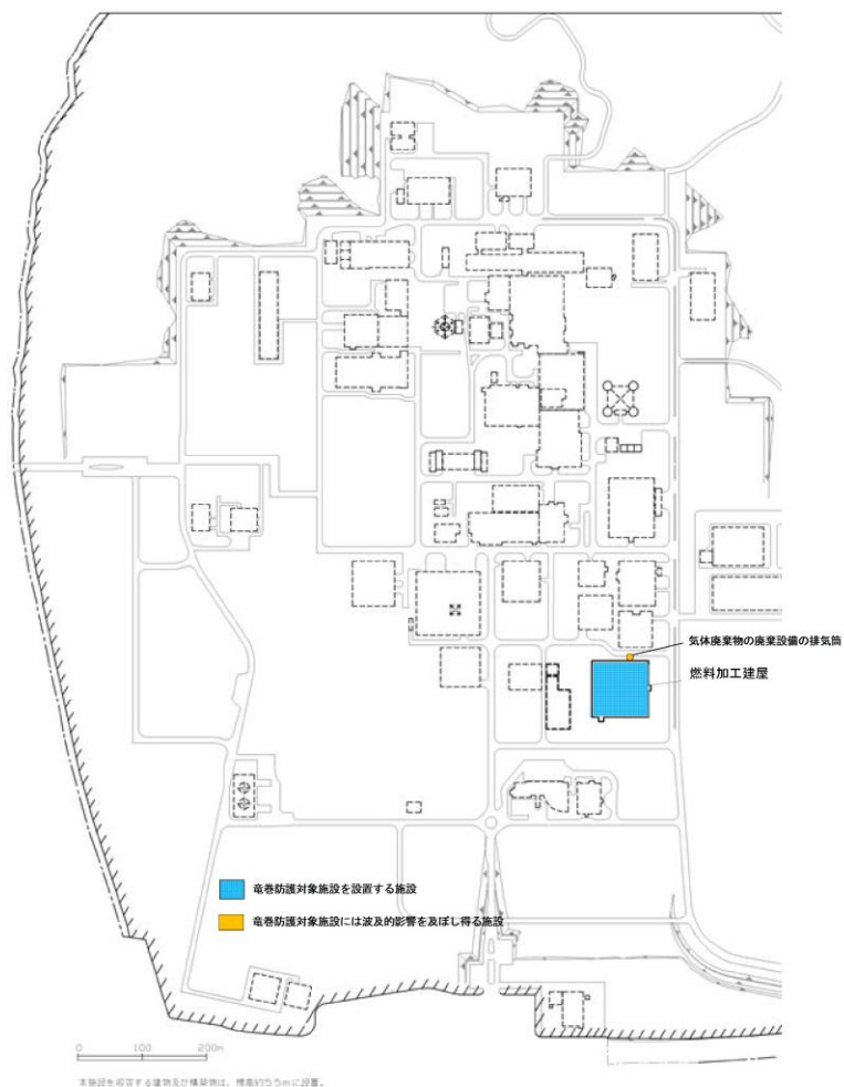
図8 設計対処施設の配置
