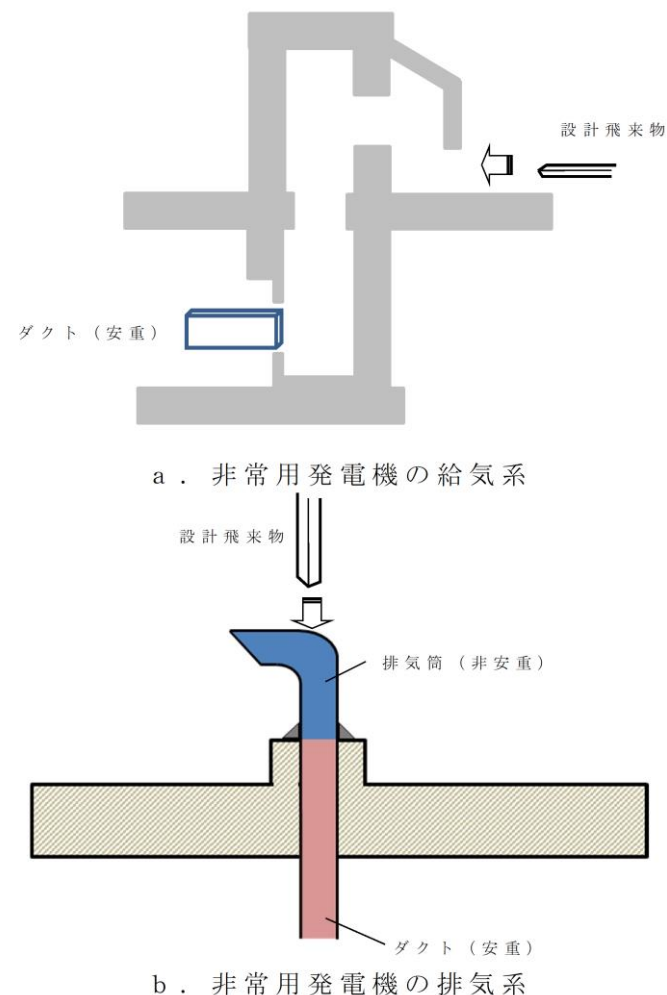
図12 非常用発電機の給気系及び排気系に対する竜巻防護設計のイメージ
