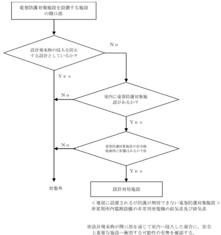
図5 開口部に対する設計対処施設の選定フロー
