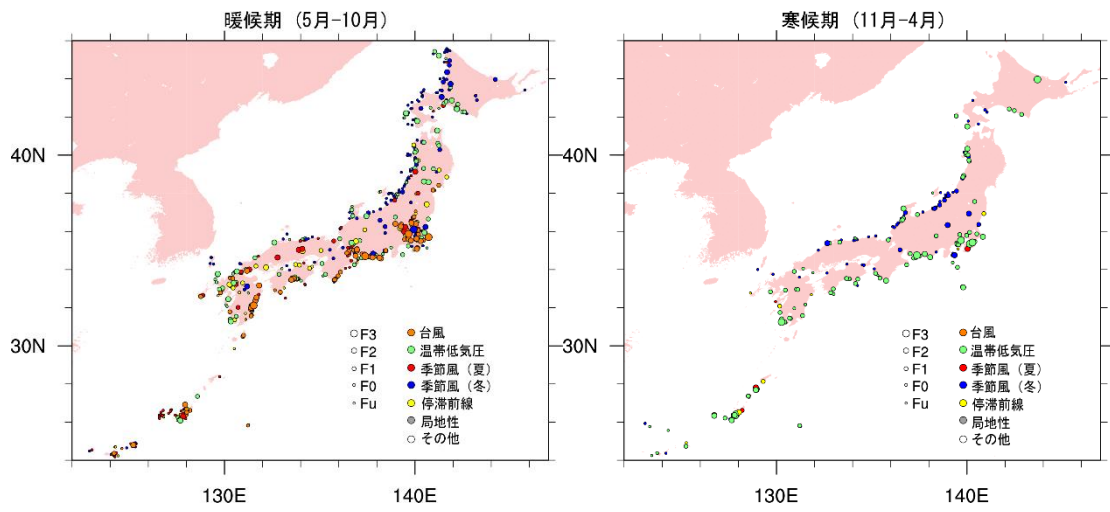
第 4 - 1 - 1 図 季節別の竜巻発生位置 (左：暖候期，右：寒候期)
