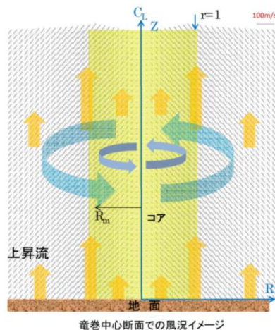
第 8 - 1 - 3 図 ランキン渦モデル (2)
