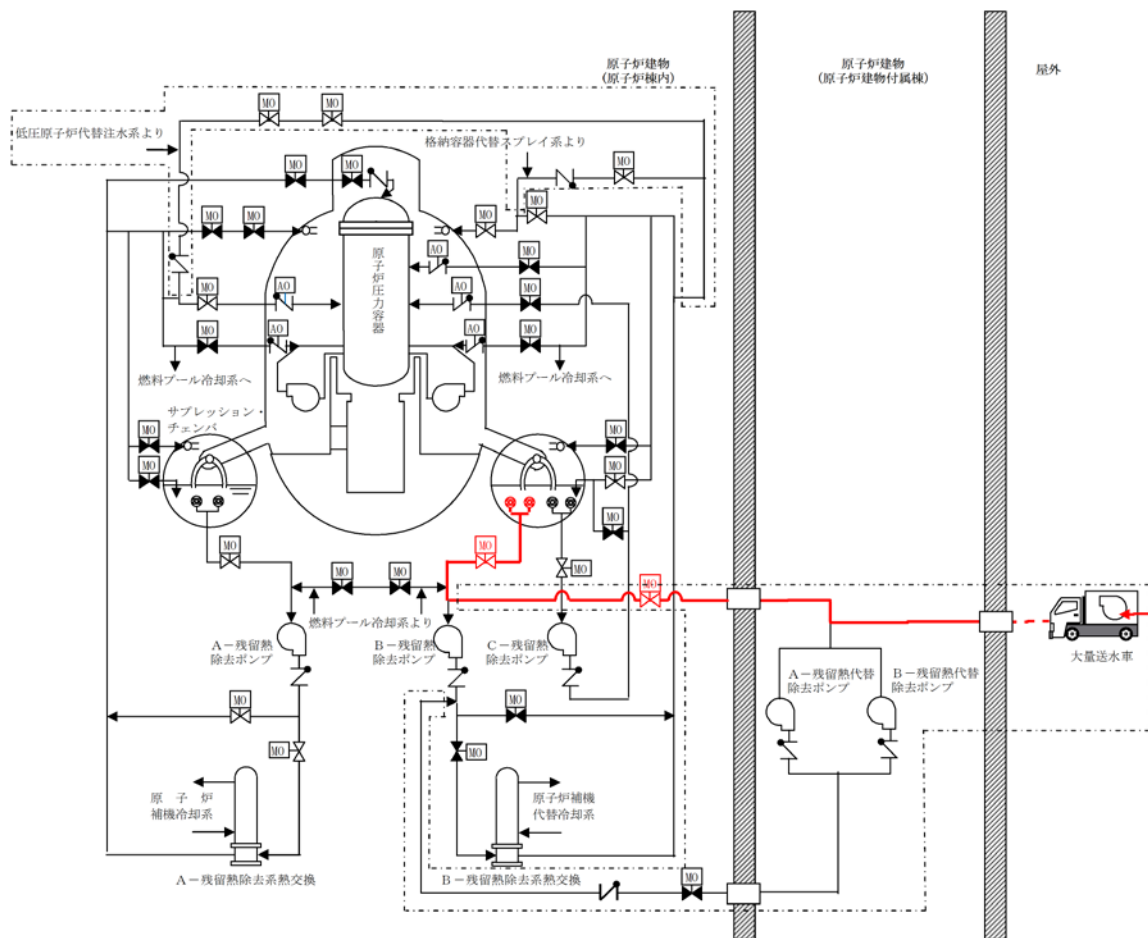
第5図 残留熱除去系ストレナー逆洗操作時の系統構成
