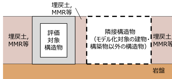
評価対象構造物の周辺にモデル化対象の建物・構築物以外の構造物が隣接する場合
