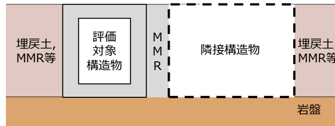
評価対象構造物と隣接構造物との間がMMRの場合
