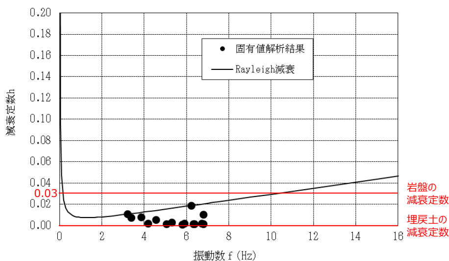
設定したRayleigh減衰（取水槽の例）
