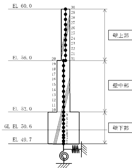
免震重要棟遮蔽壁の解析モデル図
