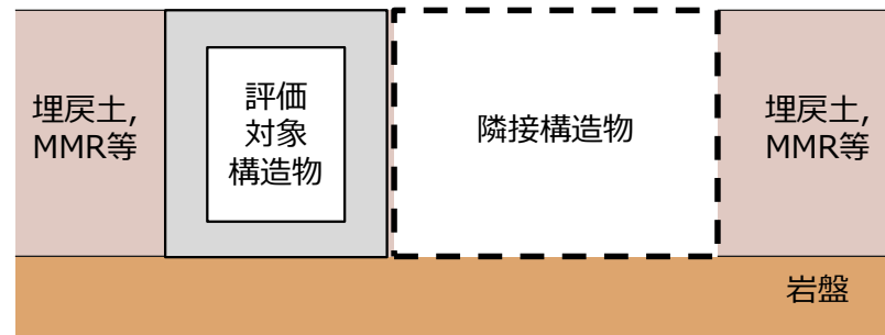
評価対象構造物と隣接構造物が接している場合
