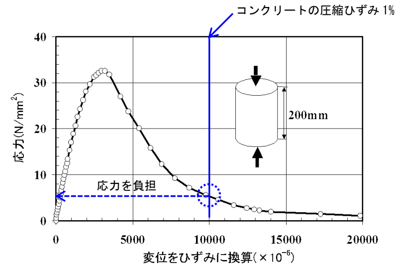
コンクリートの圧縮試験例
