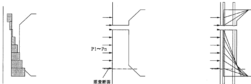
(a) 応答せん断力分布
