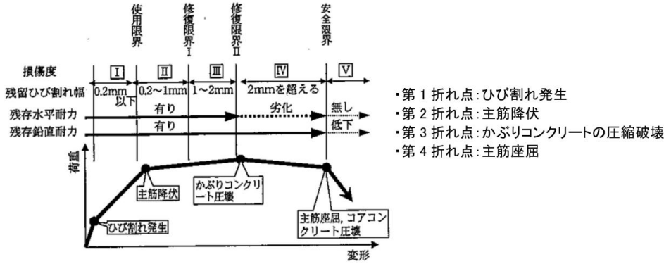
曲げ降伏先行型の部材の復元力特性と限界状態（損傷度）の関係の概念図（日本建築学会）
