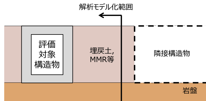
評価対象構造物の周辺に隣接構造物が存在しない場合又は十分な離隔を有する場合
