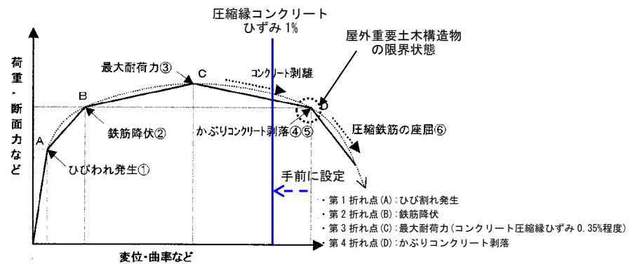
鉄筋コンクリートはり部材の荷重－変位関係と損傷状態に対する概念図（土木学会マニュアル）
