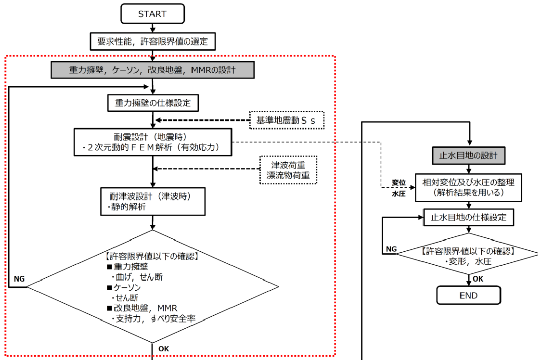
第 1-93 図 防波壁（波返重力擁壁）の設計フロー
