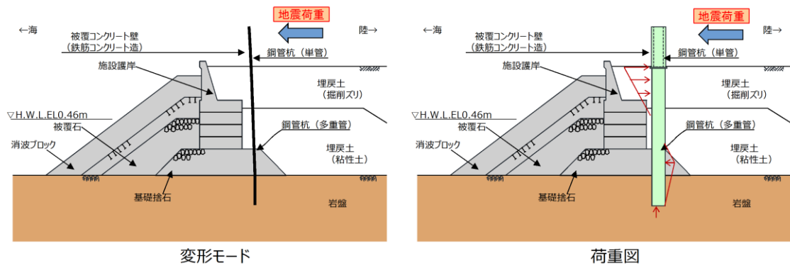
第 1-71 図 防波壁（多重鋼管杭式擁壁）の変形モード及び荷重図（地震時）
