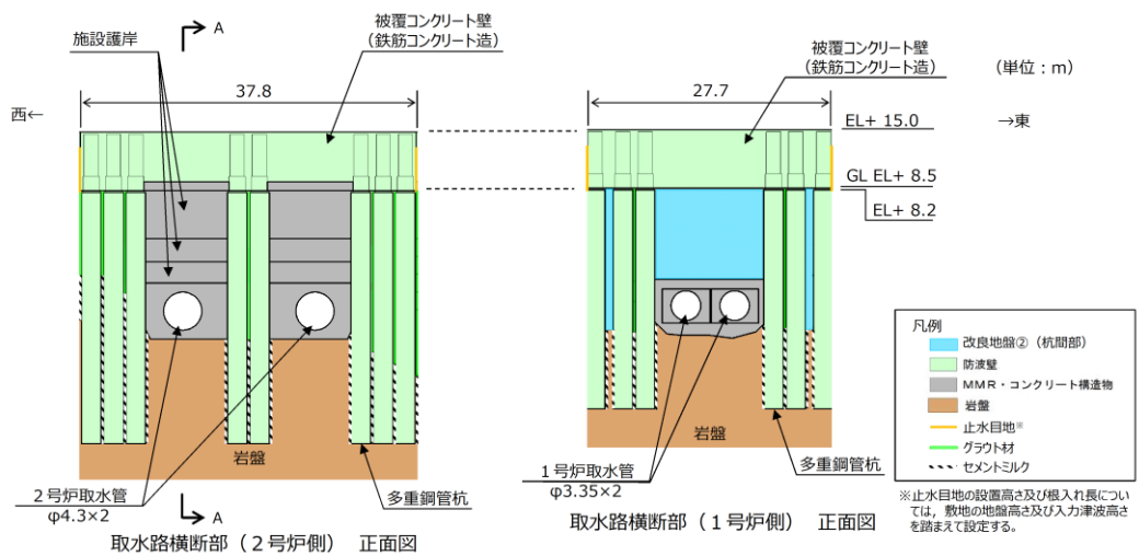
第 1-79 図 防波壁（多重鋼管杭式擁壁）取水路横断部正面図
