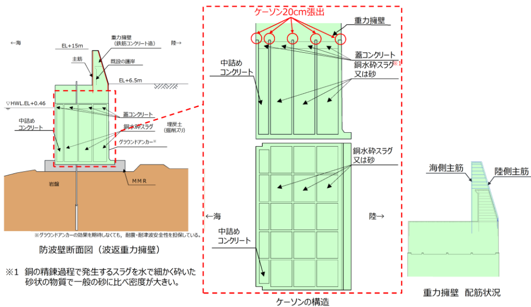
第2図 防波壁 (波返重力擁壁) ケーソンの構造
