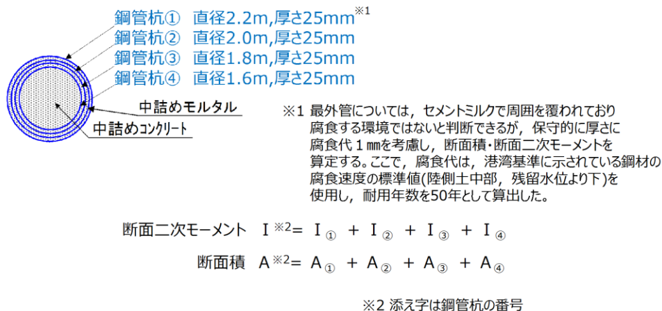
第1図 多重鋼管杭の概要
