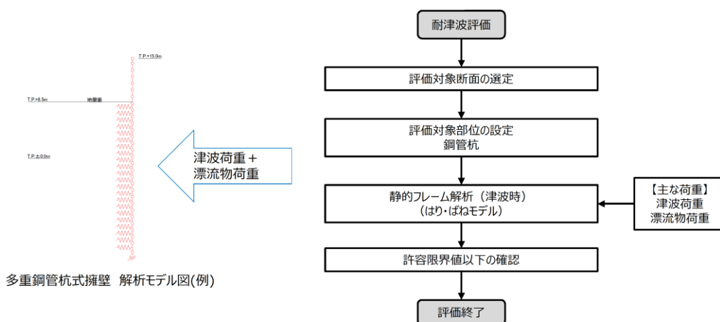
第 1-99 図 設計フロー
