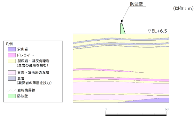
第 1-70 図 防波壁（波返重力擁壁）の地質断面図（⑥－⑥）
