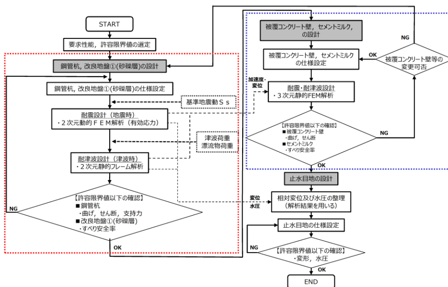
第 1-85 図 防波壁（多重鋼管杭式擁壁）の設計フロー
