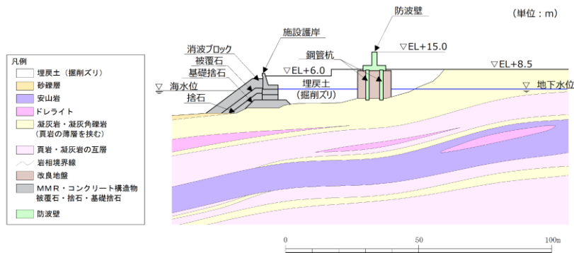
第 1-62 図 防波壁（鋼管杭式逆 T 擁壁）の地質断面図（①－①）
