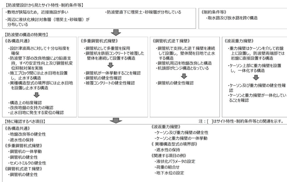
第1-77図 防波壁の各構造の特異性と特に確認すべき項目の整理
