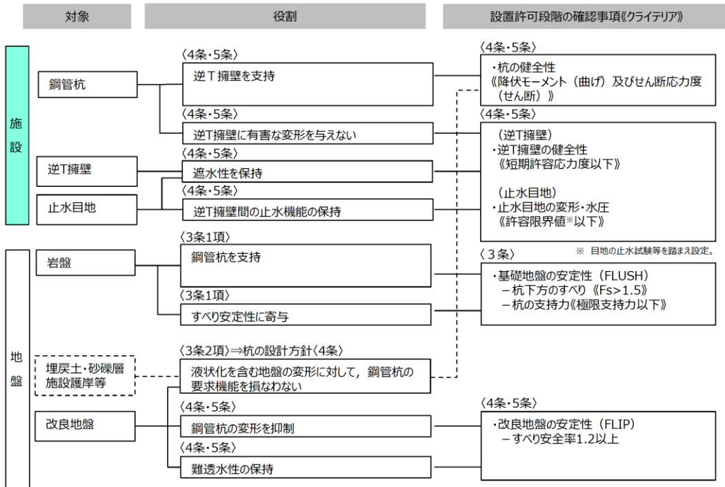
第 1-92 図 設置許可段階における確認項目 [防波壁（鋼管杭式逆T擁壁）]
