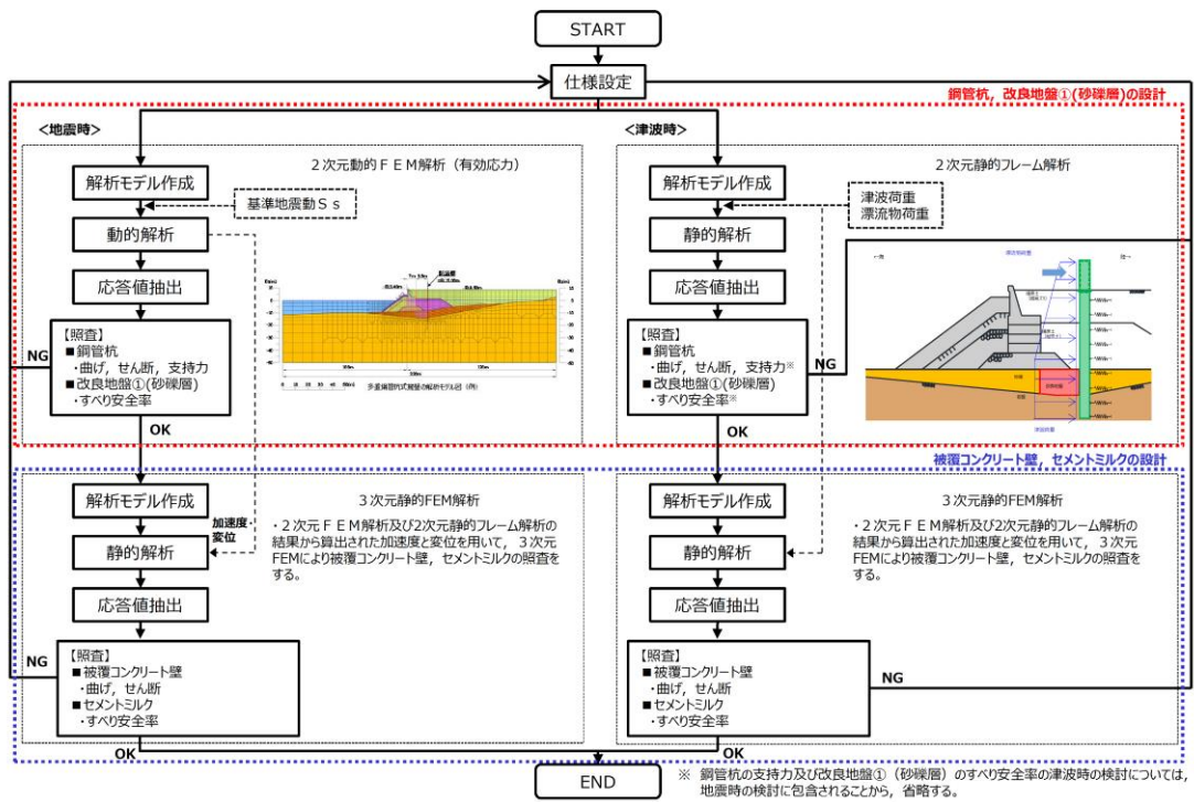
第 1-87 図 防波壁（多重鋼管杭式擁壁）の解析概要
