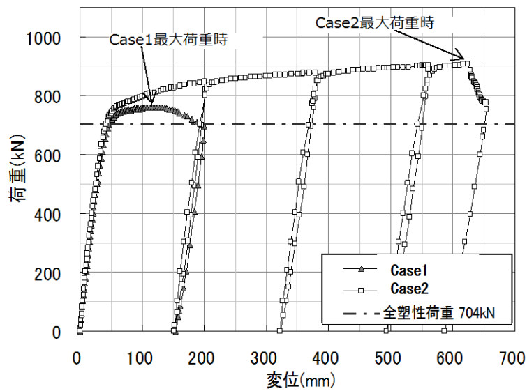
第 5 図 Case1 及び Case2 の最大荷重時の荷重変位関係
