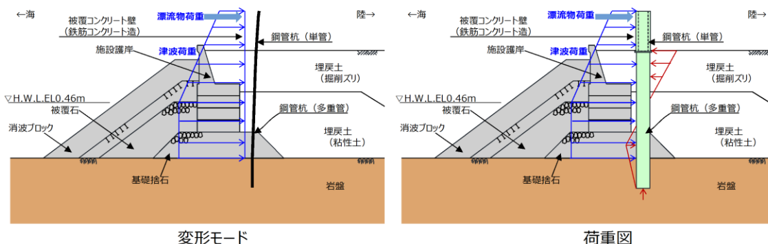
第 1-74 図 防波壁（多重鋼管杭式擁壁）の変形モード及び荷重図（津波時）
