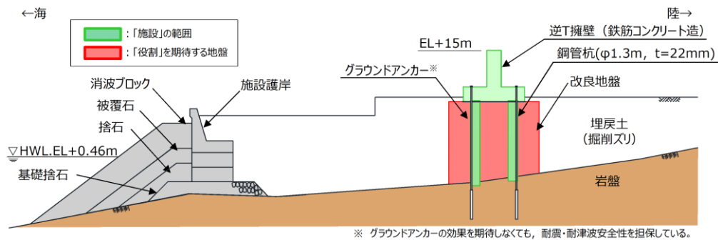
第 1-20 図 防波壁（鋼管杭式逆 T 擁壁）（一般部）における「施設」と「地盤」の区分
