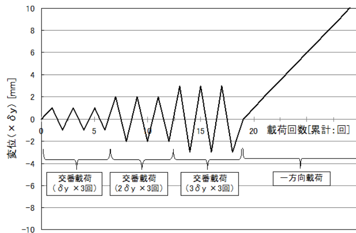
第4図 交番水平载荷変位
