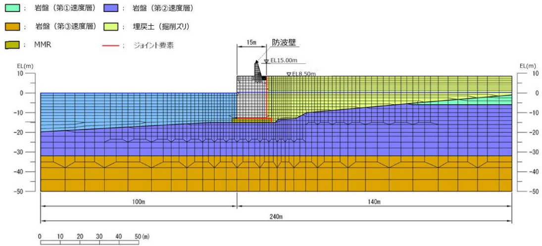
第 1-94 図 防波壁（波返重力擁壁）の解析モデル
