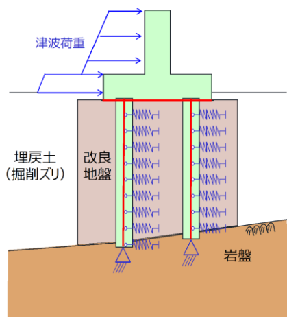
第 2-28 図 骨組計算モデル図（標準部）
