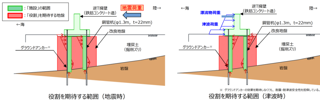
第 1-6 図 防波壁（鋼管杭式逆 T 擁壁）の役割を期待する範囲
