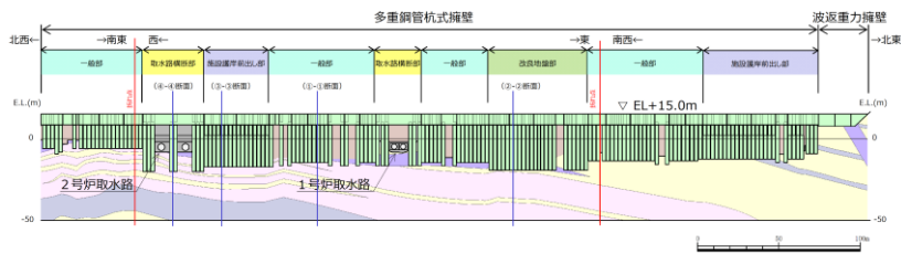
第 1-54 図 防波壁（多重鋼管杭式擁壁）の岩相縦断面図
