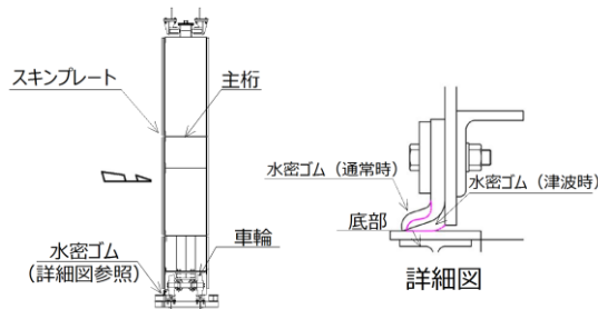
第 1-40 図 防波壁通路防波扉（1，2号炉北側）③ 断面図
