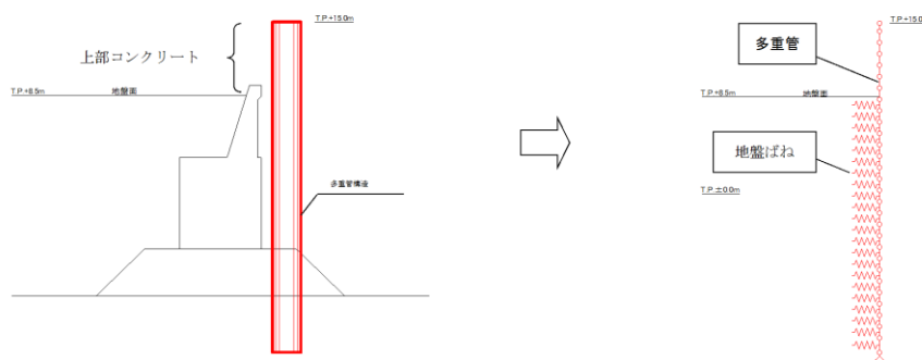
第 2-18 図 多重鋼管杭のモデル化（津波時）
