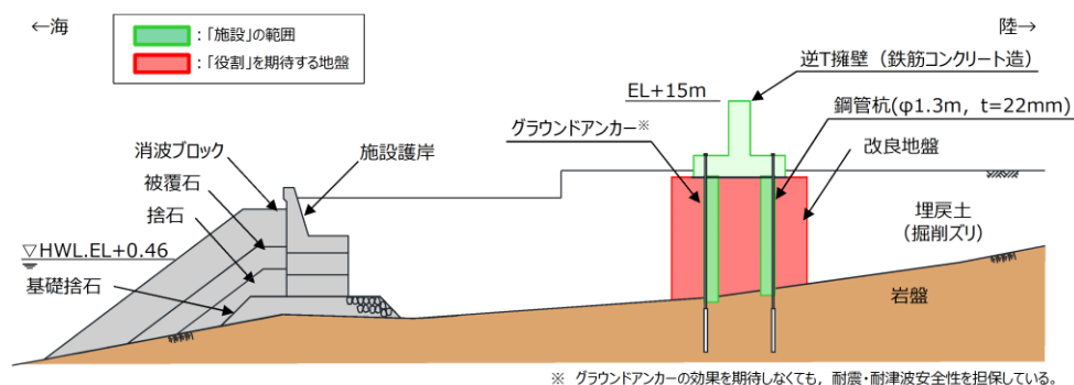
第1-5図 防波壁（鋼管杭式逆T擁壁）の「施設」の範囲
