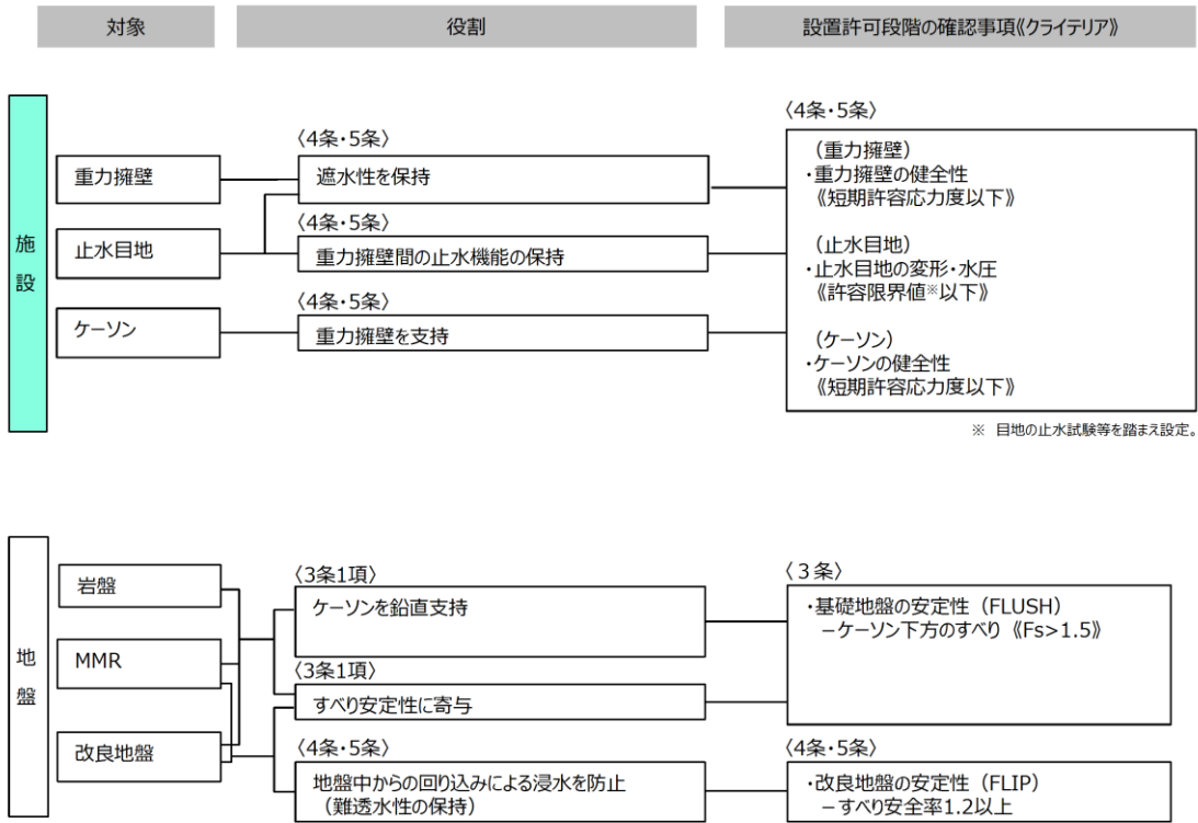
第 1-96 図 設置許可段階における確認項目 [防波壁 (波返重力擁壁)]
