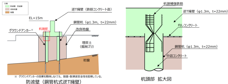
第2図 防波壁（鋼管式逆T擁壁）の杭頭部の構造概要図
