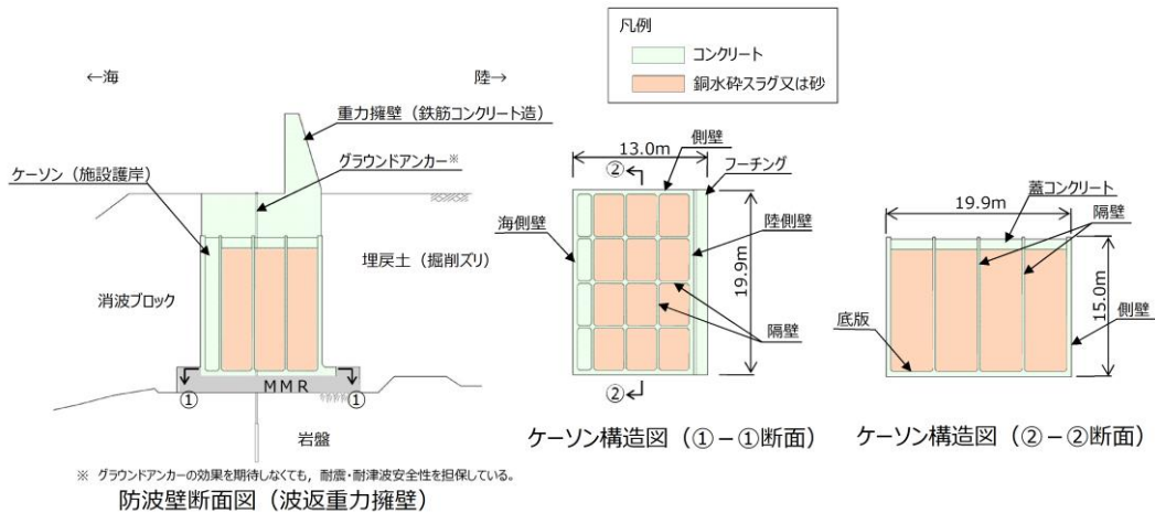
第 1-83 図 防波壁（波返重力擁壁）ケーソン構造図
