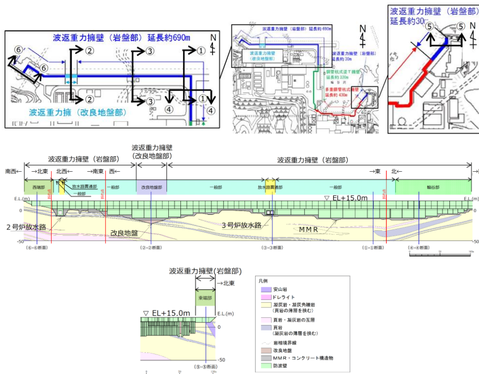
第 1-63 図 防波壁（波返重力擁壁）の岩相縦断図
