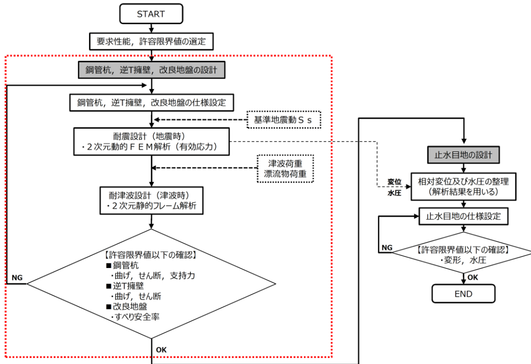
第 1-89 図 防波壁（鋼管杭式逆T擁壁）の設計フロー
