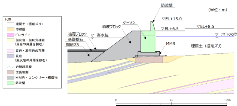
第 1-66 図 防波壁（波返重力擁壁）の地質断面図 (②-②)
