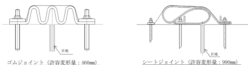
第 2-39 図 止水目地の設定例
