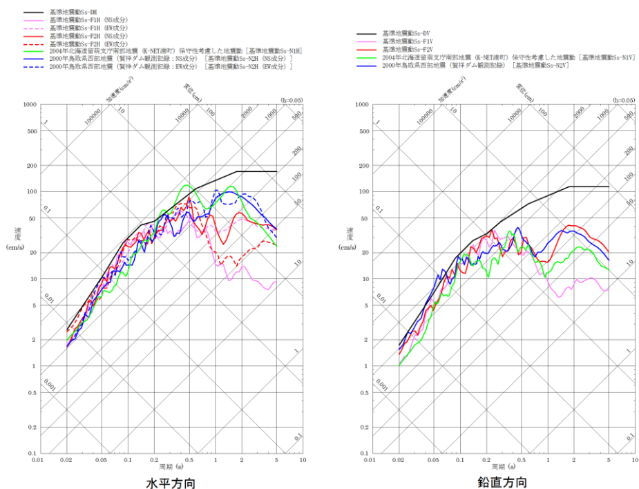
第 1-105 図 基準地震動 S s の応答スペクトル
