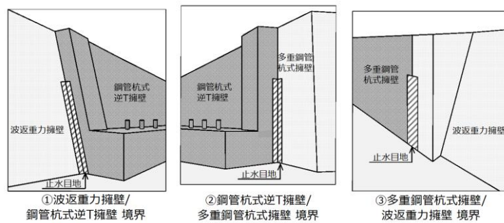
第 1-52 図 防波壁構造形式境界部の止水目地形状
