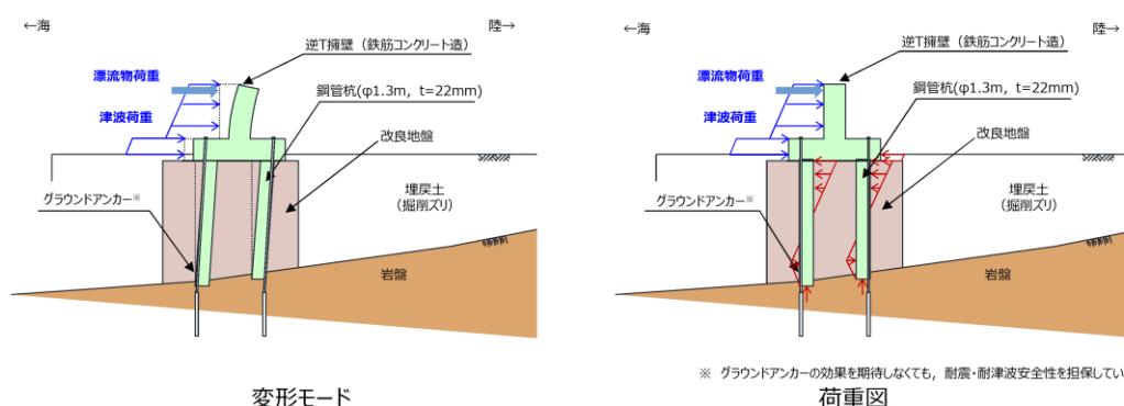
第1-75図 防波壁（鋼管杭式逆T擁壁）の変形モード及び荷重図（津波時）
