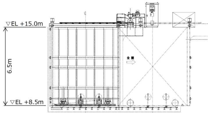
第 1-41 図 防波壁通路防波扉（1，2号炉北側）④ 正面図
