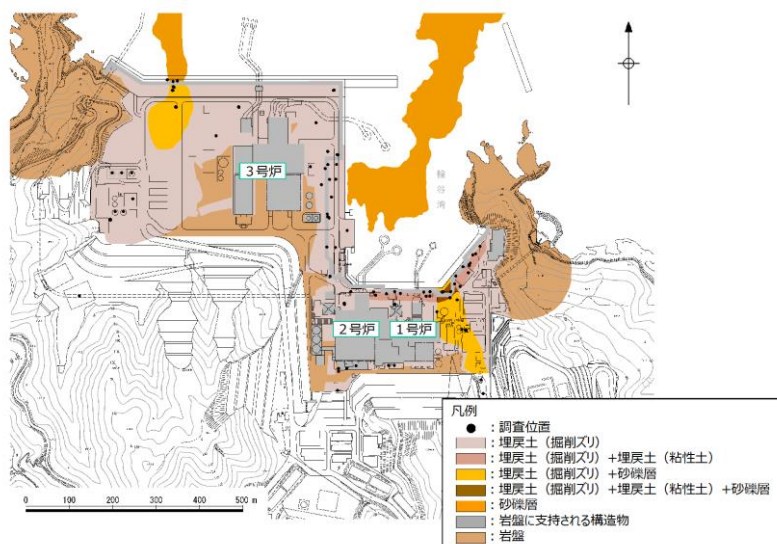
第1-53図 敷地の被覆層 平面図
