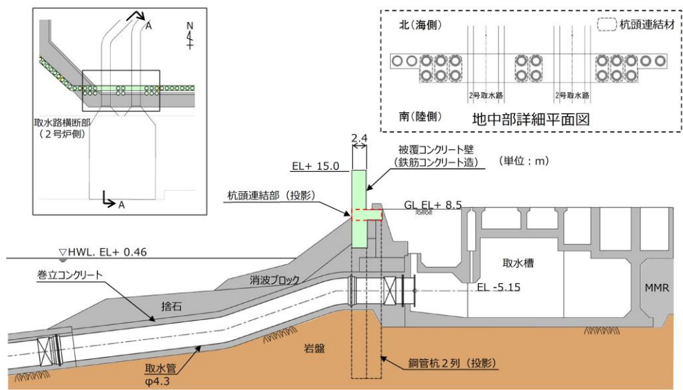
第 1-80 図 防波壁（多重鋼管杭式擁壁）取水路横断部 （2号炉側，A－A断面） 断面図
