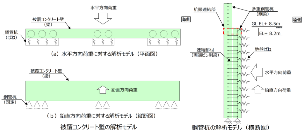
第 1-100 図 解析モデル
