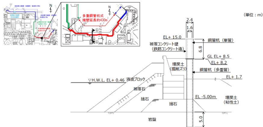
第1-14(1) 図 防波壁（多重鋼管杭式擁壁）一般部（①－①）断面図
