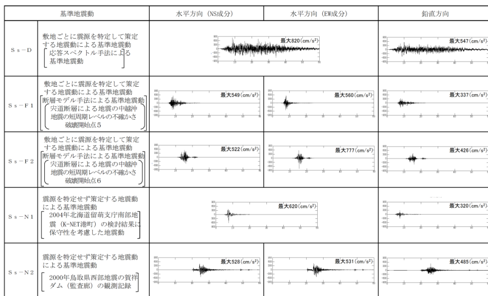
第 1-104 図 基準地震動 S s の時刻歴波形
