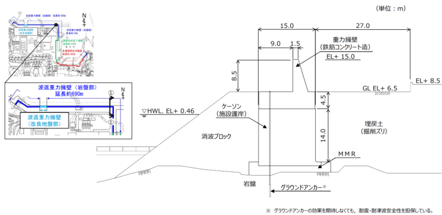
第 1-24(1) 図 防波壁（波返重力擁壁）一般部（①－①）断面図
