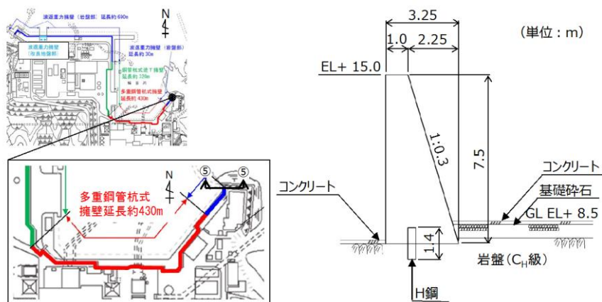
第1-24(5) 図 防波壁 (波返重力擁壁) 東端部 (⑤-⑤) 断面図
