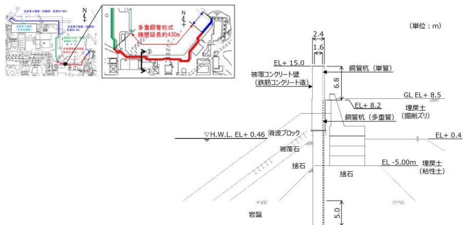
第1-14(3) 図 防波壁（多重鋼管杭式擁壁）施設護岸前出し部（③－③）断面図
