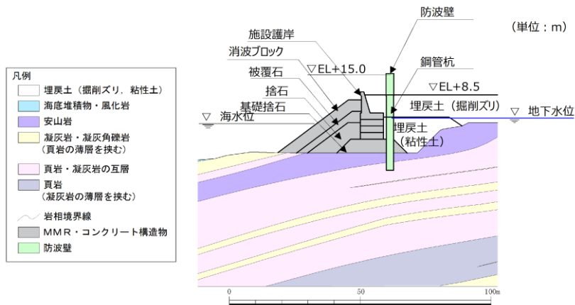
第 1-56 図 防波壁 (多重鋼管杭式擁壁) の地質断面図 (①-①)
