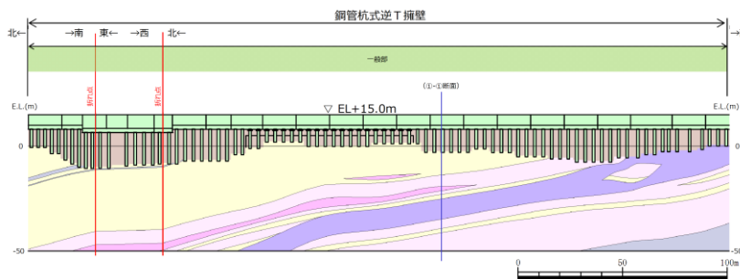
第1-60図 防波壁（鋼管杭式逆T擁壁）の岩相縦断面図
