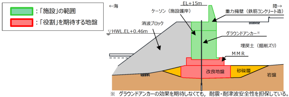
第 1-26 図 防波壁（波返重力擁壁）（地盤改良部）における「施設」と「地盤」の区分
