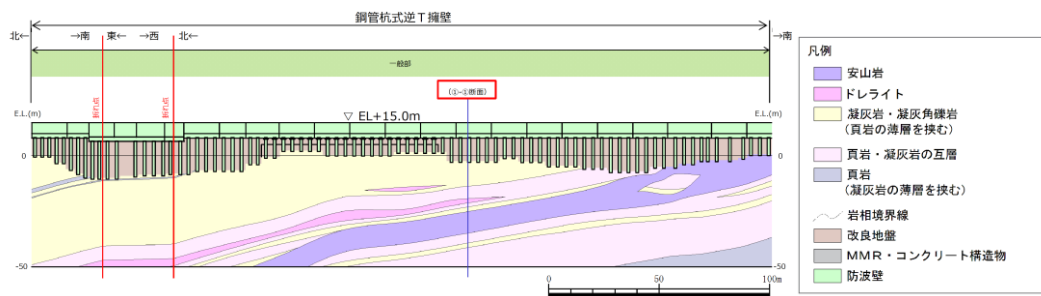
第 2-6 図 構造成立性評価断面候補地点の断面図（防波壁（鋼管杭式逆 T 擁壁））
