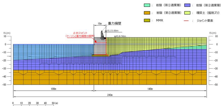
第4図 波返重力擁壁の解析モデル図 (例)
