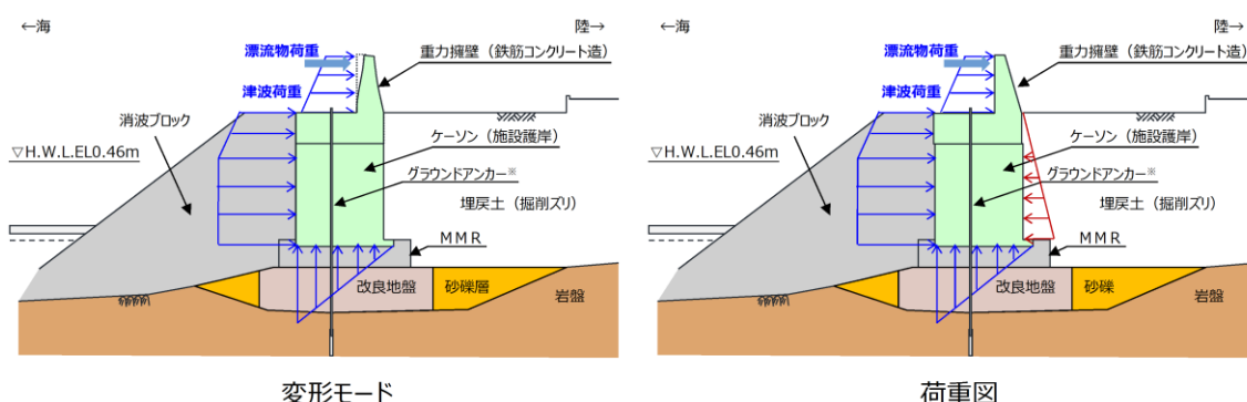
第 1-73 図 防波壁（波返重力擁壁）の変形モード及び荷重図（地震時）
