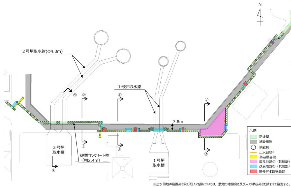
第 1-13 図 防波壁（多重鋼管杭式擁壁）の平面図
