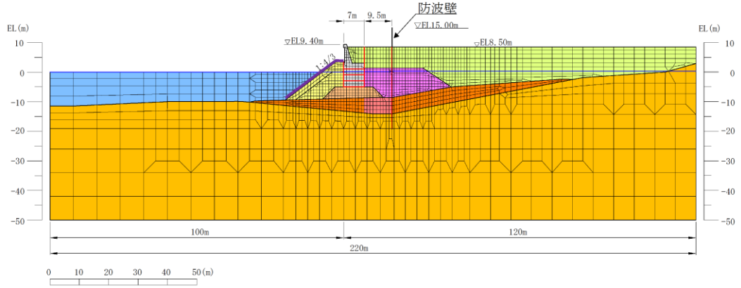
第 1-86 図 防波壁（多重鋼管杭式擁壁）の解析モデル
