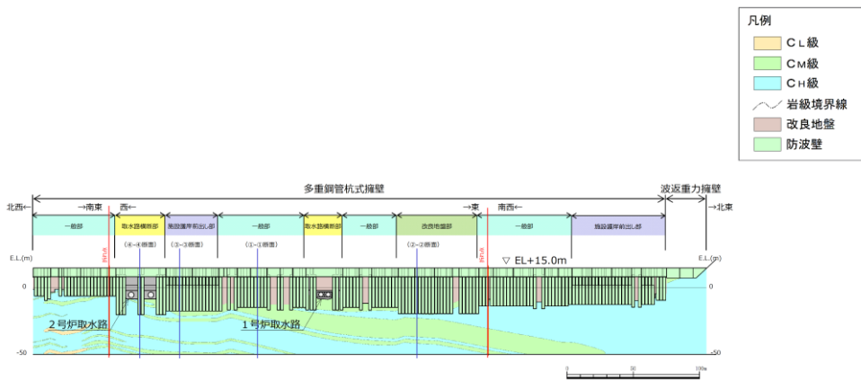
第 1-55 図 防波壁（多重鋼管杭式擁壁）の岩級縦断面図
