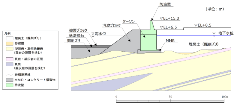
第 1-65 図 防波壁（波返重力擁壁）の地質断面図 (①-①)
