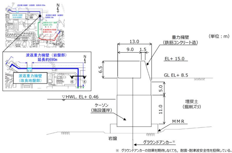
第1-24(4) 図 防波壁 (波返重力擁壁) 輪谷部 (④-④) 断面図
