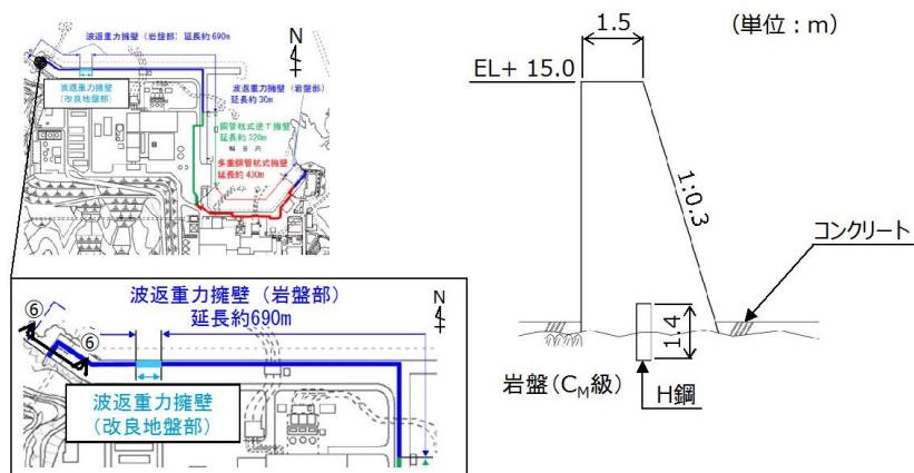
第1-24(6) 図 防波壁 (波返重力擁壁) 西端部 (⑥-⑥) 断面図
