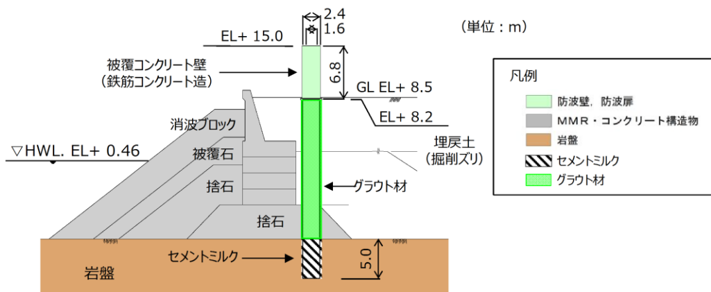
第 1-82 図 防波壁（多重鋼管杭式擁壁）杭間部（A-A 断面） 断面図
