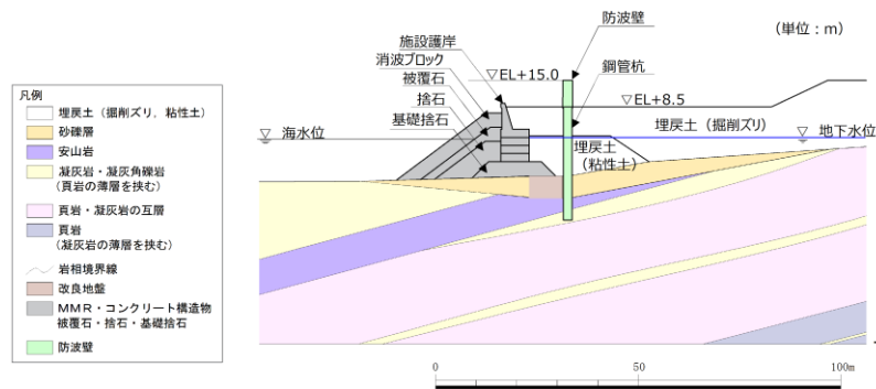
第 1-57 図 防波壁 (多重鋼管杭式擁壁) の地質断面図 (②-②)
