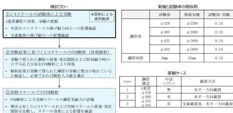
第 2 図 試験の概要
