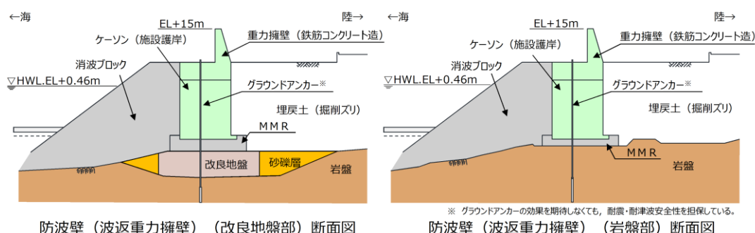
第1-21図 防波壁（波返重力擁壁）の構造概要図
