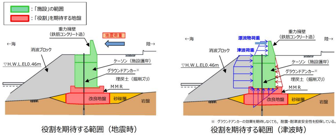
第 1-8 図 防波壁（波返重力擁壁）の役割を期待する範囲
