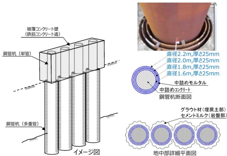
第 1-11 図 防波壁（多重鋼管杭式擁壁）の構造概要図
