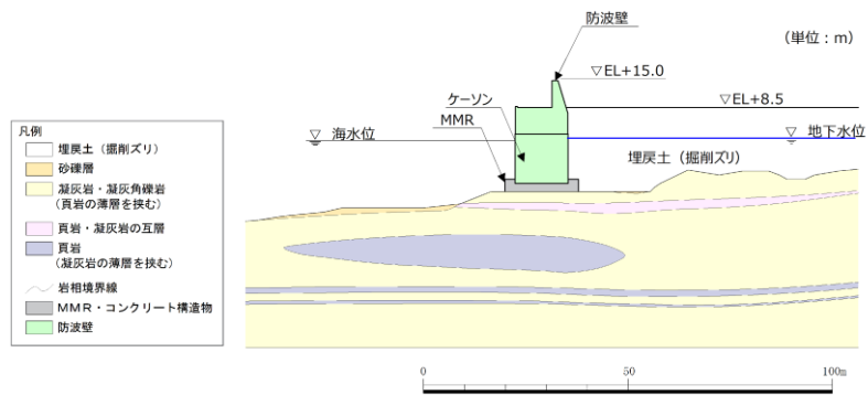
第 1-68 図 防波壁 (波返重力擁壁) の地質断面図 (④-④)
