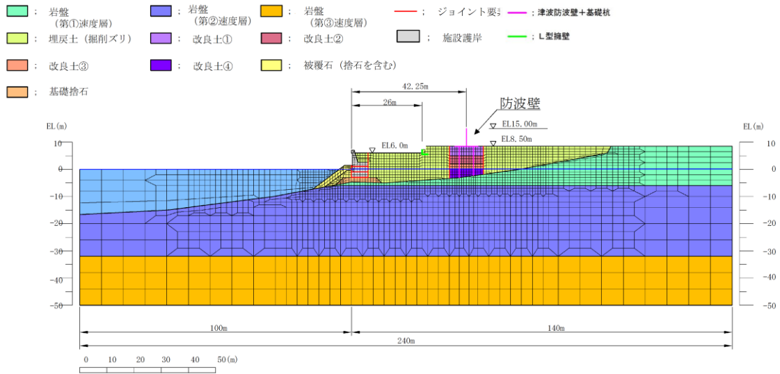
第 1-90 図 防波壁（鋼管杭式逆 T 擁壁）の解析モデル
