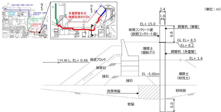
第1-14(2) 図 防波壁（多重鋼管杭式擁壁）改良地盤部（②－②）断面図
