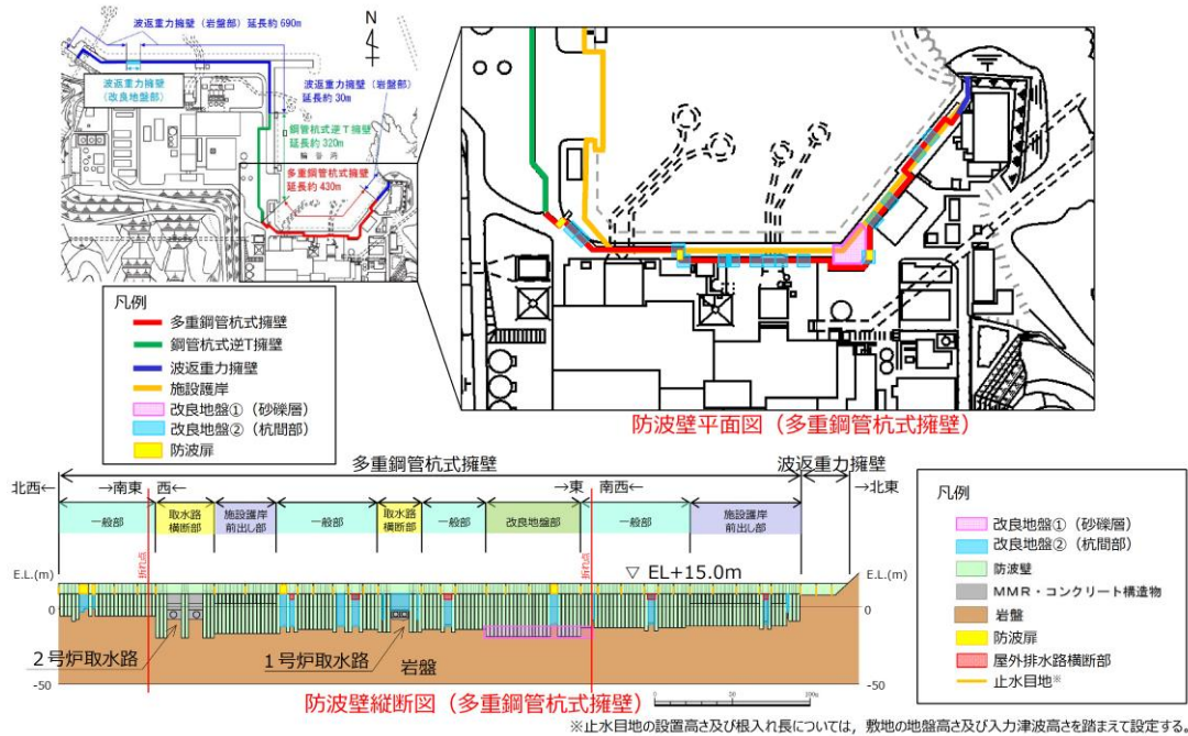
第 1-12 図 防波壁（多重鋼管杭式擁壁）の縦断図
