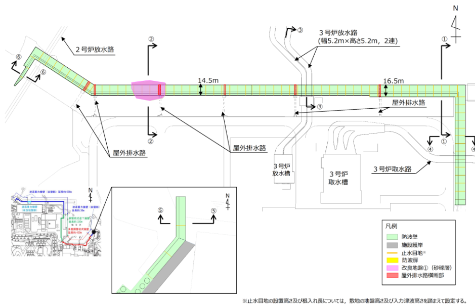
第 1-23 図 防波壁 (波返重力擁壁) の平面図
