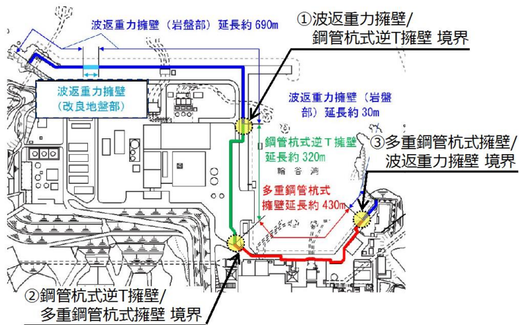
第 1-51 図 防波壁の構造形式の境界位置図
