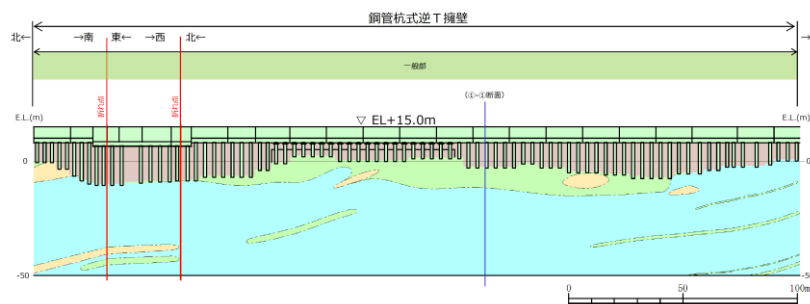
第1-61図 防波壁（鋼管杭式逆T擁壁）の岩級縦断面図
