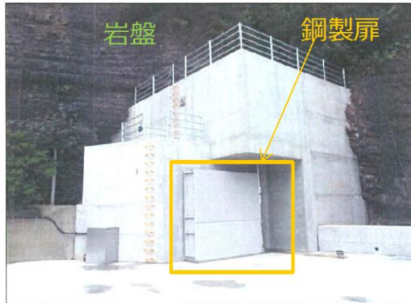
第 1-48 図 防波壁通路防波扉（1号放水連絡通路防波扉）⑤ 設置状況
