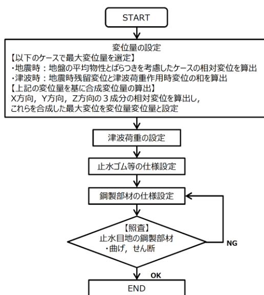
第 1-97 図 設計フロー
