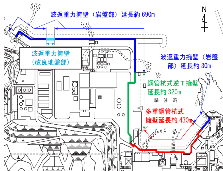
第 1-1 図 防波壁の平面図
