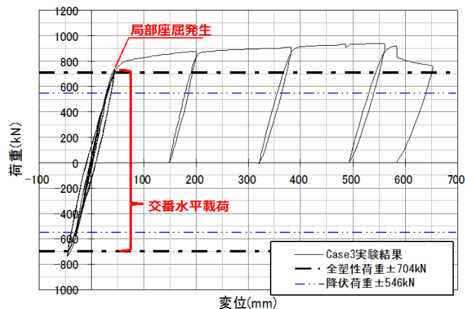
第7 図 水平荷重と変位の関係
