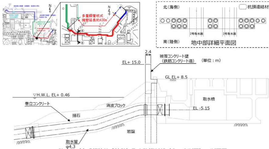
第1-14(4) 図 防波壁（多重鋼管杭式擁壁）取水路横断面（④－④）断面図
