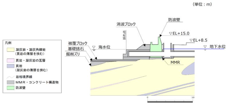
第 1-67 図 防波壁 (波返重力擁壁) の地質断面図 (③-③)
