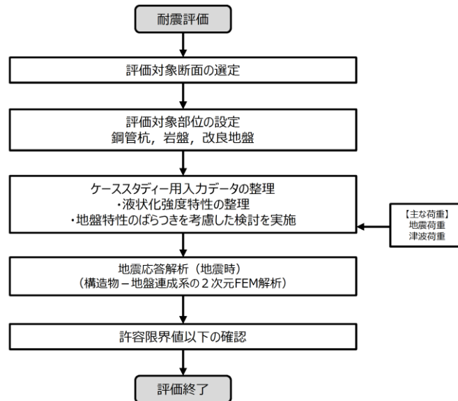
第 1-98 図 設計フロー
