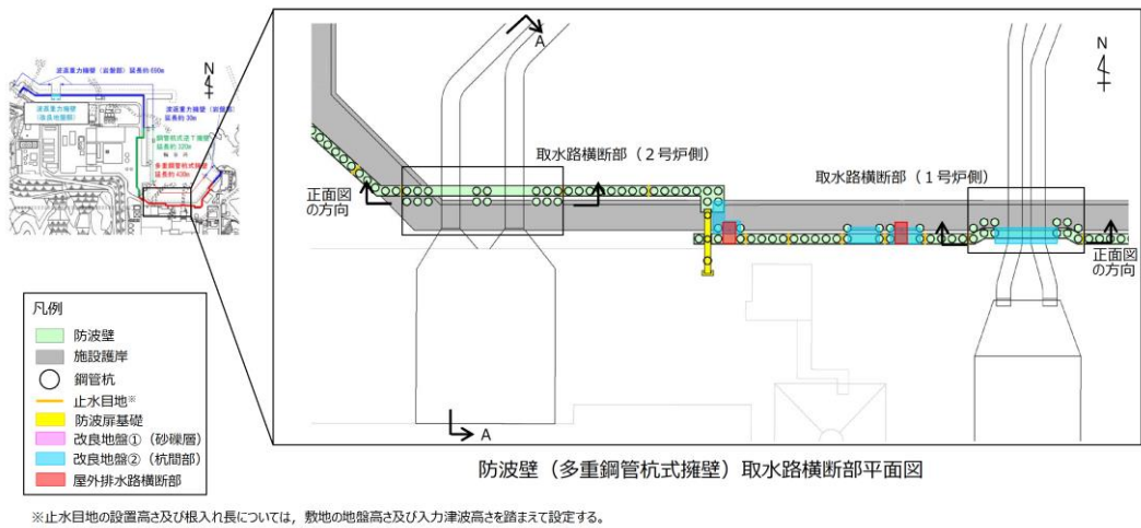
第 1-78 図 防波壁（多重鋼管杭式擁壁）取水路横断部平面図
