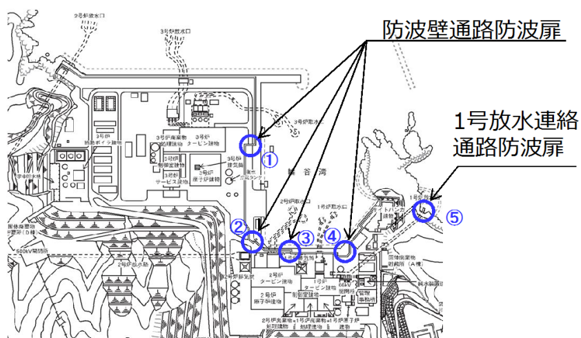
第1-34 図 防波壁通路防波扉の位置図
