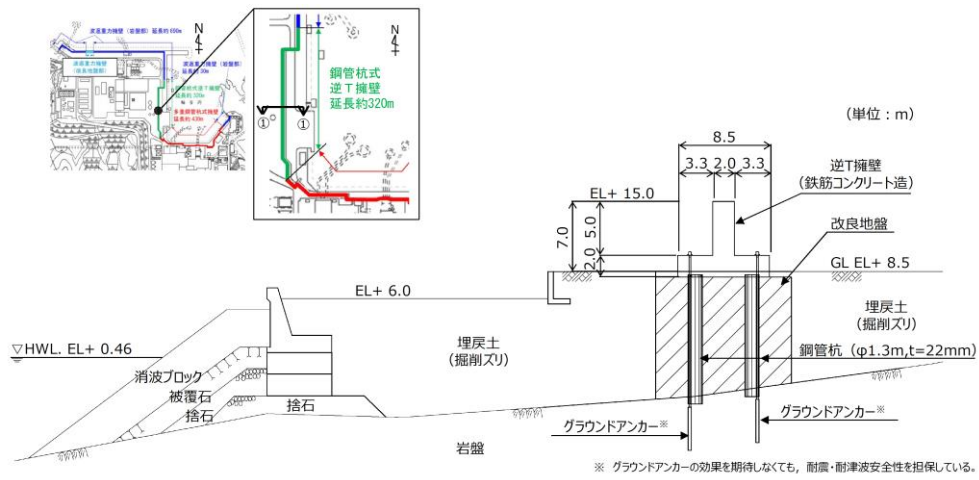
第 1-19 図 防波壁（鋼管杭式逆T擁壁）一般部（①—①断面）断面図
