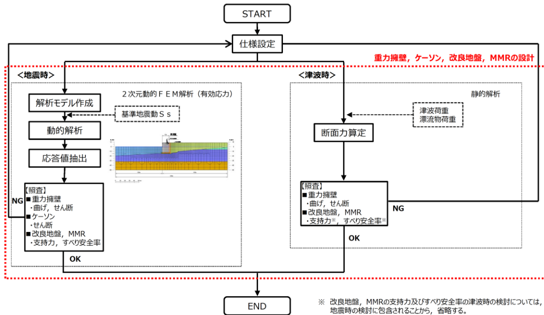
第 1-95 図 防波壁（波返重力擁壁）の解析概要
