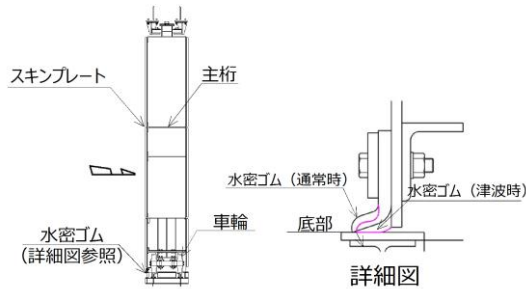
第 1-42 図 防波壁通路防波扉（1，2号炉北側）④ 断面図
