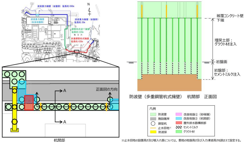
第 1-81 図 防波壁（多重鋼管杭式擁壁）杭間部正面図
