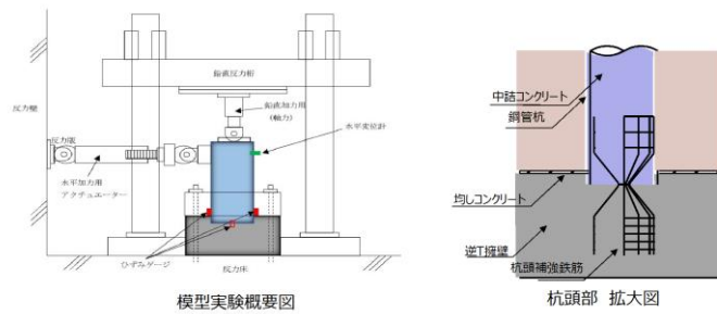
第3図 模型実験概要図
