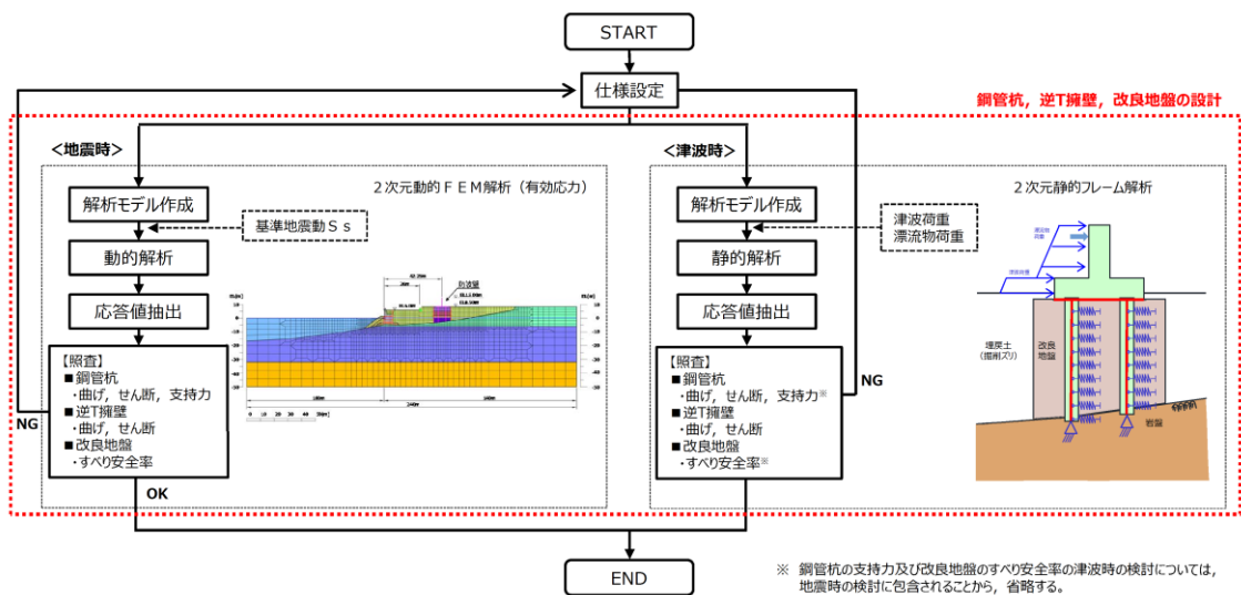
第 1-91 図 防波壁（鋼管杭式逆 T 擁壁）の解析概要
