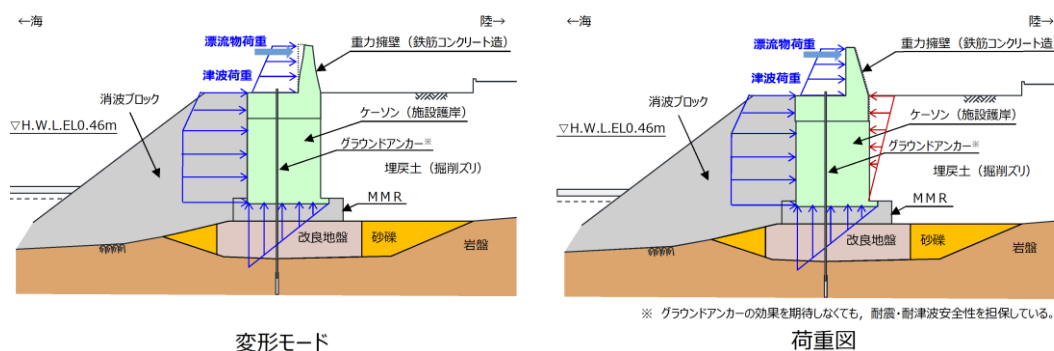
第 1-76 図 防波壁（波返重力擁壁）の変形モード及び荷重図（津波時）
