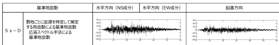
第 2-27 図 解析に用いた SS
