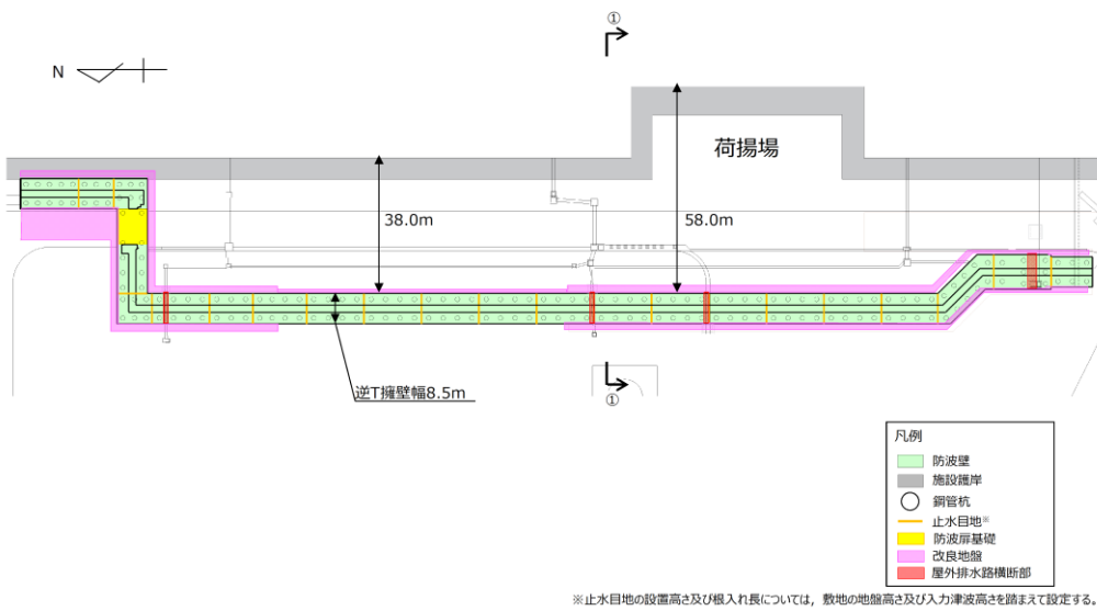
第 1-18 図 防波壁 (鋼管杭式逆 T 擁壁) 平面図
