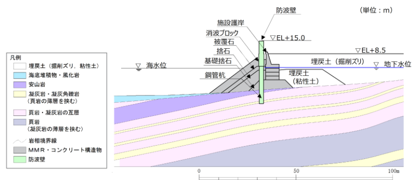
第 1-58 図 防波壁 (多重鋼管杭式擁壁) の地質断面図 (③-③)
