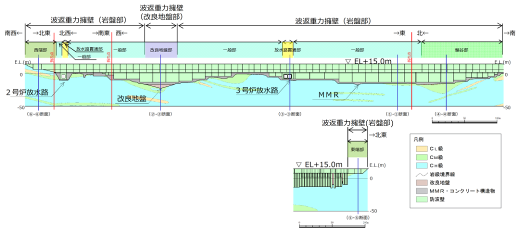
第 1-64 図 防波壁（波返重力擁壁）の岩級縦断図
