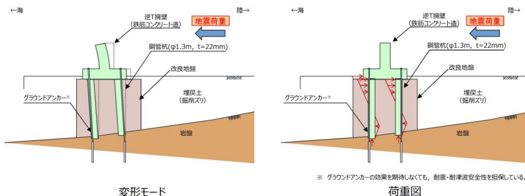
第1-72図 防波壁（鋼管杭式逆T擁壁）の変形モード及び荷重図（地震時）
