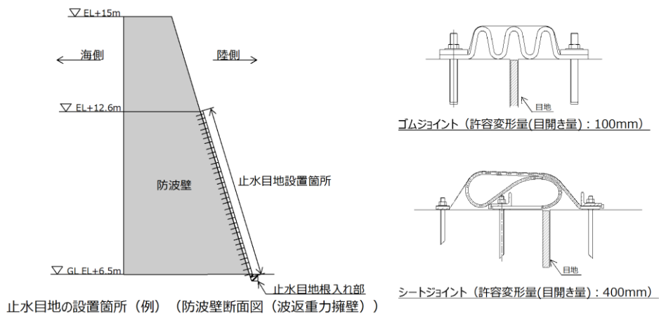
第 1-50 図 防波壁の止水目地の設置箇所及び概要図
