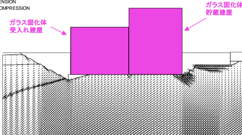
主応力図
