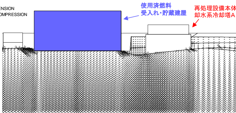
主応力図
