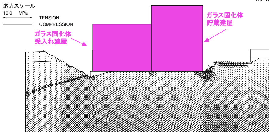
主応力図
