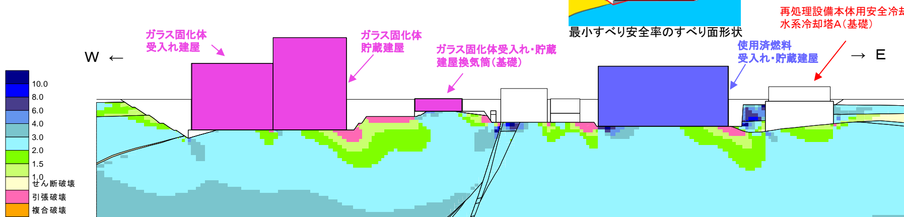
局所安全係数分布図
