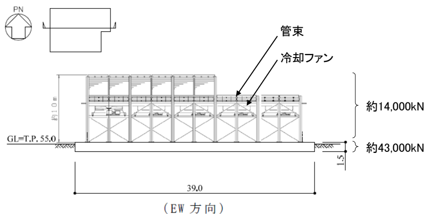
再処理設備本体用安全冷却水系冷却塔 断面図
