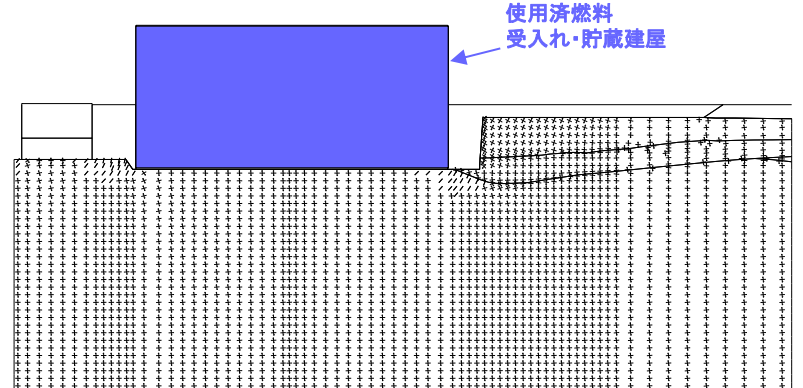
モビライズド面 (使用済燃料受入れ・貯蔵建屋周辺拡大)
