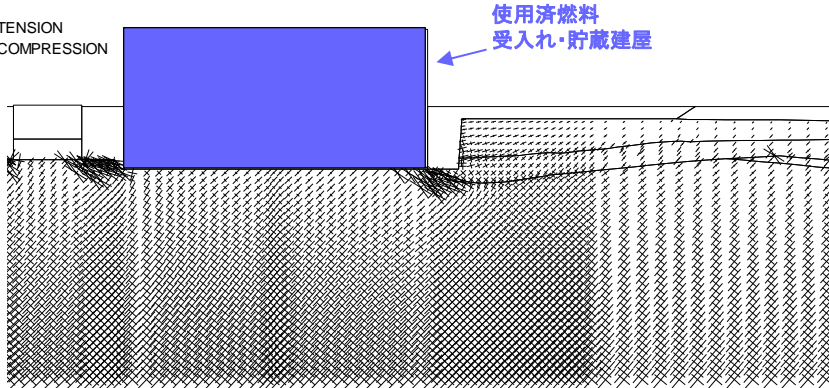
主応力図 (使用済燃料受入れ・貯蔵建屋周辺拡大)
