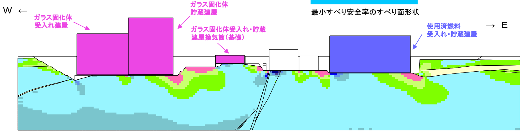
応カスケール 10.0 MPa ← TENSION COMPRESSION →
