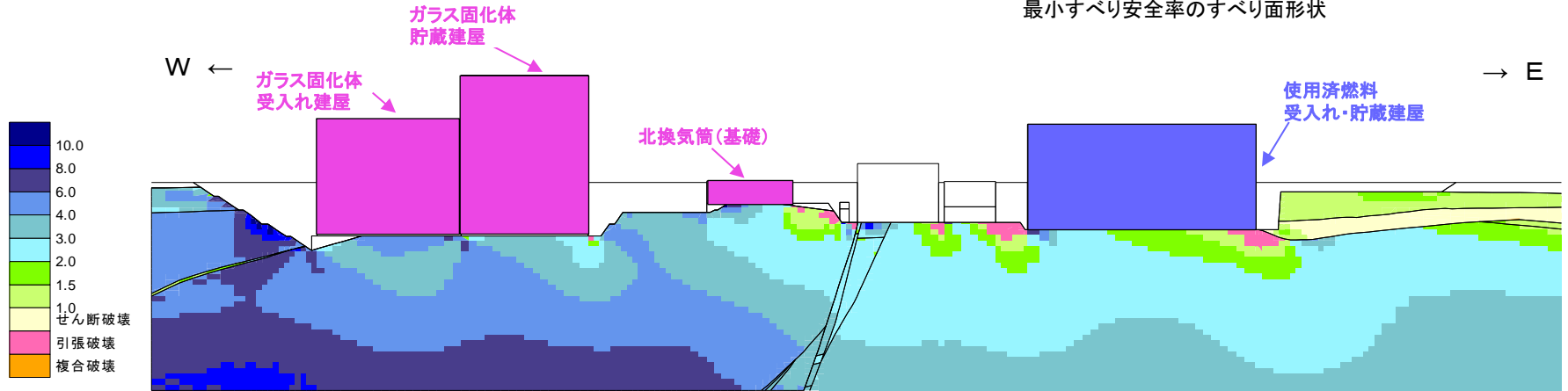
局所安全係数分布図
