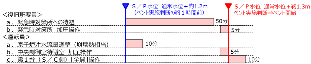
図2 ベント実施に係る対応の流れ
