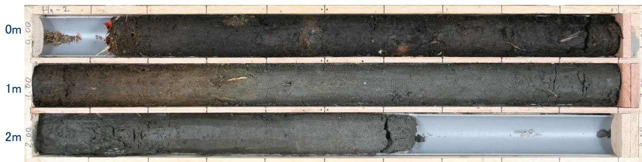
【Hn-2(孔口標高:T.P.+2.67m)】
