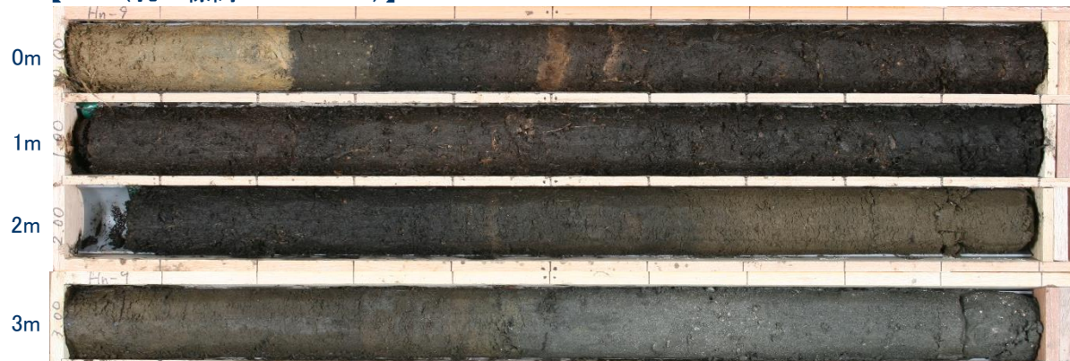
【Hn-9(孔口標高:T.P.+5.47m)】
