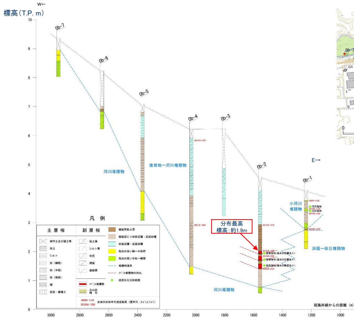
尾駮老部川地点における調査結果(地質断面図)
