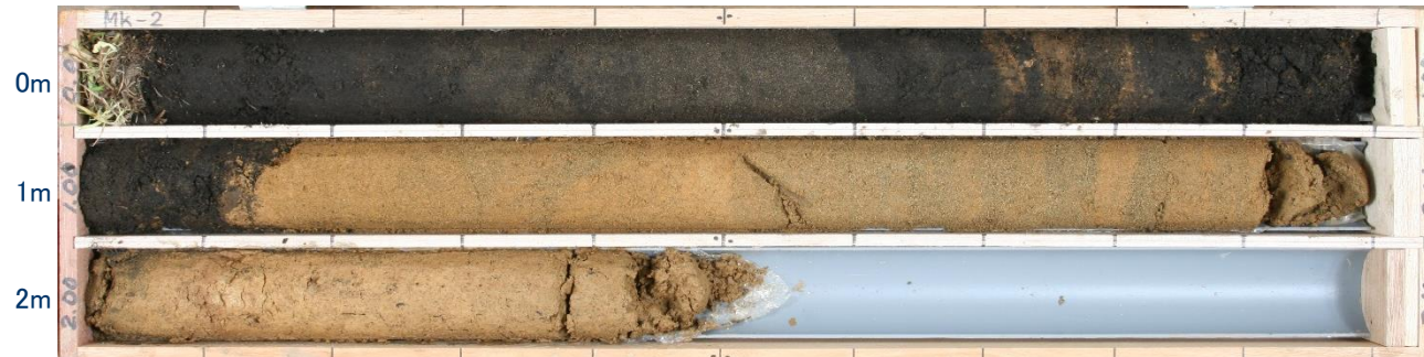
【Mk-2(孔口標高:T.P.+9.04m)】
