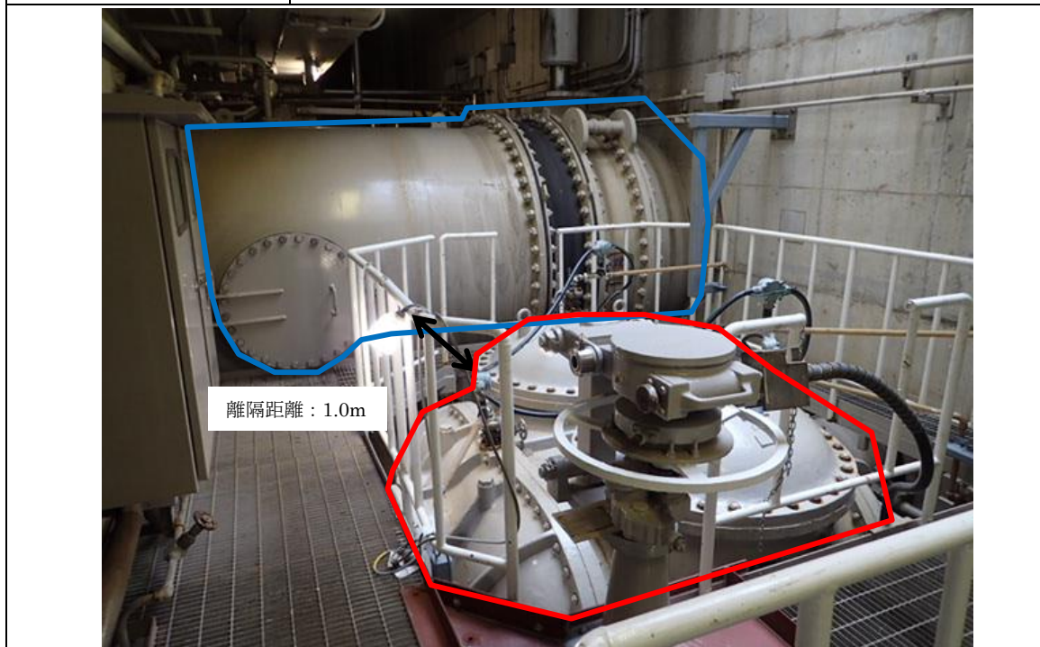
図 4-6 上位クラス施設と下位クラス施設の位置関係 (例④)
