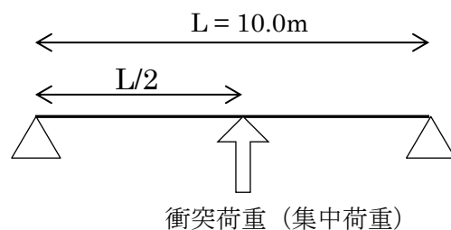
図 3.4-4 応力算出モデル
