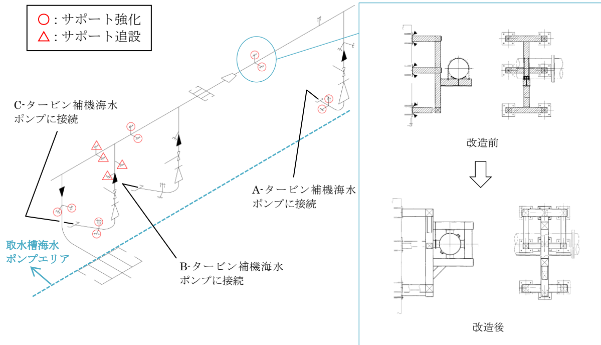
図 5-2 タービン補機海水系配管の耐震補強概要図（案）
