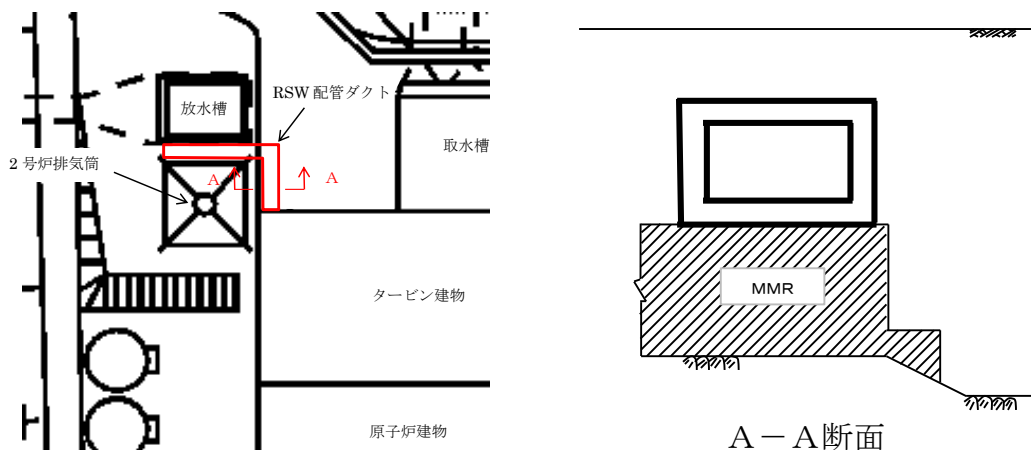
第 2-2 図 RSW 配管ダクト配置概要図
