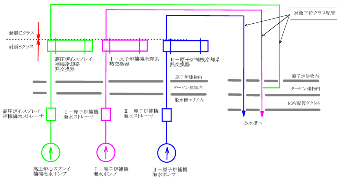
第 2-1 図 原子炉補機海水系及び高圧炉心スプレー補機海水系の系統概要図
