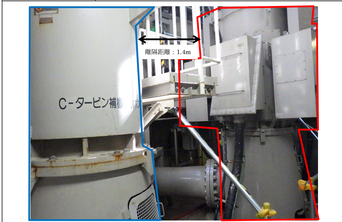
図 4-3 上位クラス施設と下位クラス施設の位置関係 (例①)
