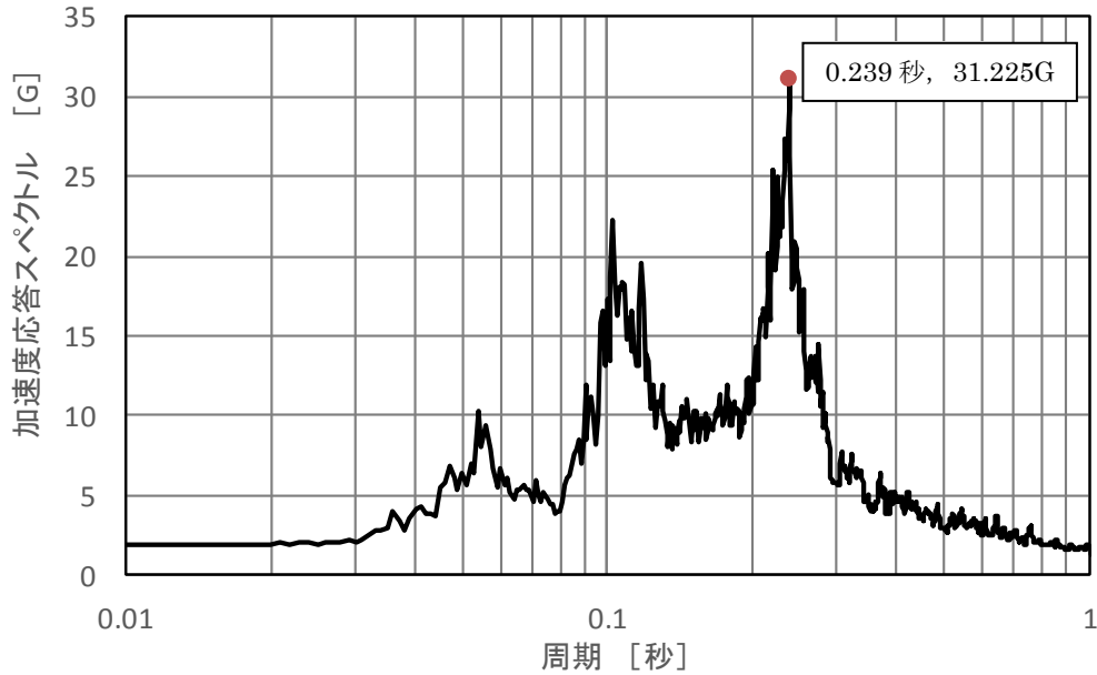
図 2.2-1 加速度応答スペクトル (減衰 0.5%)
