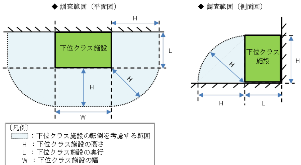
図 4-2 下位クラス施設の転倒を想定した抽出方法（概要図）
