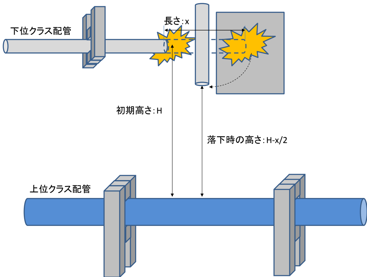
図 3.3-1 下位クラス配管の初期高さ及び長さ設定の概要図
