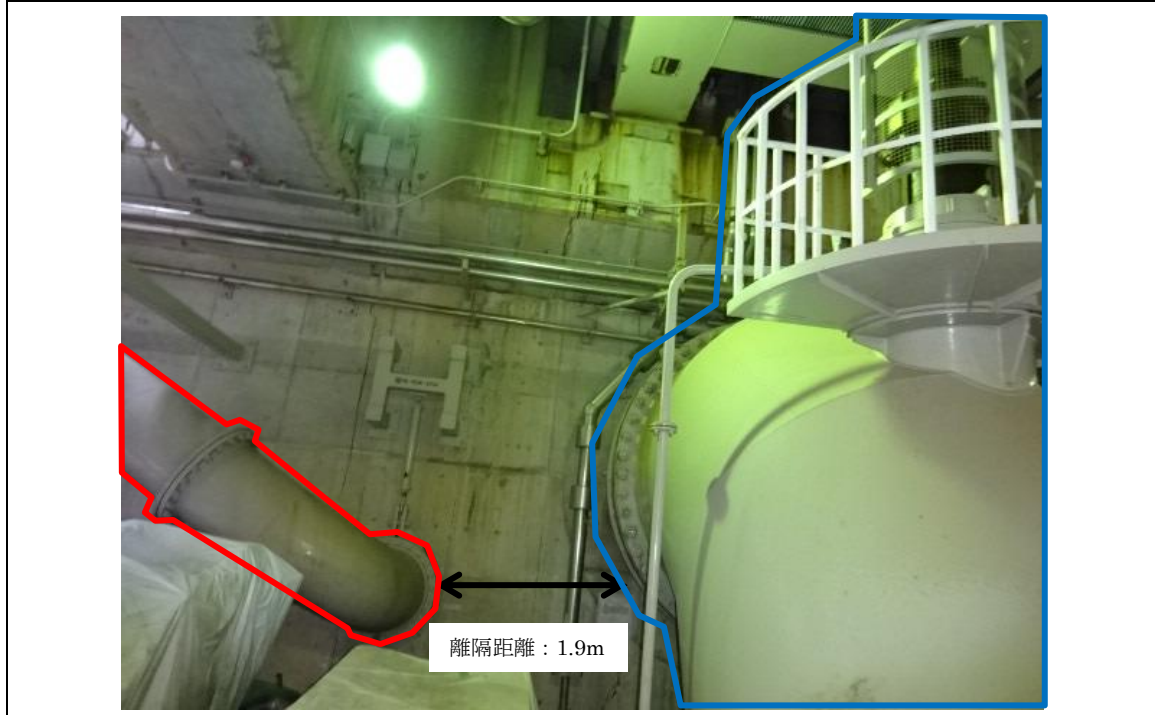
図 4-5 上位クラス施設と下位クラス施設の位置関係 (例③)
