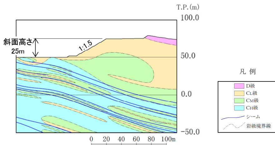
第22図 ⑥-⑥'断面の検討断面の選定根拠
