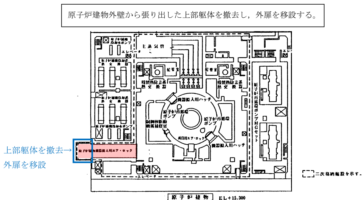
第3図 大物搬入口の耐震対策工事概要
