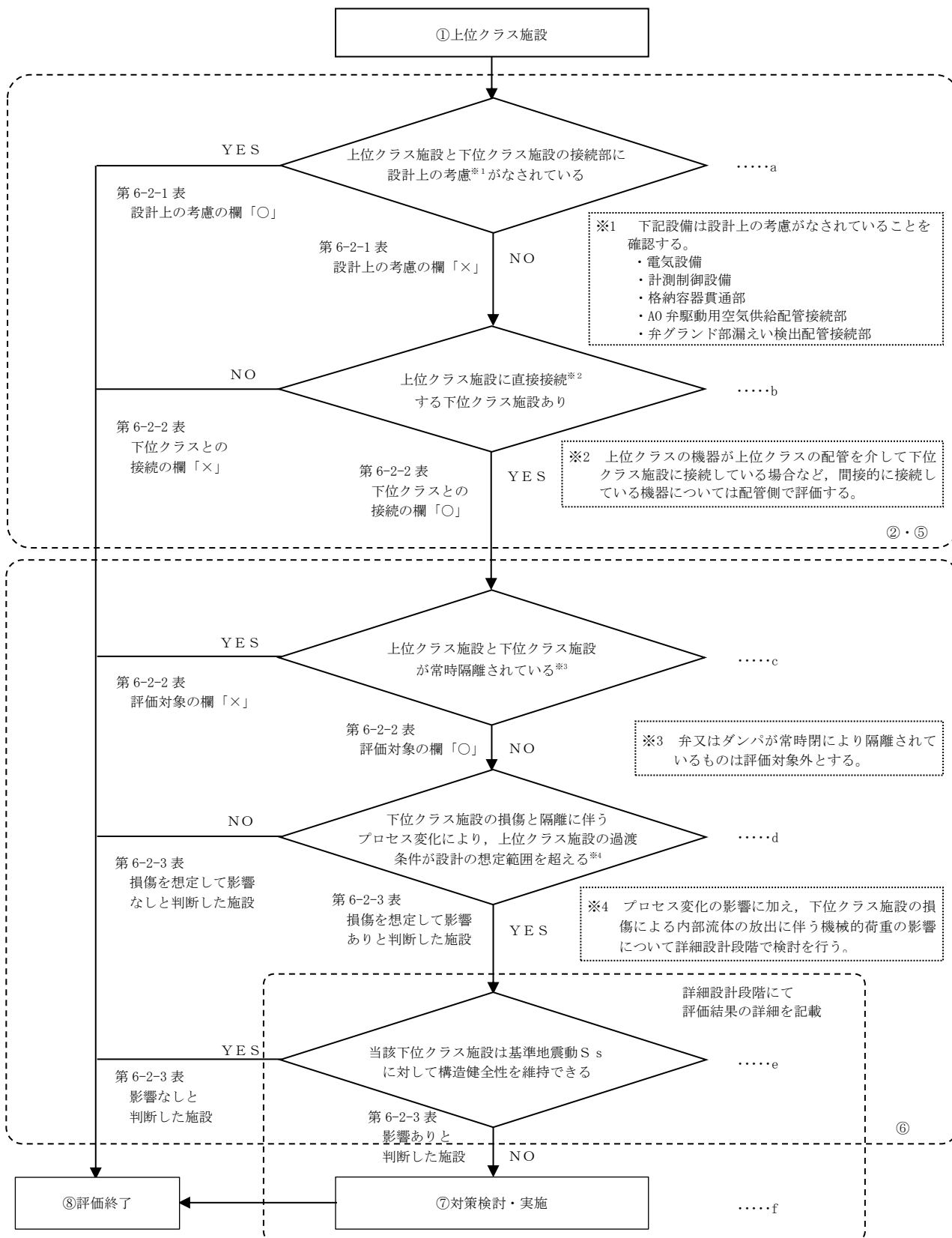
第5-2-7図 上位クラス施設と接続する下位クラス施設の抽出及び評価フロー
