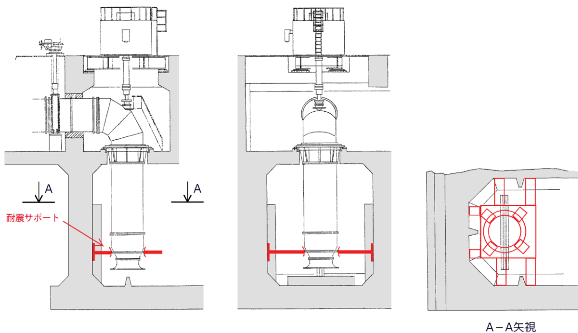
図 5-1 循環水ポンプ耐震補強概要図（案）
