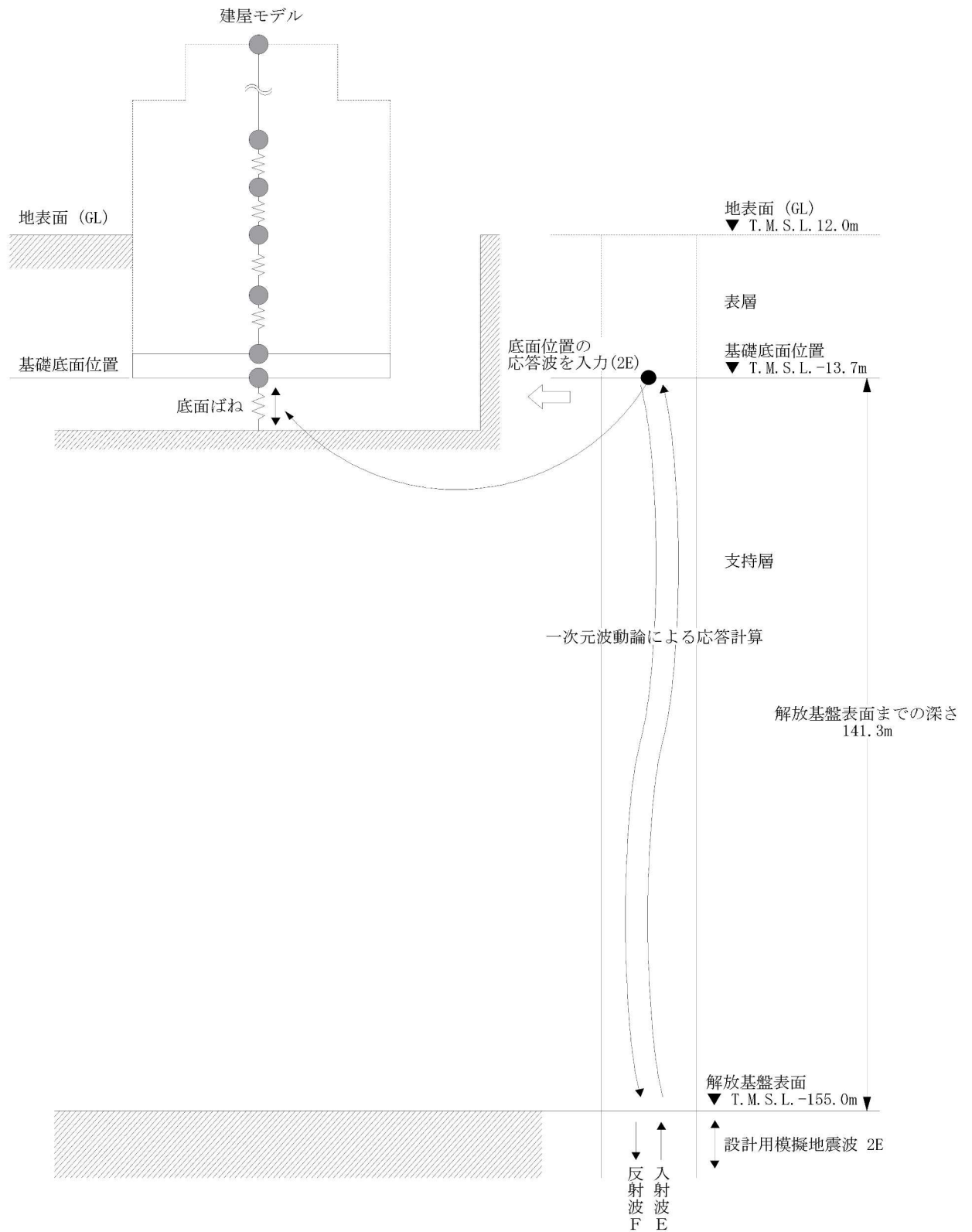
図3-14 地震応答解析モデルに入力する地震動の概念図（鉛直方向）
