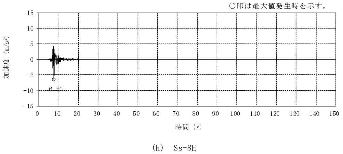
図3-1 加速度時刻歴波形（基準地震動 S s ，NS方向）（3/3）
