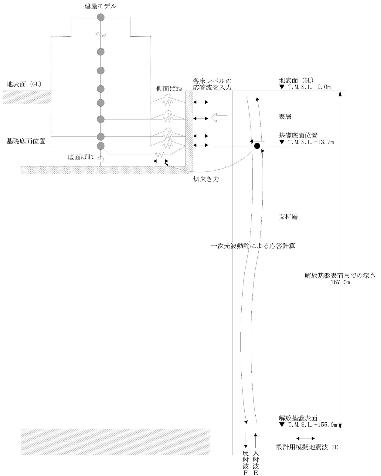
図3-10 地震応答解析モデルに入力する地震動の概念図（水平方向）
