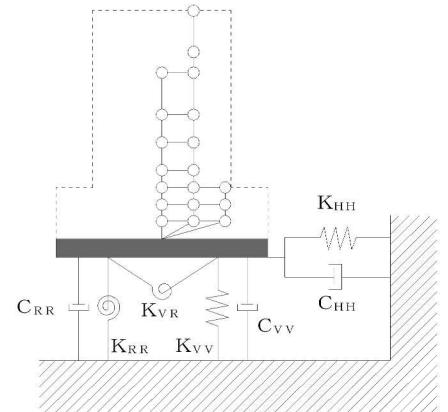
図3-22 誘発上下動を考慮する場合の地震応答解析モデルの概念図
