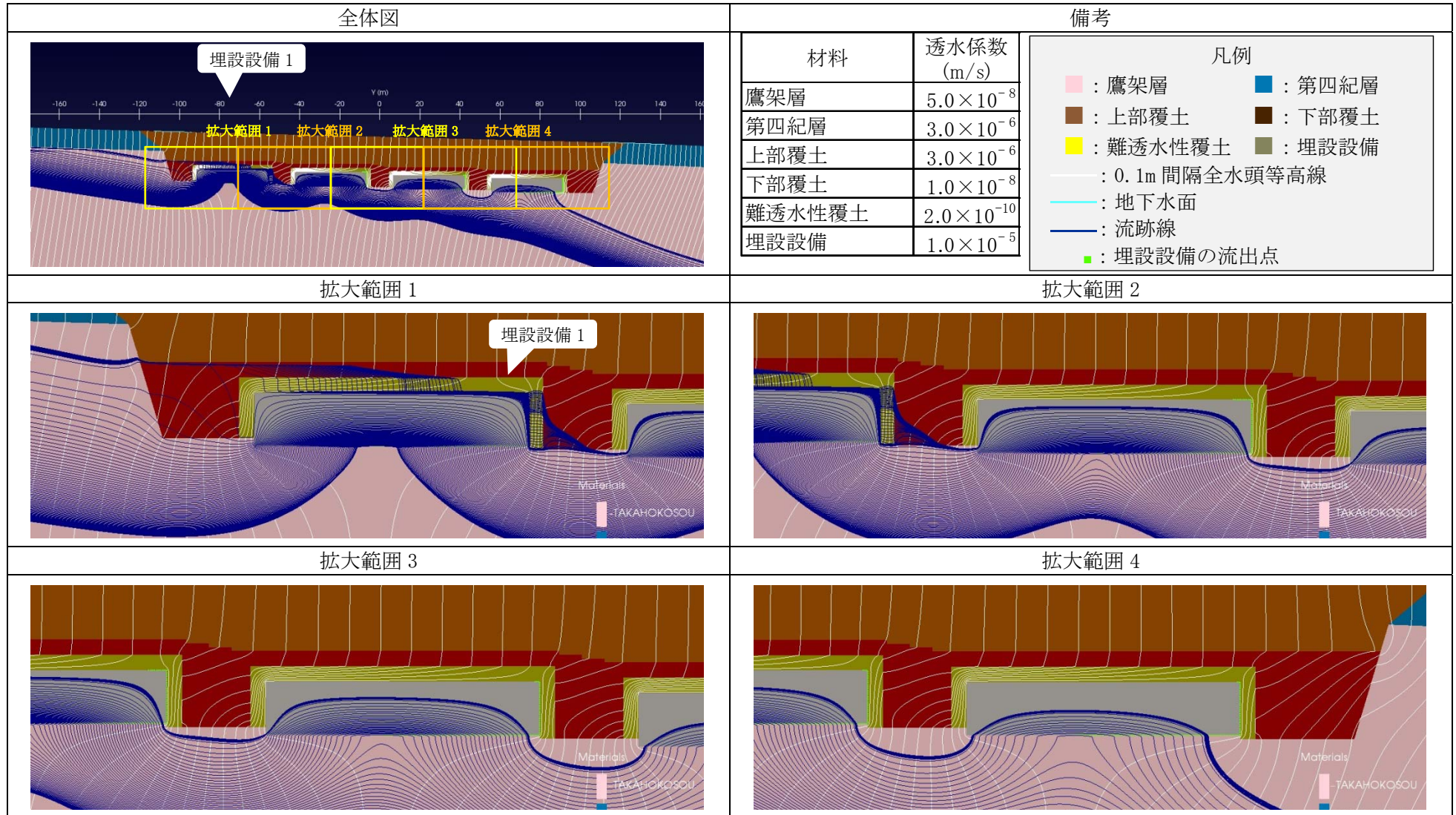
第1図 2次元地下水浸透流解析結果【3号廃棄物埋設地】(確からしい設定 1,000年後) (2/5) <埋設設備1の流出点を通る流跡線>
