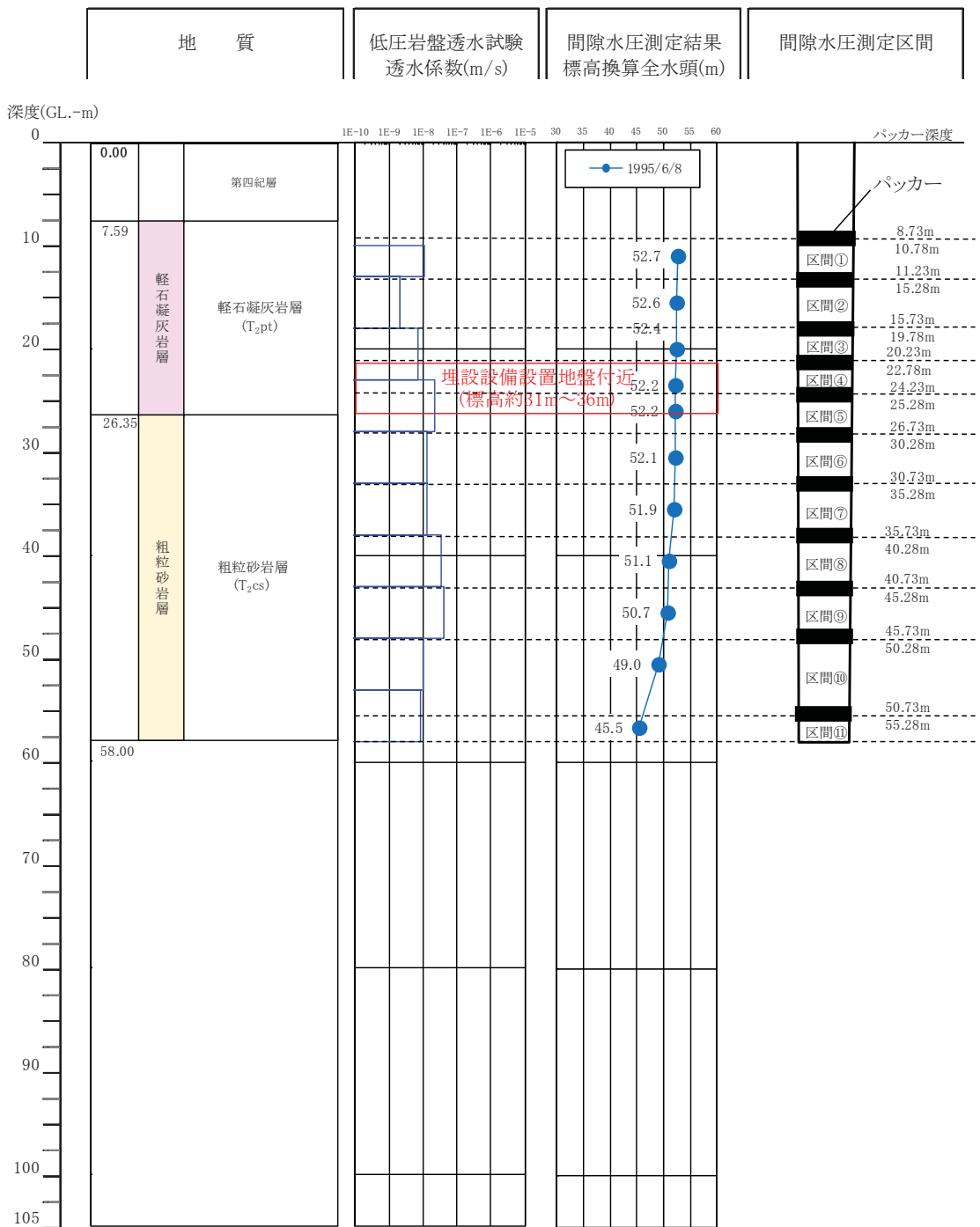
第 18 図 埋設設備設置地盤付近の間隙水圧測定孔における間隙水圧測定結果 (9/9) (2号廃棄物埋設地付近、B4-60孔、1995年6月測定)* 1
