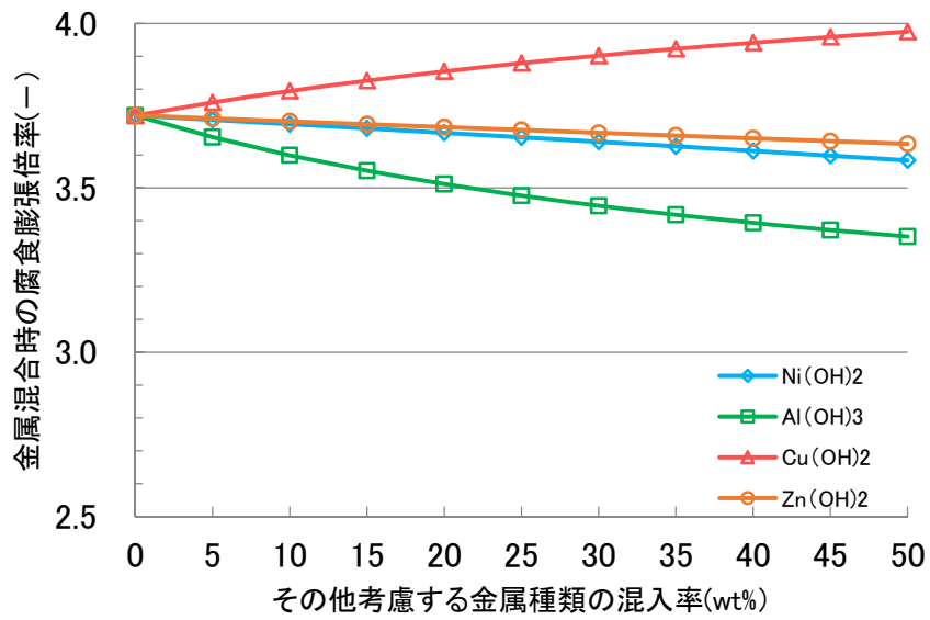
第 6 図 厳しい設定における腐食膨張倍率への影響評価
