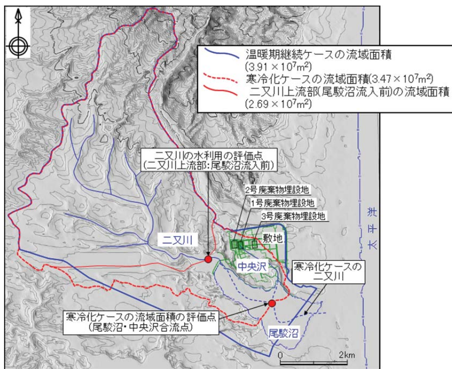
第 22 図 二又川流域の設定図
