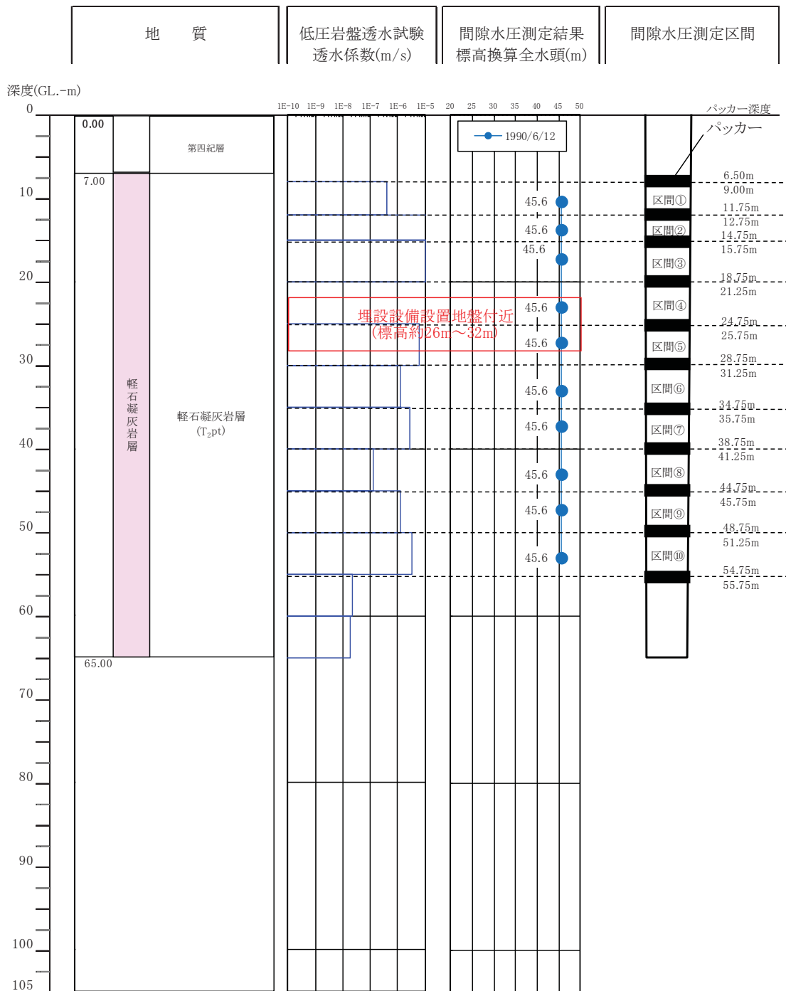
第 18 図 埋設設備設置地盤付近の間隙水圧測定孔における間隙水圧測定結果 (6/9)
