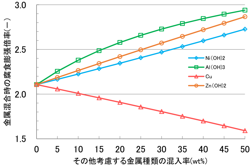
第 5 図 確からしい設定における腐食膨張倍率への影響評価
