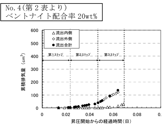
第5図 (1/2) 透気試験における圧力、応力及び排気量 (7)(8)
