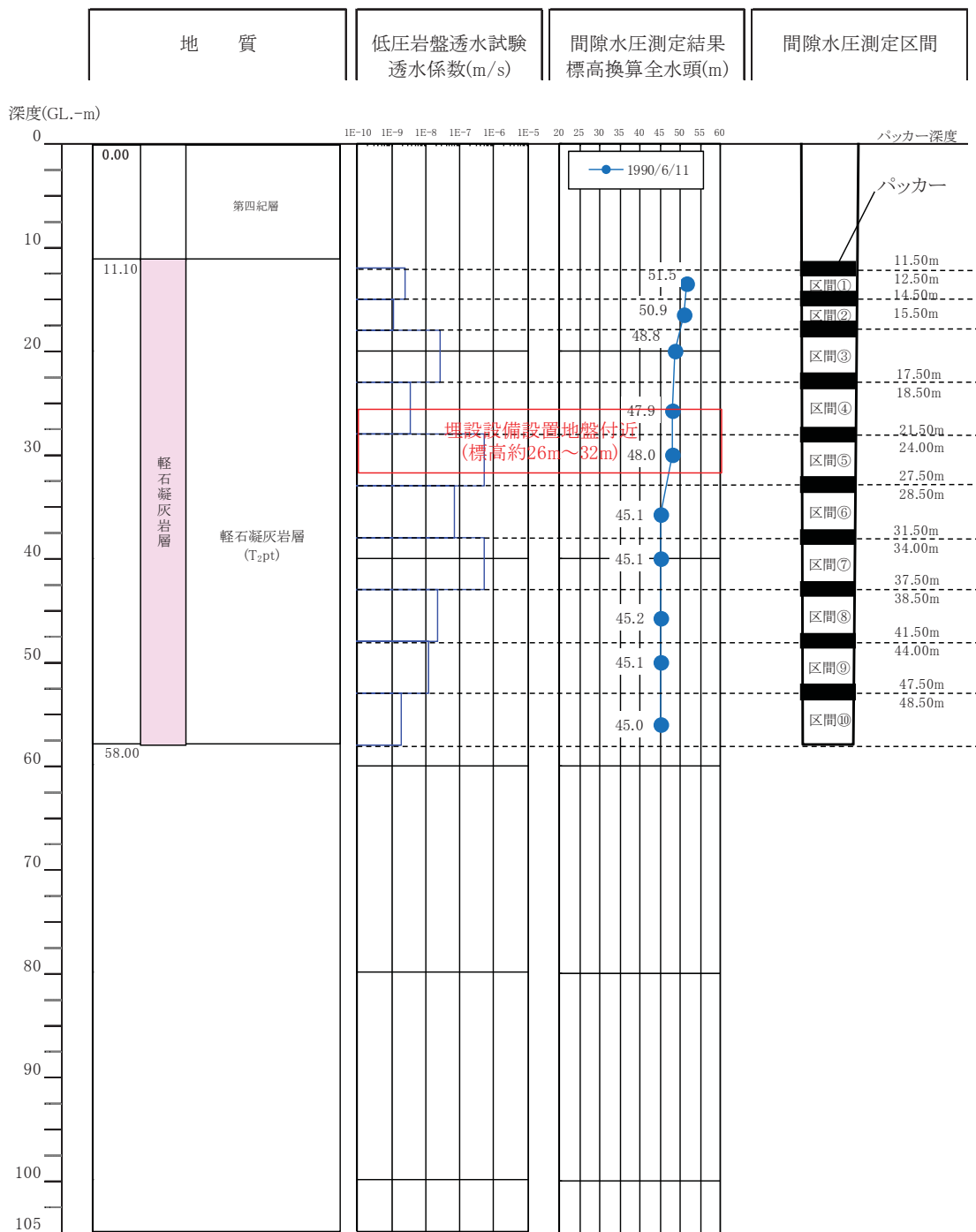
第 18 図 埋設設備設置地盤付近の間隙水圧測定孔における間隙水圧測定結果 (7/9)
