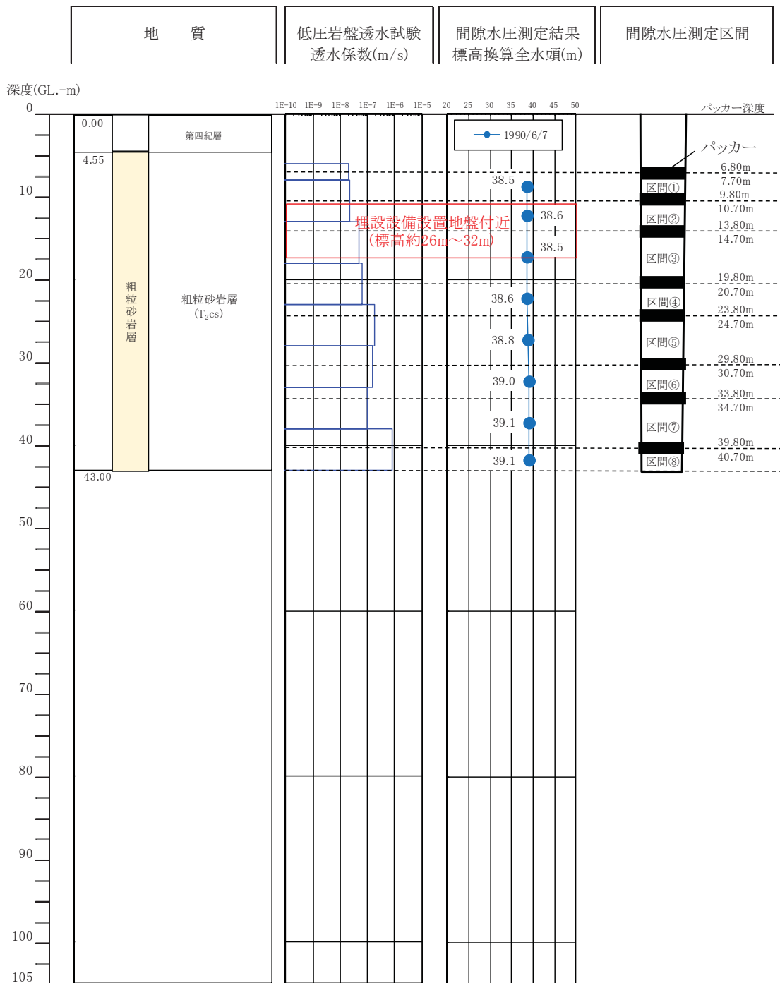
第 18 図 埋設設備設置地盤付近の間隙水圧測定孔における間隙水圧測定結果 (4/9)
