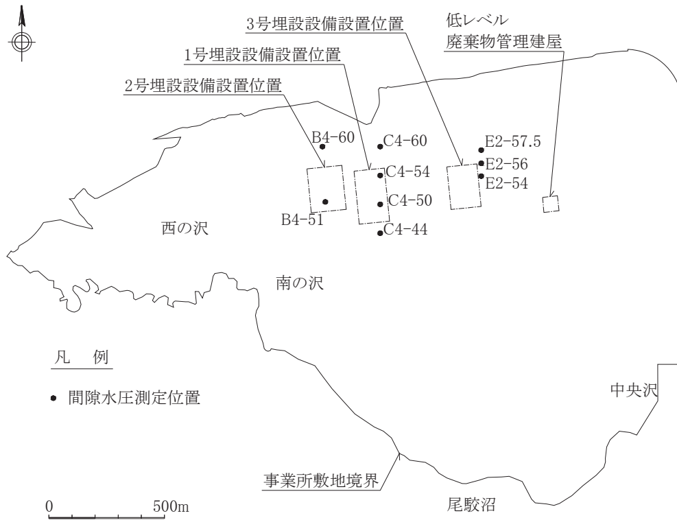
第 17 図 間隙水圧測定位置図
