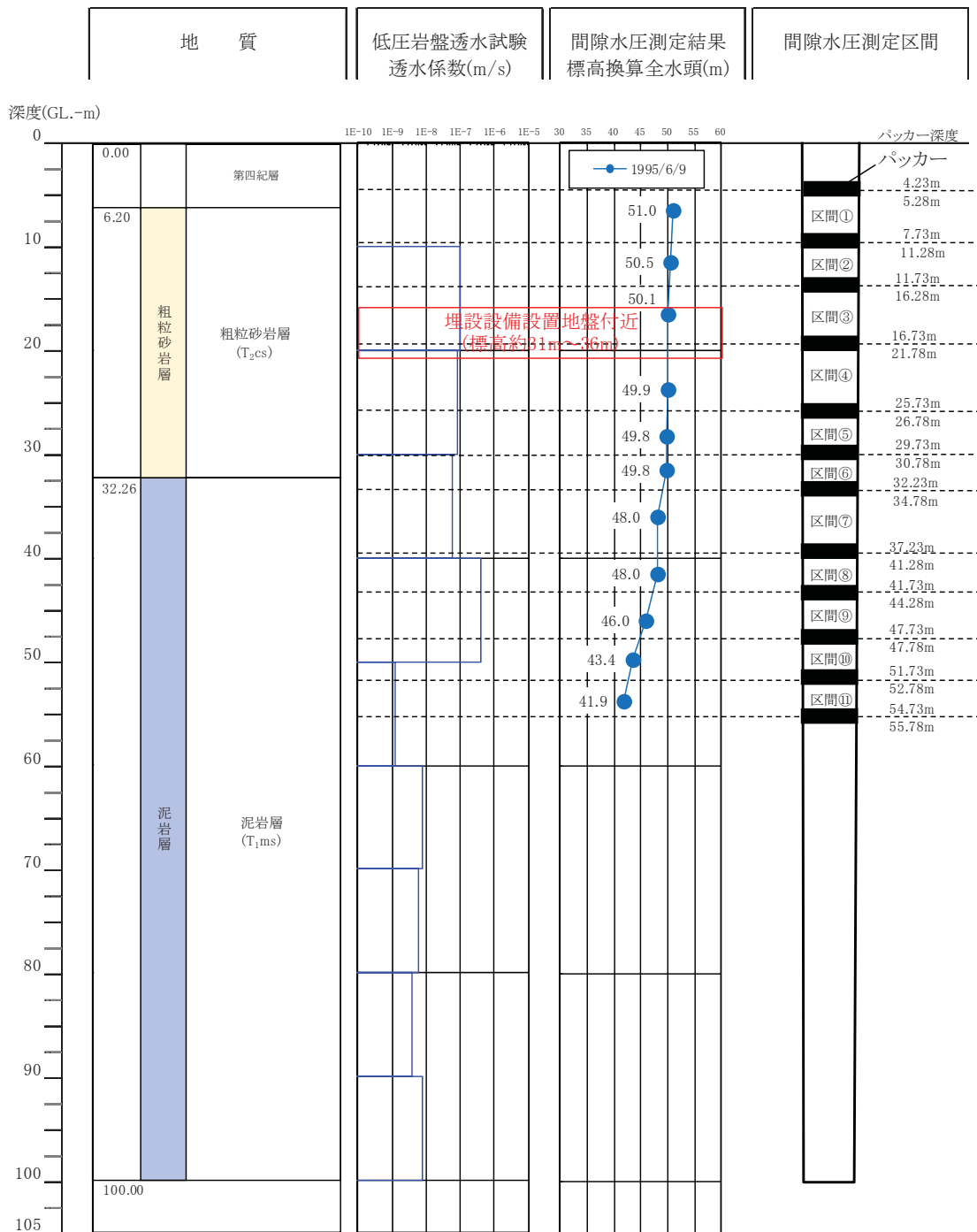
第 18 図 埋設設備設置地盤付近の間隙水圧測定孔における間隙水圧測定結果 (8/9)
