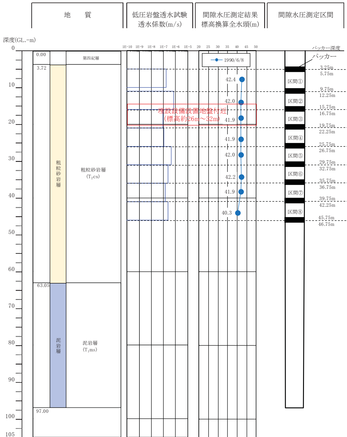
第 18 図 埋設設備設置地盤付近の間隙水圧測定孔における間隙水圧測定結果 (5/9)
