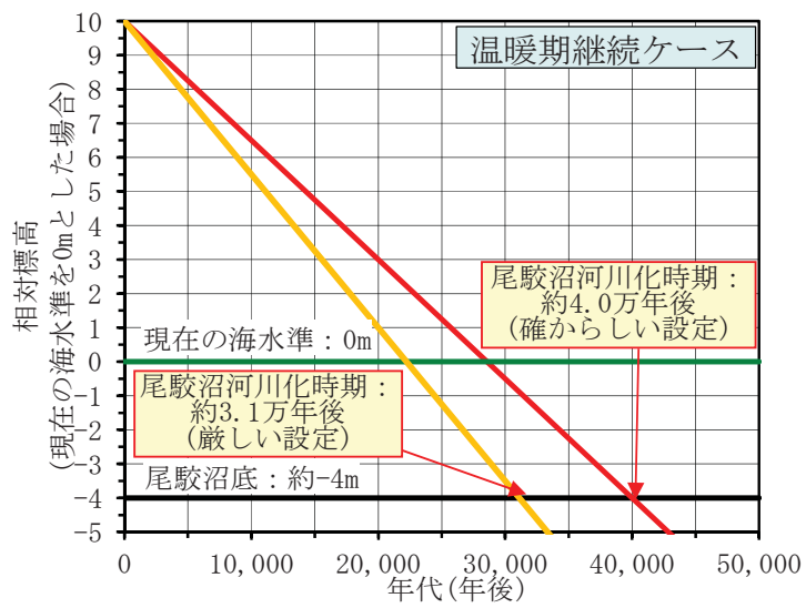
第 27 図 相対海水準の低下による尾駁沼の河川化時期*1
