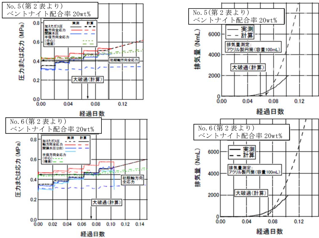
第5図(2/2) 透気試験における圧力、応力及び排気量 (7)(8)
