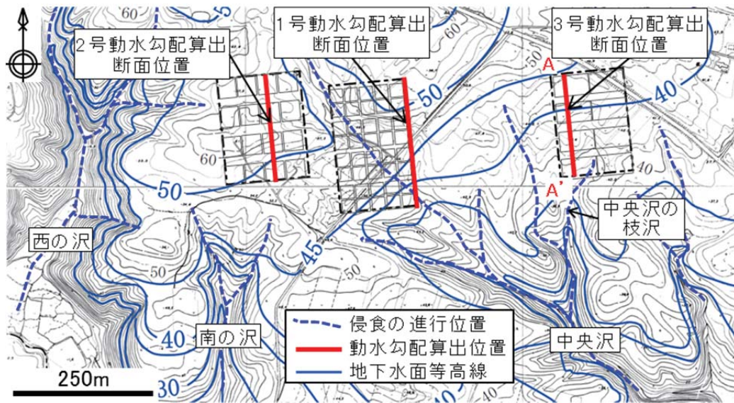
第 20 図 動水勾配の算出位置
