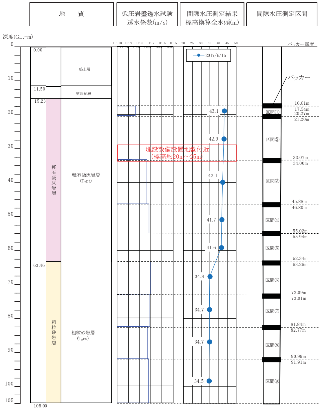
第 18 図 埋設設備設置地盤付近の間隙水圧測定孔における間隙水圧測定結果 (1/9)
