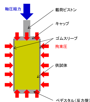
b. 三軸圧縮試験の応力状態
