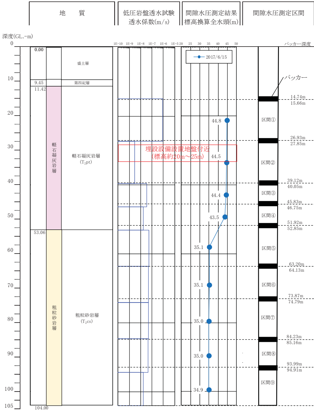
第 18 図 埋設設備設置地盤付近の間隙水圧測定孔における間隙水圧測定結果 (2/9)
