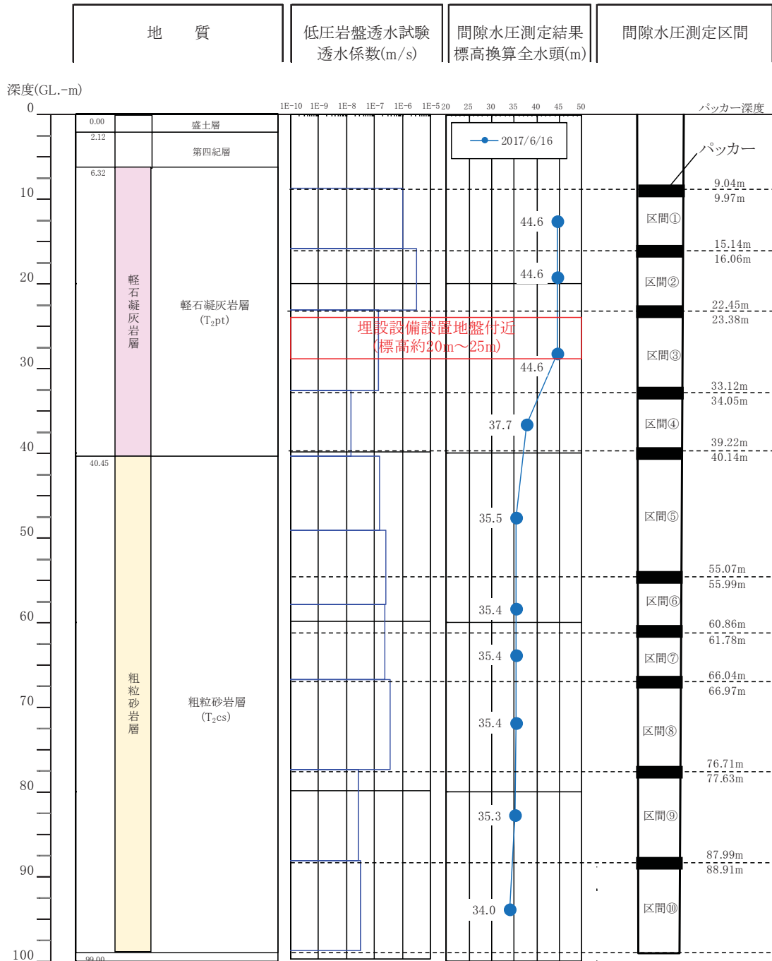
第 18 図 埋設設備設置地盤付近の間隙水圧測定孔における間隙水圧測定結果 (3/9)
