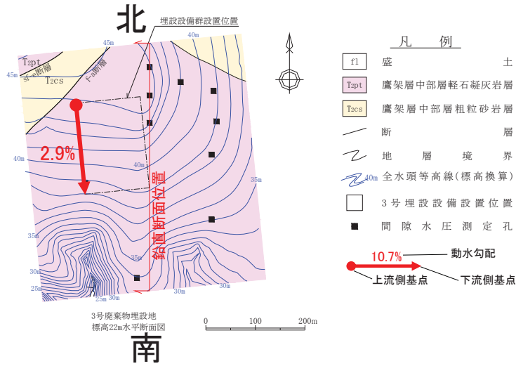
標高+22m 水平断面
