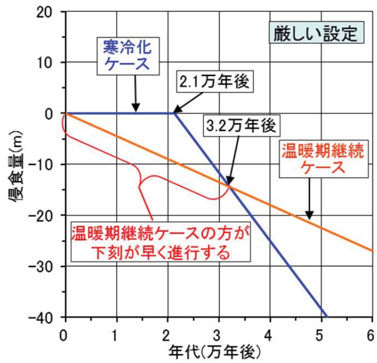
第 24 図 侵食量の関係(厳しい設定の例)
