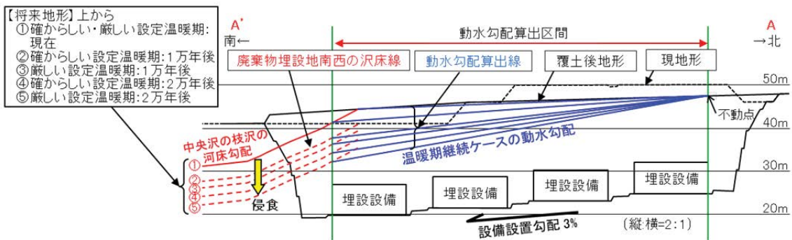
第 21 図 3号廃棄物埋設地南北断面における将来の地形変化と動水勾配の算出*1
