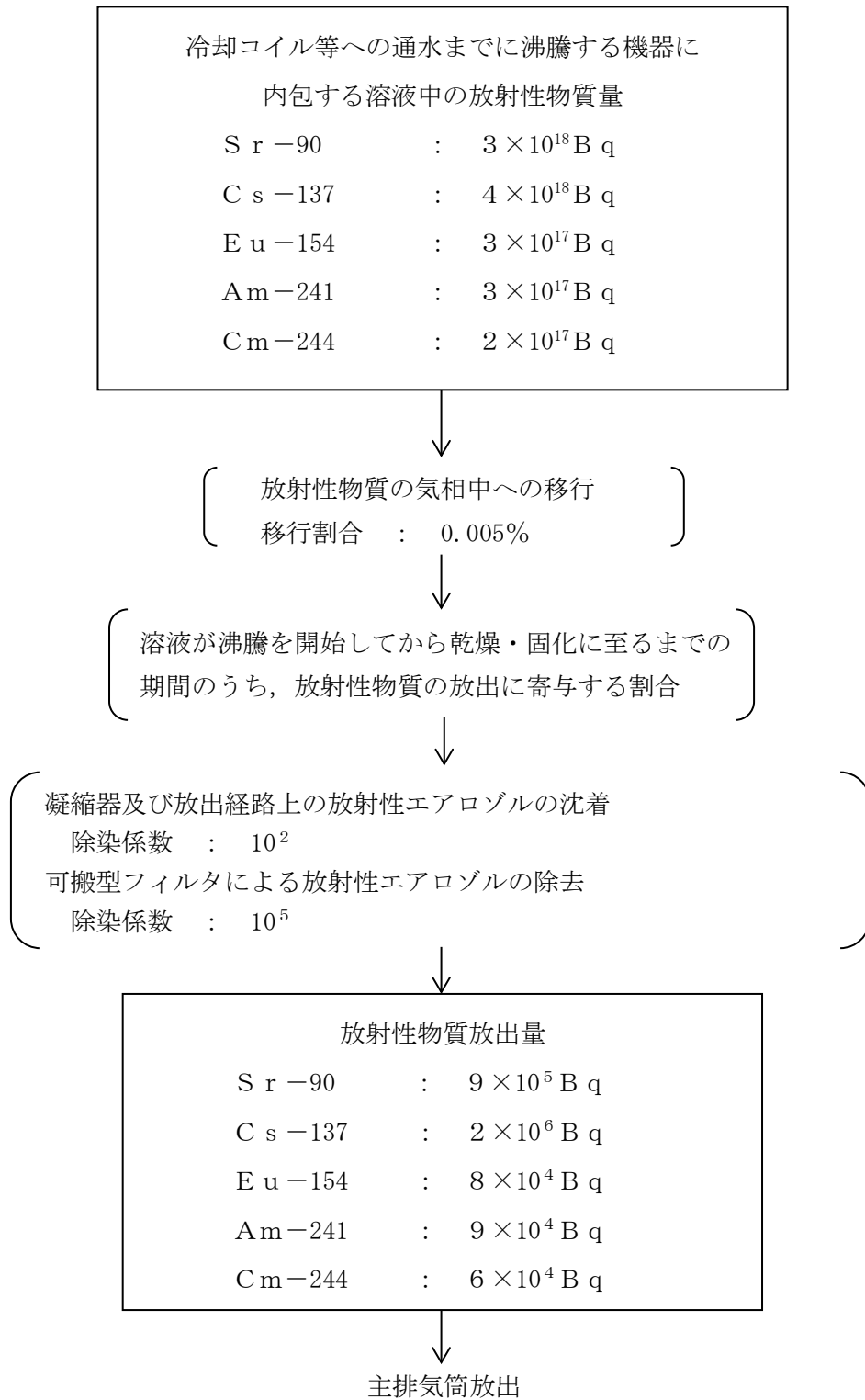
第 7.2.2-19 図 放射性物質の大気放出過程 (高レベル廃液ガラス固化建屋)
