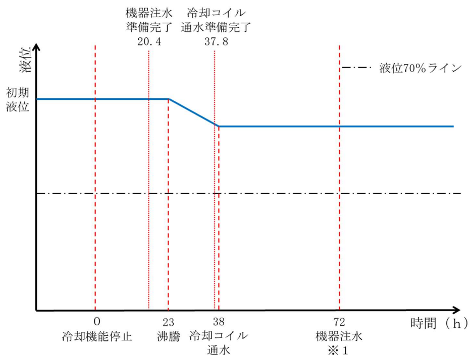
第 7.2.2-5 図 冷却コイル等通水及び機器注水実施時の高レベル廃液混合槽に内包する溶液の温度及び液位傾向
