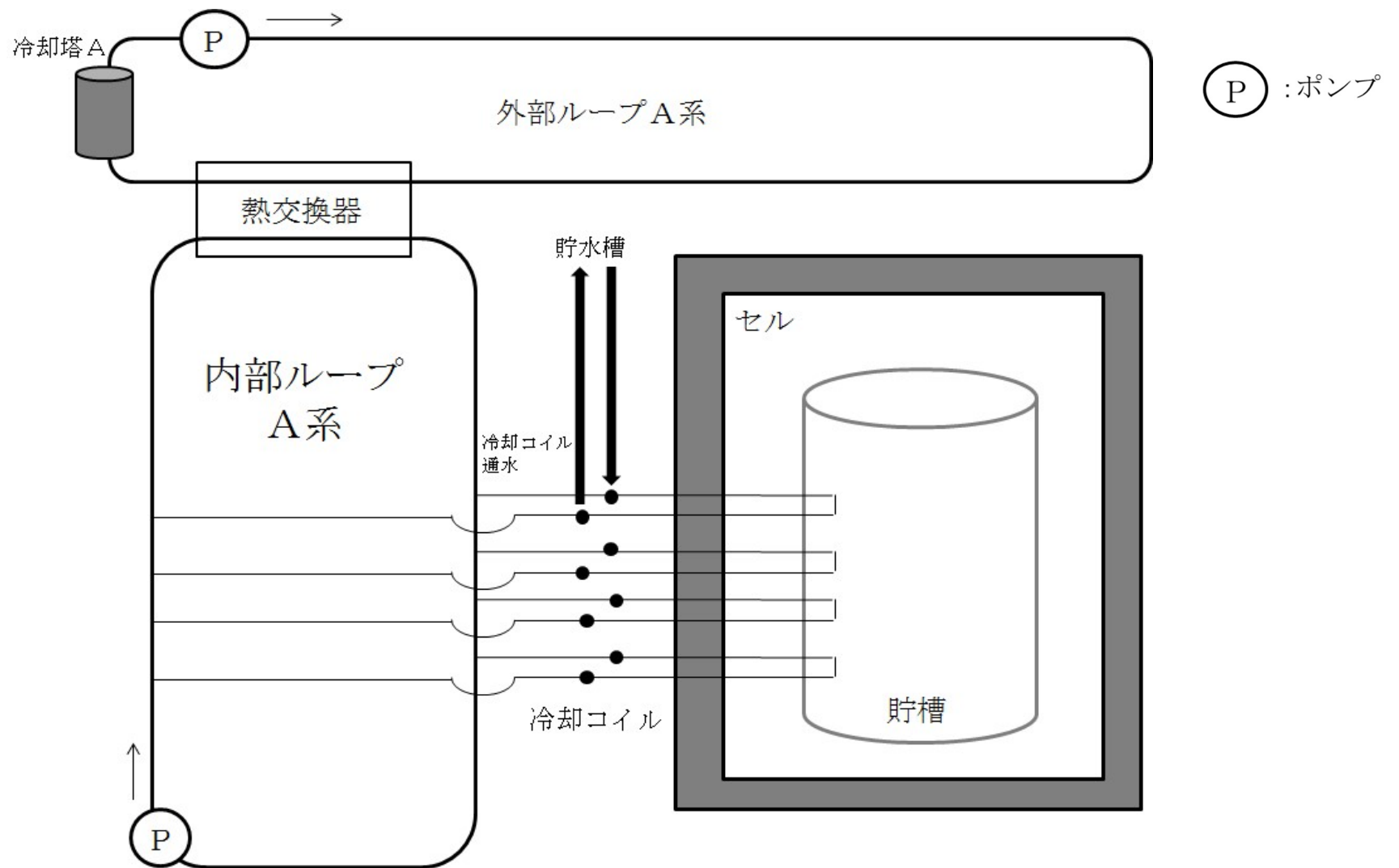
第 7 - 2 図 冷却コイル等への通水の概要図
