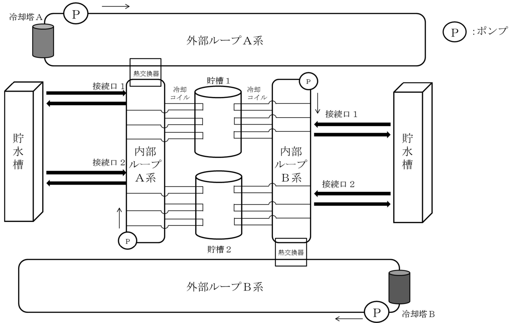
第 7 - 1 図 内部ループへの通水の概要図
