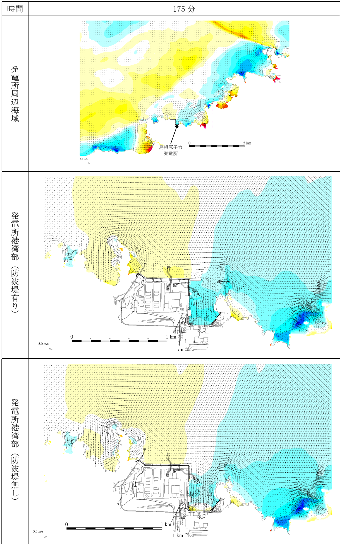
第 2.5-13-1 図(151) 基準津波 1 の水位変動・流向ベクトル
