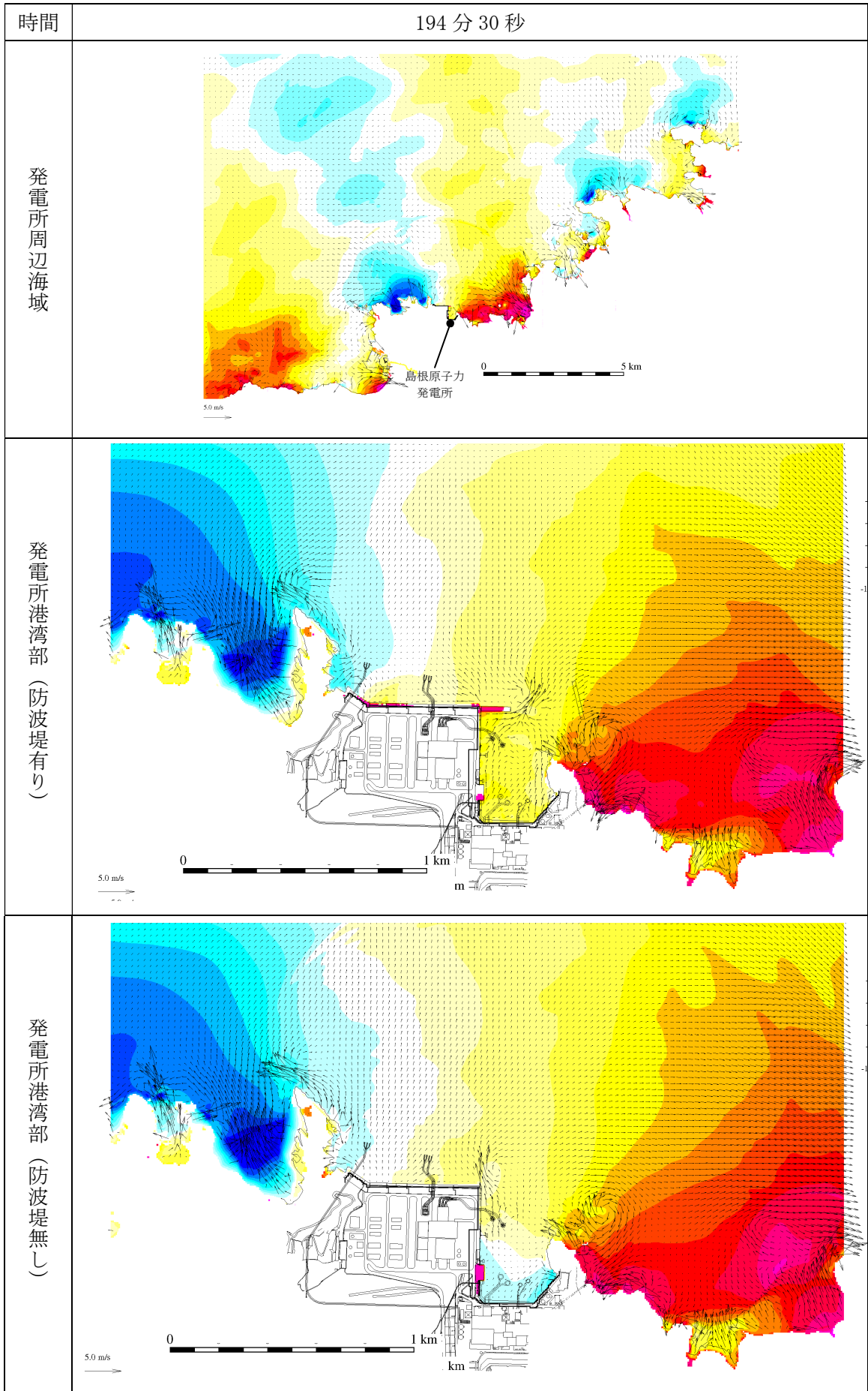
第 2.5-13-1 図(190) 基準津波 1 の水位変動・流向ベクトル
