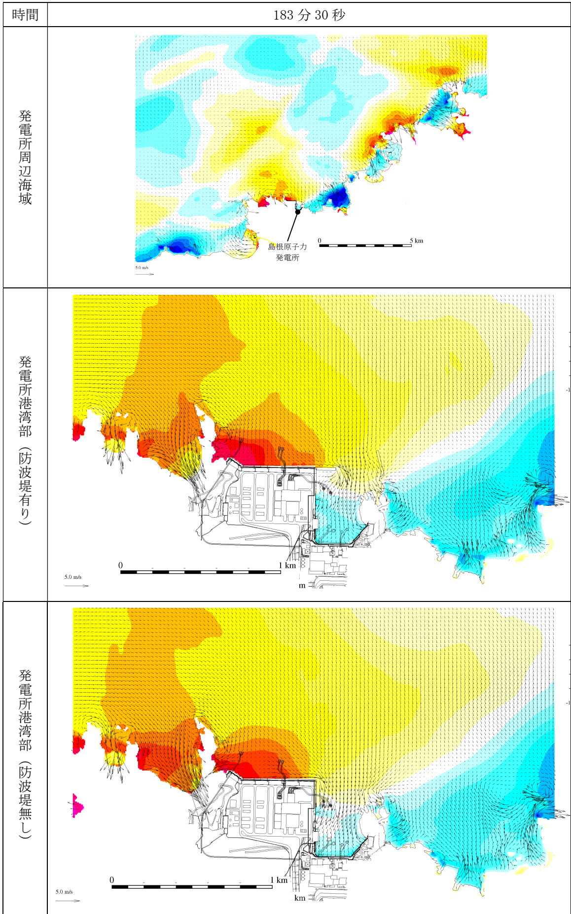
第 2.5-13-1 図(168) 基準津波 1 の水位変動・流向ベクトル
