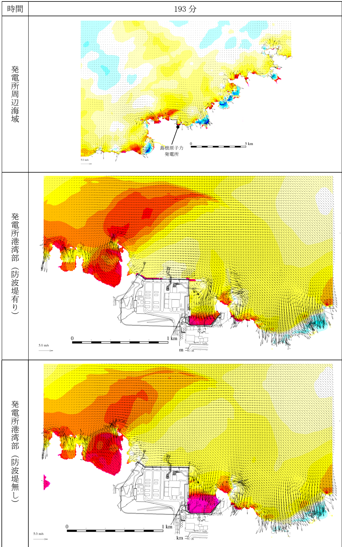
第 2.5-13-1 図(187) 基準津波 1 の水位変動・流向ベクトル
