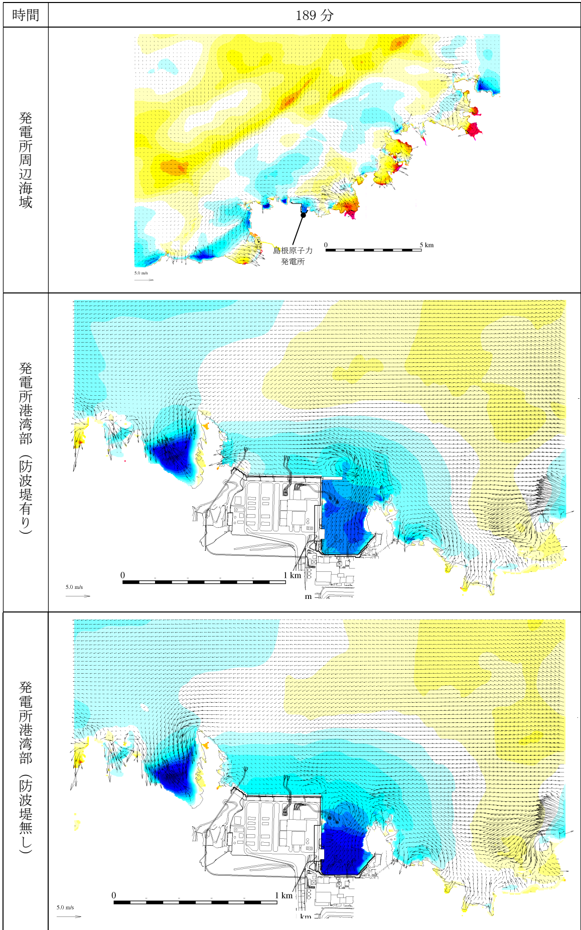
第 2.5-13-1 図(179) 基準津波 1 の水位変動・流向ベクトル
