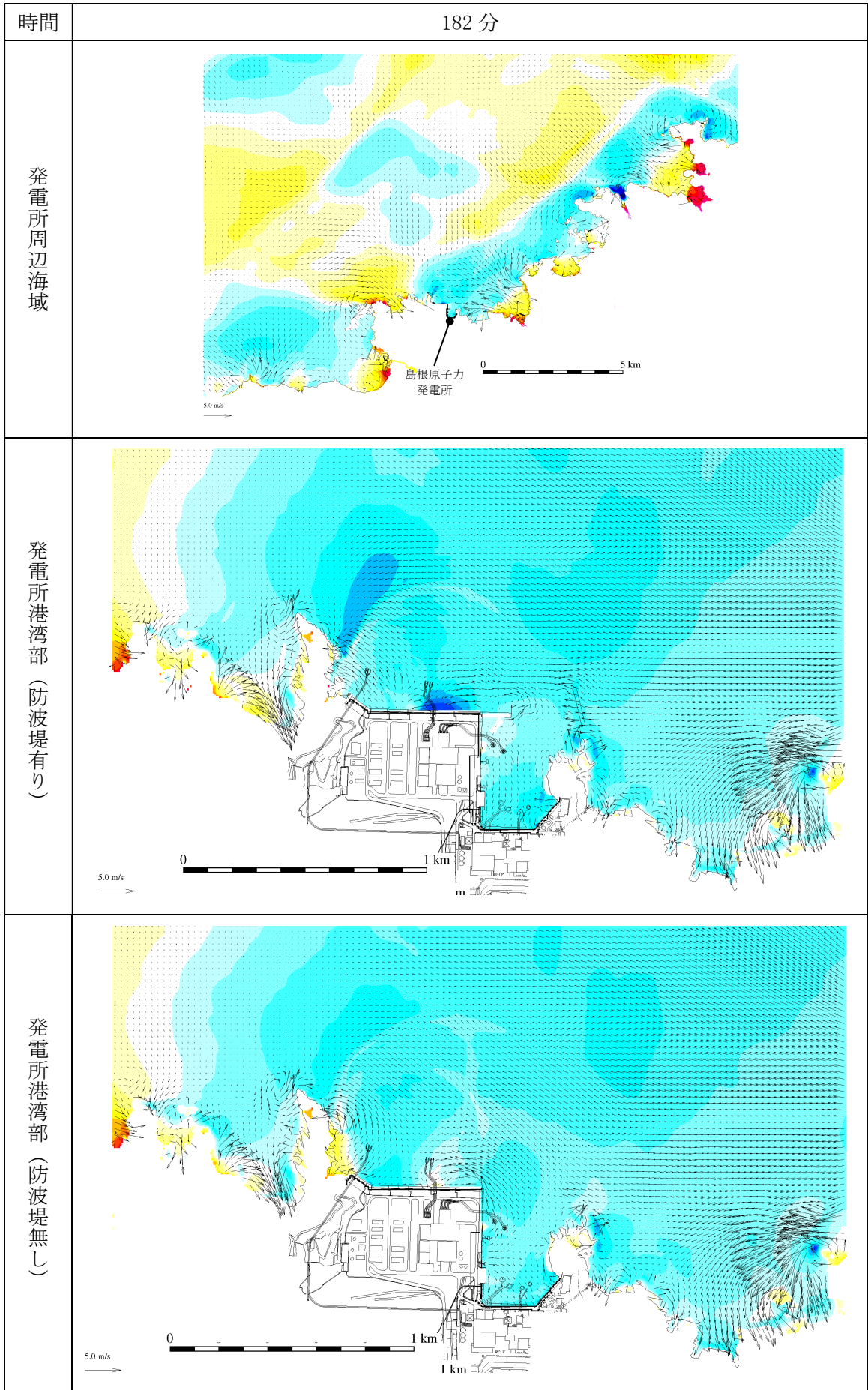
第 2.5-13-1 図(165) 基準津波 1 の水位変動・流向ベクトル
