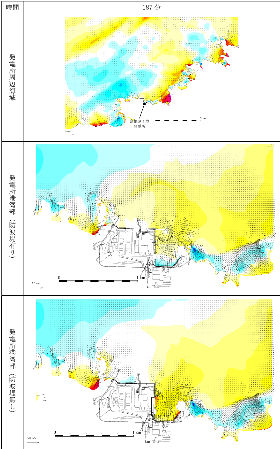
第 2.5-13-1 図(175) 基準津波 1 の水位変動・流向ベクトル
