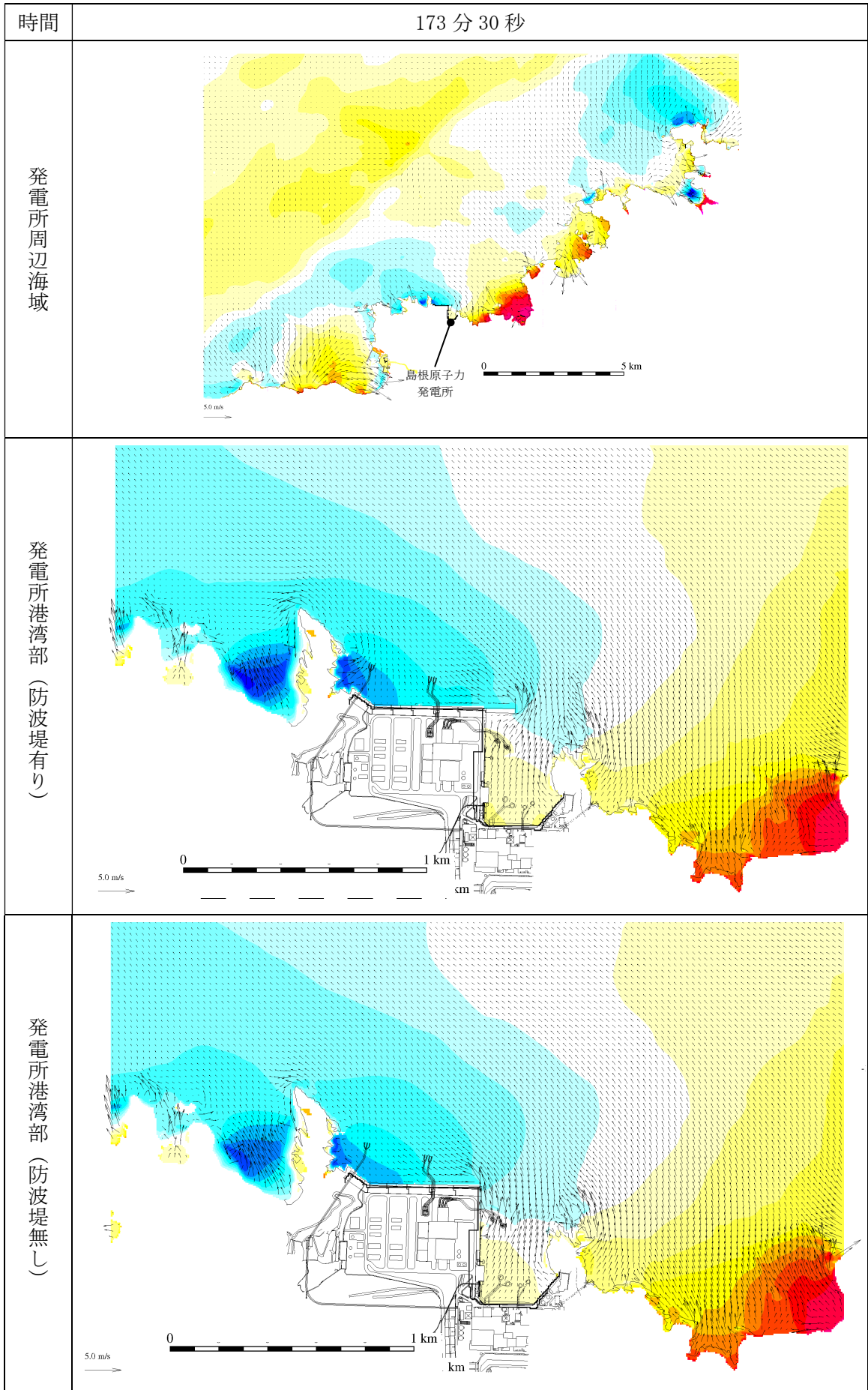
第 2.5-13-1 図(148) 基準津波 1 の水位変動・流向ベクトル
