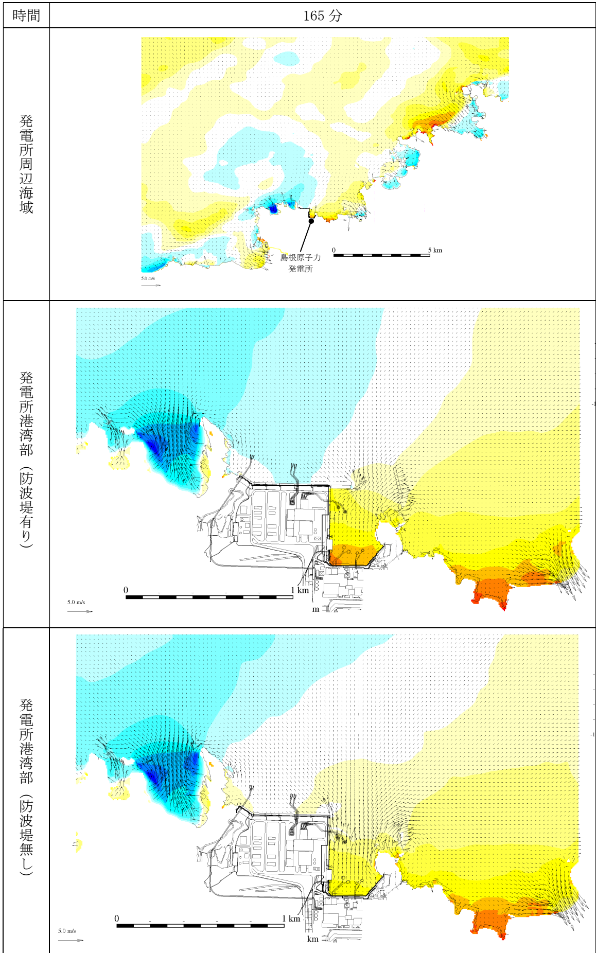
第 2.5-13-1 図(131) 基準津波 1 の水位変動・流向ベクトル
