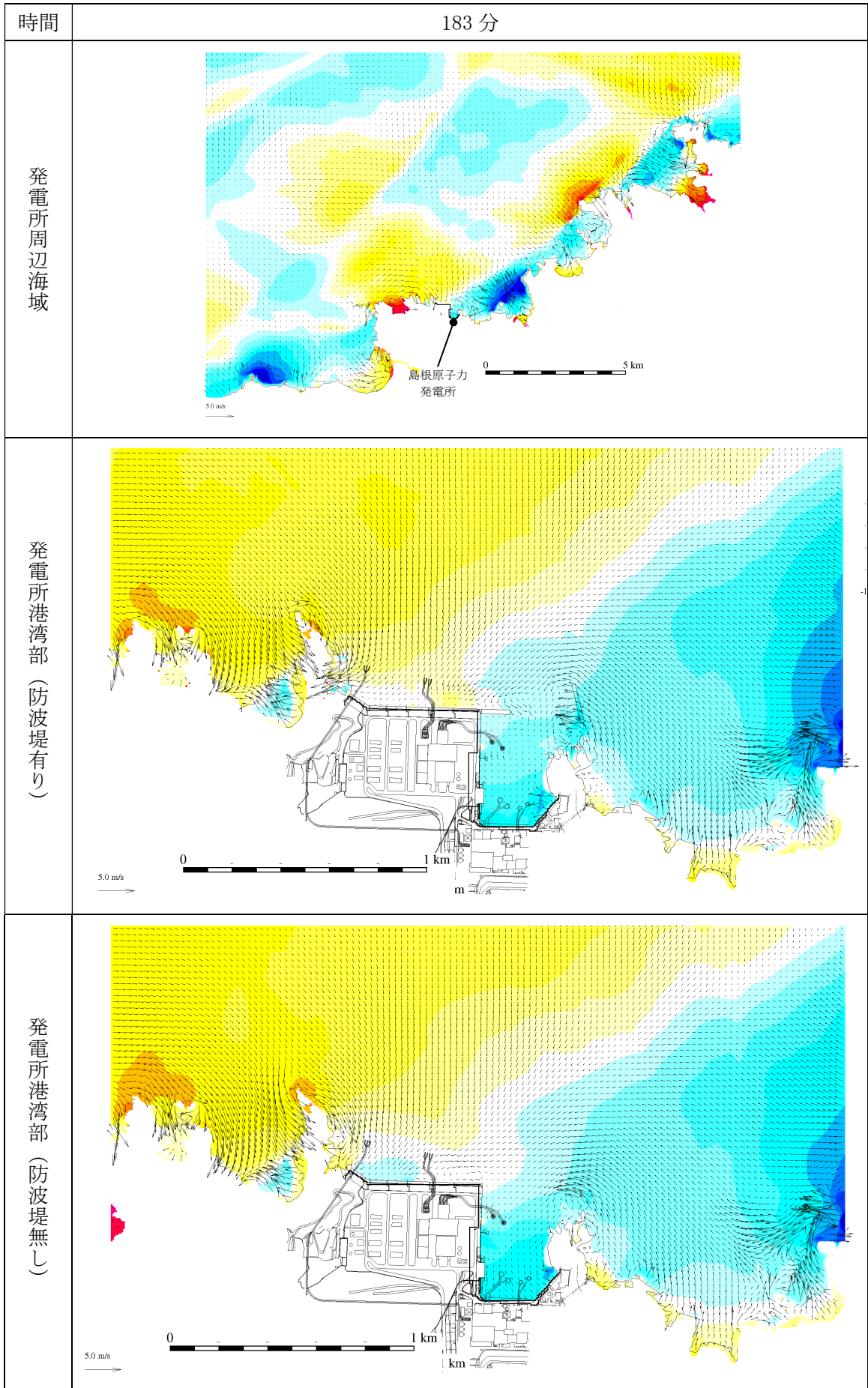
第 2.5-13-1 図(167) 基準津波 1 の水位変動・流向ベクトル
