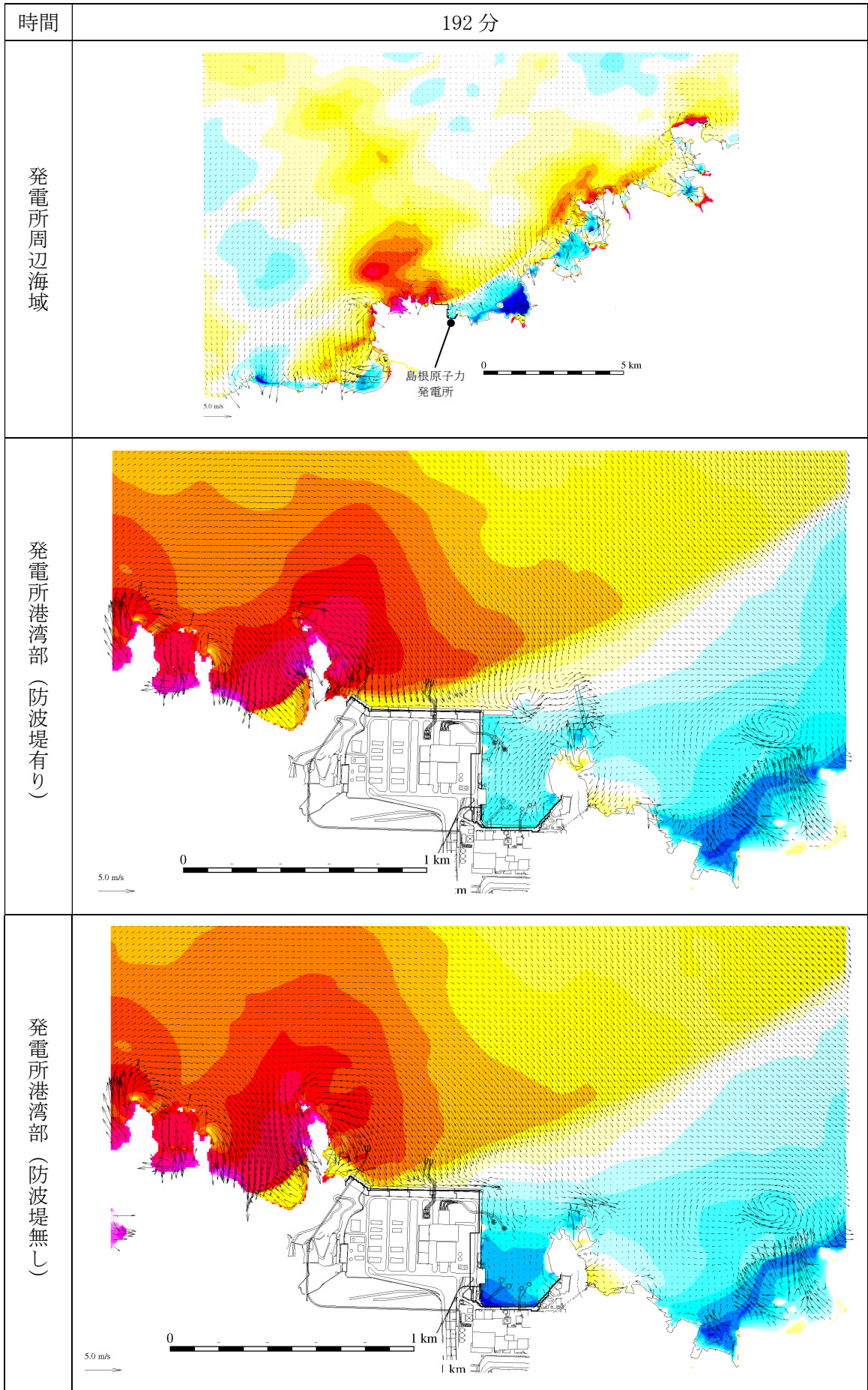
第 2.5-13-1 図(185) 基準津波 1 の水位変動・流向ベクトル
