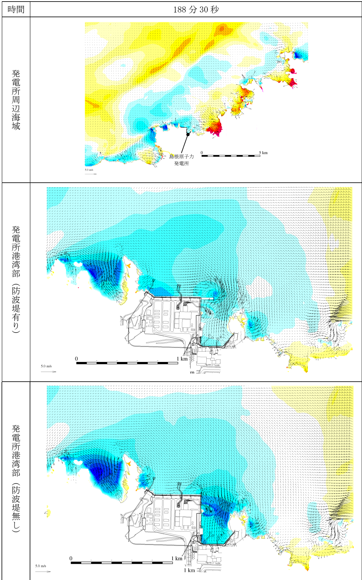
第 2.5-13-1 図(178) 基準津波 1 の水位変動・流向ベクトル
