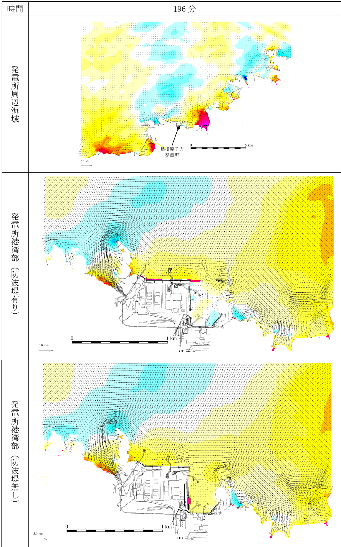
第 2.5-13-1 図(193) 基準津波 1 の水位変動・流向ベクトル
