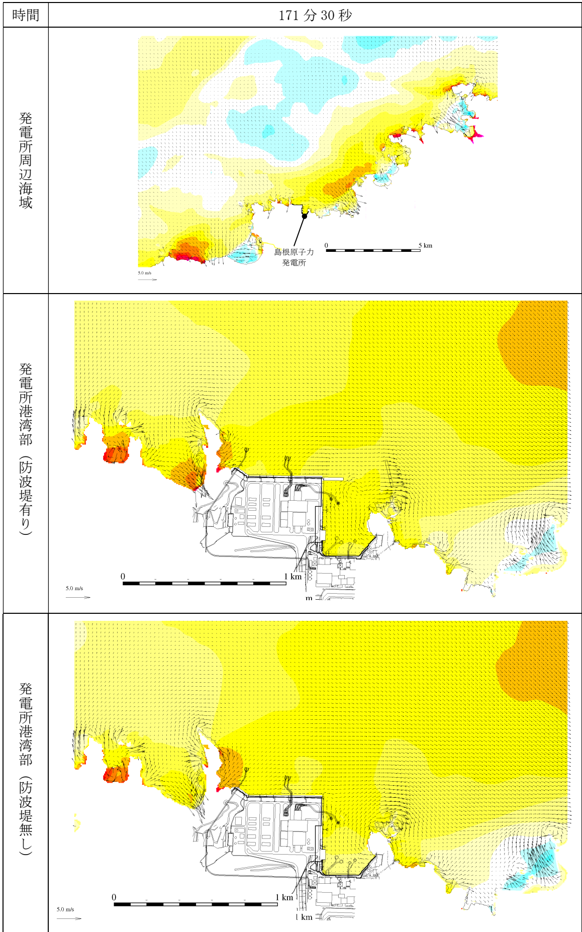
第 2.5-13-1 図(144) 基準津波 1 の水位変動・流向ベクトル
