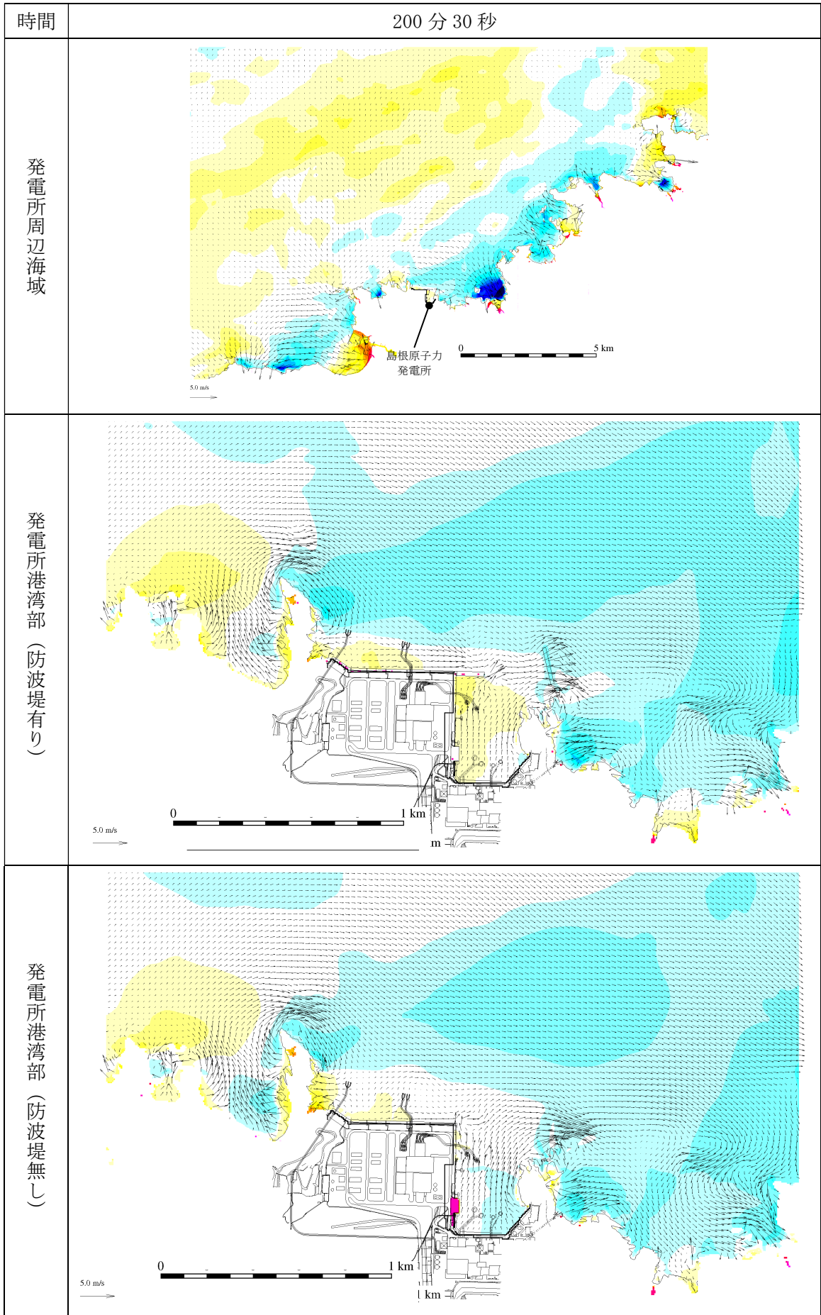
第 2.5-13-1 図(202) 基準津波 1 の水位変動・流向ベクトル
