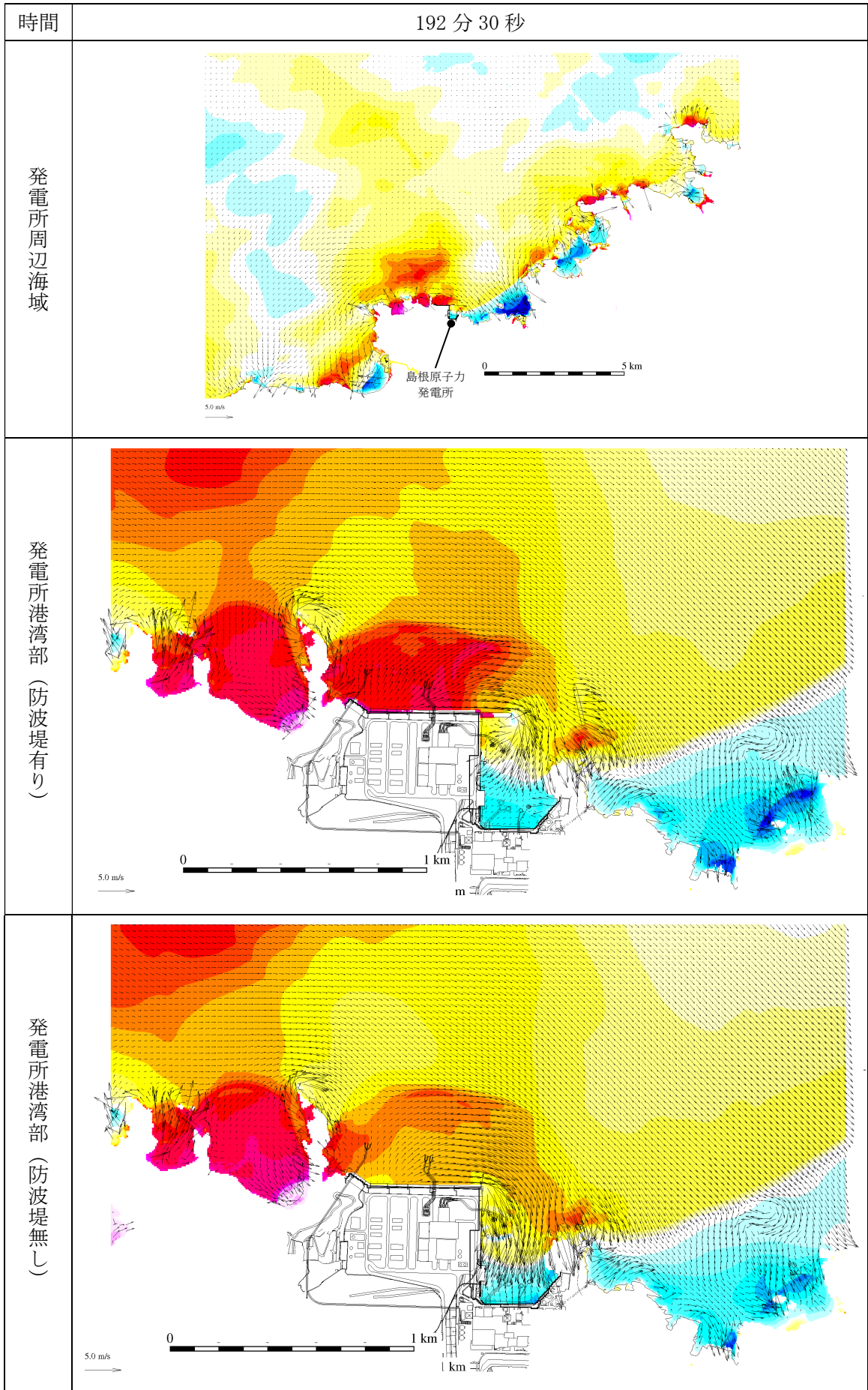
第 2.5-13-1 図(186) 基準津波 1 の水位変動・流向ベクトル
