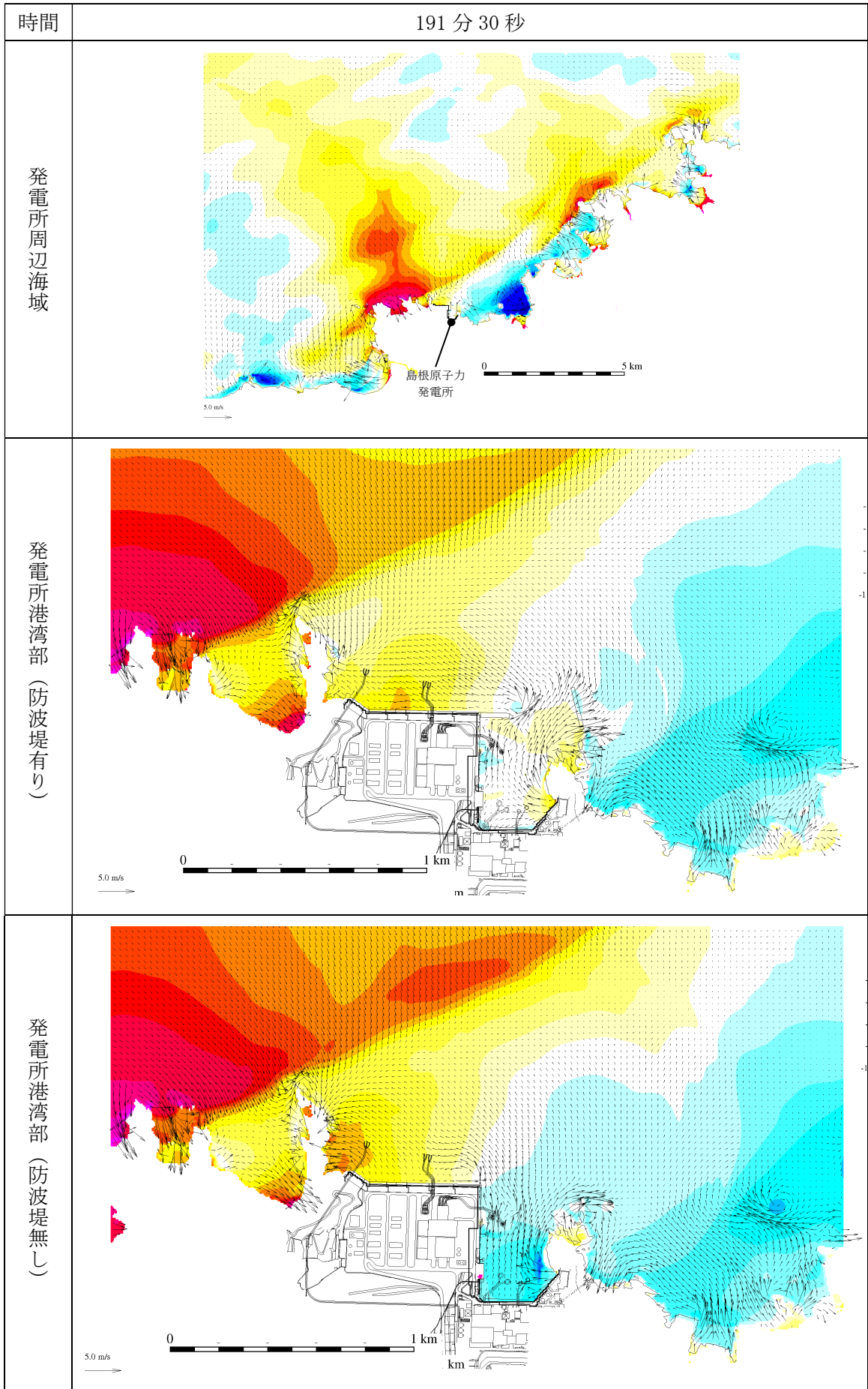
第 2.5-13-1 図(184) 基準津波 1 の水位変動・流向ベクトル
