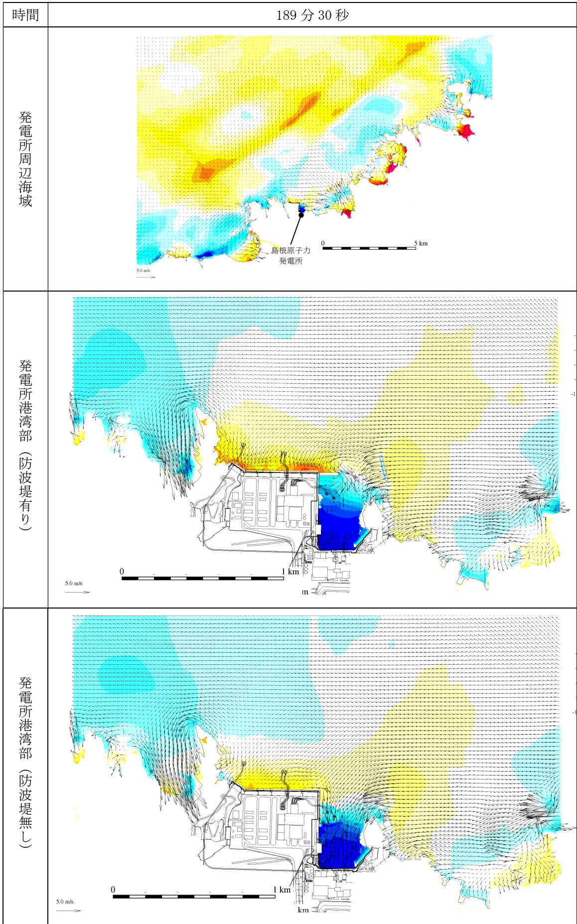
第 2.5-13-1 図(180) 基準津波 1 の水位変動・流向ベクトル
