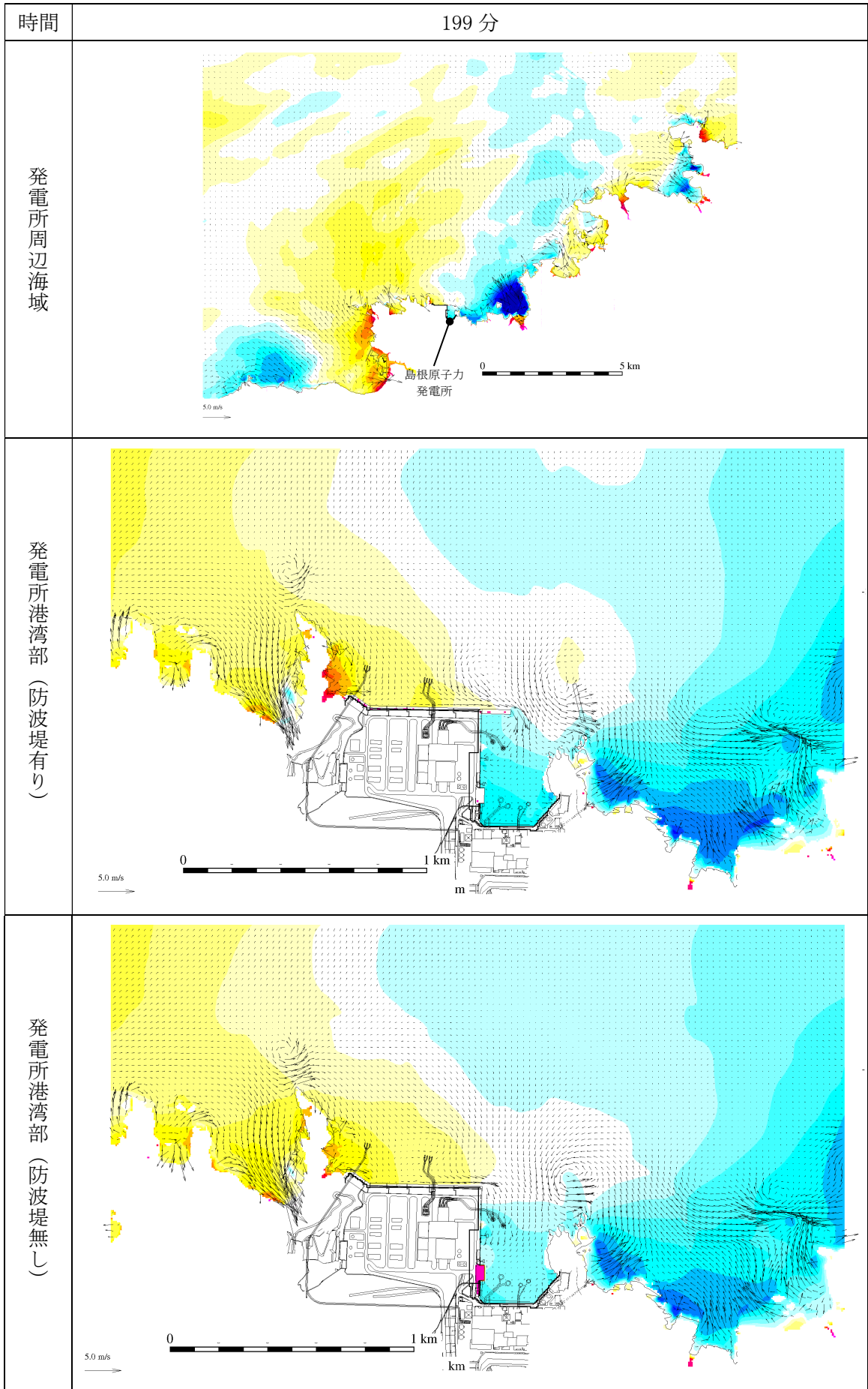
第 2.5-13-1 図(199) 基準津波 1 の水位変動・流向ベクトル
