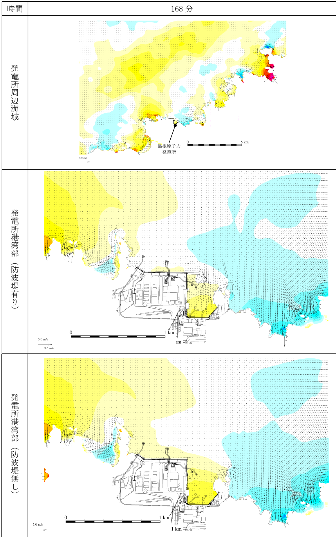
第 2.5-13-1 図(137) 基準津波 1 の水位変動・流向ベクトル
