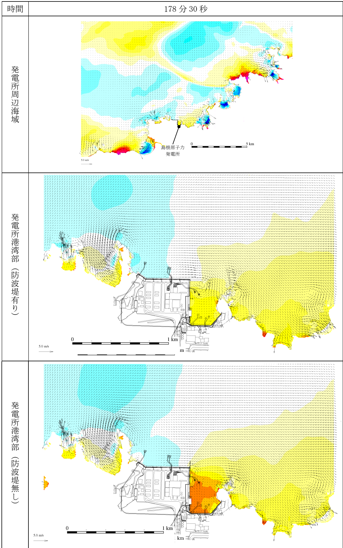
第 2.5-13-1 図(158) 基準津波 1 の水位変動・流向ベクトル
