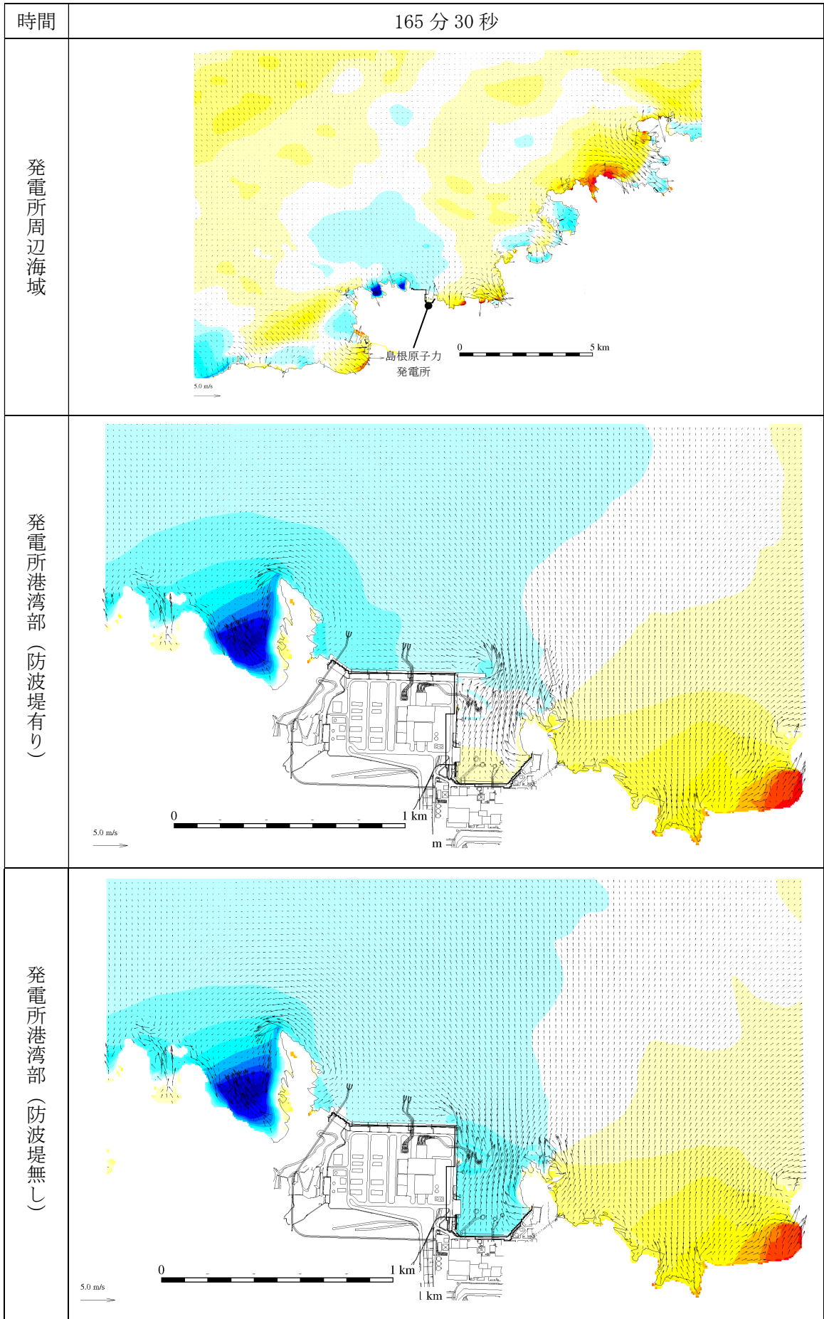
第 2.5-13-1 図(132) 基準津波 1 の水位変動・流向ベクトル
