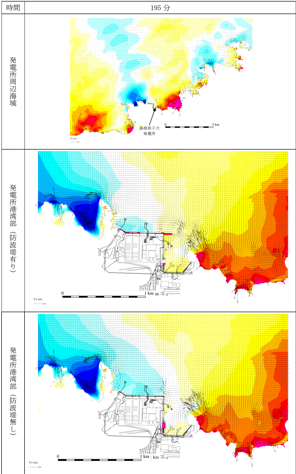
第 2.5-13-1 図(191) 基準津波 1 の水位変動・流向ベクトル
