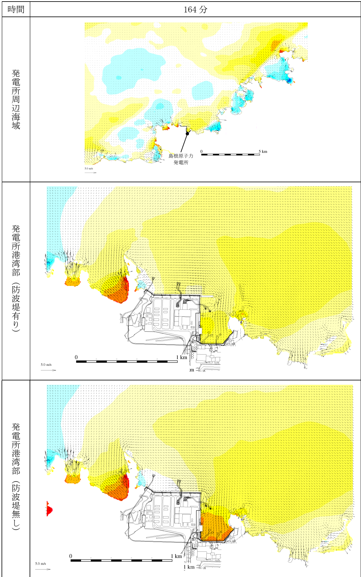
第 2.5-13-1 図(129) 基準津波 1 の水位変動・流向ベクトル
