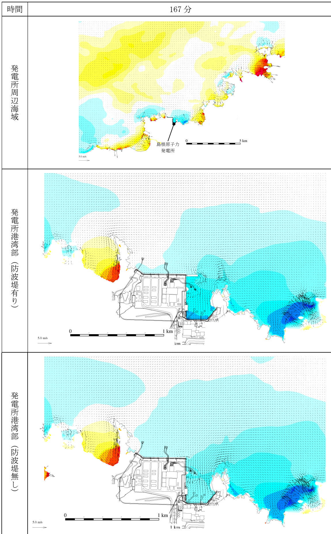
第 2.5-13-1 図(135) 基準津波 1 の水位変動・流向ベクトル
