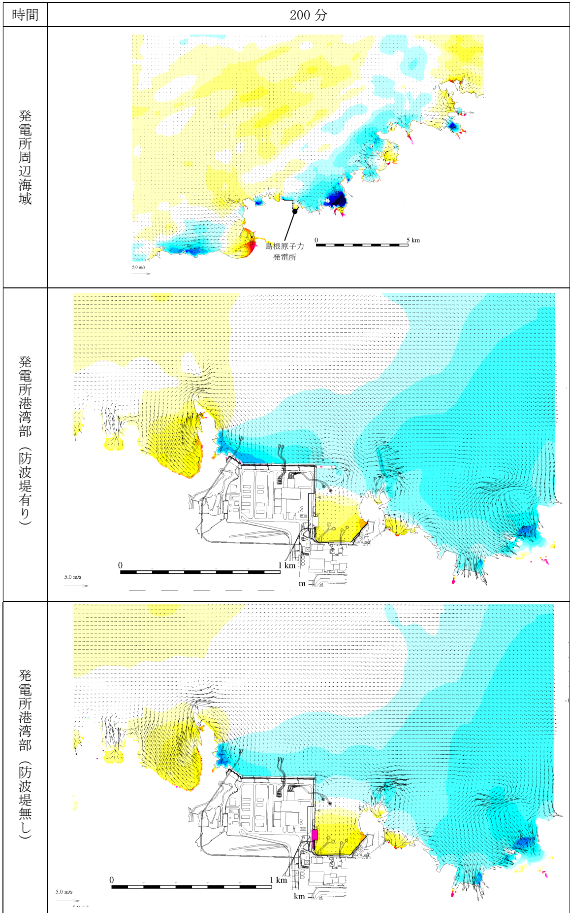
第 2.5-13-1 図(201) 基準津波 1 の水位変動・流向ベクトル
