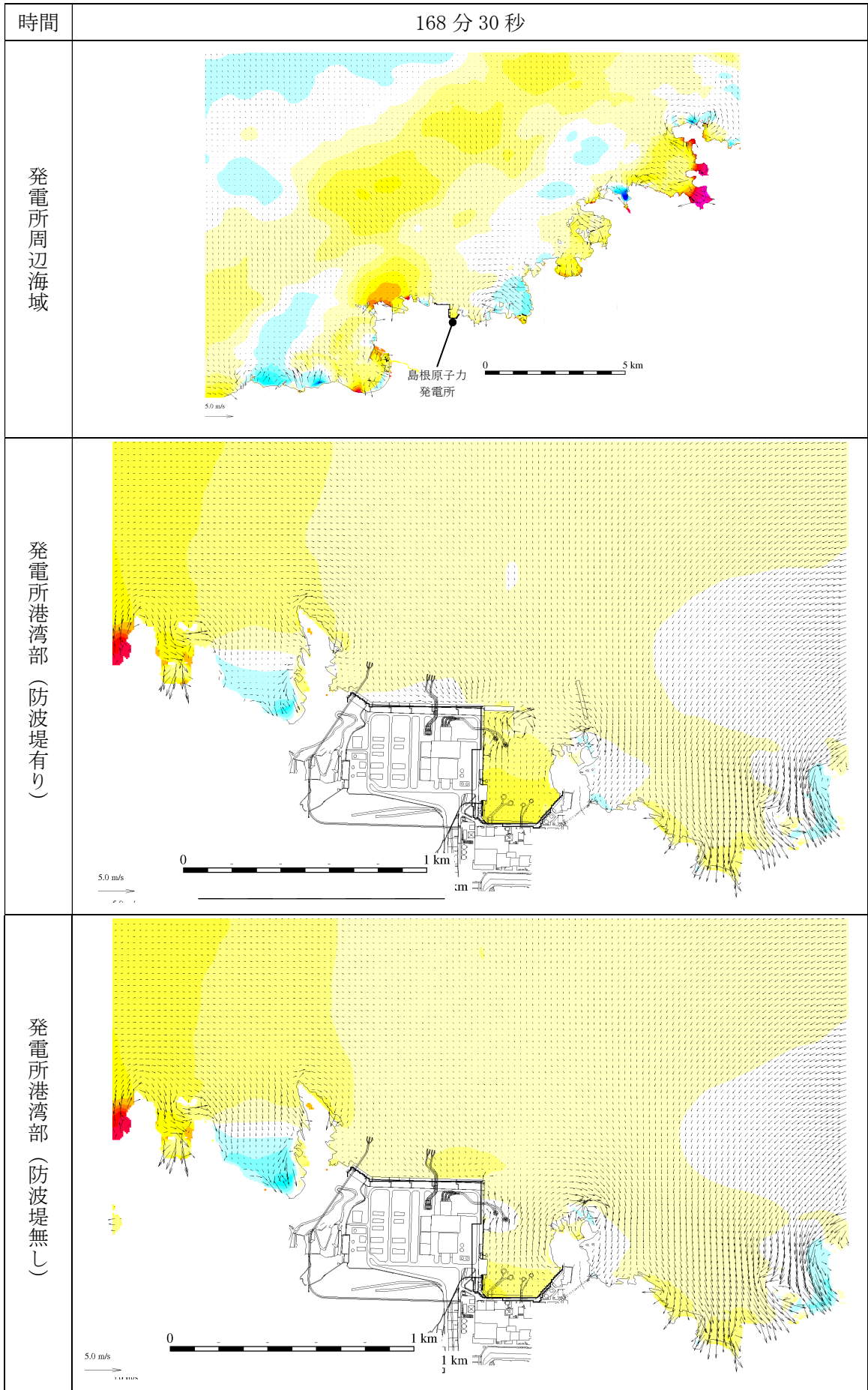
第 2.5-13-1 図(138) 基準津波 1 の水位変動・流向ベクトル
