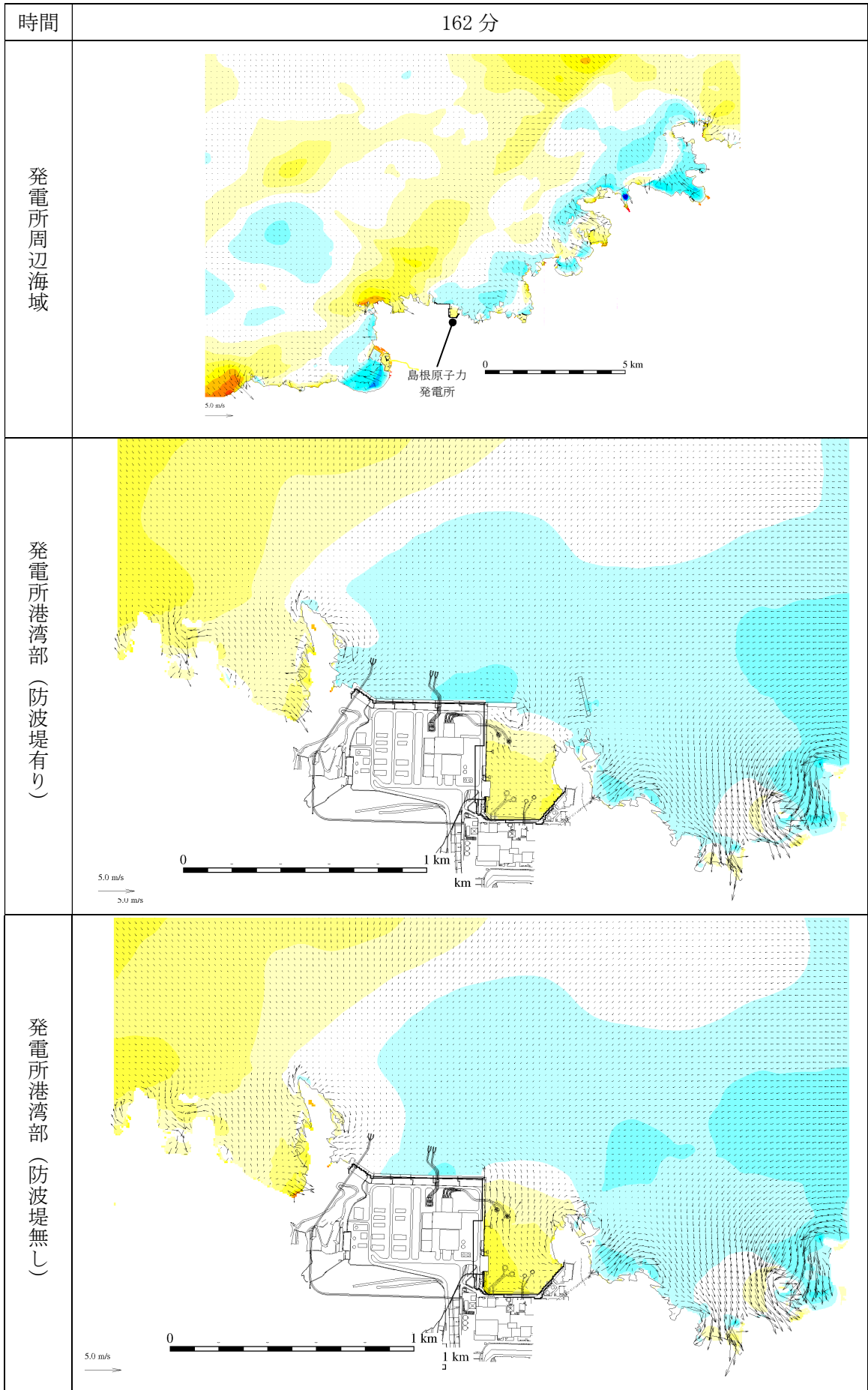
第 2.5-13-1 図(125) 基準津波 1 の水位変動・流向ベクトル
