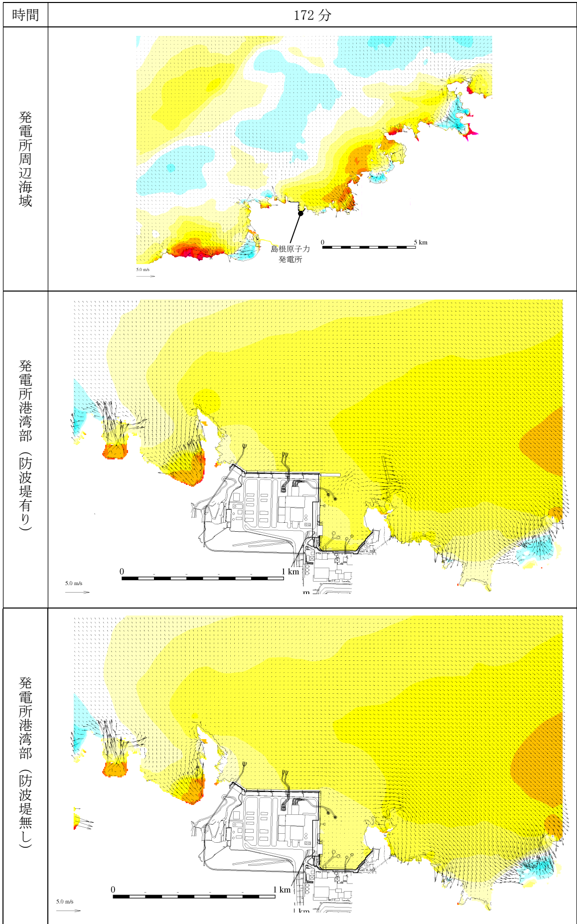
第 2.5-13-1 図(145) 基準津波 1 の水位変動・流向ベクトル
