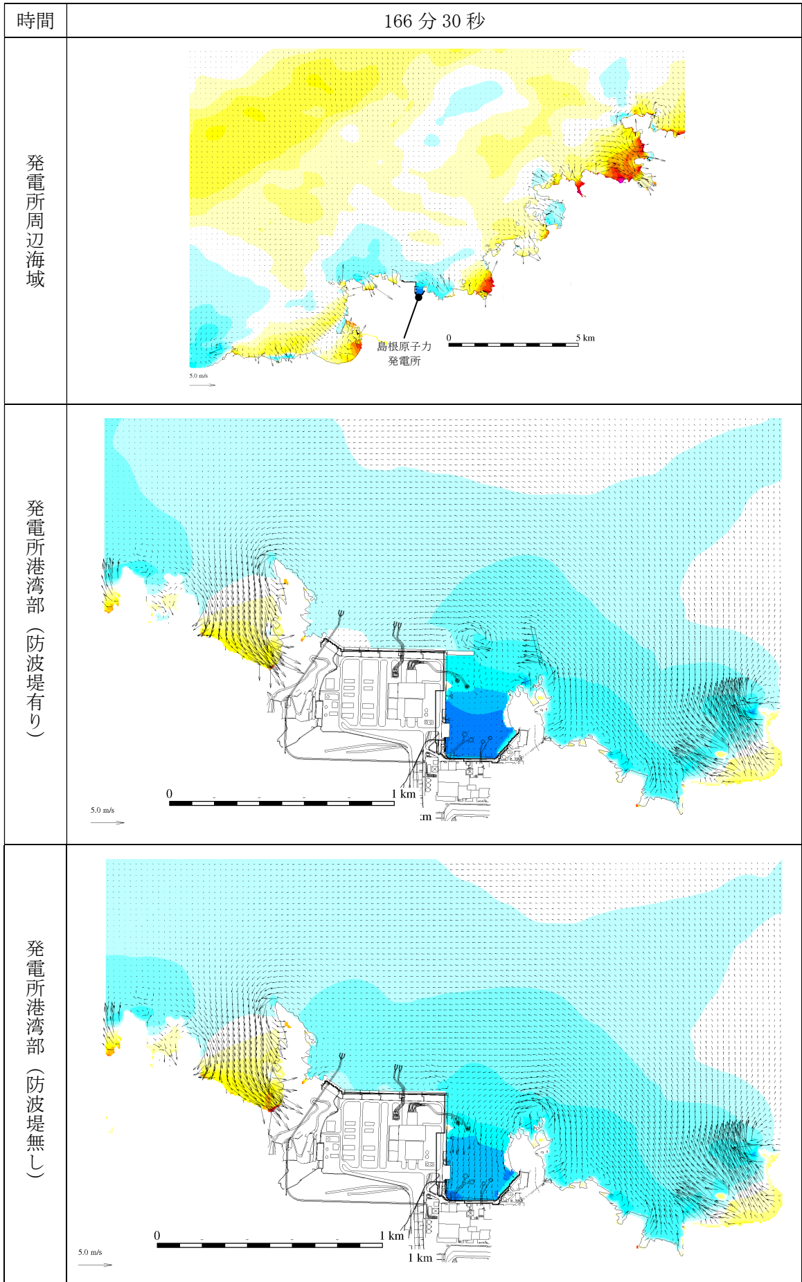
第 2.5-13-1 図(134) 基準津波 1 の水位変動・流向ベクトル
