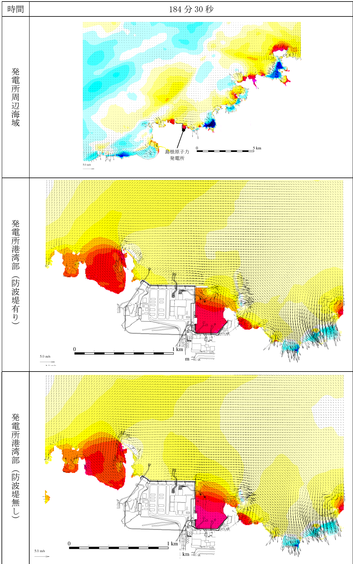
第 2.5-13-1 図(170) 基準津波 1 の水位変動・流向ベクトル
