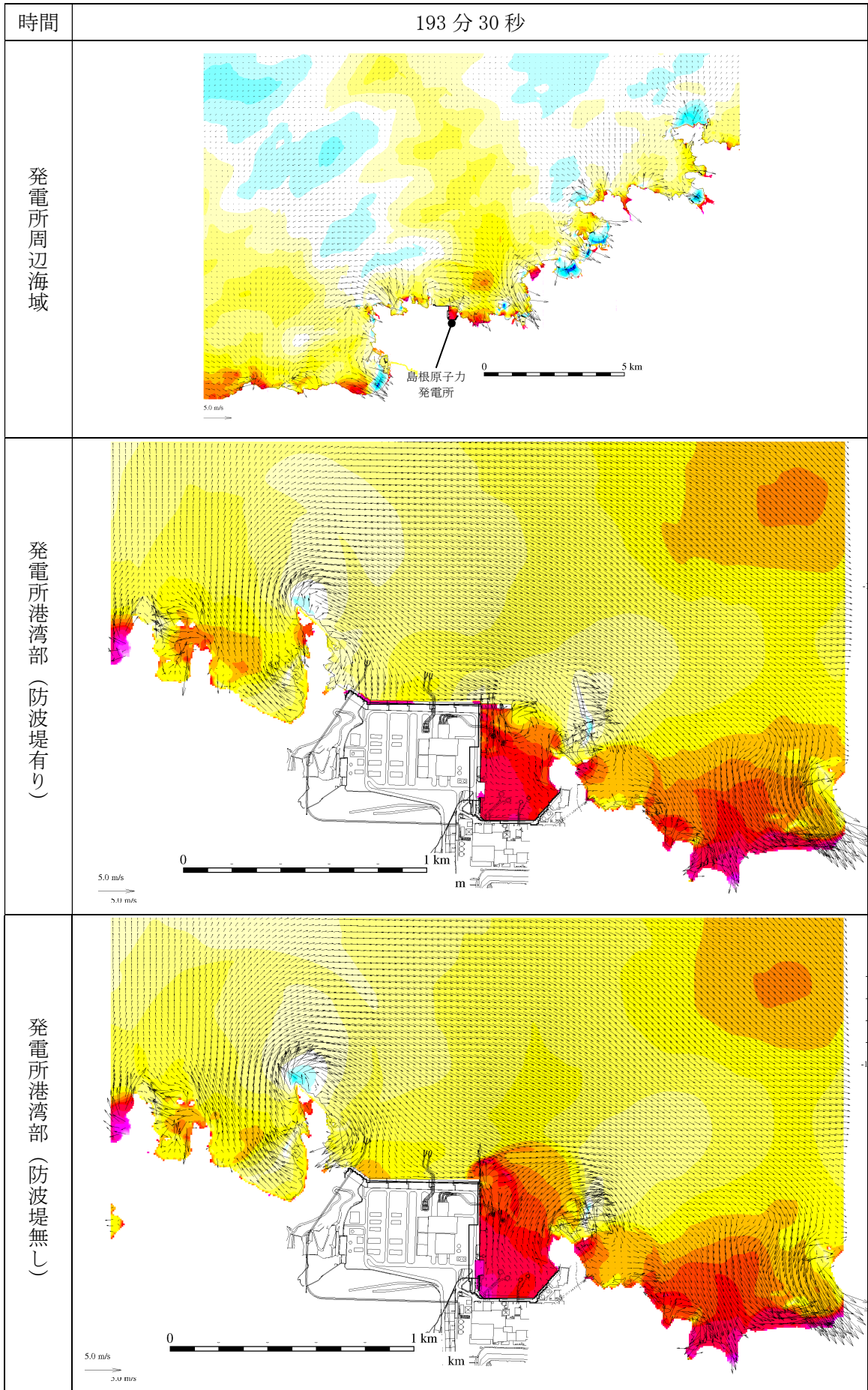
第 2.5-13-1 図(188) 基準津波 1 の水位変動・流向ベクトル
