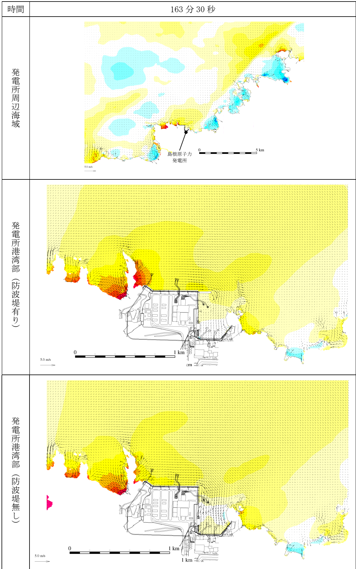
第 2.5-13-1 図(128) 基準津波 1 の水位変動・流向ベクトル
