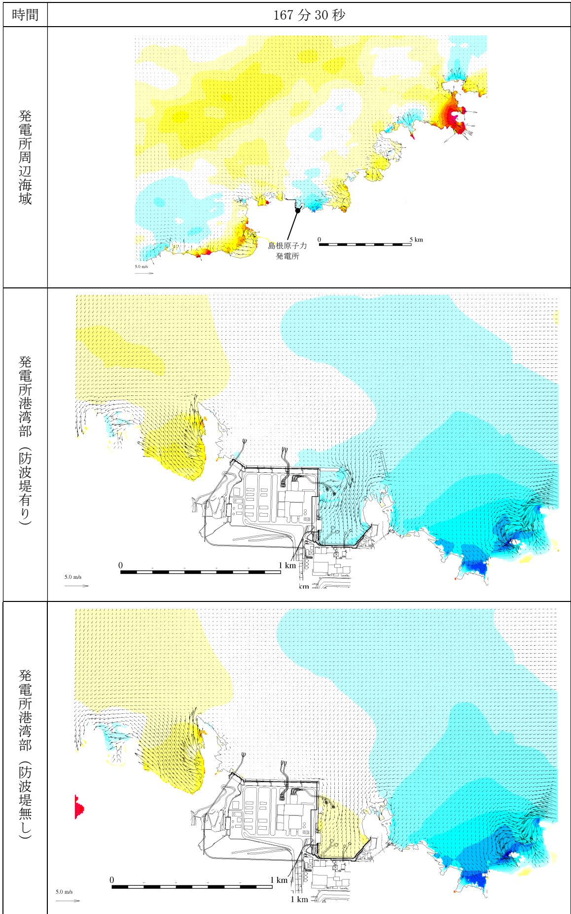
第 2.5-13-1 図(136) 基準津波 1 の水位変動・流向ベクトル
