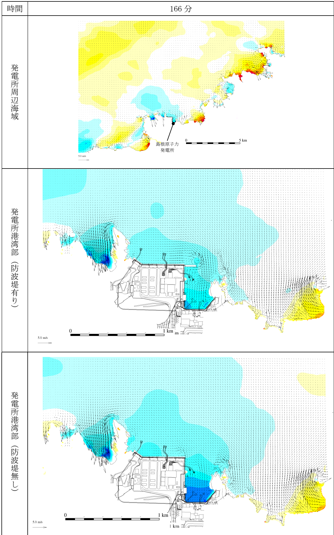
第 2.5-13-1 図(133) 基準津波 1 の水位変動・流向ベクトル
