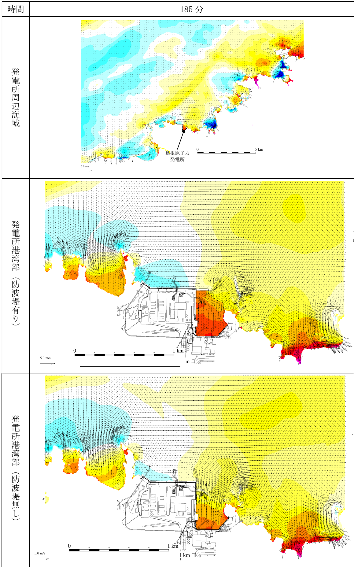
第 2.5-13-1 図(171) 基準津波 1 の水位変動・流向ベクトル
