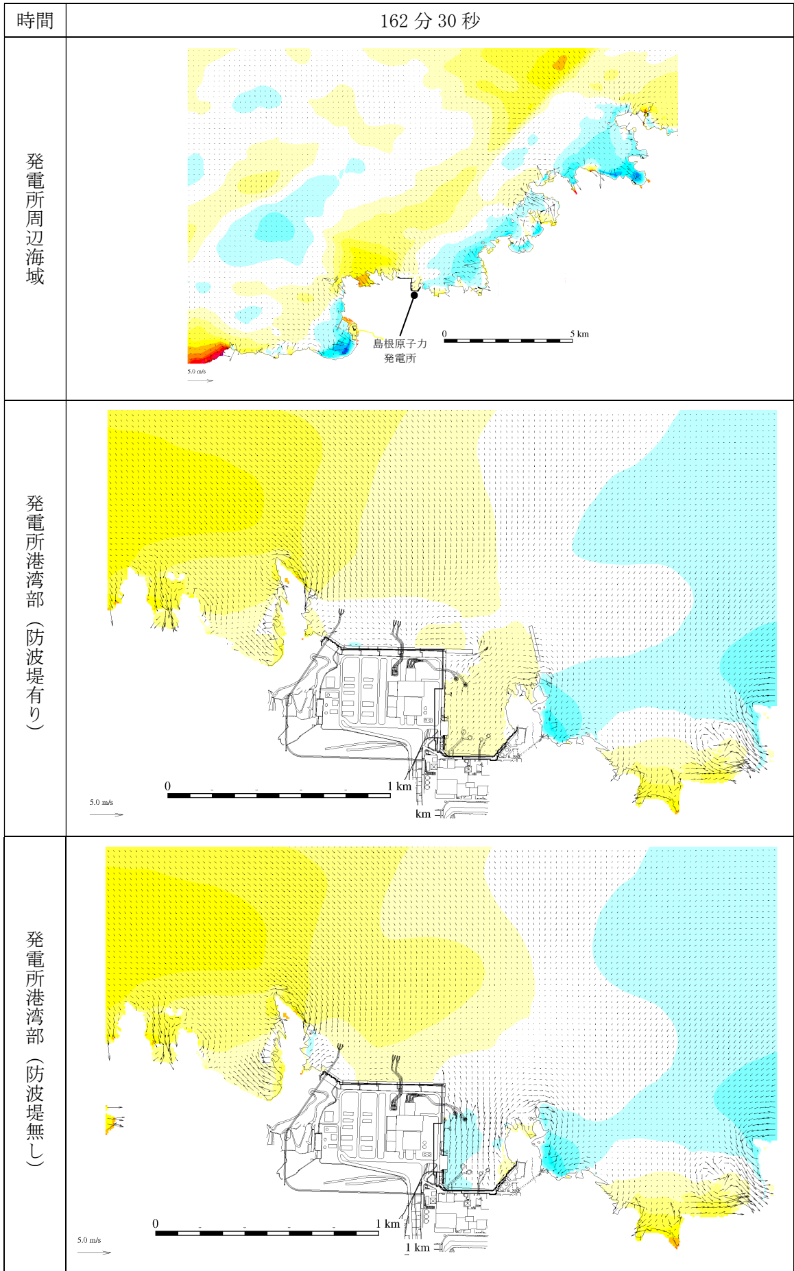
第 2.5-13-1 図(126) 基準津波 1 の水位変動・流向ベクトル
