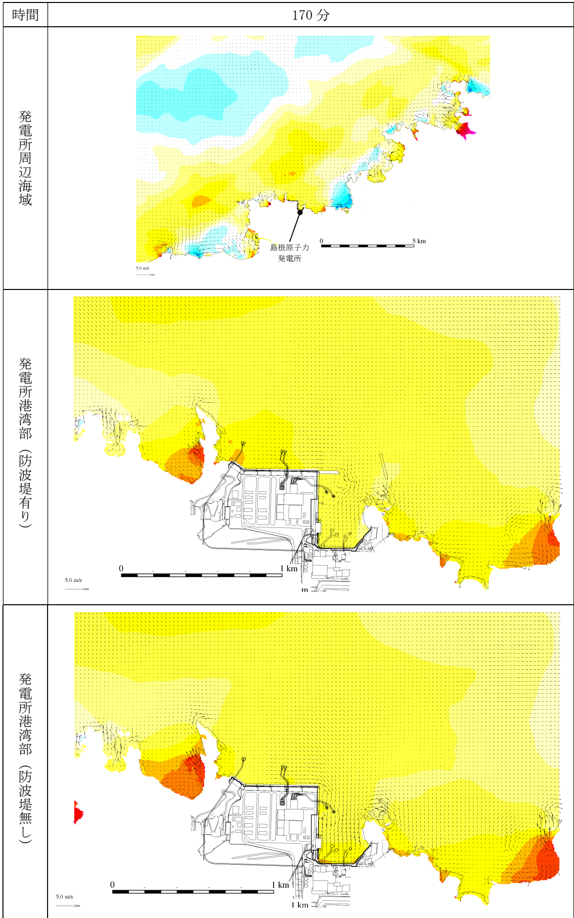
第 2.5-13-1 図(141) 基準津波 1 の水位変動・流向ベクトル
