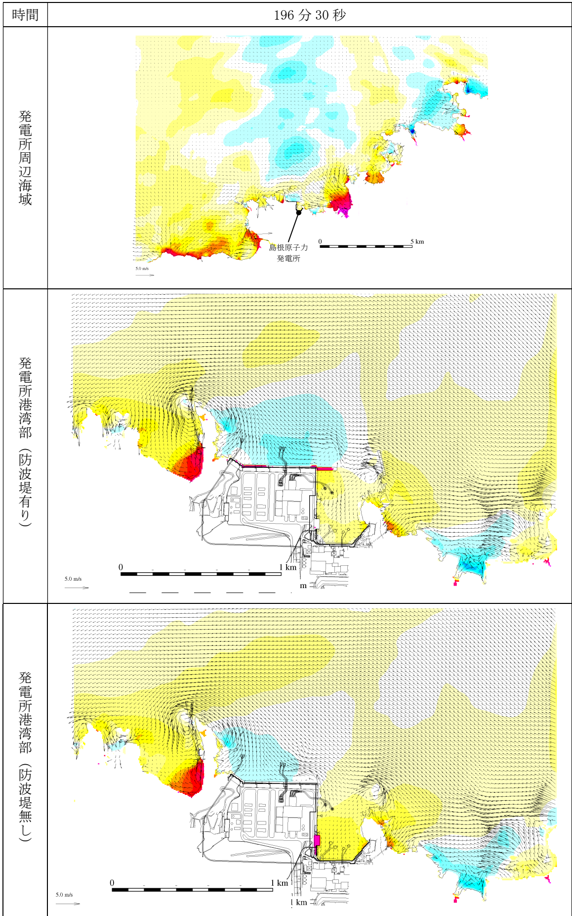
第 2.5-13-1 図(194) 基準津波 1 の水位変動・流向ベクトル
