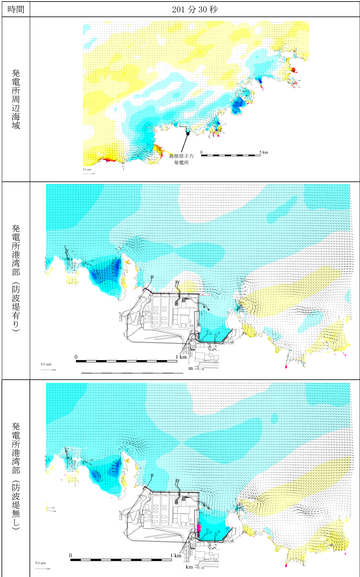
第 2.5-13-1 図(204) 基準津波 1 の水位変動・流向ベクトル
