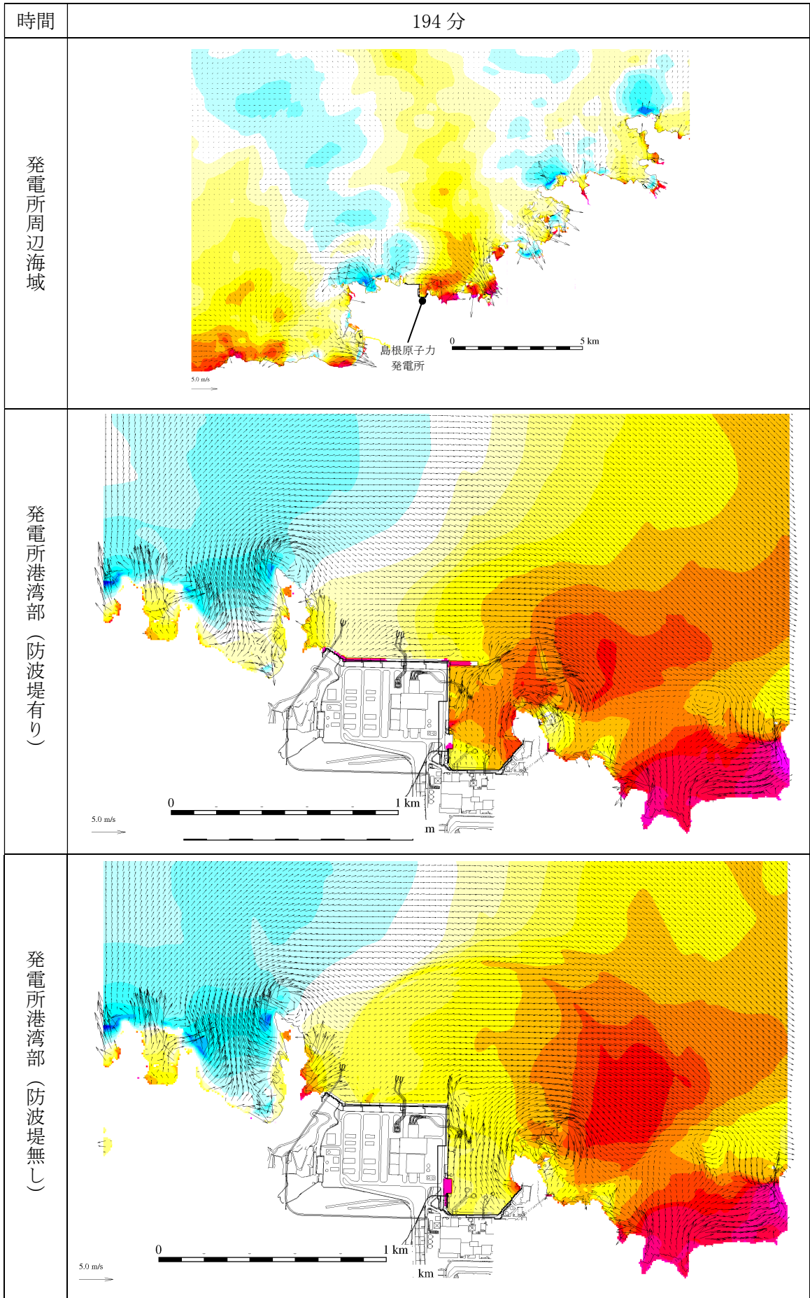
第 2.5-13-1 図(189) 基準津波 1 の水位変動・流向ベクトル
