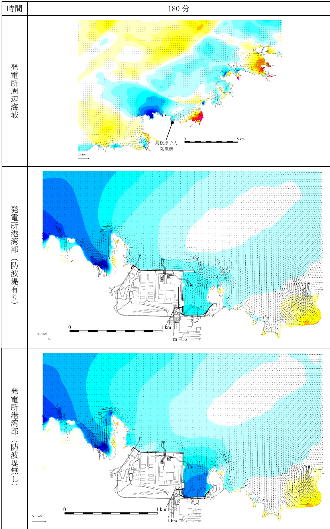
第 2.5-13-1 図(161) 基準津波 1 の水位変動・流向ベクトル
