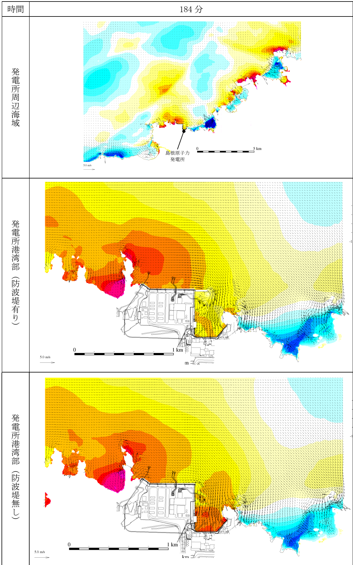
第 2.5-13-1 図(169) 基準津波 1 の水位変動・流向ベクトル
