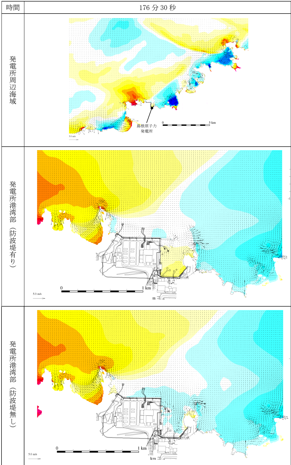
第 2.5-13-1 図(154) 基準津波 1 の水位変動・流向ベクトル
