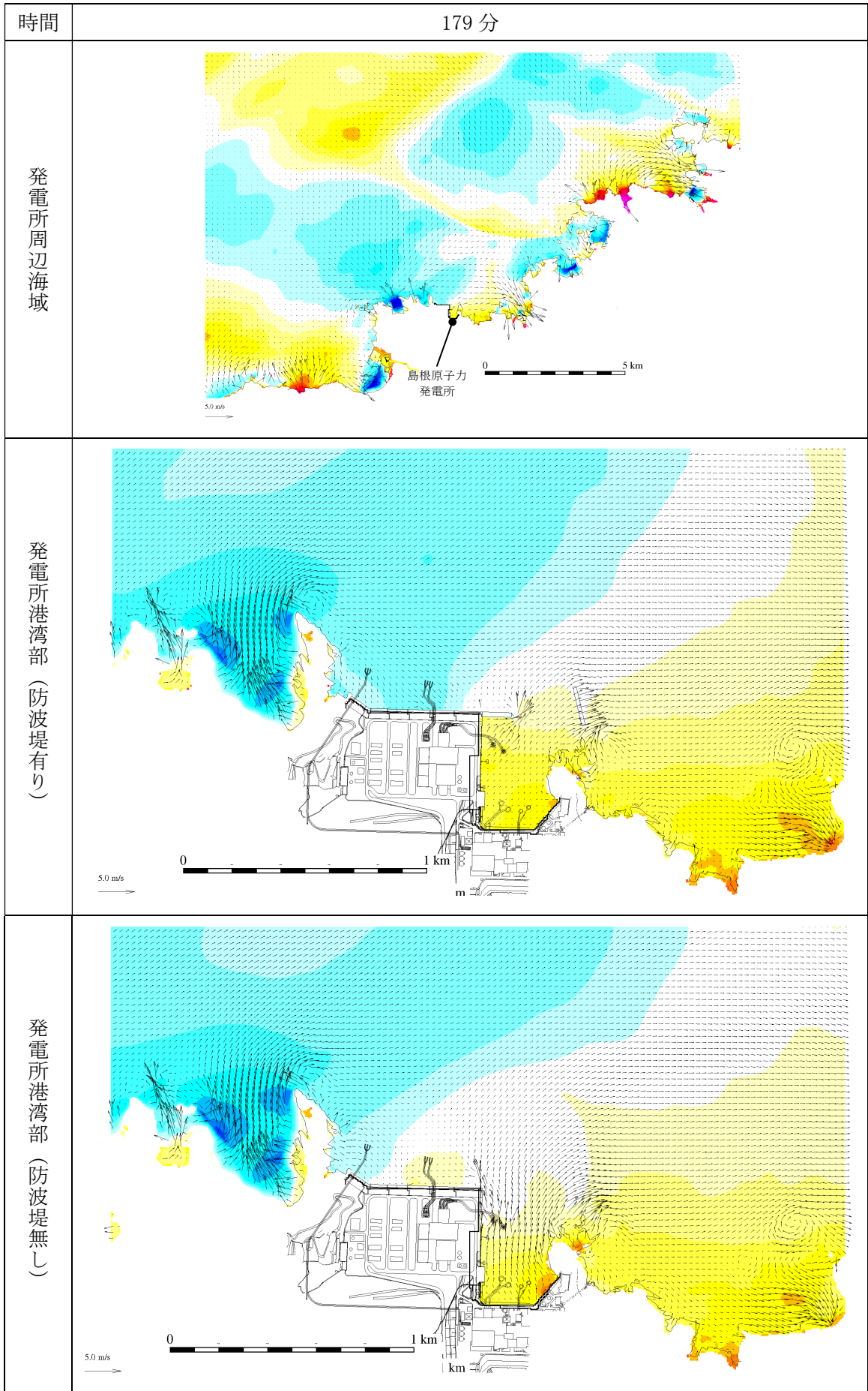
第 2.5-13-1 図(159) 基準津波 1 の水位変動・流向ベクトル
