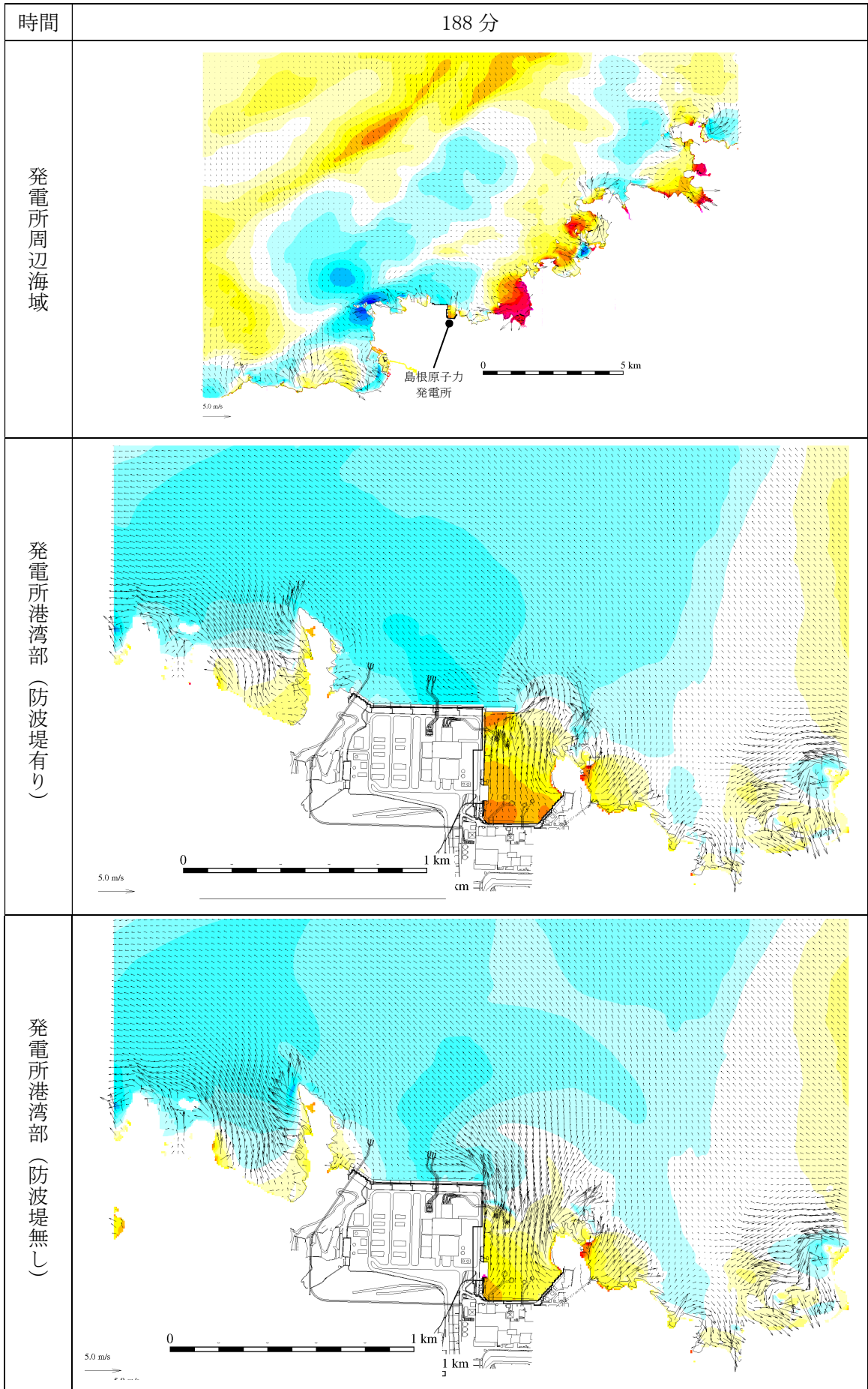
第 2.5-13-1 図(177) 基準津波 1 の水位変動・流向ベクトル
