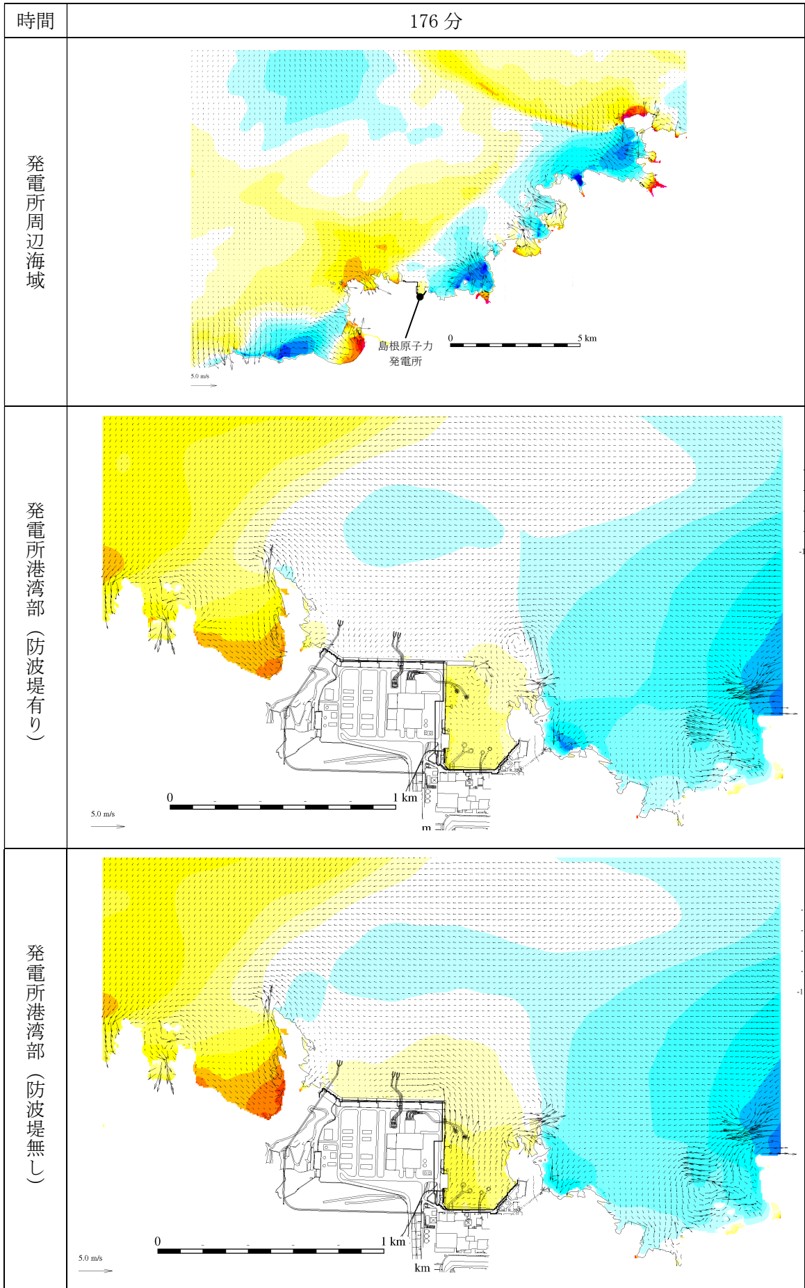
第 2.5-13-1 図(153) 基準津波 1 の水位変動・流向ベクトル
