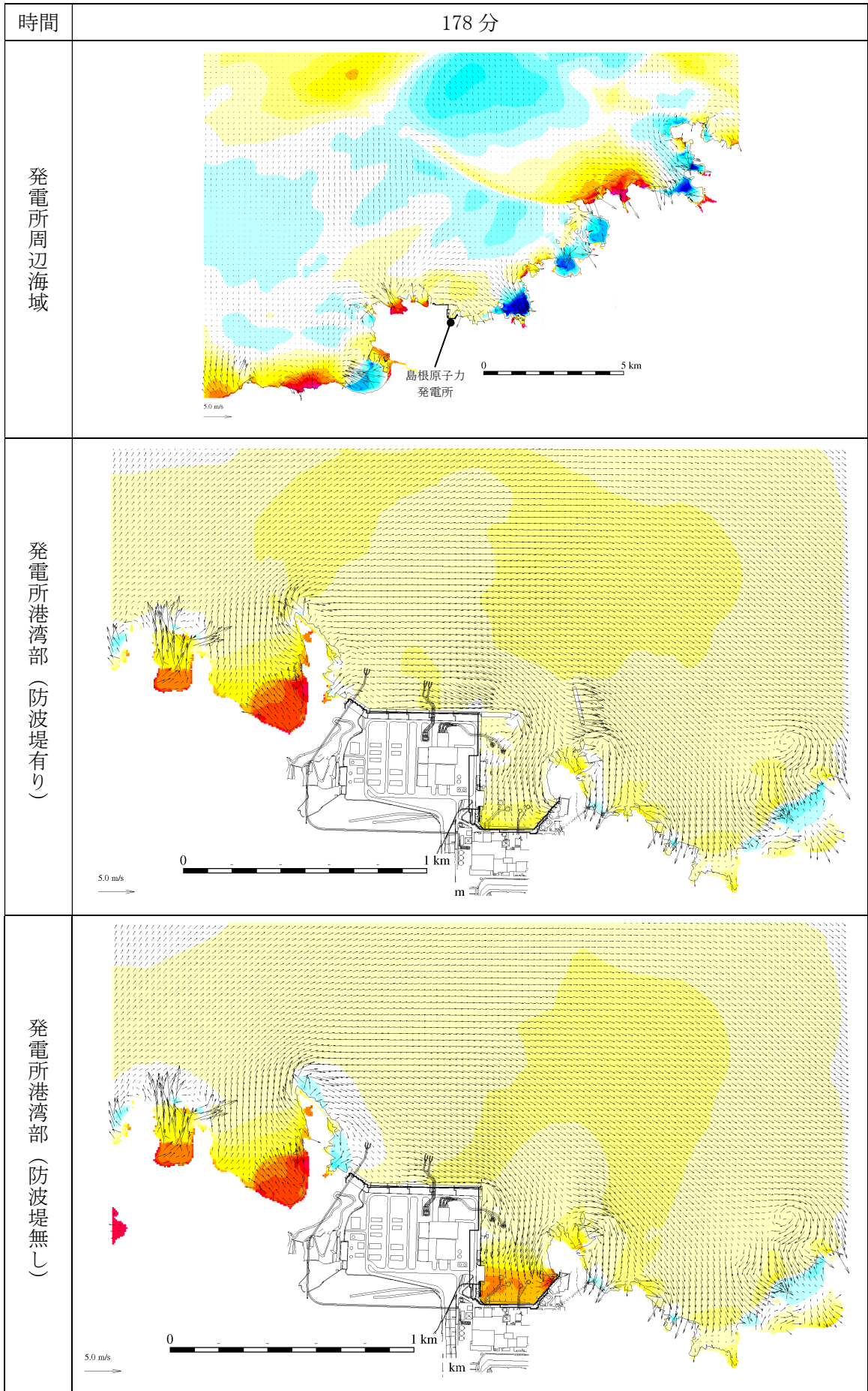
第 2.5-13-1 図(157) 基準津波 1 の水位変動・流向ベクトル
