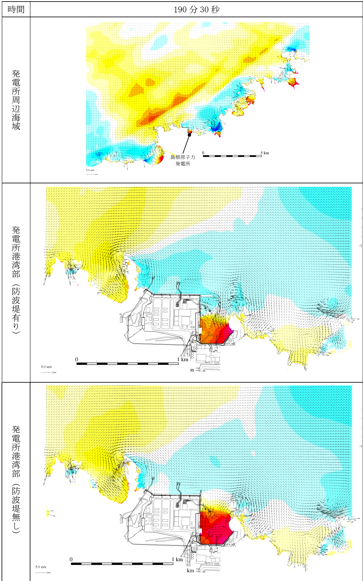
第 2.5-13-1 図(182) 基準津波 1 の水位変動・流向ベクトル
