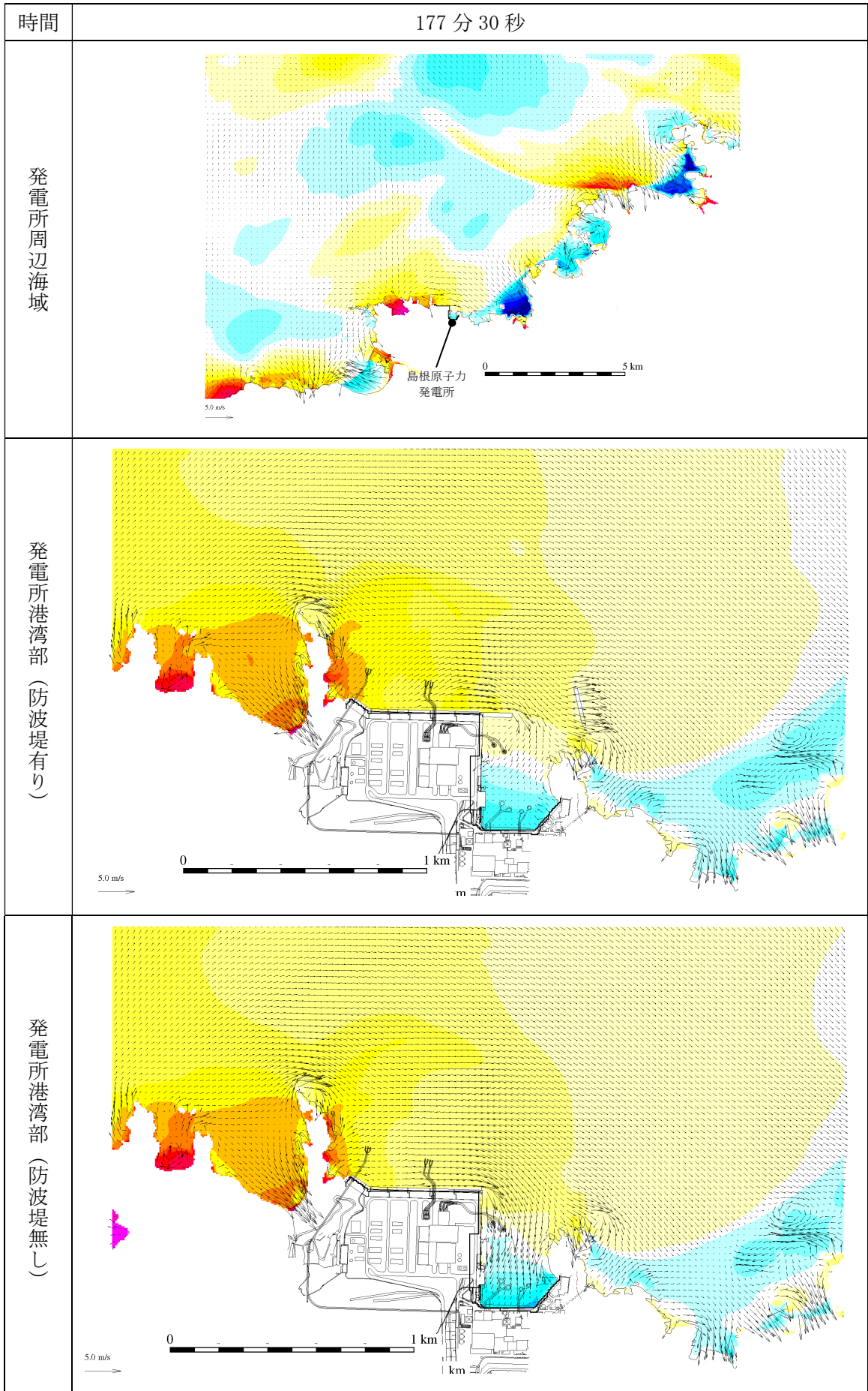
第 2.5-13-1 図(156) 基準津波 1 の水位変動・流向ベクトル
