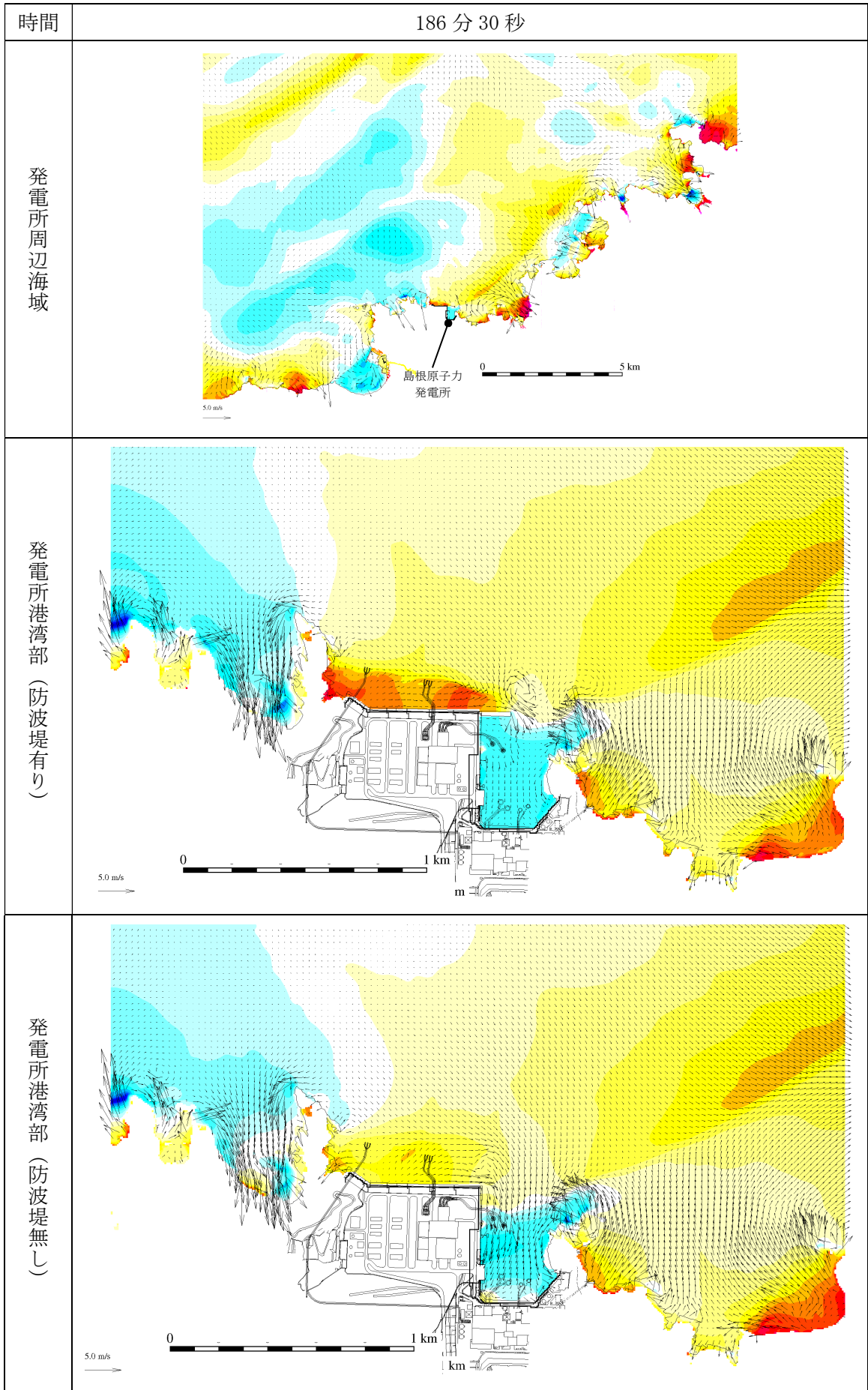
第 2.5-13-1 図(174) 基準津波 1 の水位変動・流向ベクトル
