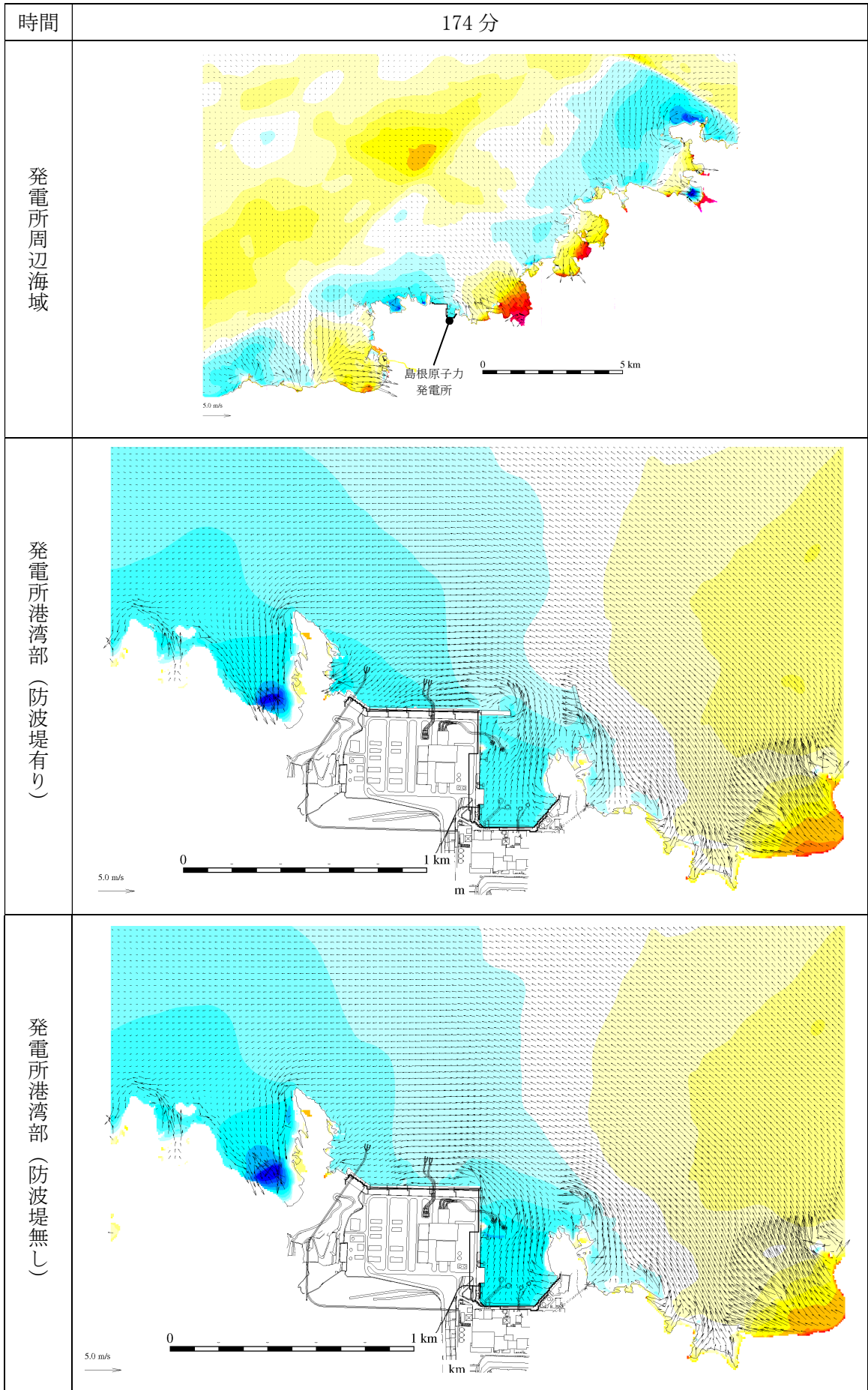
第 2.5-13-1 図(149) 基準津波 1 の水位変動・流向ベクトル
