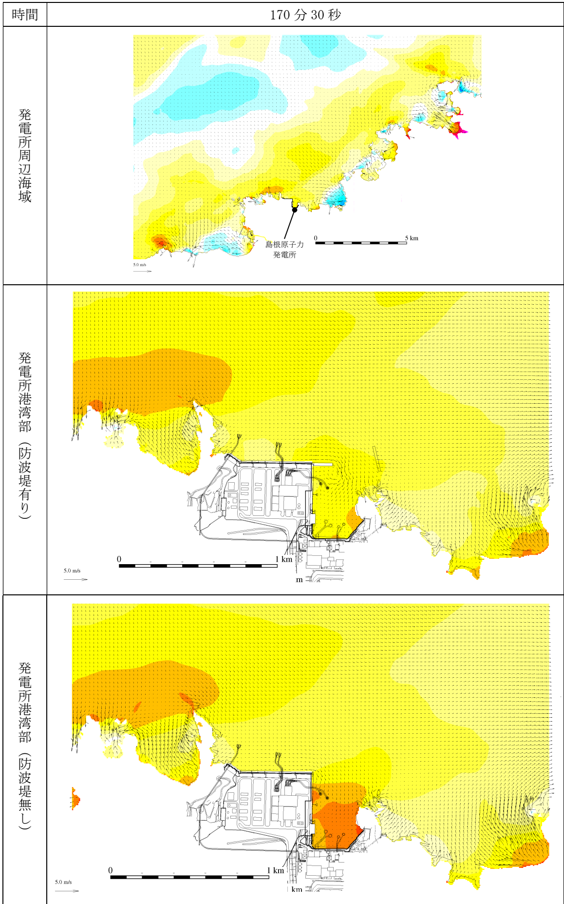
第 2.5-13-1 図(142) 基準津波 1 の水位変動・流向ベクトル
