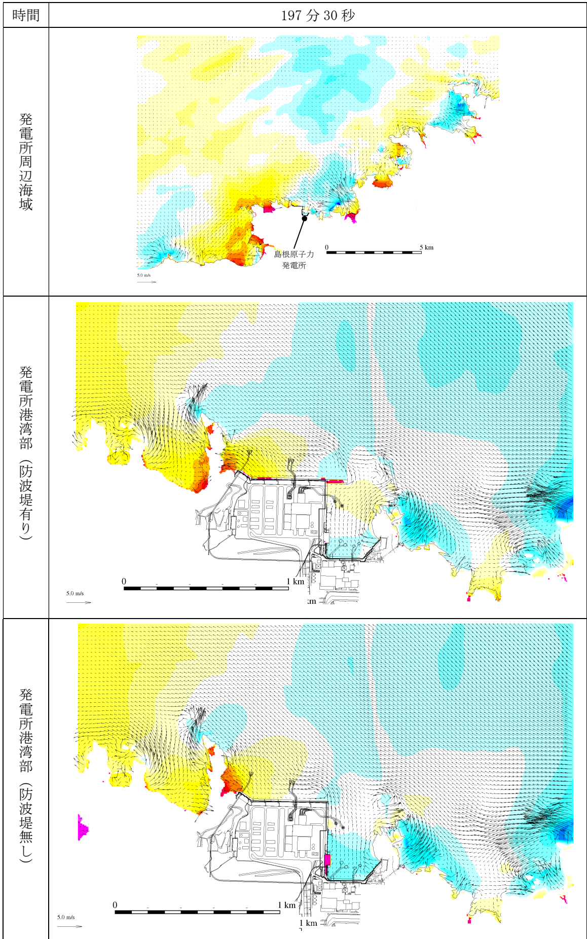
第 2.5-13-1 図(196) 基準津波 1 の水位変動・流向ベクトル
