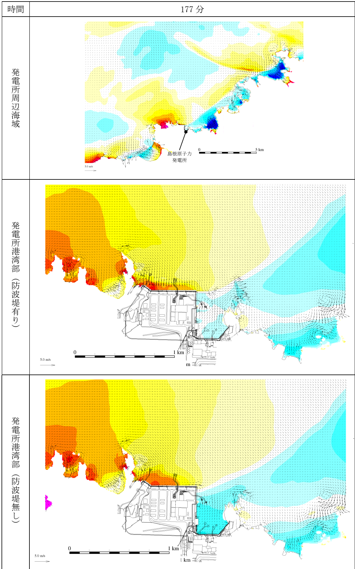
第 2.5-13-1 図(155) 基準津波 1 の水位変動・流向ベクトル
