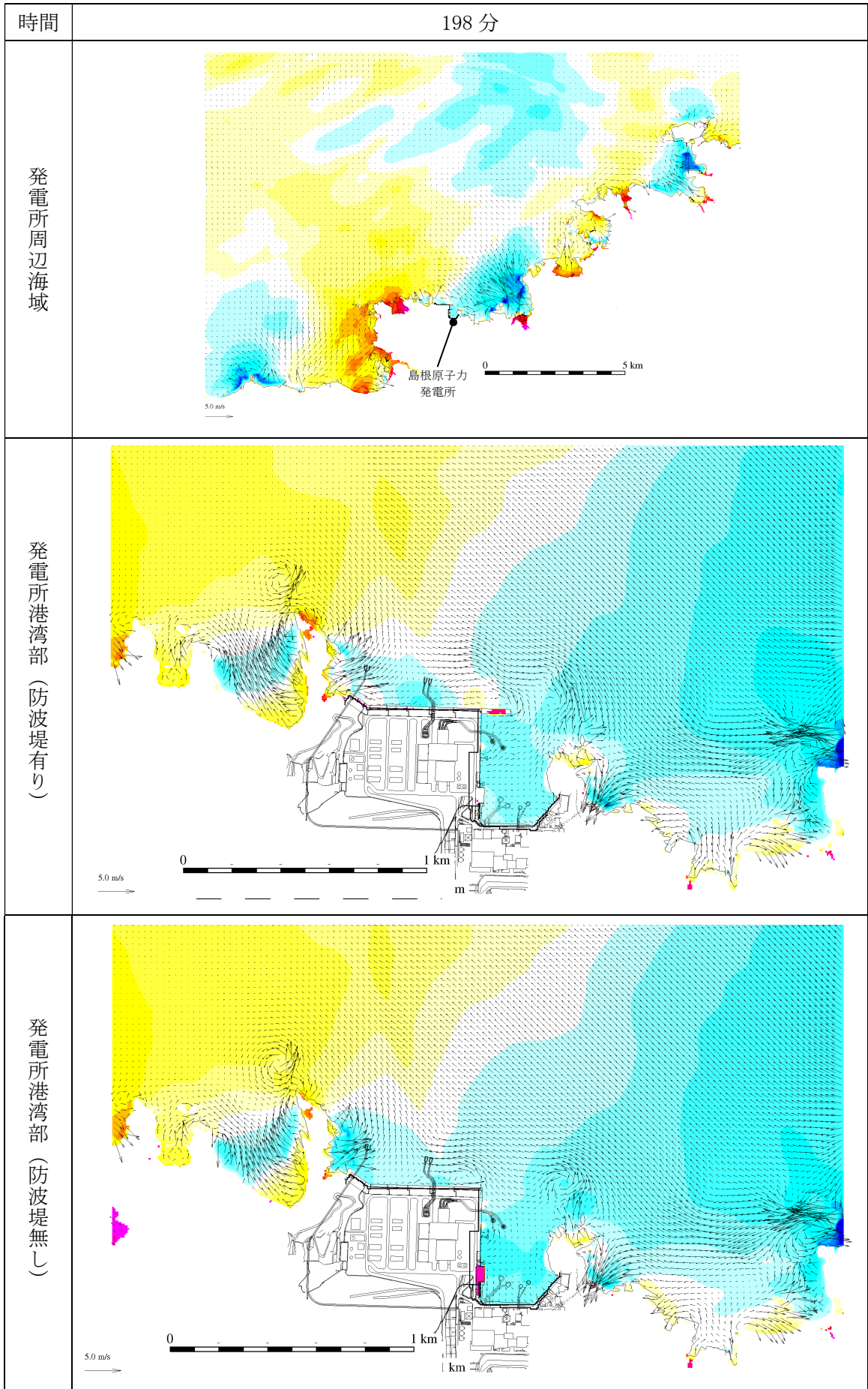
第 2.5-13-1 図(197) 基準津波 1 の水位変動・流向ベクトル
