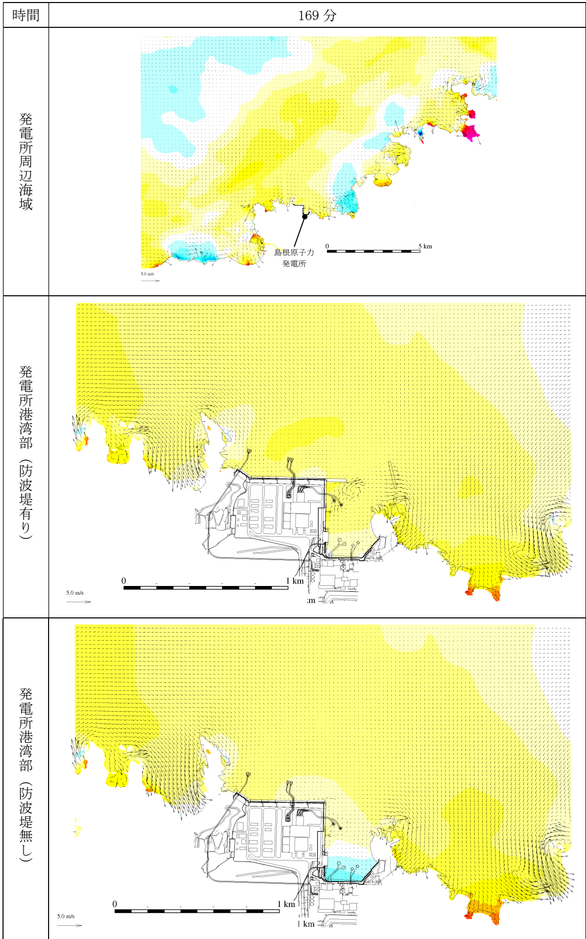
第 2.5-13-1 図(139) 基準津波 1 の水位変動・流向ベクトル
