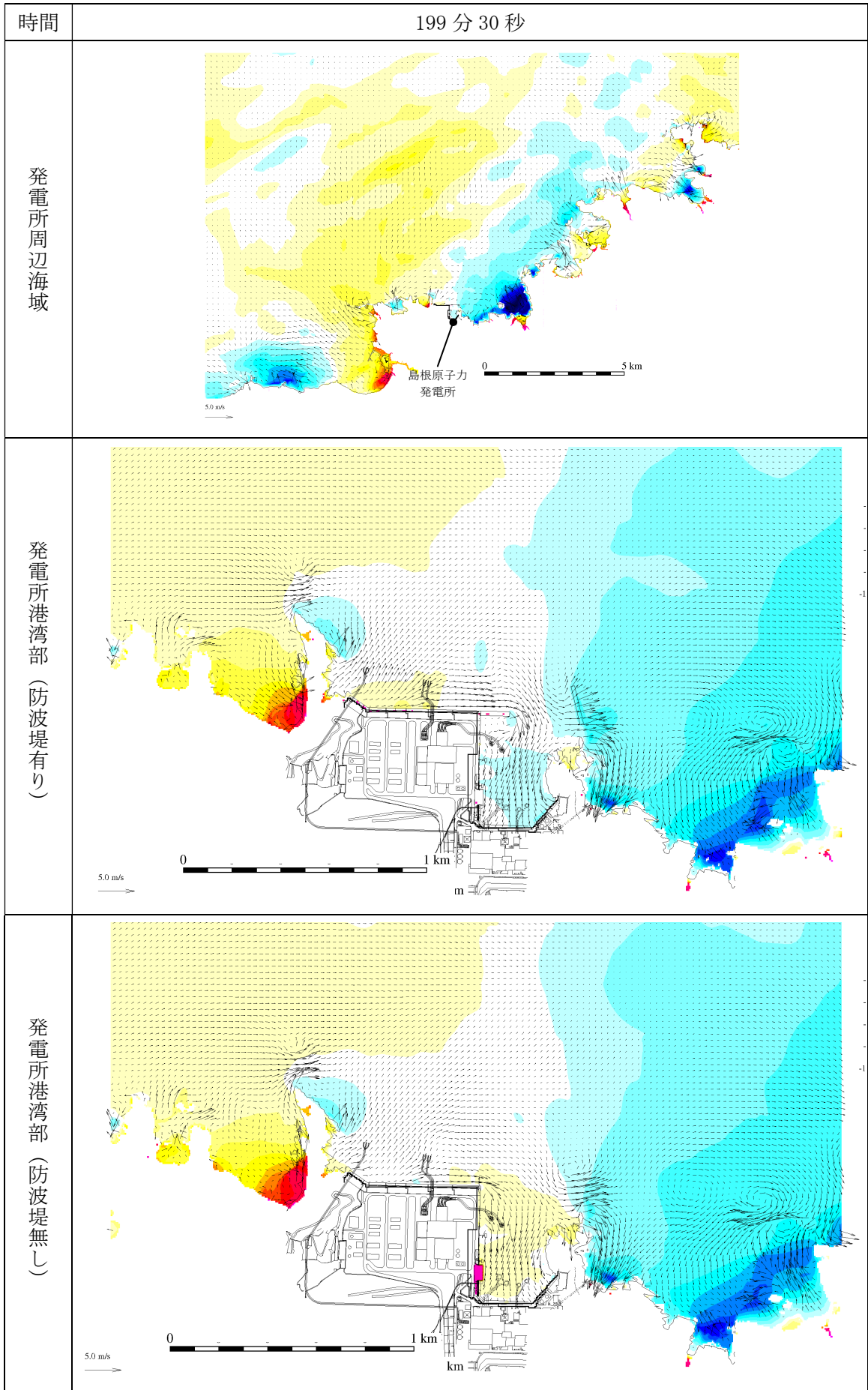
第 2.5-13-1 図(200) 基準津波 1 の水位変動・流向ベクトル
