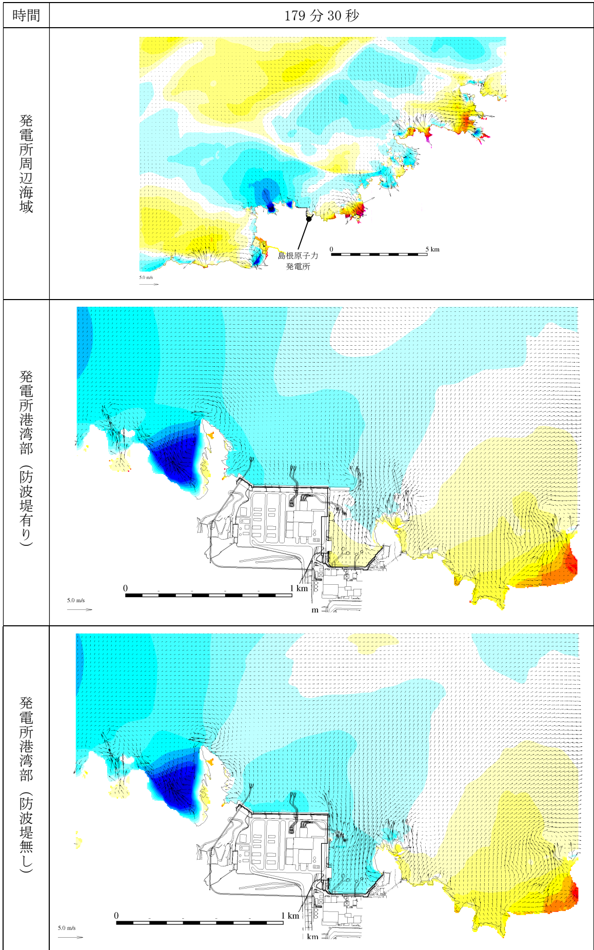
第 2.5-13-1 図(160) 基準津波 1 の水位変動・流向ベクトル
