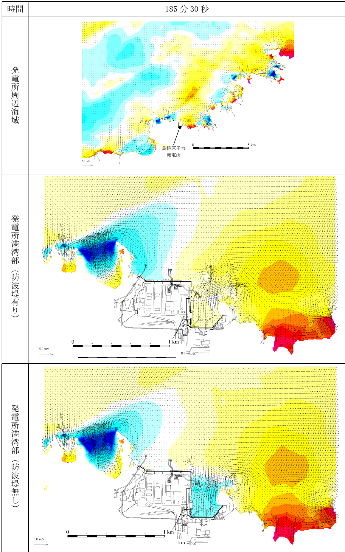
第 2.5-13-1 図(172) 基準津波 1 の水位変動・流向ベクトル
