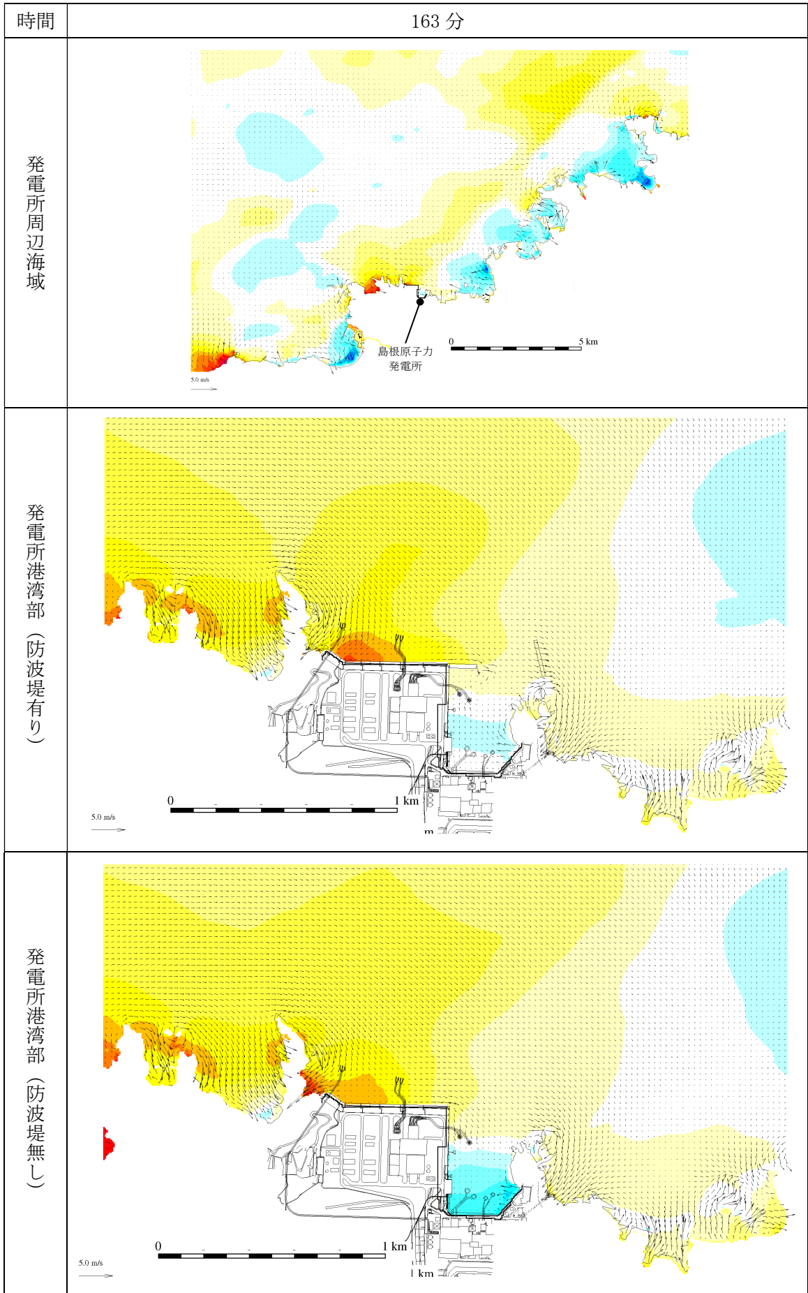
第 2.5-13-1 図(127) 基準津波 1 の水位変動・流向ベクトル
