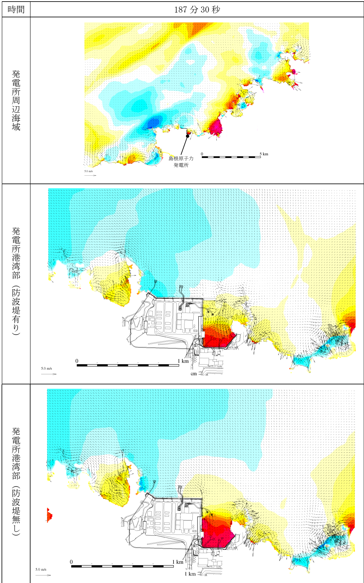
第 2.5-13-1 図(176) 基準津波 1 の水位変動・流向ベクトル
