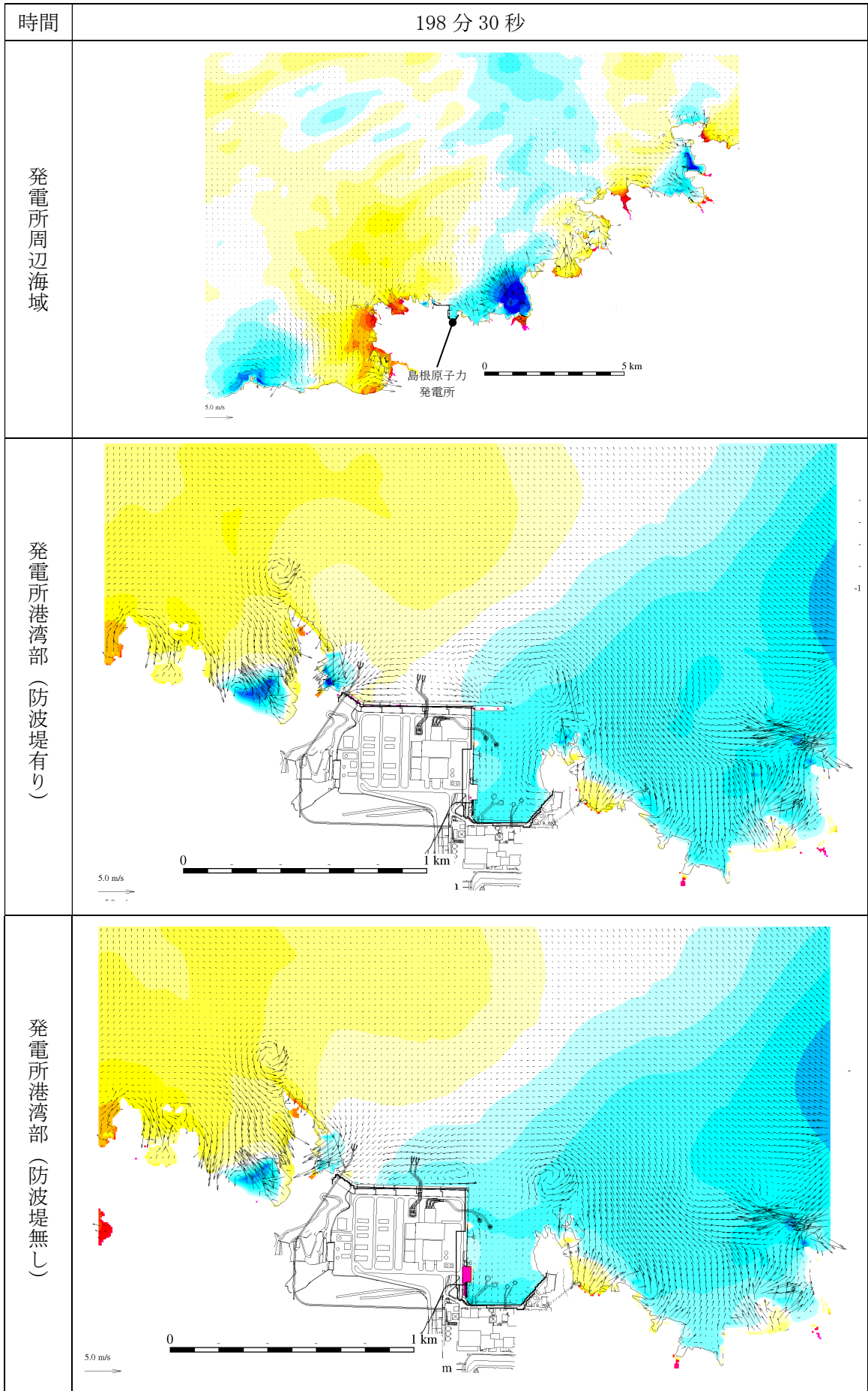
第 2.5-13-1 図(198) 基準津波 1 の水位変動・流向ベクトル
