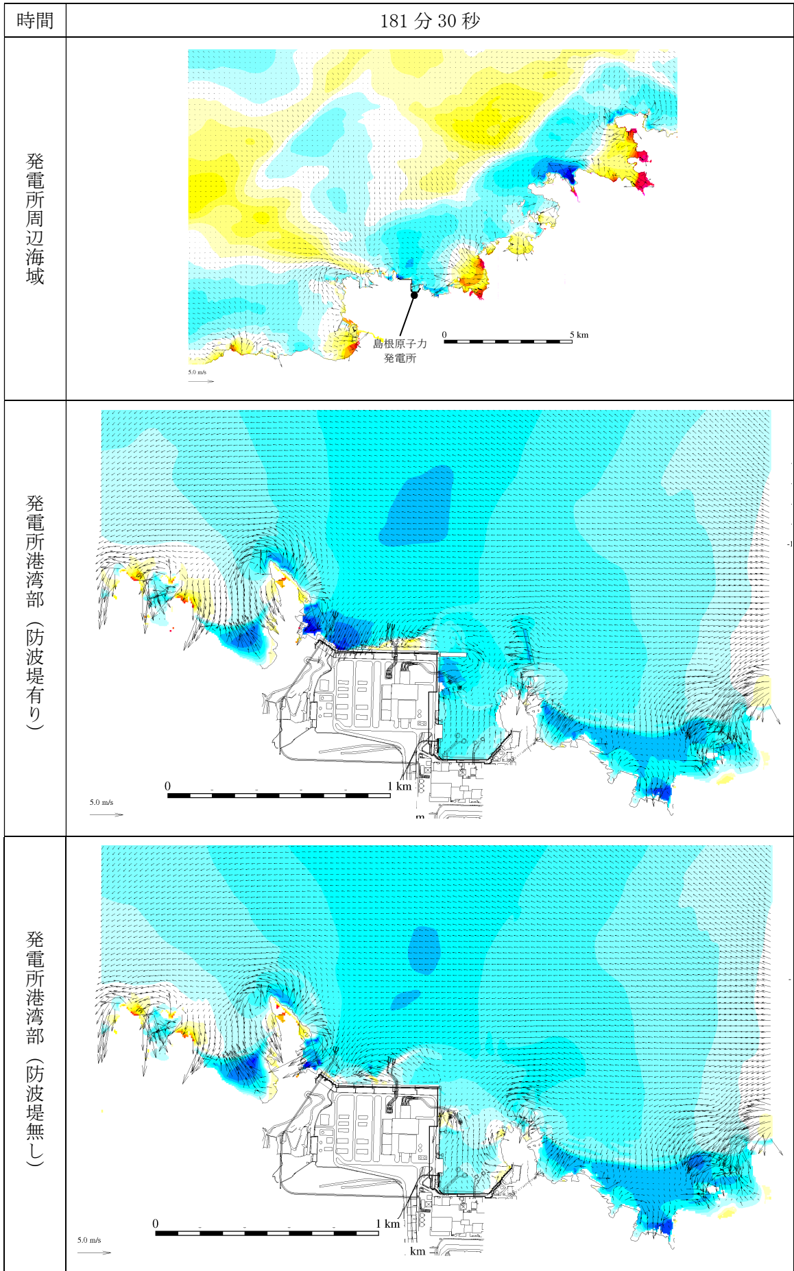
第 2.5-13-1 図(164) 基準津波 1 の水位変動・流向ベクトル
