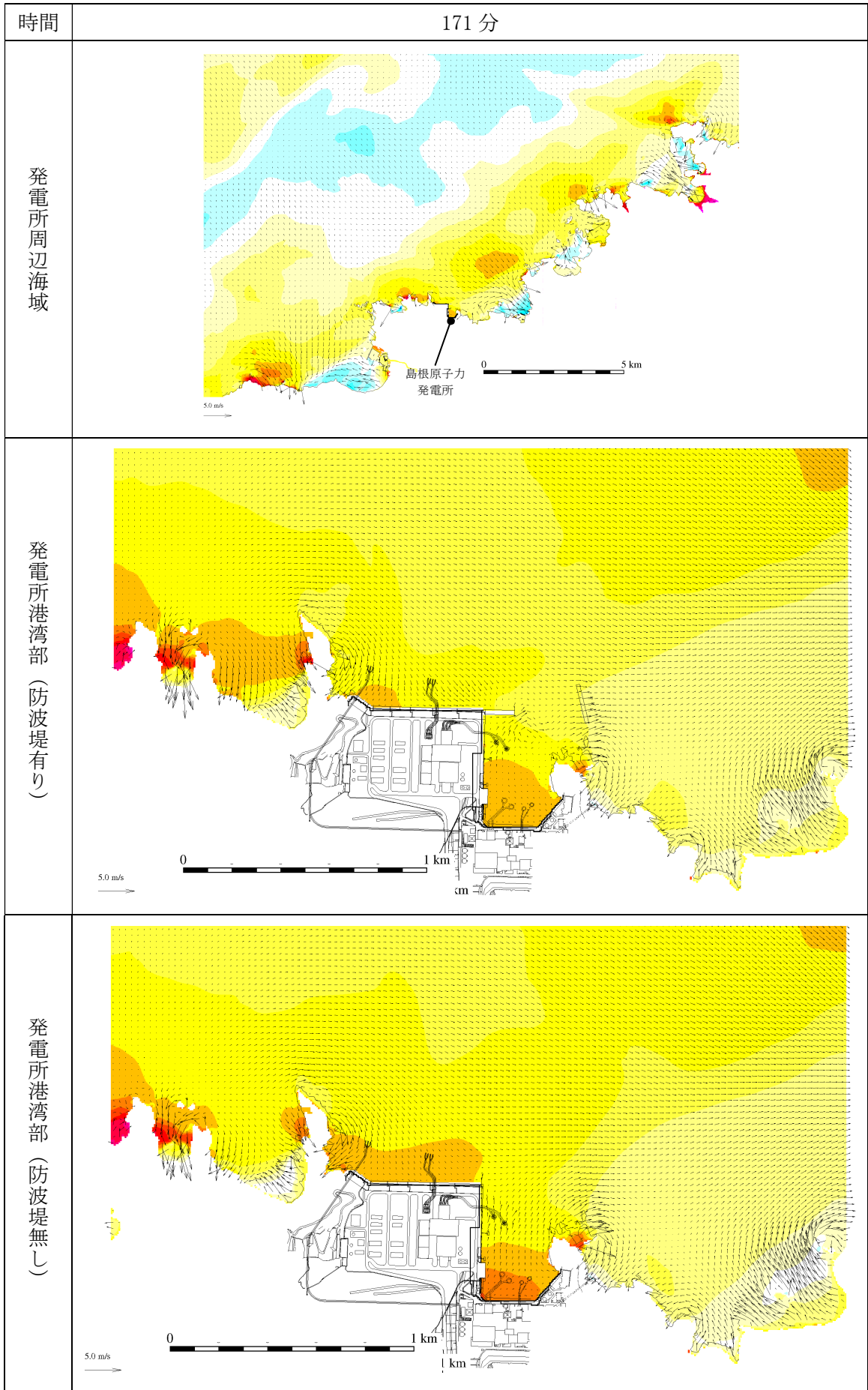
第 2.5-13-1 図(143) 基準津波 1 の水位変動・流向ベクトル
