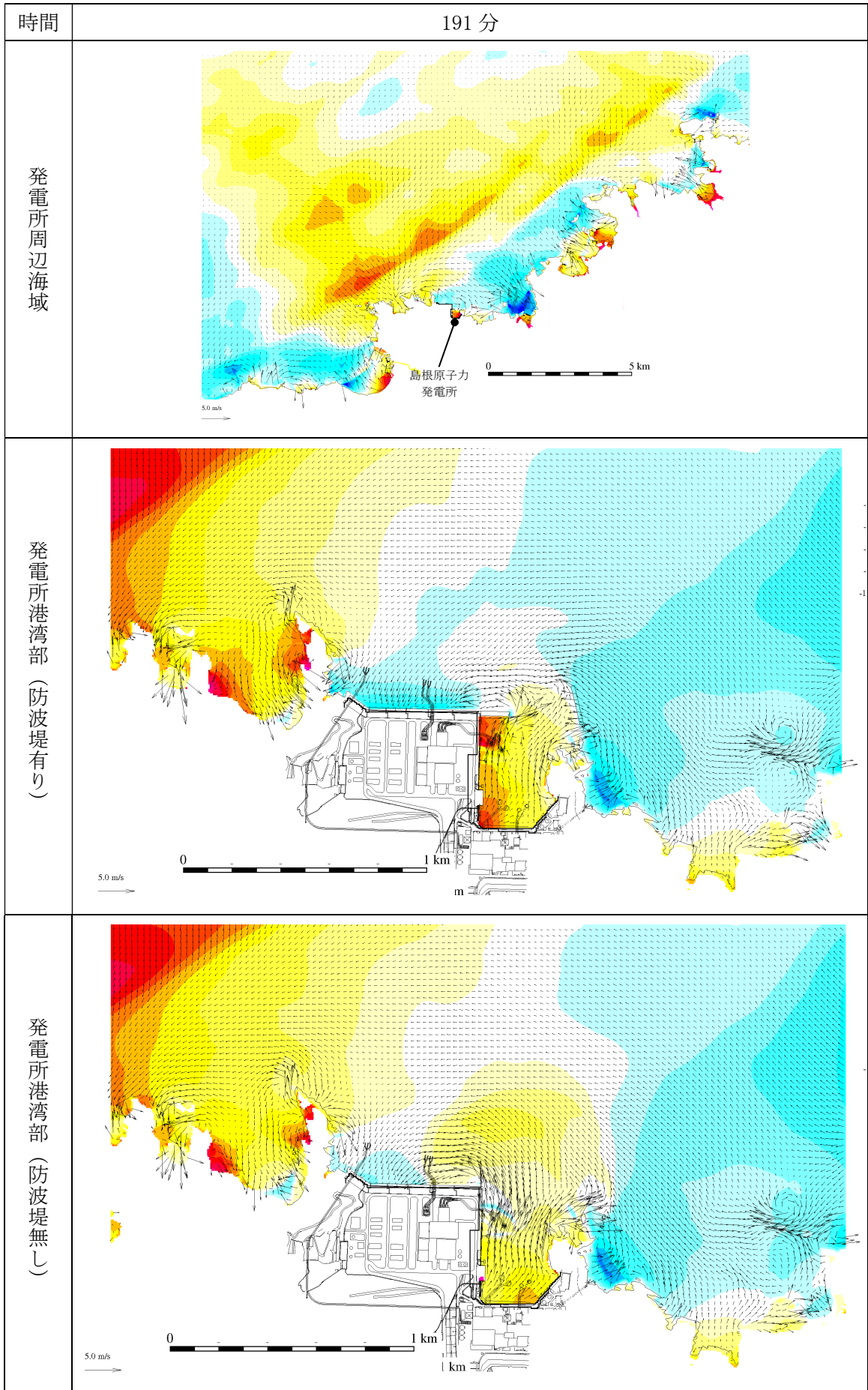
第 2.5-13-1 図(183) 基準津波 1 の水位変動・流向ベクトル
