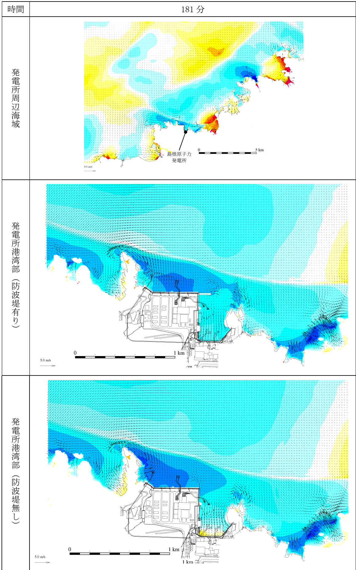
第 2.5-13-1 図(163) 基準津波 1 の水位変動・流向ベクトル
