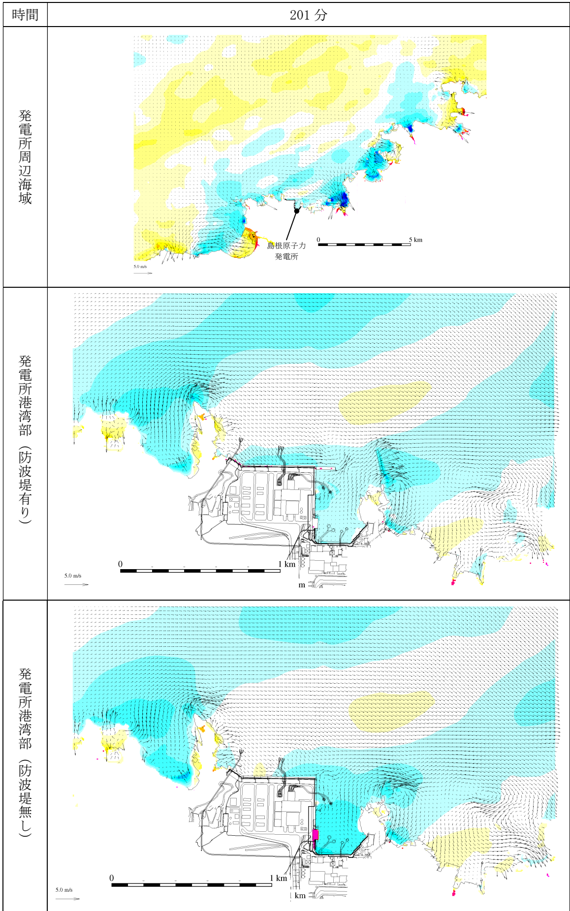
第 2.5-13-1 図(203) 基準津波 1 の水位変動・流向ベクトル
