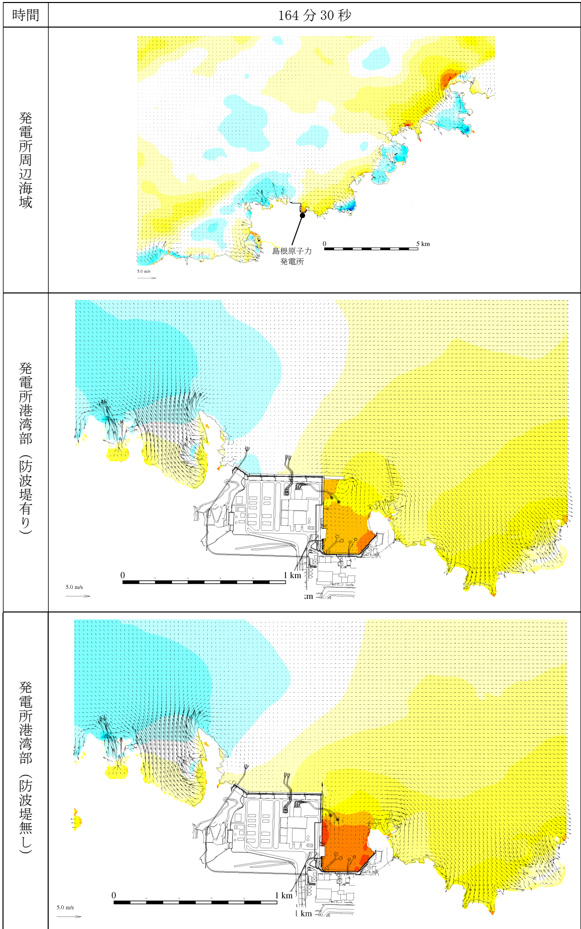
第 2.5-13-1 図(130) 基準津波 1 の水位変動・流向ベクトル
