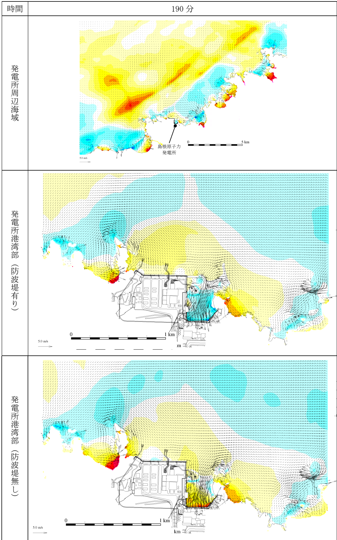
第 2.5-13-1 図(181) 基準津波 1 の水位変動・流向ベクトル
