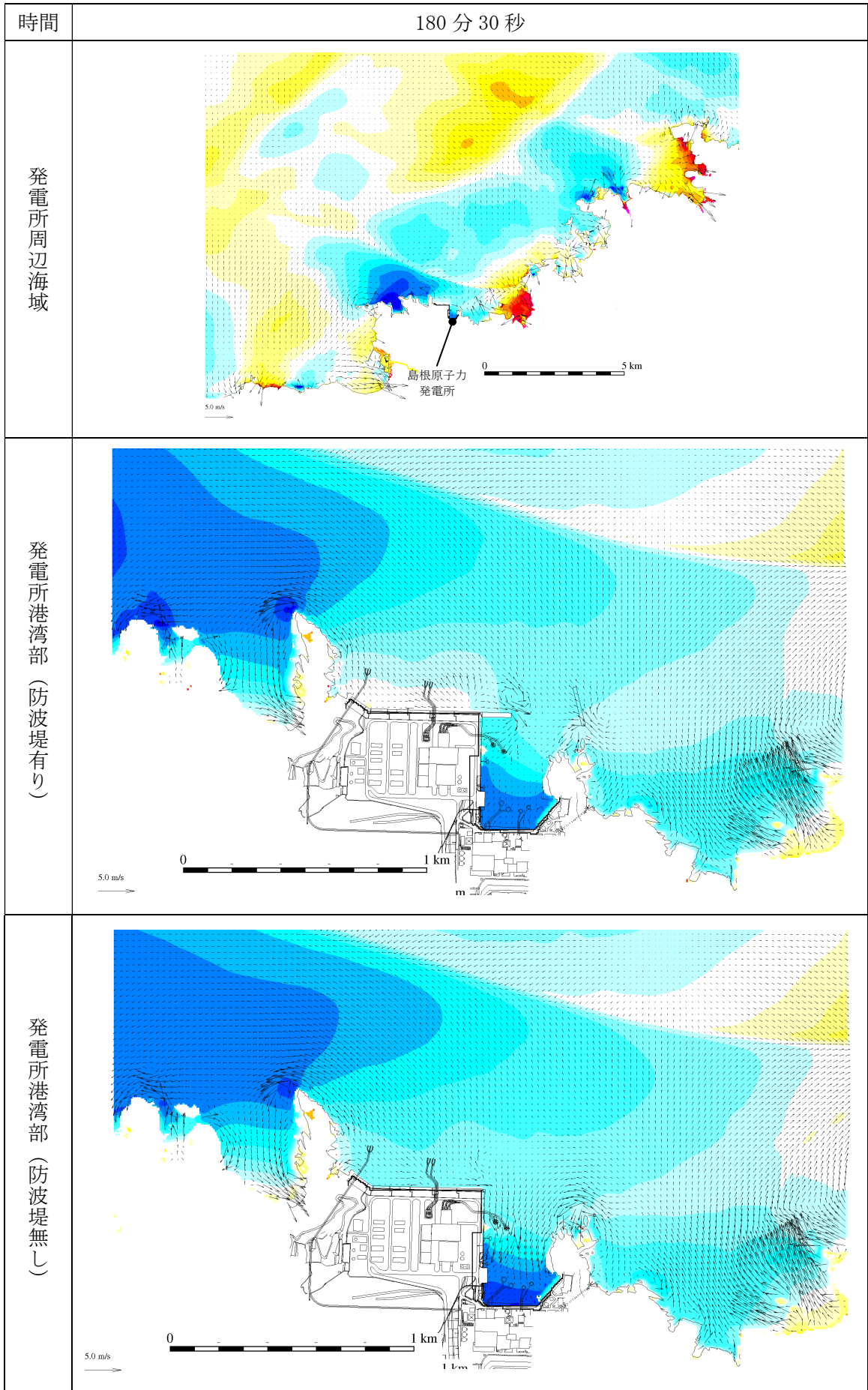
第 2.5-13-1 図(162) 基準津波 1 の水位変動・流向ベクトル
