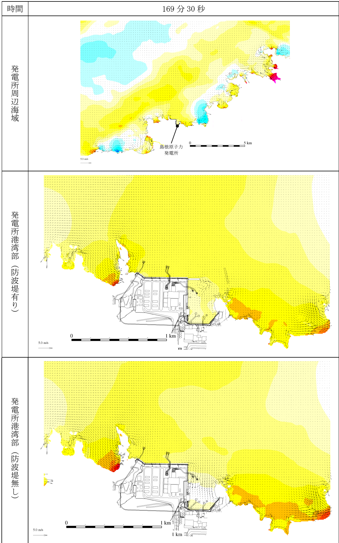
第 2.5-13-1 図(140) 基準津波 1 の水位変動・流向ベクトル
