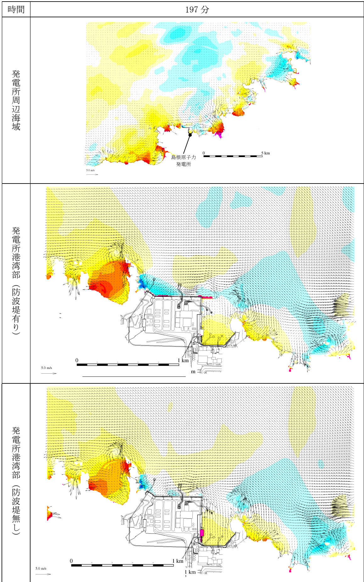
第 2.5-13-1 図(195) 基準津波 1 の水位変動・流向ベクトル
