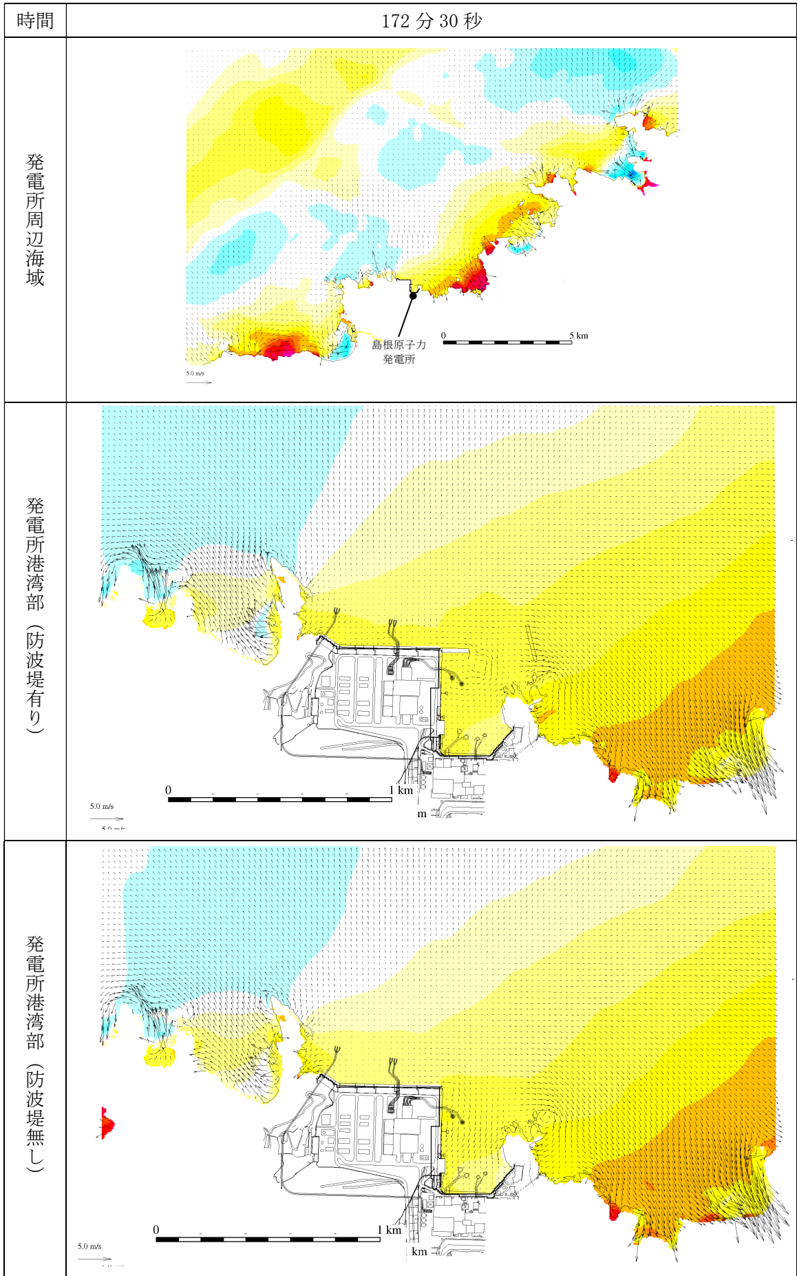
第 2.5-13-1 図(146) 基準津波 1 の水位変動・流向ベクトル
