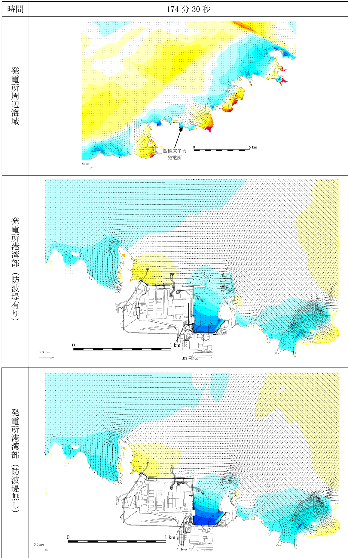
第 2.5-13-1 図(150) 基準津波 1 の水位変動・流向ベクトル
