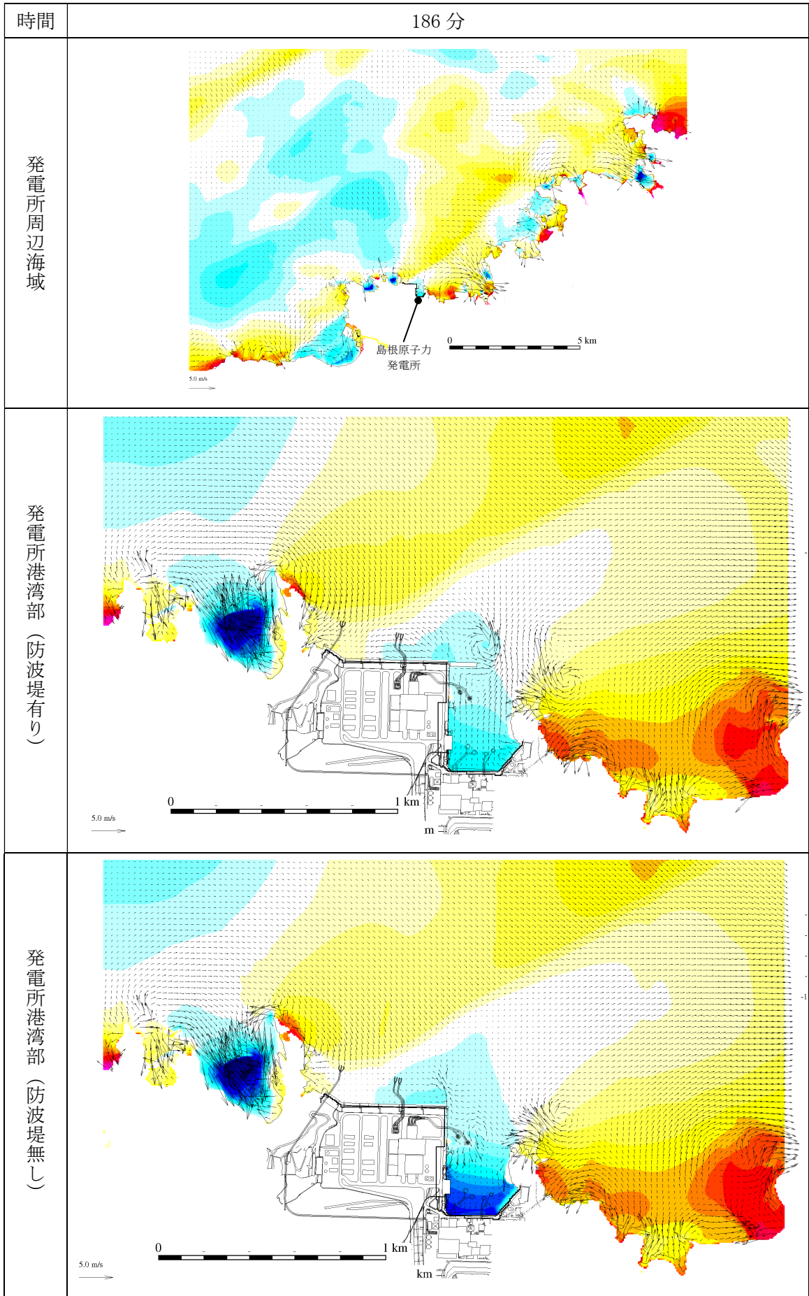
第 2.5-13-1 図(173) 基準津波 1 の水位変動・流向ベクトル
