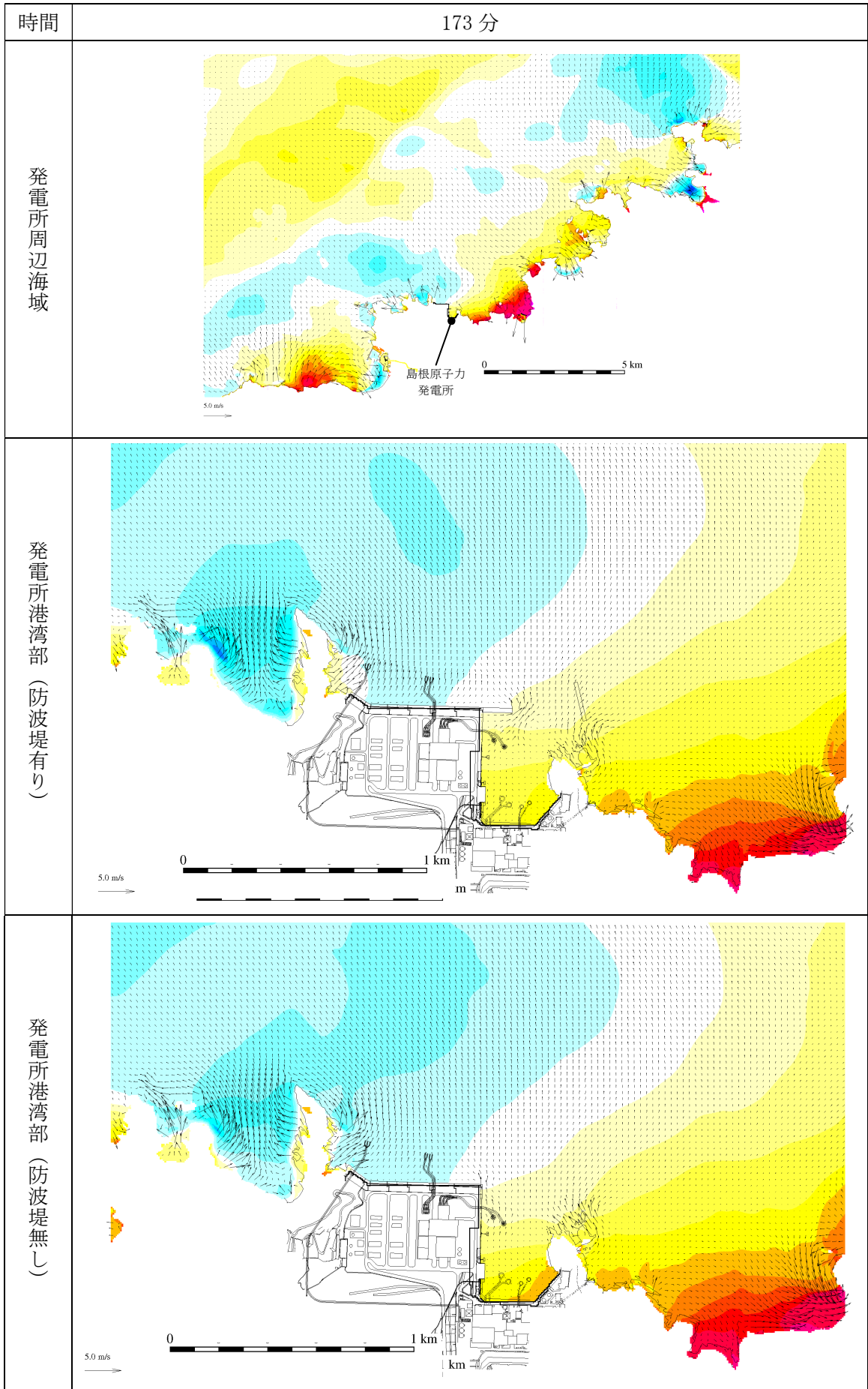
第 2.5-13-1 図(147) 基準津波 1 の水位変動・流向ベクトル
