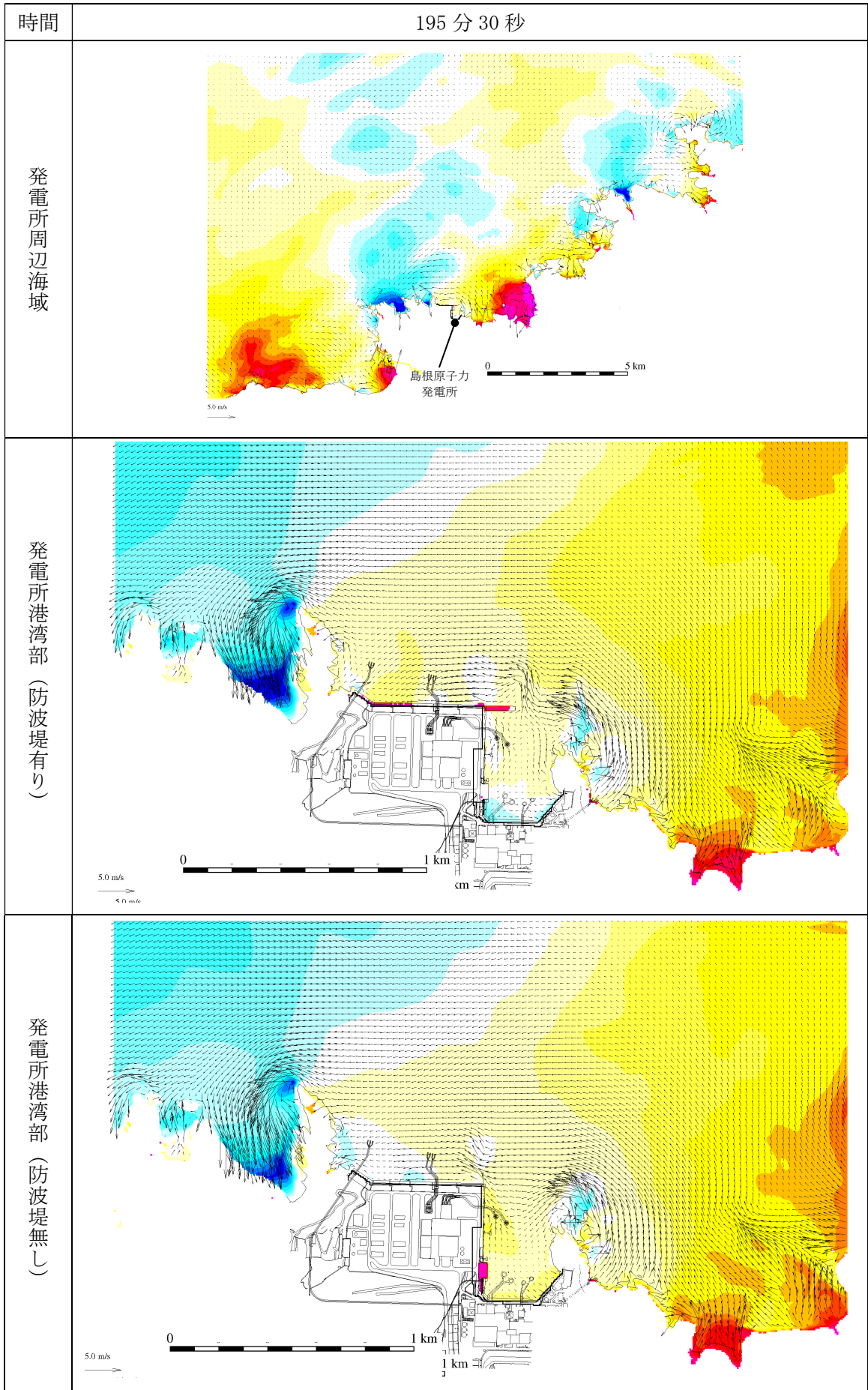
第 2.5-13-1 図(192) 基準津波 1 の水位変動・流向ベクトル
