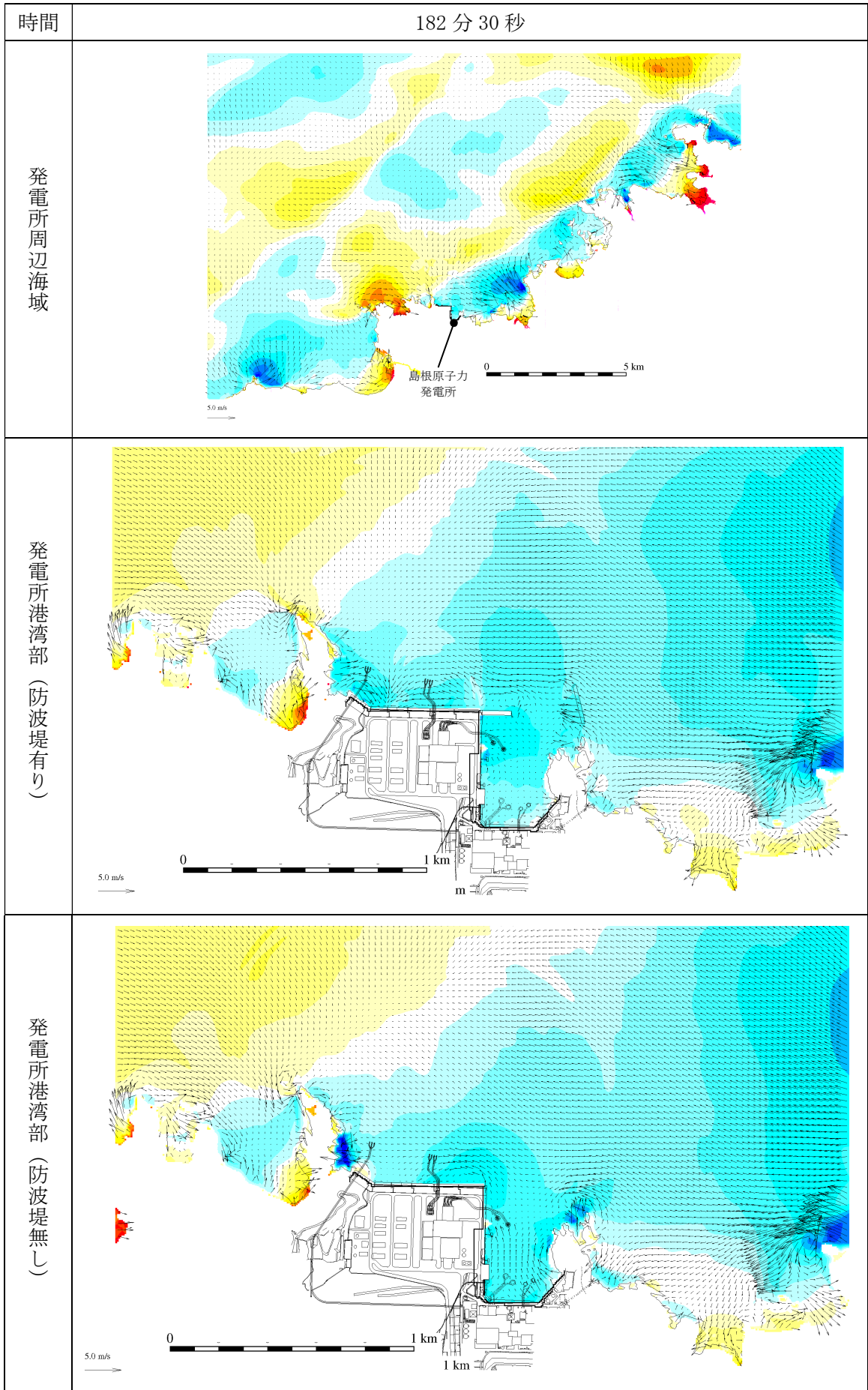
第 2.5-13-1 図(166) 基準津波 1 の水位変動・流向ベクトル
