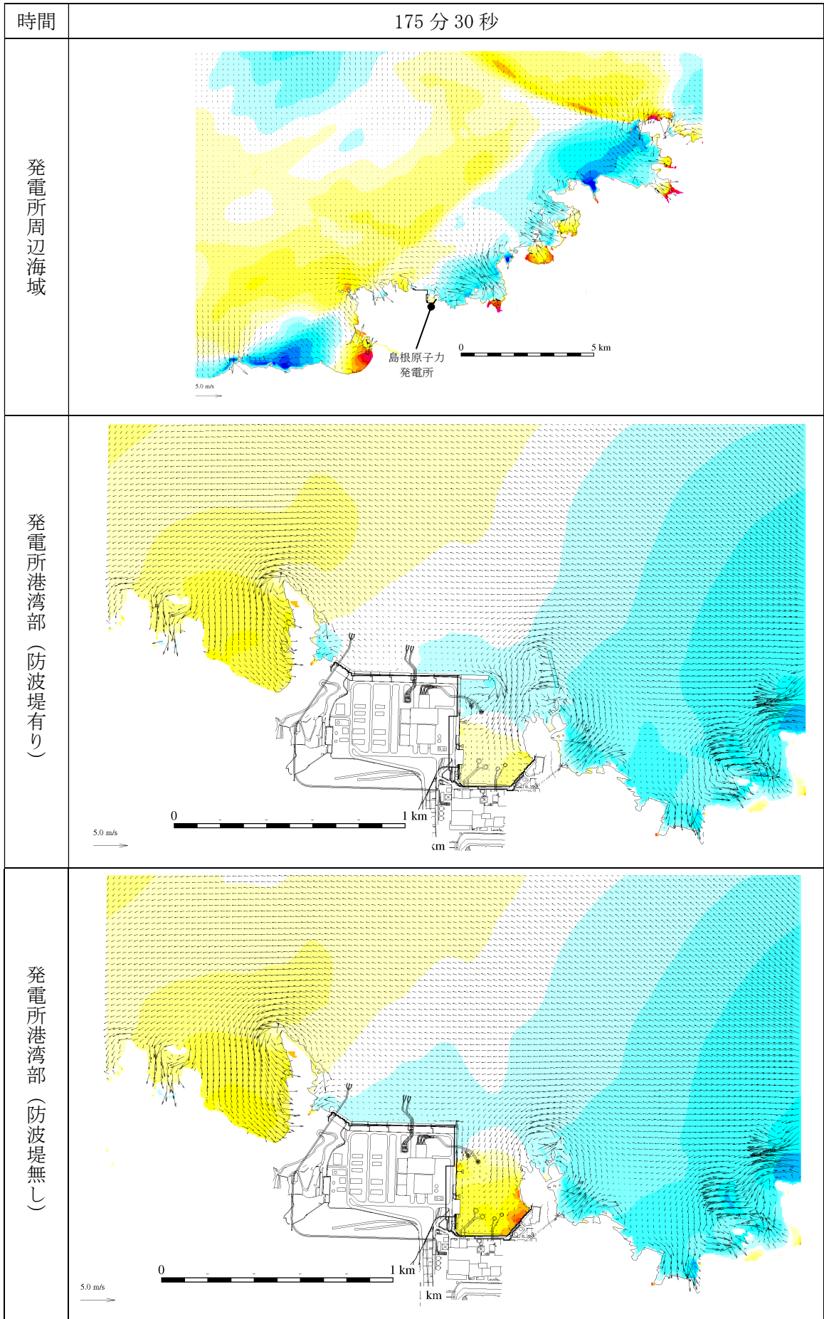
第 2.5-13-1 図(152) 基準津波 1 の水位変動・流向ベクトル
