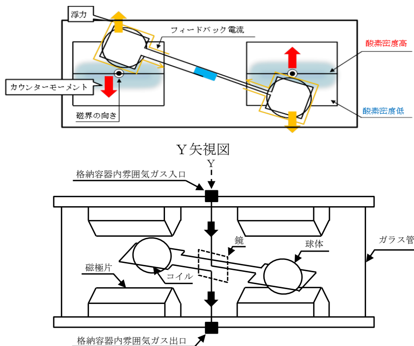
図3 格納容器酸素濃度 (SA) の概要図
