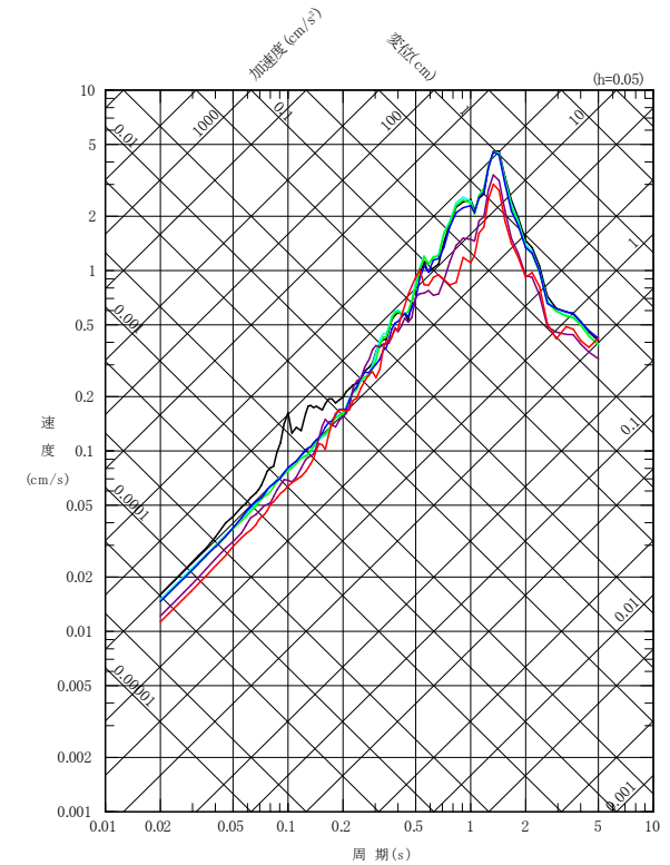
UD成分
