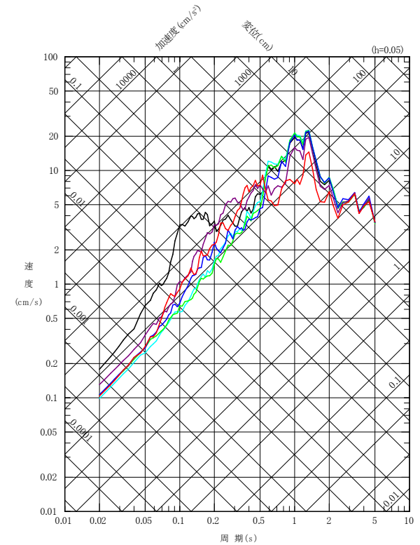
UD成分
