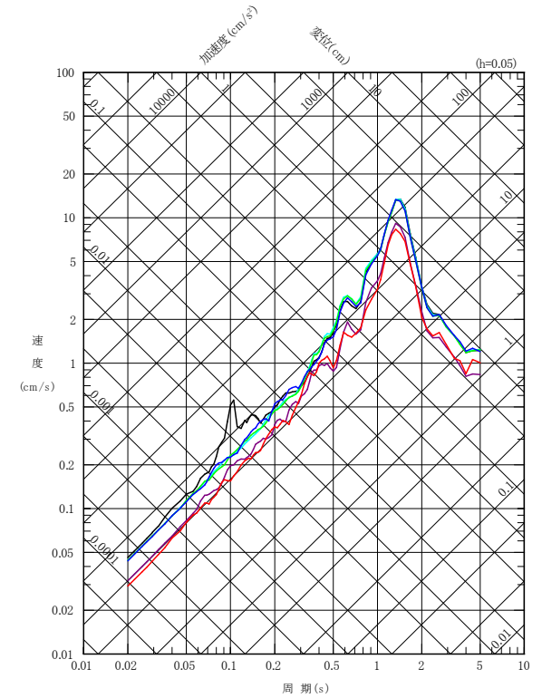
UD成分
