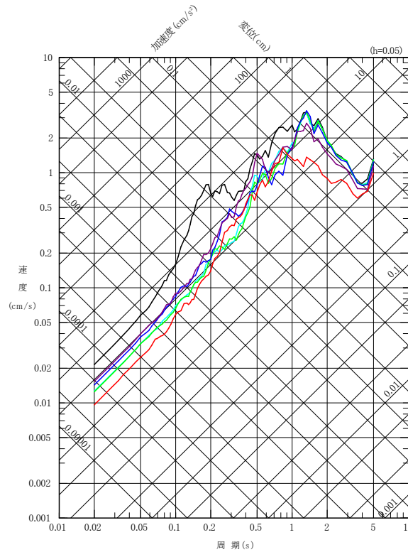
EW成分
