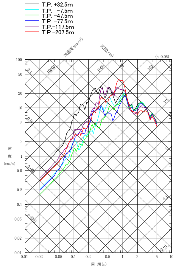
NS成分
