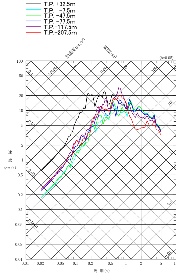
EW成分
