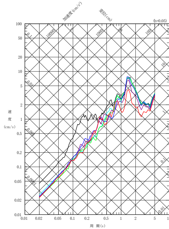
EW成分
