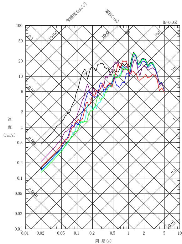
NS成分
