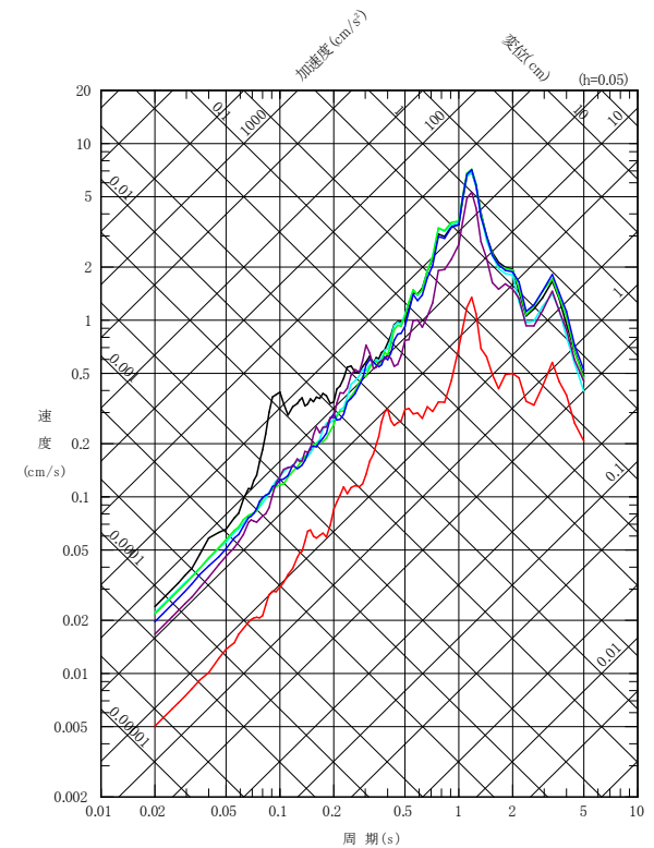
UD成分
