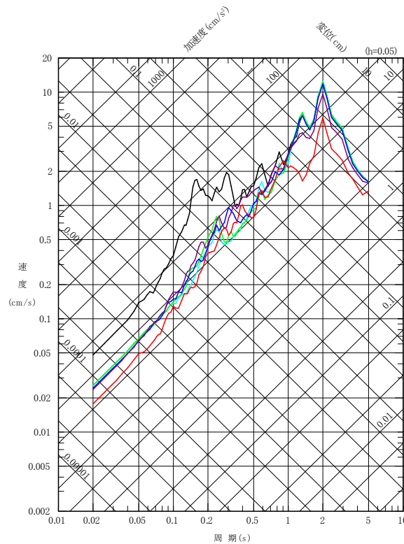
EW成分
