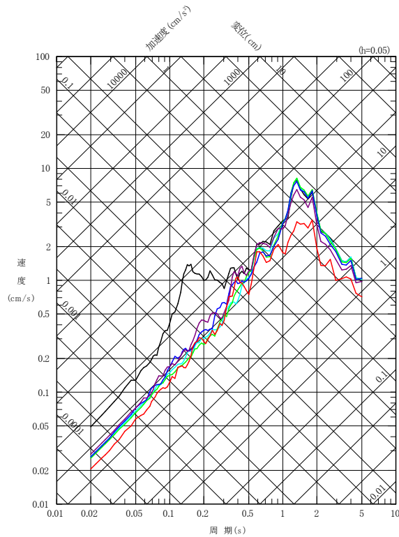
NS成分
