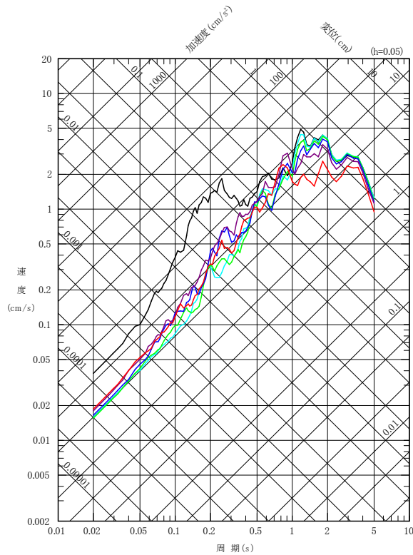
NS成分
