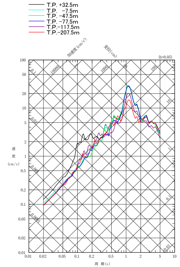
UD成分
