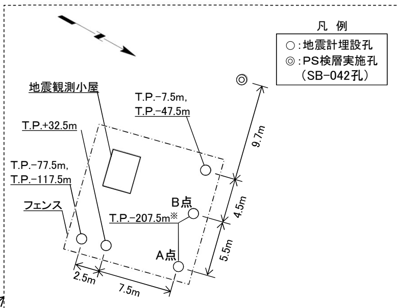
鉛直アレイ地震観測地点の詳細
