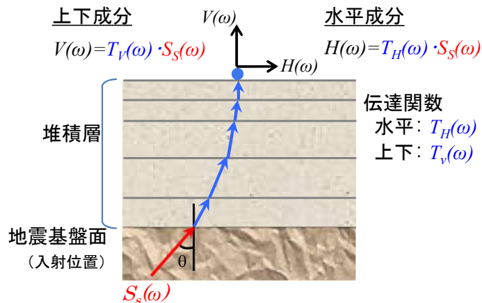
地震波の伝播の概念図
