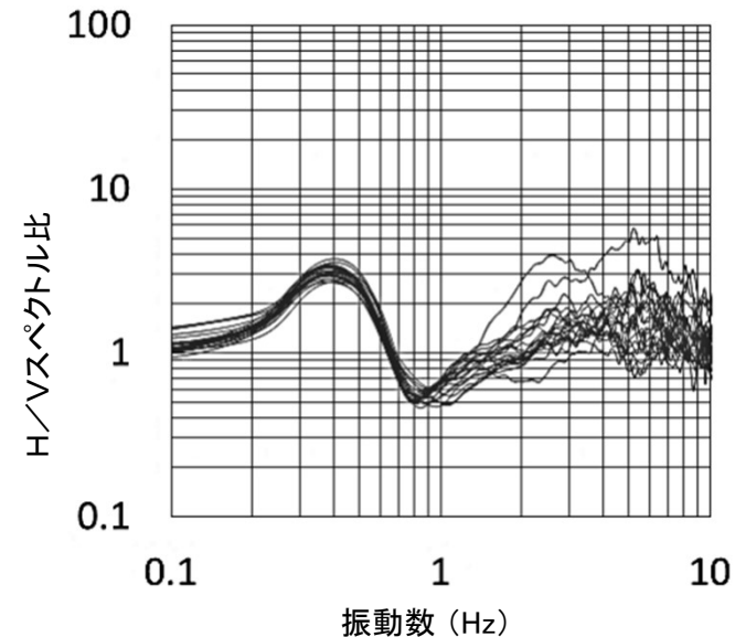
全観測点のH/Vスペクトル比※2, 3
