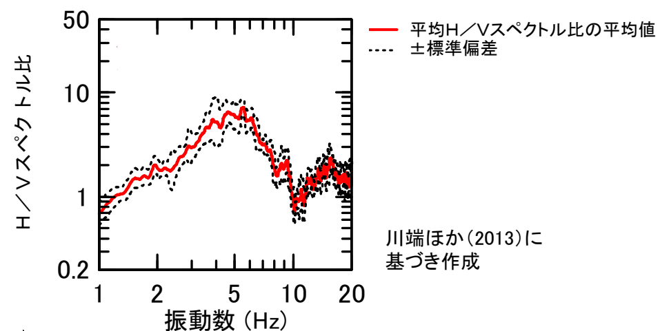
(c) 平均H/Vスペクトル比の平均値と標準偏差
