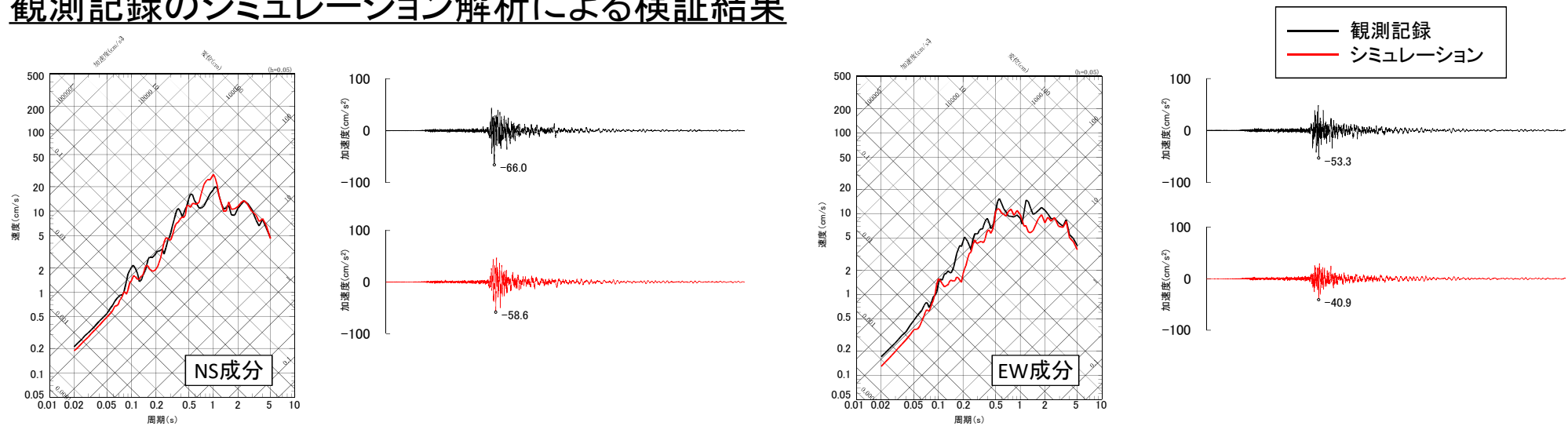
①平成5年(1993年)釧路沖地震の観測記録とシミュレーション解析結果の比較 (T.P.-7.5m)
