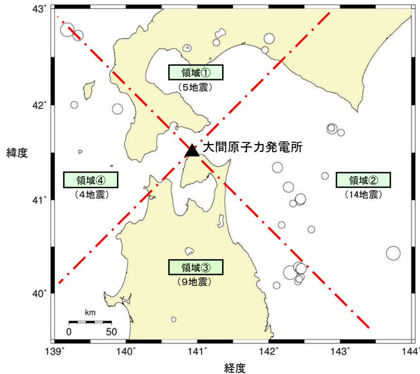
検討対象地震の震央分布
