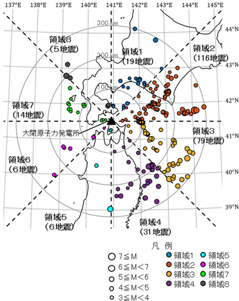
検討に用いた地震の震央分布
