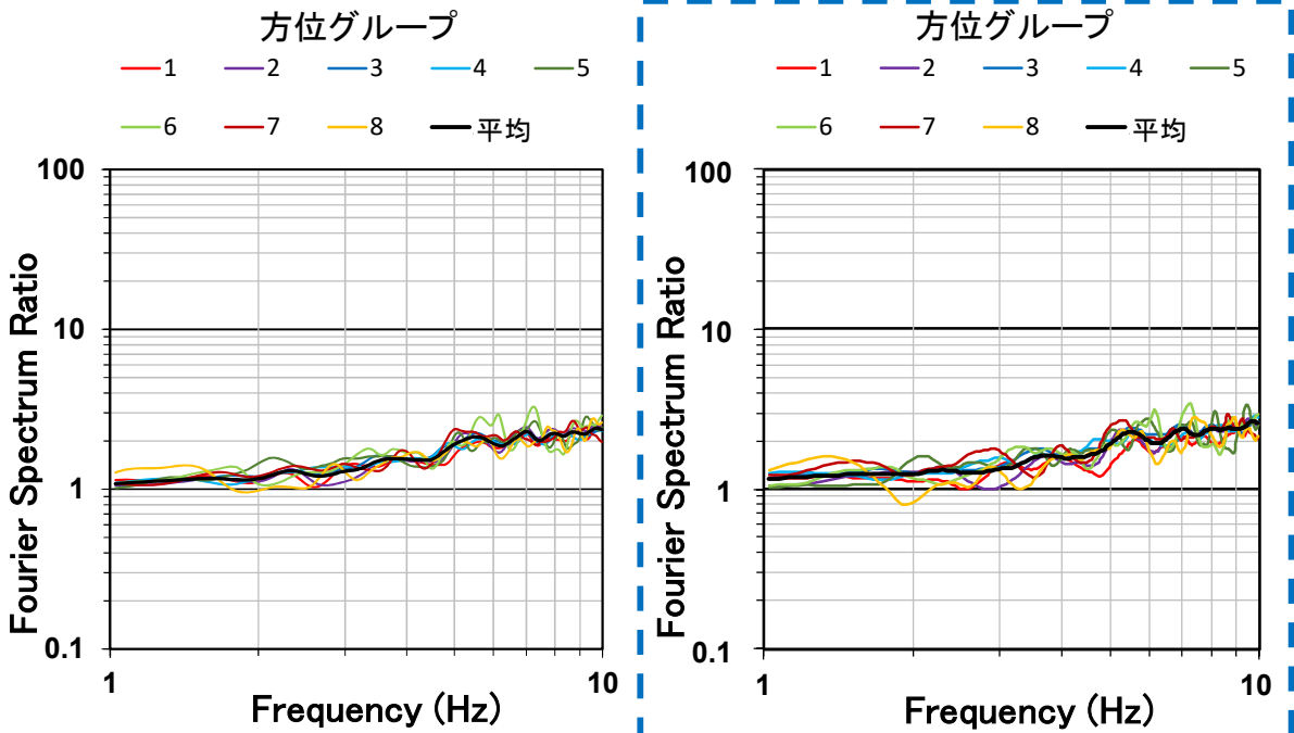
方位グループごとの平均基準化スペクトル (P.3-13に示すNo.5観測点における評価※)
