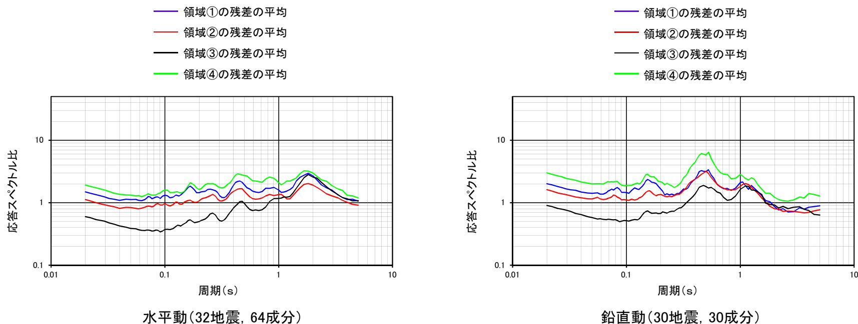
到来方向別の応答スペクトル比(残差)の平均値の比較
