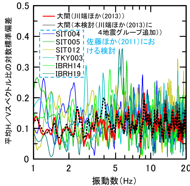
(b) 関東平野外縁部の観測点 (■●) との比較 (地下構造の不整形性が大きい観測点)
