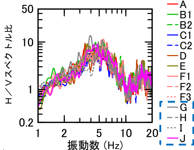
(b) 平均H/Vスペクトル比の比較
