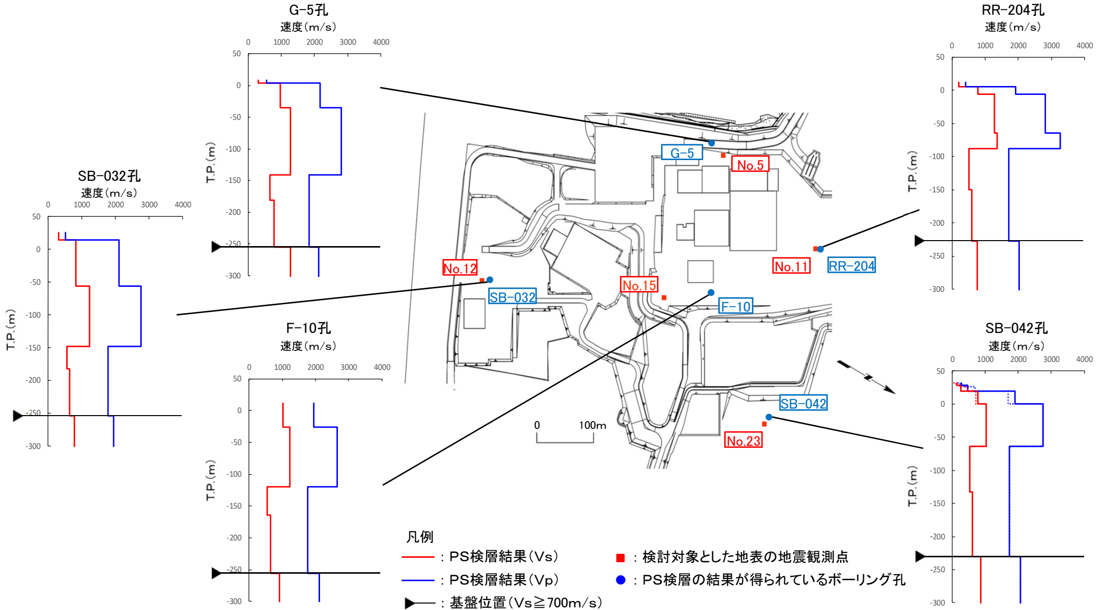
検討対象とした観測点付近のPS検層結果
