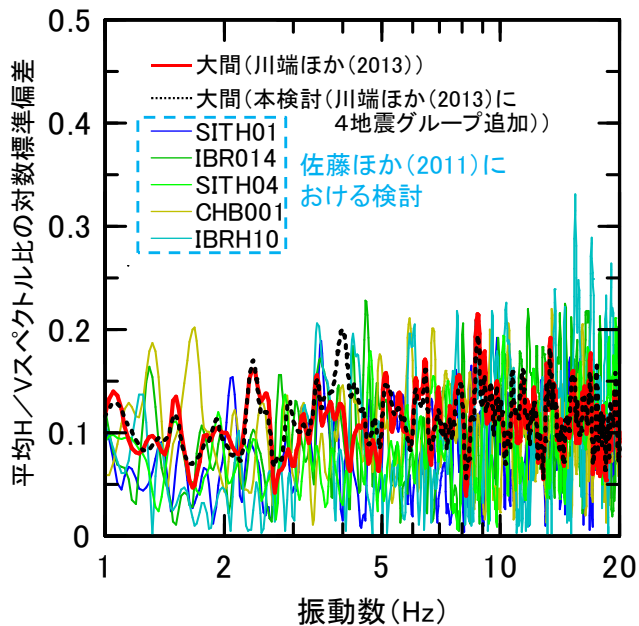
(a) 関東平野中央部の観測点 (■●) との比較 (地下構造の不整形性が小さい観測点)
