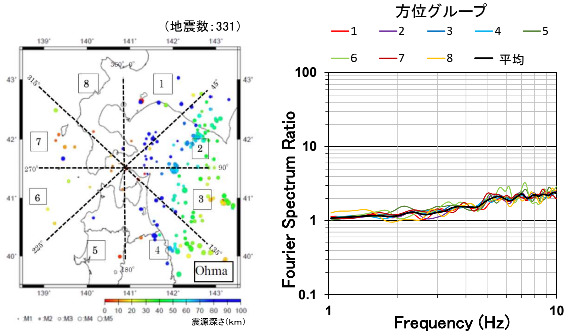
観測地震の震央分布及び方位グループ分け
