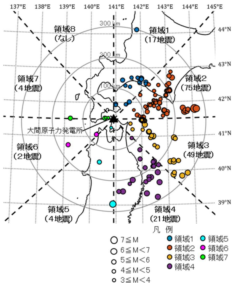
検討に用いた地震の震央分布
