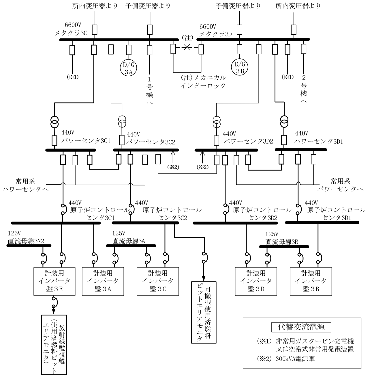
第1図 エリアモニタリング設備の概略電源系統図
