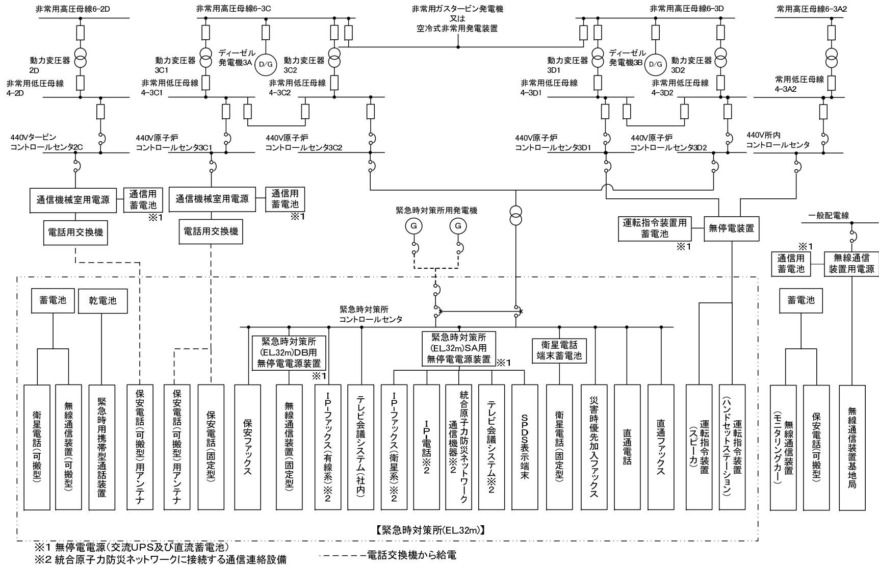
第1図 通信連絡設備の電源概略構成図(1/2)
