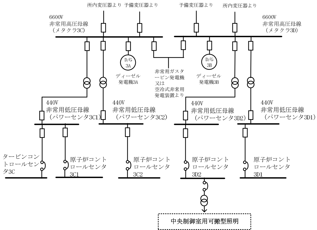
第1図 中央制御室用照明電源系統図
