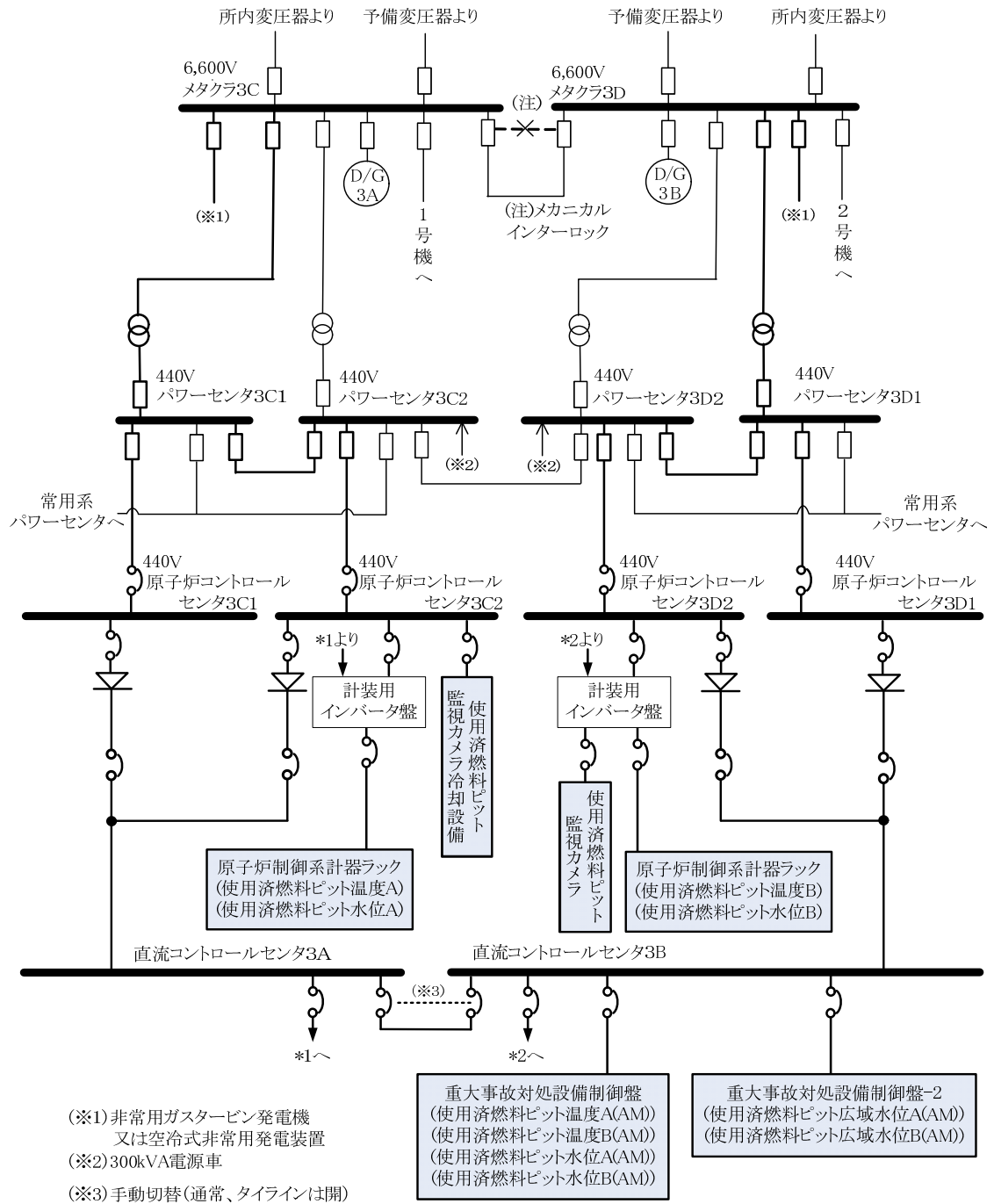
第1図 使用済燃料貯蔵槽の温度及び水位等を監視する装置の概略電源系統図
