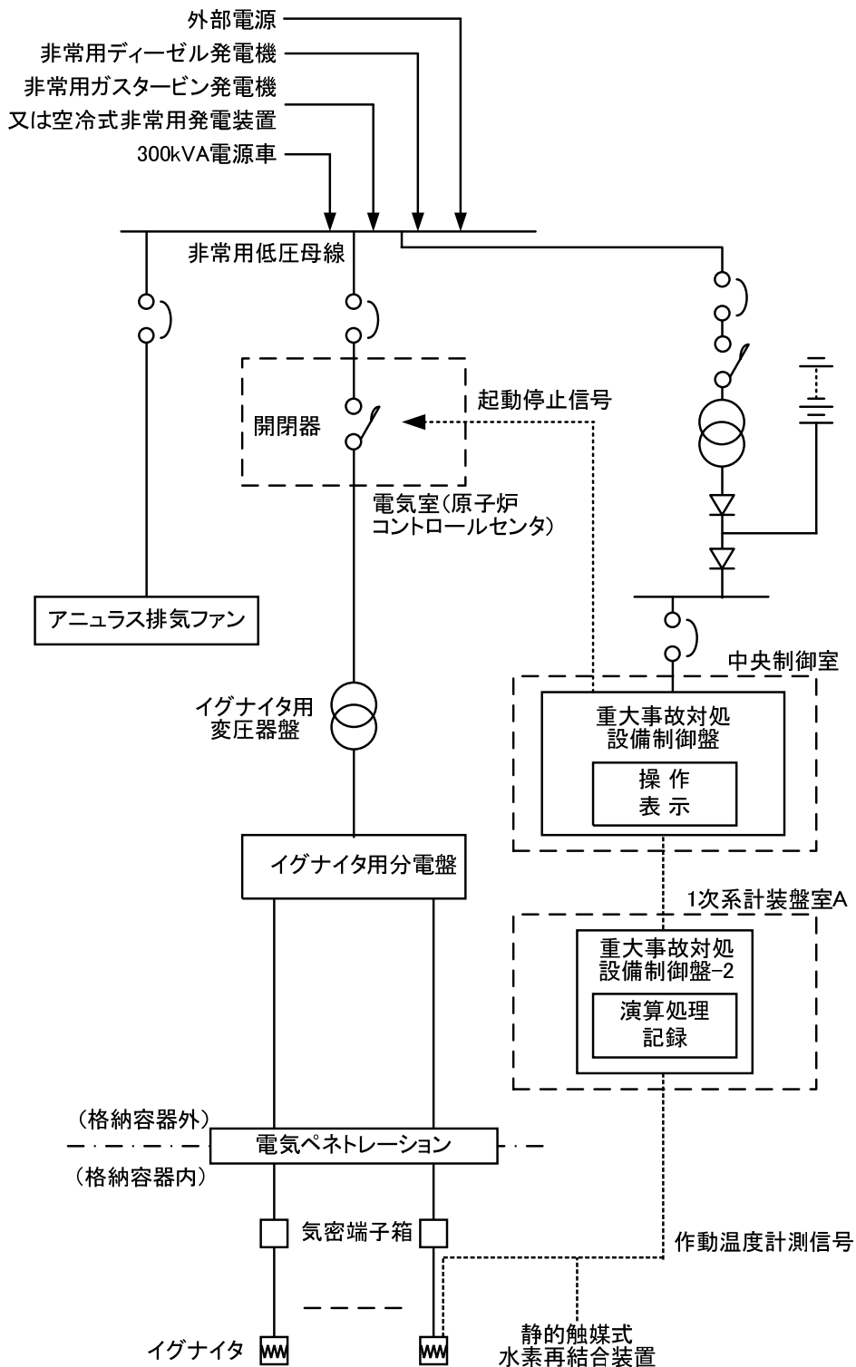
第1図 電源系統構成図
