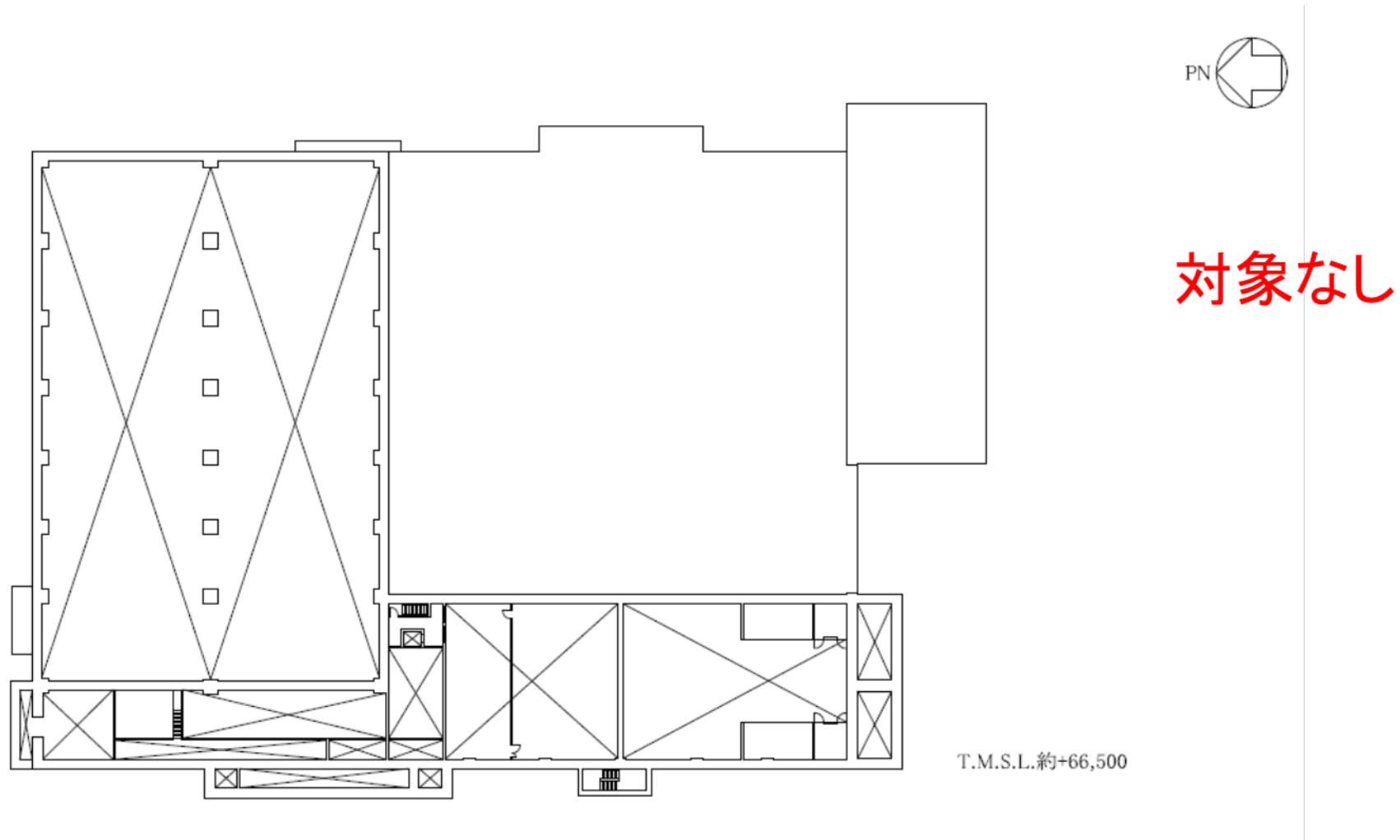
第 16 図 使用済燃料受入れ・貯蔵建屋の使用済燃料貯蔵槽の冷却等のための設備の機器配置概要図（地上 3 階）
