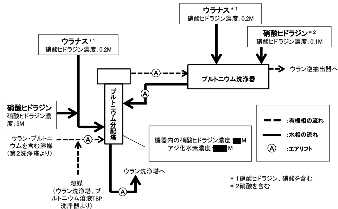
図 3：分配設備のプルトニウム分配塔の系統概要及びアジ化水素濃度
