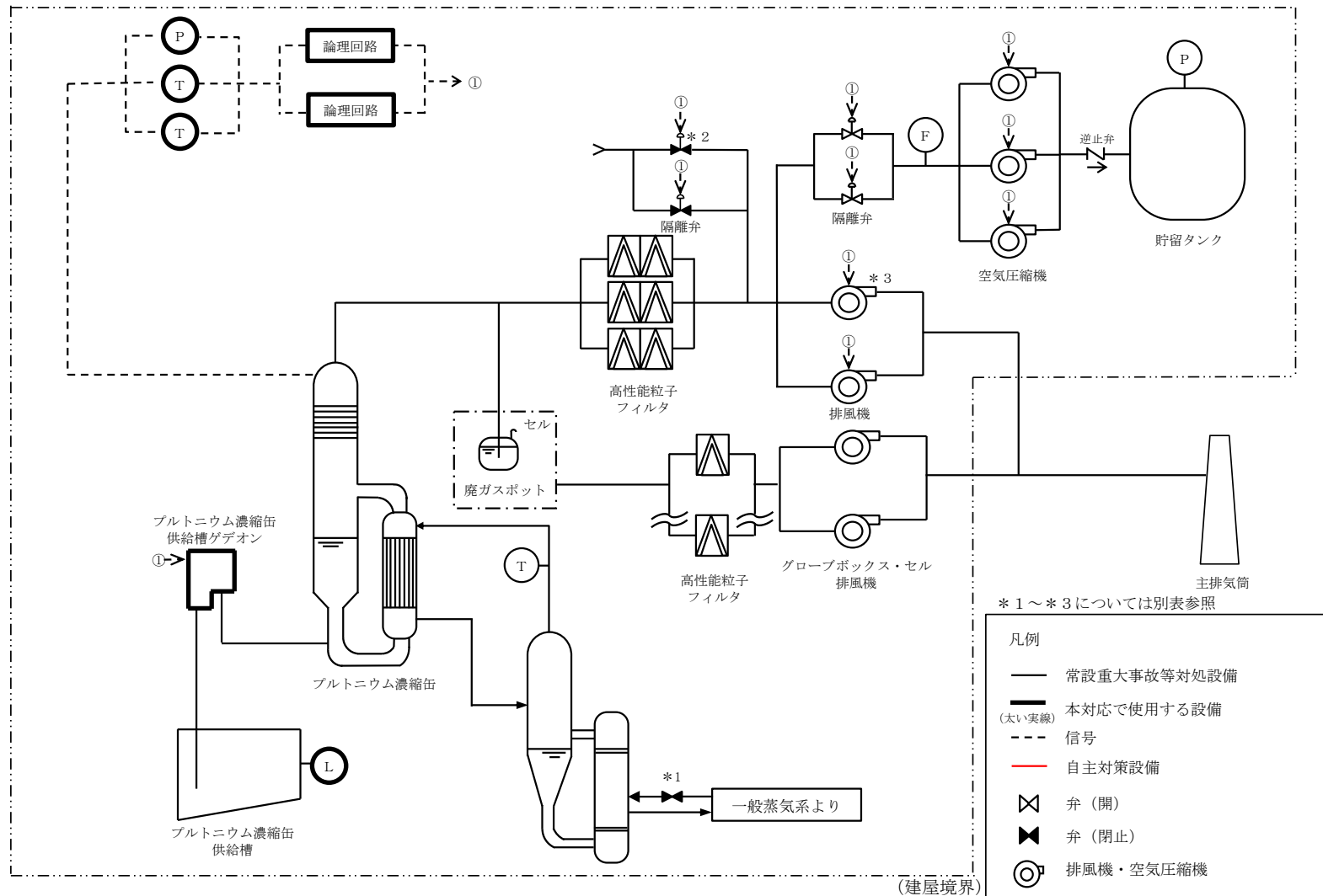
第2図 精製建屋 TBP等の錯体の急激な分解反応に対処するための設備の系統概要図 (プルトニウム濃縮缶への供給停止)
