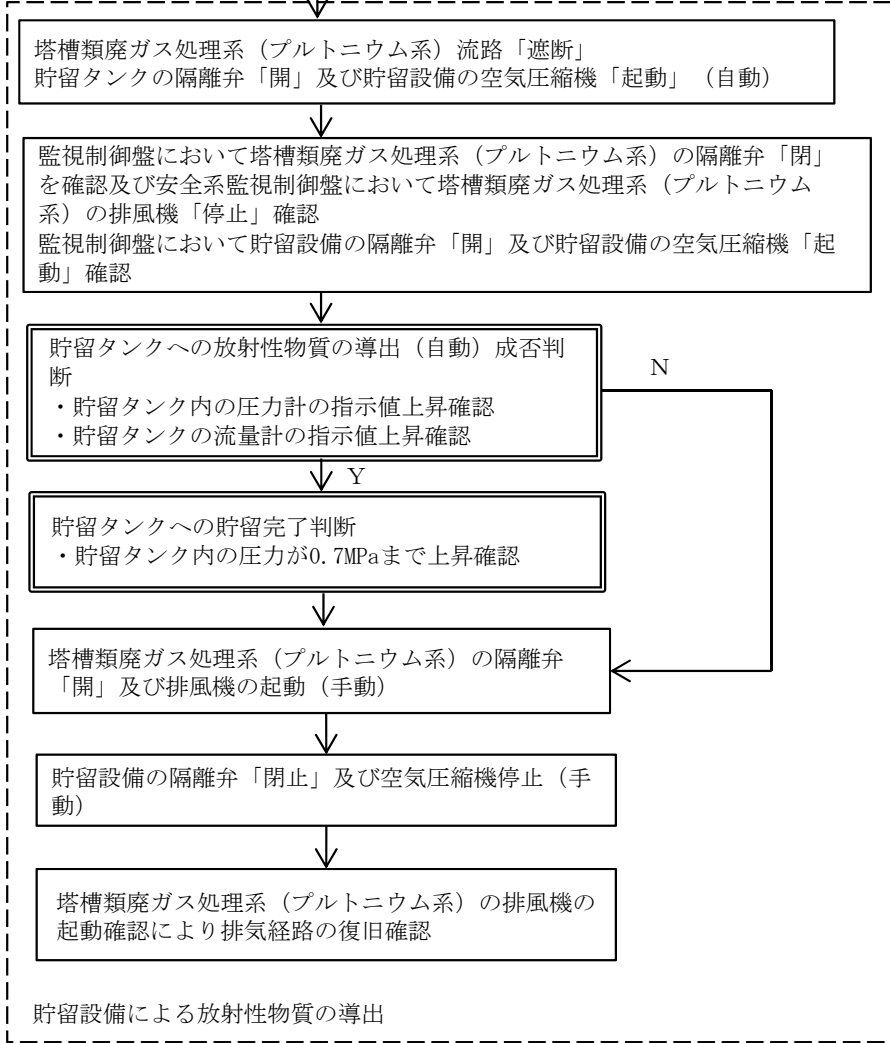
第10.1.1-2 図 「精製建屋におけるプルトニウム精製設備のプルトニウム濃縮缶のTBP等の錯体の急激な分解反応」 の手順の概要
