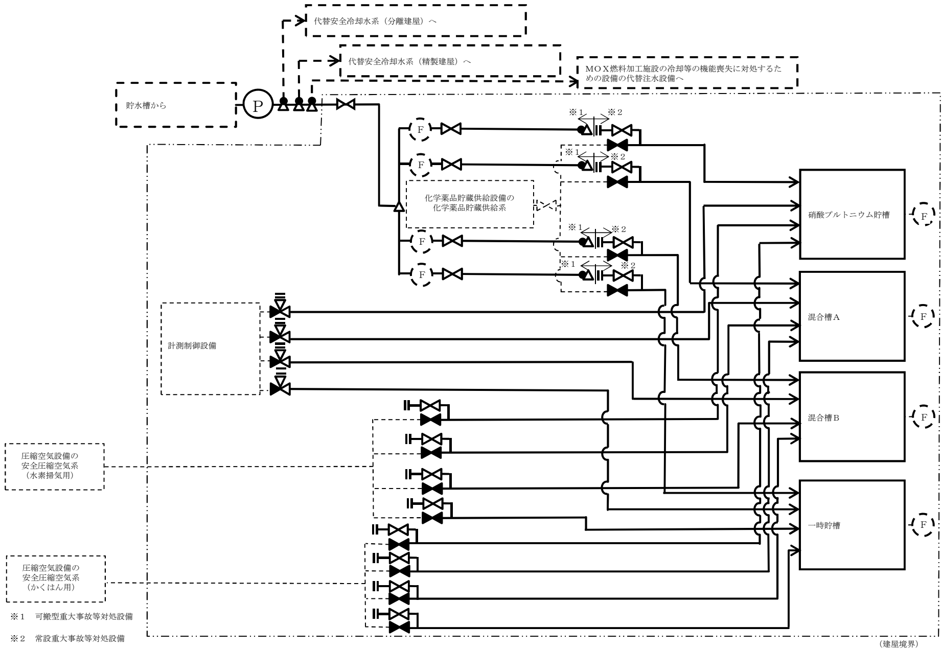
第1.2-29図 ウラン・プルトニウム混合脱硝建屋の貯水槽から機器への注水の系統概要図
