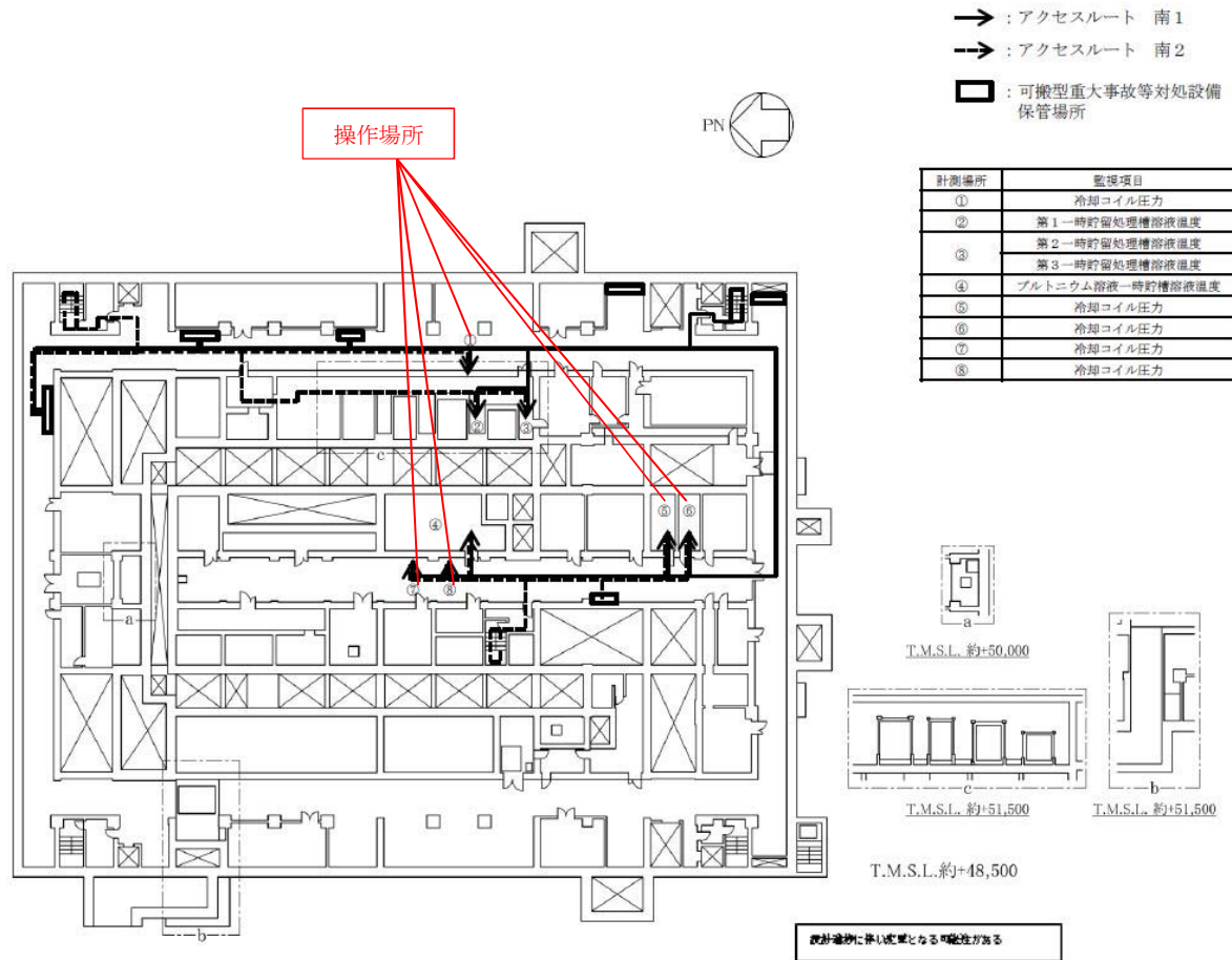
精製建屋 蒸発乾固の拡大の防止のための措置のアクセスルート（地下1階）（冷却コイル通水による冷却）
