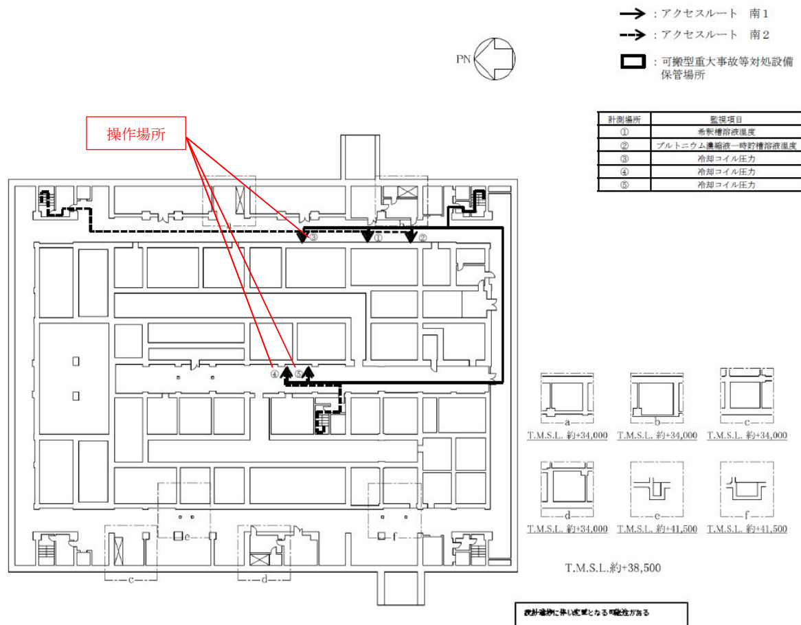
精製建屋 蒸発乾固の拡大の防止のための措置のアクセスルート（地下3階）（冷却コイル通水による冷却）
