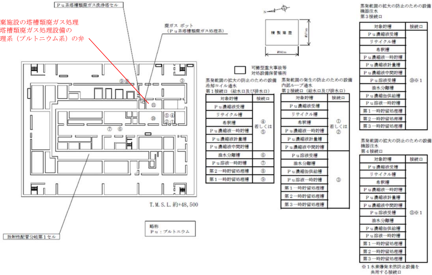
精製建屋 蒸発乾固の拡大の防止のための措置の機器配置概要図 (地下1階) (放出低減対策)
