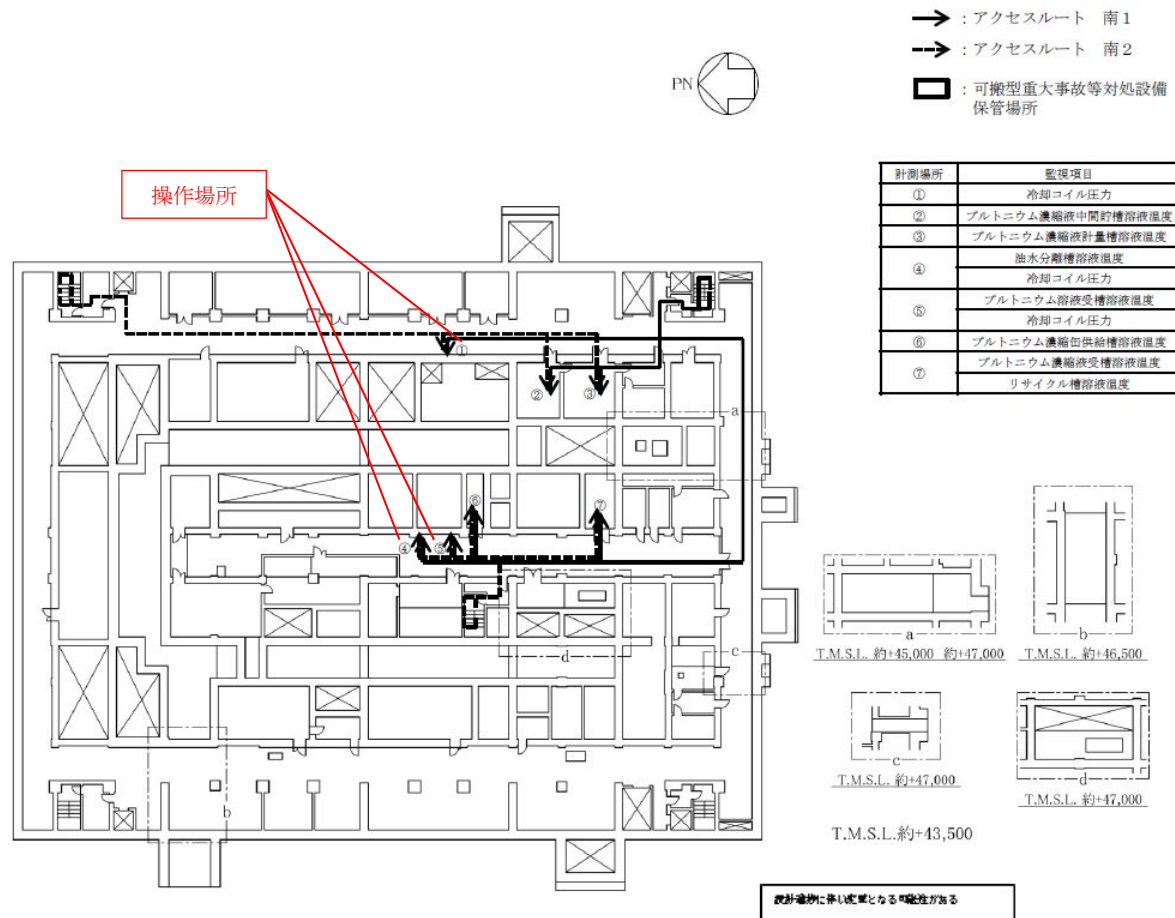
精製建屋 蒸発乾固の拡大の防止のための措置のアクセスルート（地下2階）（冷却コイル通水による冷却）
