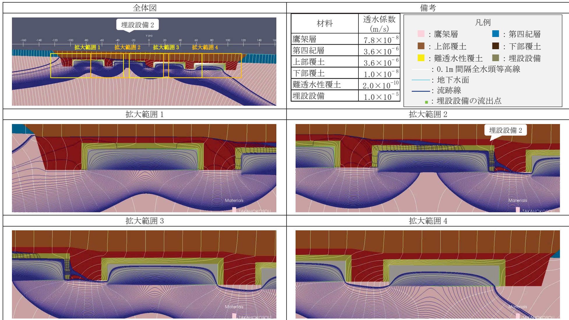
第5図 2次元地下水浸透流解析結果【2号廃棄物埋設地】(基本設定 1,000年後) (3/5) <埋設設備2の流出点を通る流跡線>
