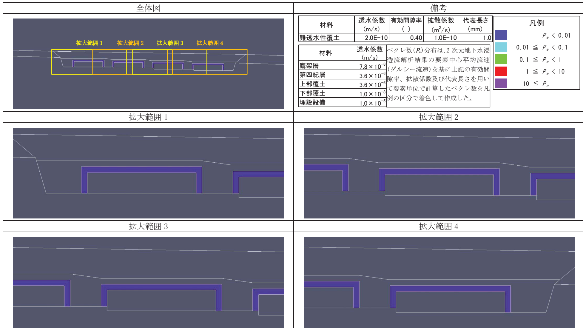
図 難透水性覆土内のペクレ数( P_e )分布(5/6)【2号廃棄物埋設地】(基本設定 1,000年後)
