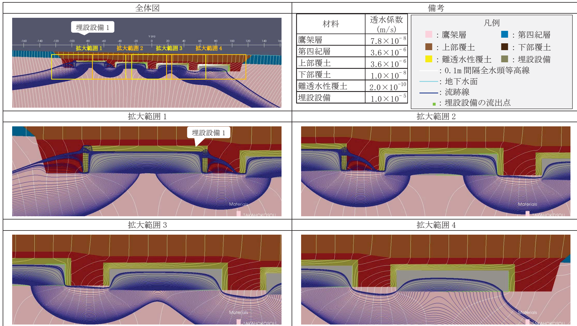
第 5 図 2 次元地下水浸透流解析結果【2 号廃棄物埋設地】(基本設定 1,000 年後) (2/5) <埋設設備 1 の流出点を通る流跡線>
